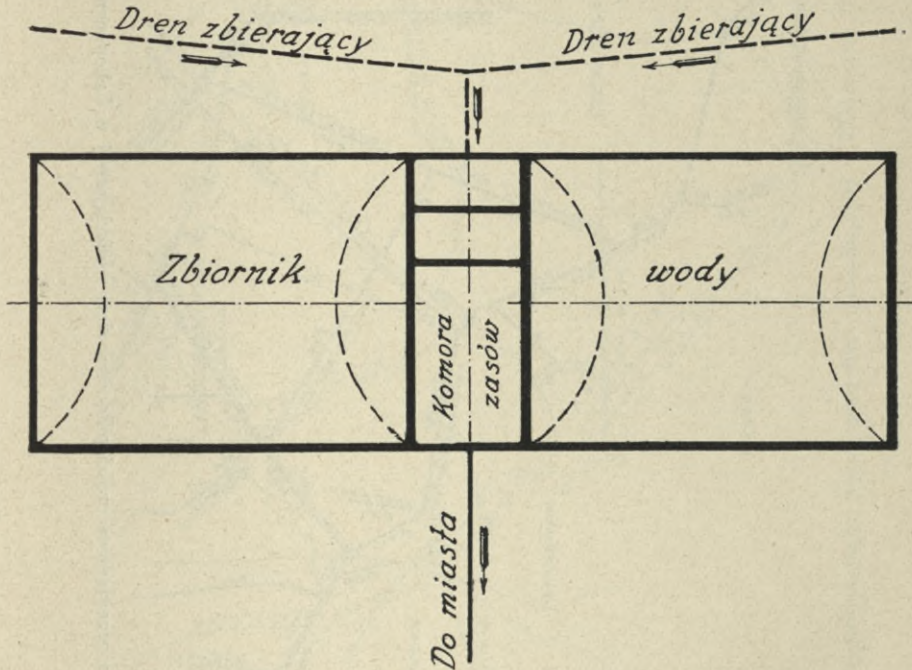
Ryc. 38. Sytuacja zbiornika wody w Makowie.
