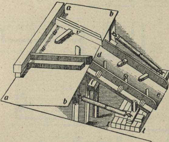
Ryc. 83. Polska przepławka ruchoma dla ryb.
