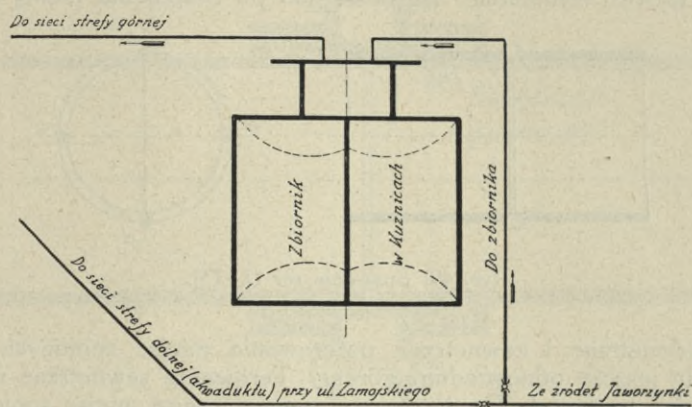
Ryc. 48. Odgałęzienie rurociągu z Jaworzynki do zbiornika w Kuźnicach.
