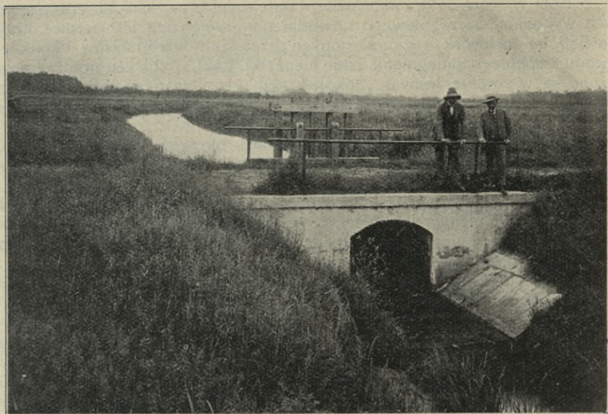
Ryc. 30. Widok uregulowanego potoku Blizna z przepustem betonowym i zastawką drewnianą.
