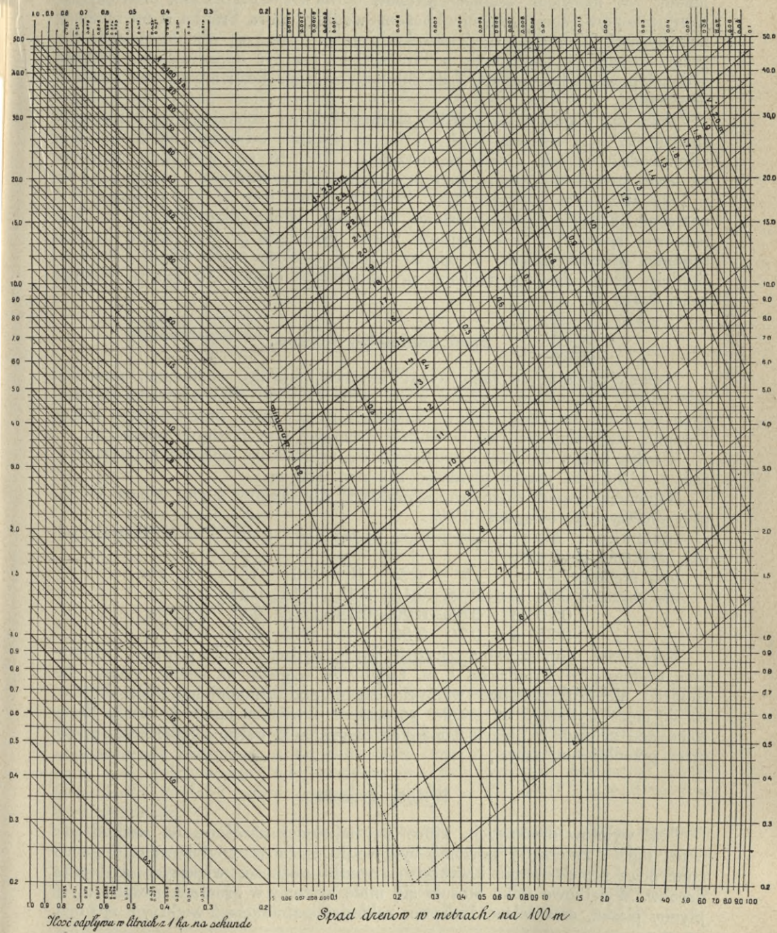
Ryc. 2. Diagram prof. Tadeusza Sikorskiego do oznaczenia średnicy rurek drenowych i chyżości wody przepływającej w drenach.
