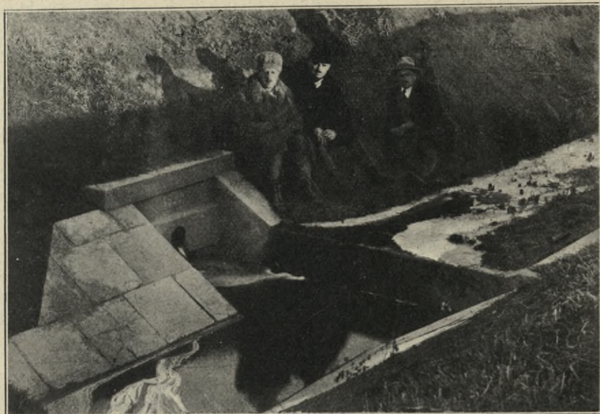
Ryc. 4. Widok stopnia na rowie i wylotu drenowego w gminie Długie (Pierwszy z lewej strony kierownik ekspozytury biura meljoracyjnego T. W. S. w Jaśle, inż. Tytus Piller).
