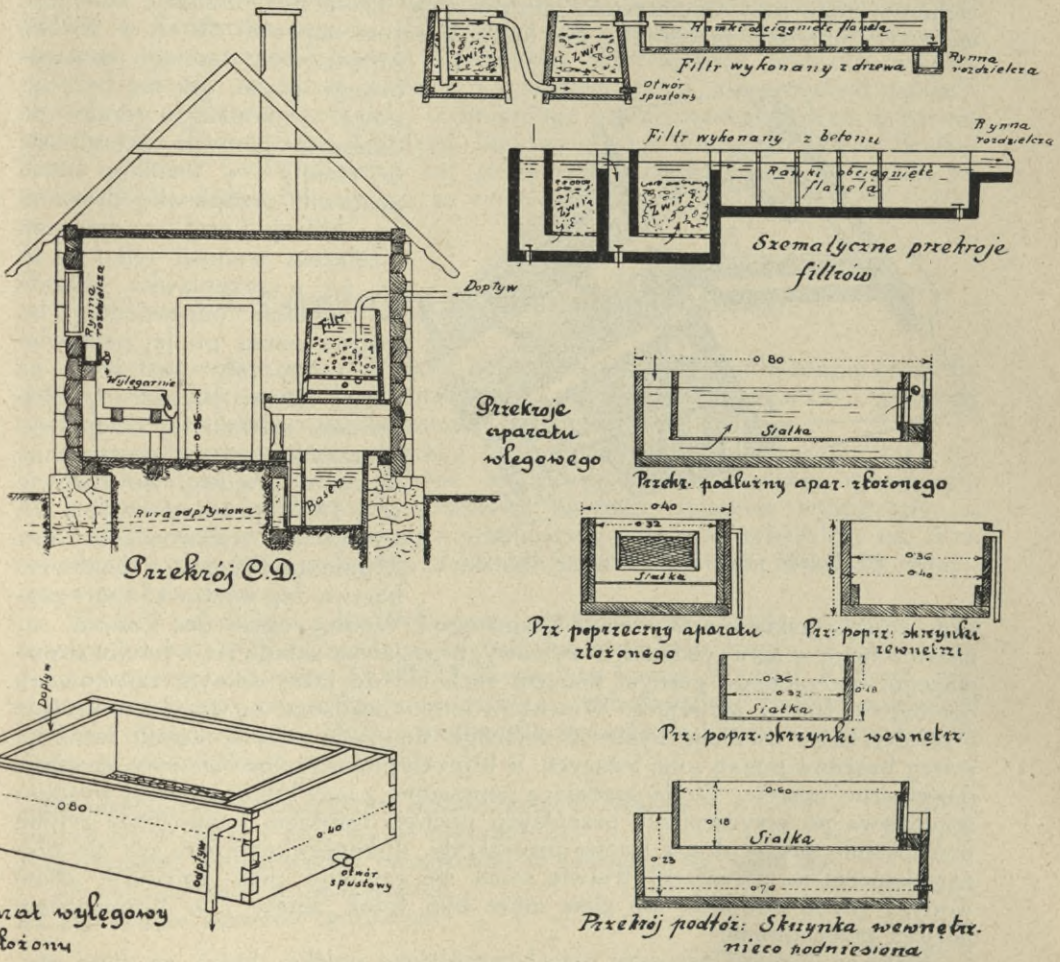
Ryc. 82. Przekrój poprzeczny wylegarni (1 : 100) i przyrządy wylegowe (1 : 20).
