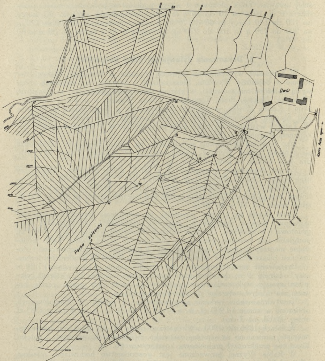
Ryc. 6. Sytuacja pola wydrenowanego w Rabin Wyżnej (1 : 7.200).
