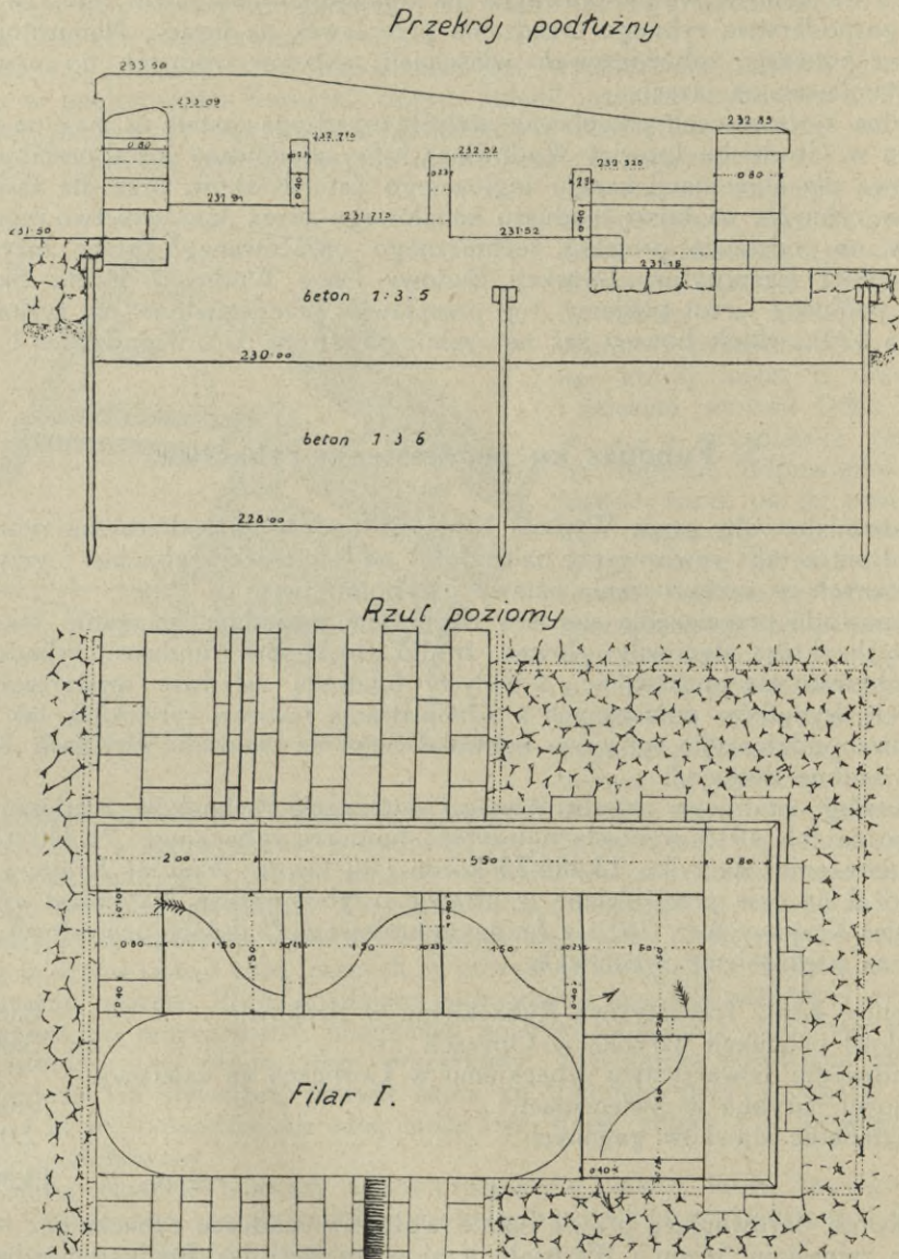
Ryc. 84. Przepławka stała na jazie na rzece Skawie w Grodzisku (1 : 100).
