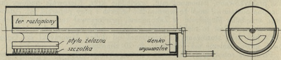
Ryc. 50. Terowanie wewnętrzne spojeń rur (1:15).
