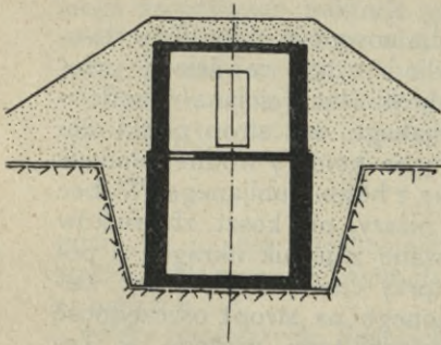
Przekrój poprzeczny
