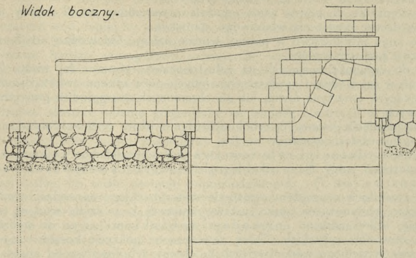
Ryc. 85. Przeplawka stała na jazie na rzece Skawie w Grodzisku (1 : 100).
