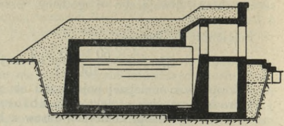
Przekrój podłużny
