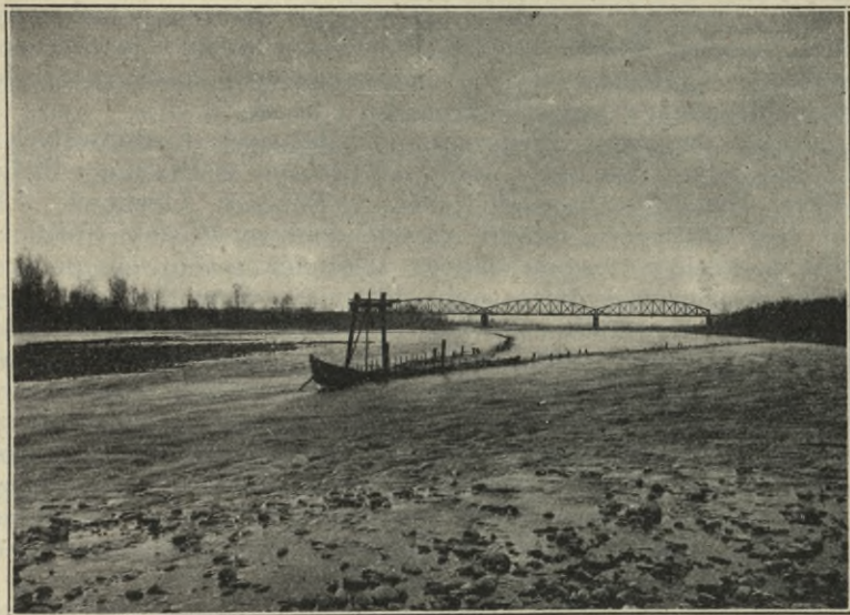
Ryc. 77. Widok laski (samolówki) na Dunajcu powyżej Nowego Sącza.
