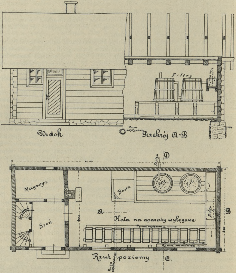
Ryc. 81. Widok, przekrój podłużny i rzut poziomy wylęgarni (1 : 100).
