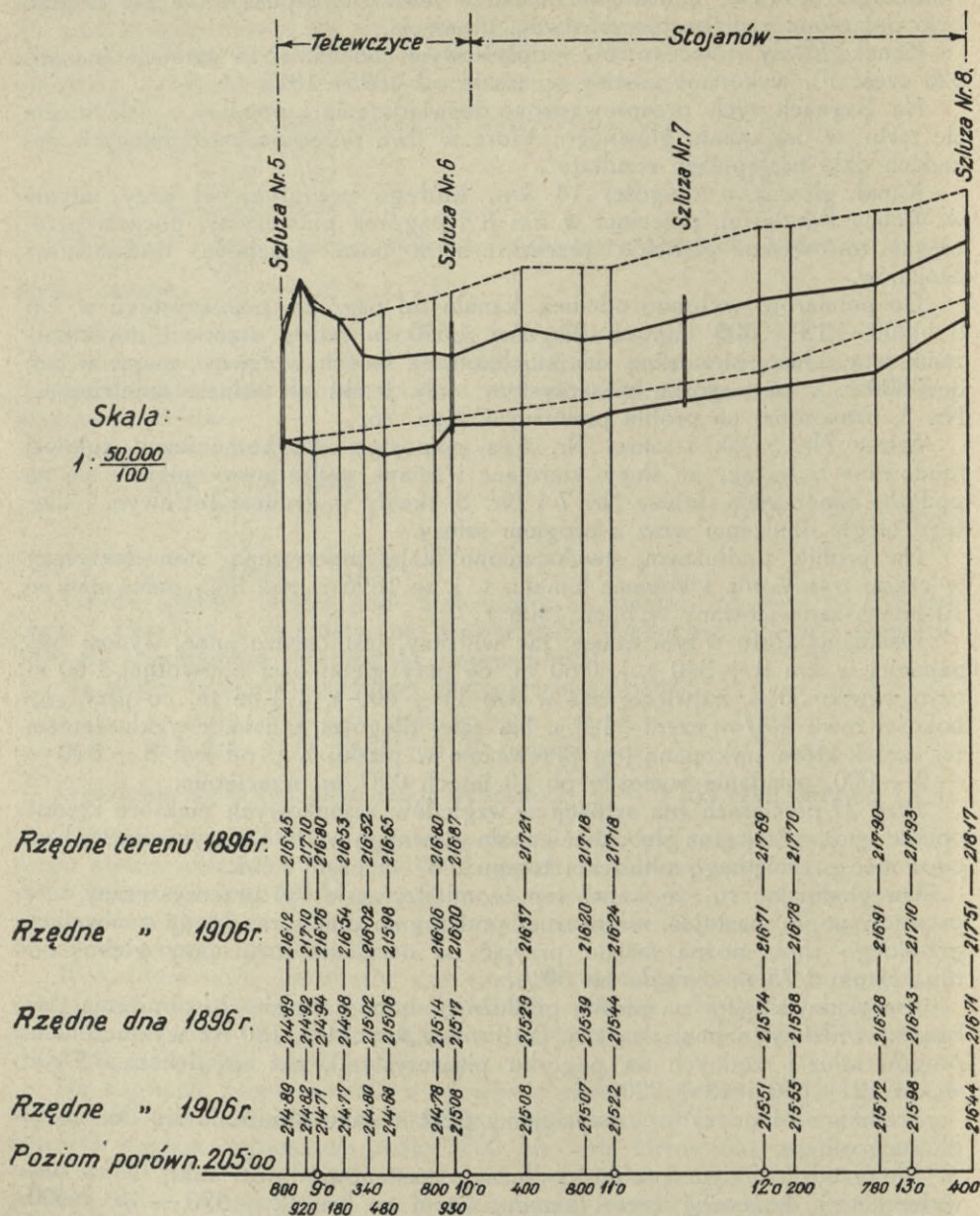
Ryc. 26. Profil podłużny głównego kanału osuszającego na bagnach Stojanowskich.
