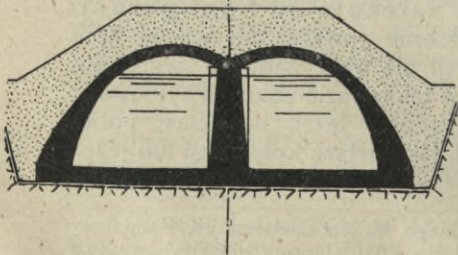
Przekrój poprzeczny
