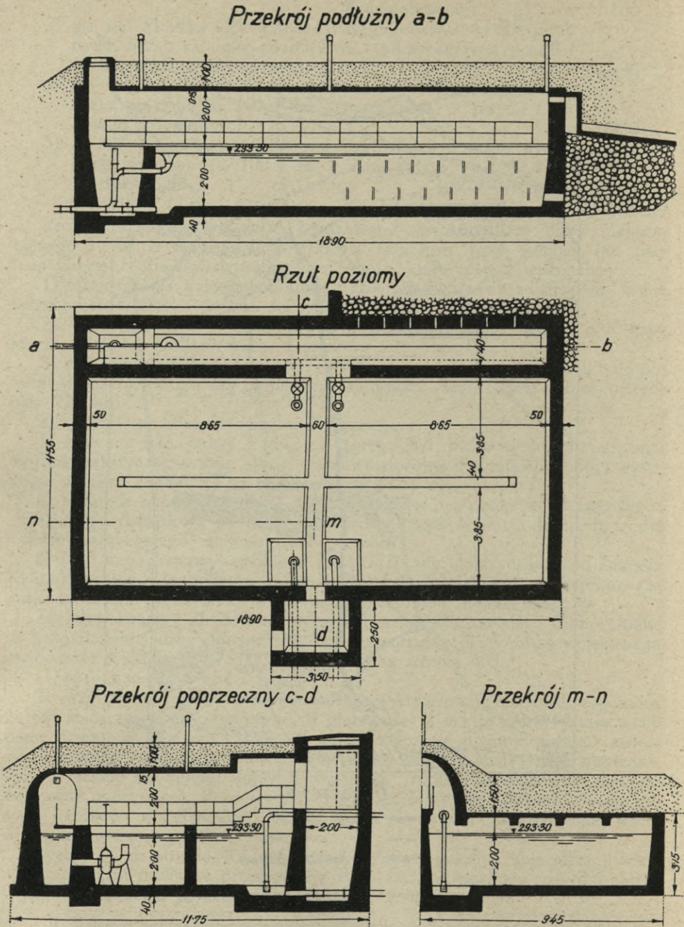
Ryc. 60. Ujęcie źródła i zbiornik w Maliczkowicach (1 : 200).
