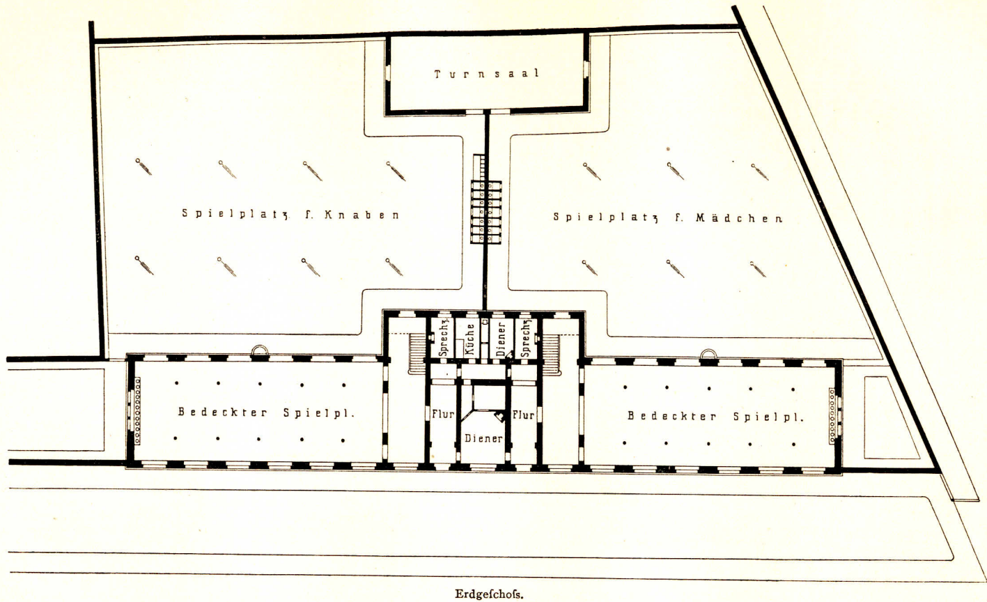
14klassige Schule für Knaben und Mädchen zu Saint-Mandé (Seine) .
