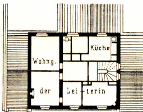
Obergeschoss.
