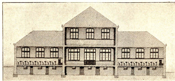
Längenschnitt.
