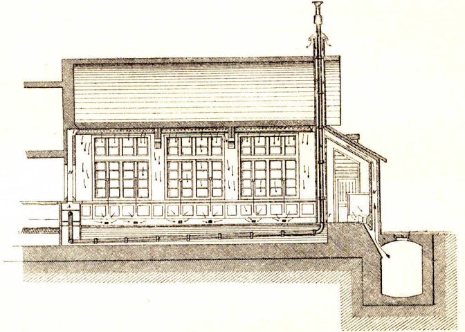
Längenschnitt.
