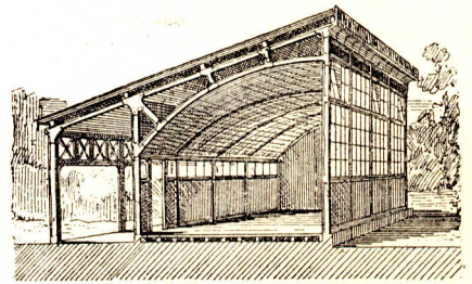
Querschnitt des Schulzimmers nach André .
