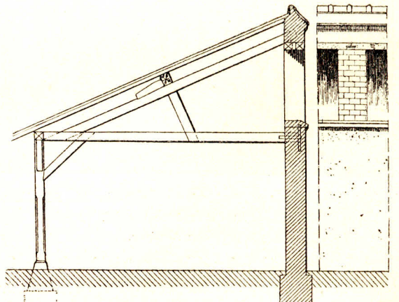
Einzelheit des bedeckten Spielplatzes der Volksschule zu Neuville aux Bois . \frac{1}{100} w. Gr.
