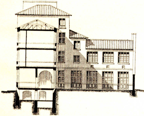
Querschnitt durch das Klaffengebäude für Knaben.
