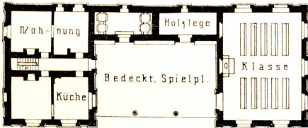
Grundriss.
