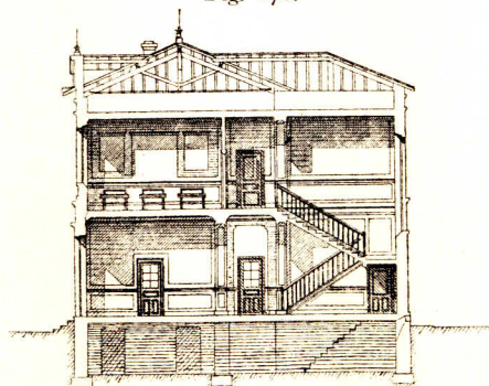
Querschnitt durch die Mitte.
