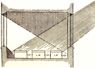
Zweifseitige Beleuchtung. 1/200 w. Gr.
