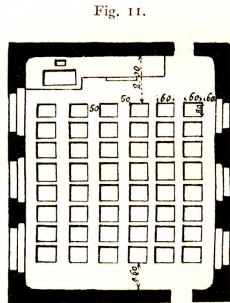
Lehrzimmer mit einfitzigem Gefühl.
