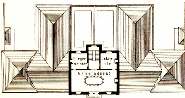
Obergechoß.
