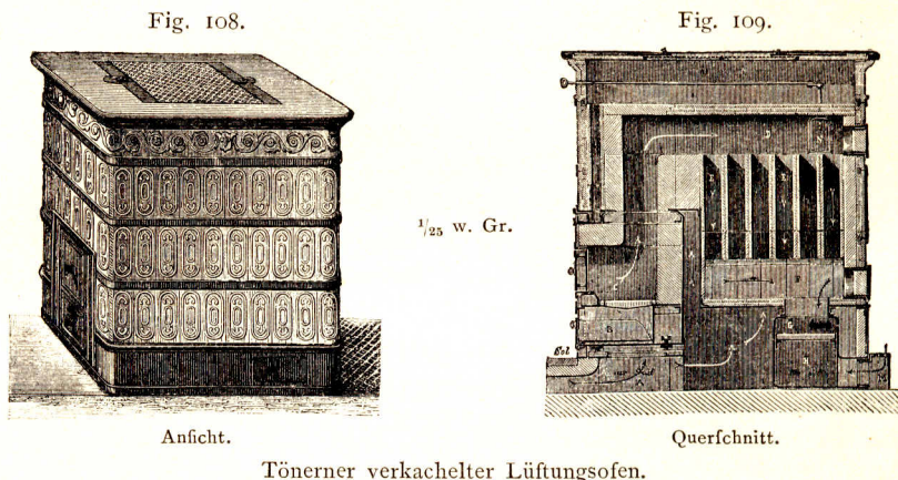
Tönerne verkachelte Lüftungsöfen.
