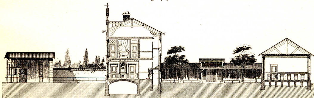
Querschnitt durch die Mitte. — \frac{1}{375} w. Gr.
