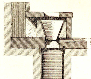
Einzelheit des Lehrer-Sitzabortes. \frac{1}{25} w. Gr.
