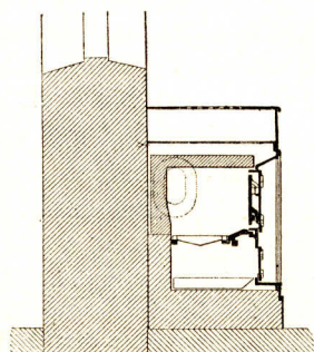
Schnitt durch den Ofen.
