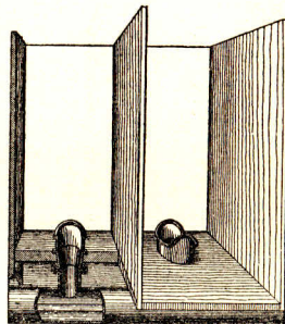
Hockaborteanlage nach Mangenot .
