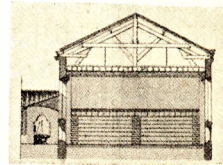
Schnitt durch den Beschäftigungssaal.
