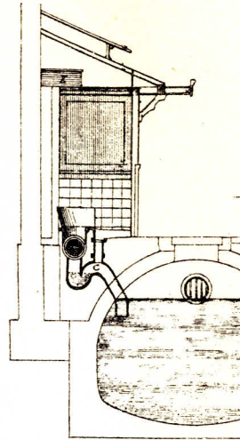
Querschnitt.
