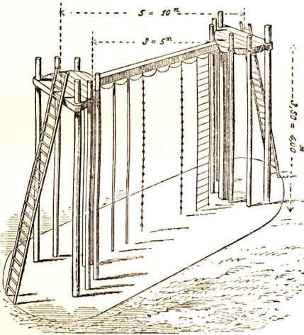
Turngerüst.
