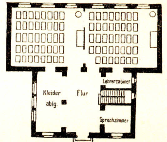
Erdgeschoß einer zweiklassigen Volksschule nach Narjoux . \frac{1}{600} w. Gr.
