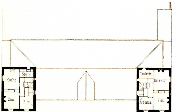
Zweiklassige Knabenschule zu Villeneuve-de-Marc (Ijère).
