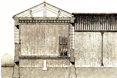
Schnitt durch das Klassengebäude.
