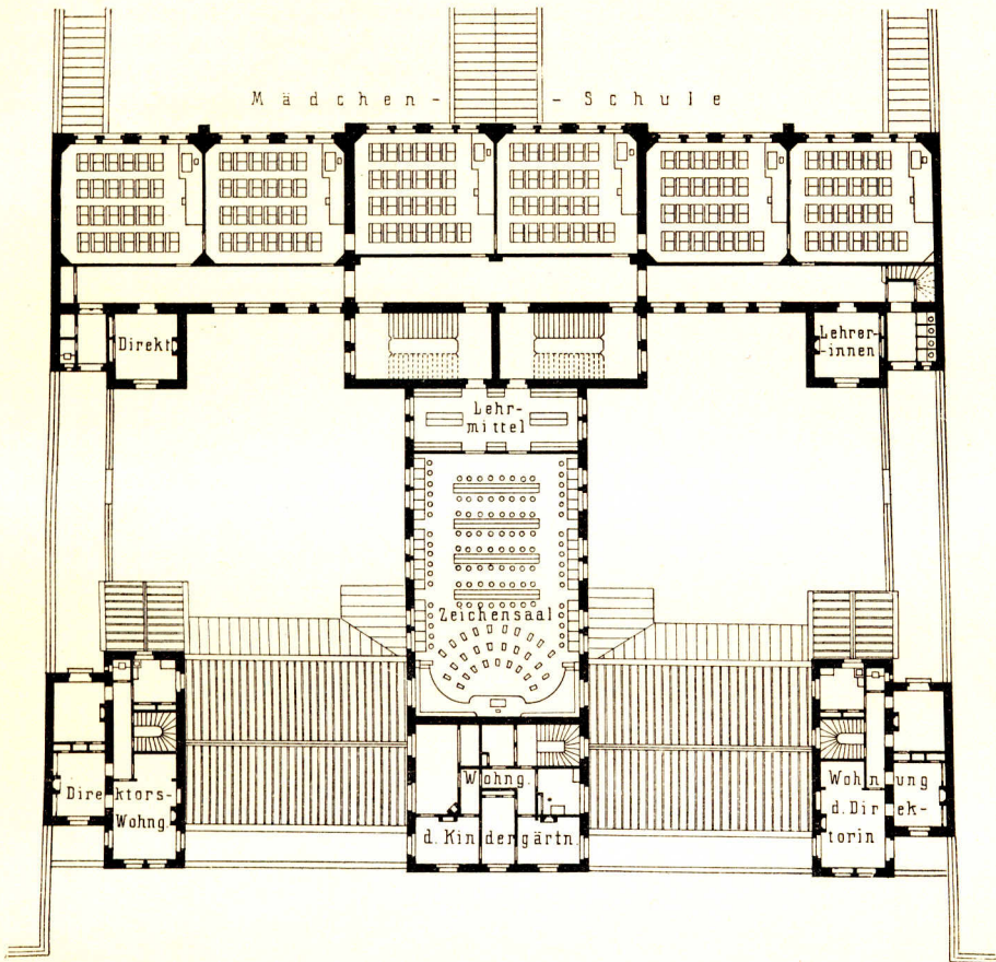
I. Obergeschoss.
