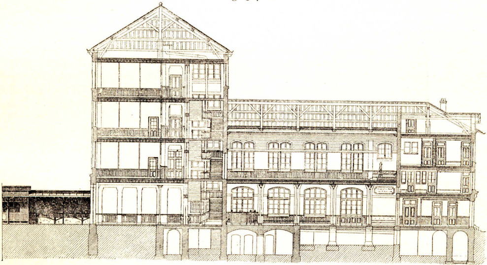
Querschnitt durch die Mitte.
