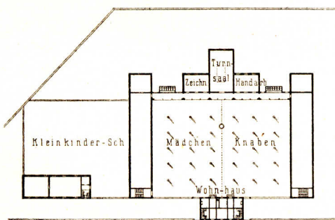
Erdgefchoß.
