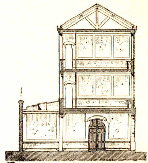
Querschnitt durch die Knabenschule.
