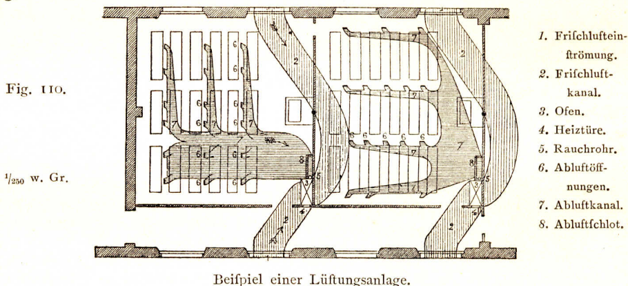
Beispiel einer Lüftungsanlage.
