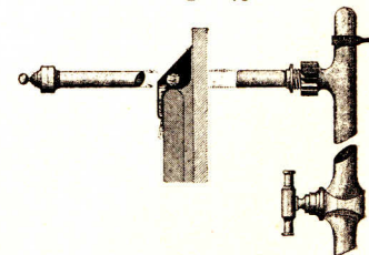
Einzelheit der Rohrleitung zur Piffoirspülung. — \frac{1}{10} w. Gr.
