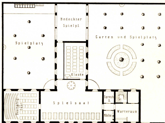
Musterplan einer städtischen Kleinkinderchule für 150 Kinder.
