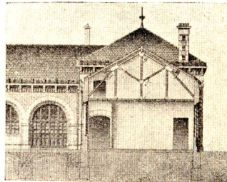
Querschnitt durch das Klassen-gebäude.
