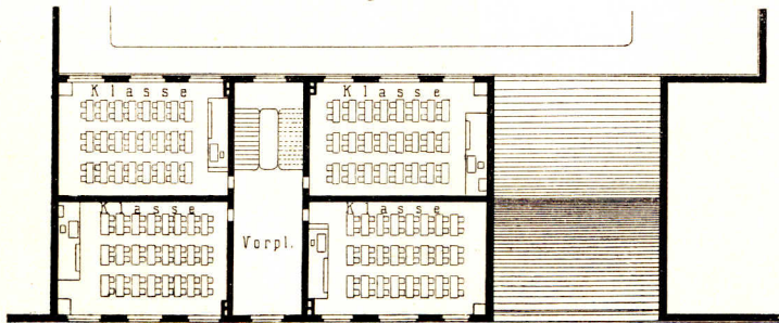
Obergeschoss. — 1/500 w. Gr.
