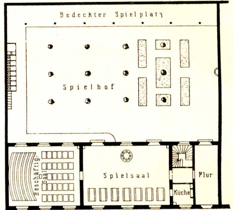
Musterplan einer Kleinkinderchule für 100 Kinder nach Narjoux .
