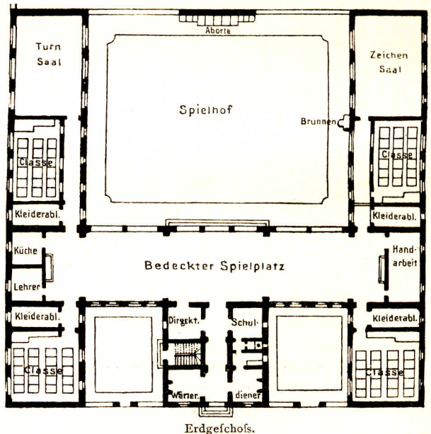
Musterplan einer vierklaffigen Volksschule.
