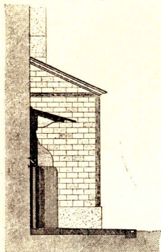
Querschnitt durch einen Pissstand.
