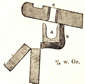
Einzelheit des Tinten- fasses nach Lemel .
