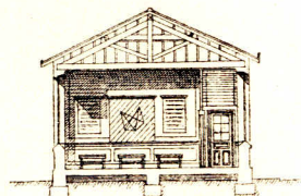
Querschnitt durch eine einseitig beleuchtete Klasse.
