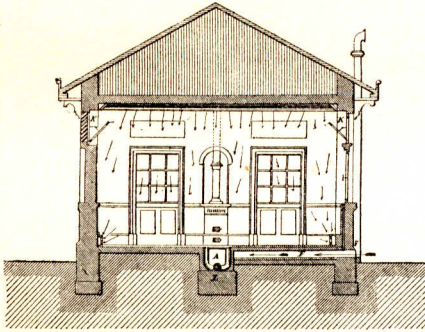
Querschnitt.
