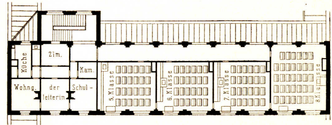
II. Obergehoßs der Mädchenfchule.
