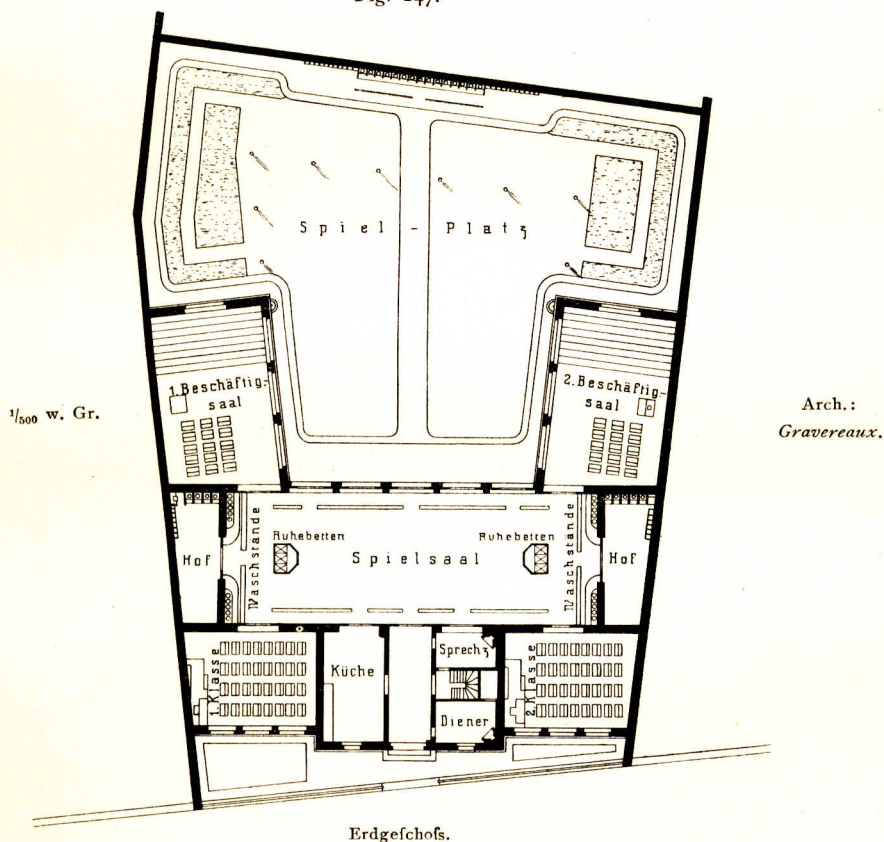
Kleinkinderchule zu Charenton.
