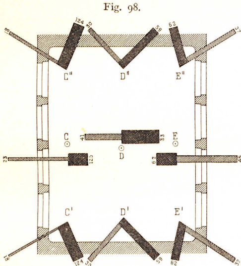
Graphische Darstellung der Licht- und Schattenstärken bei zweifseitiger ungleicher Beleuchtung.
