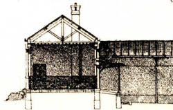
Querschnitt durch das Klassengebäude.
