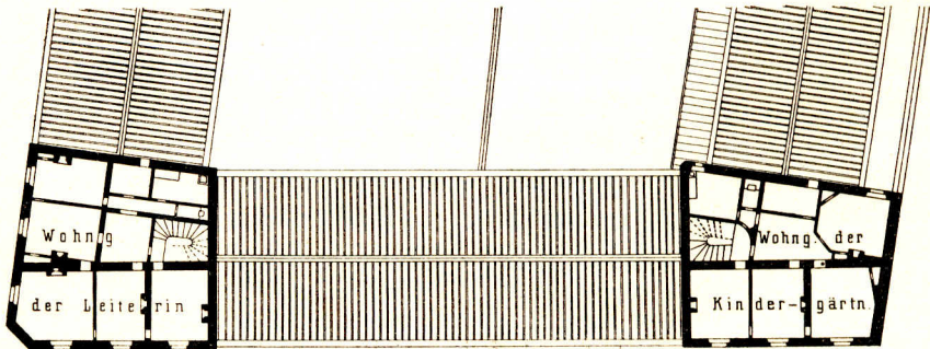
Obergeschoss.
