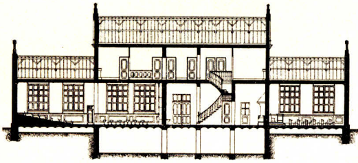
Längenschnitt.
