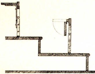
Schnitt.
