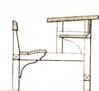
Querschnitt der kleinsten Nummer I.
