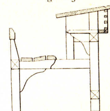
Querschnitt der Type Nummer III.
