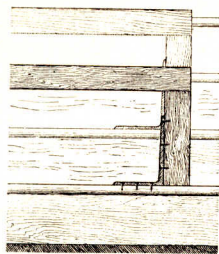
Ansicht.
