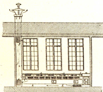
Schnitt.
