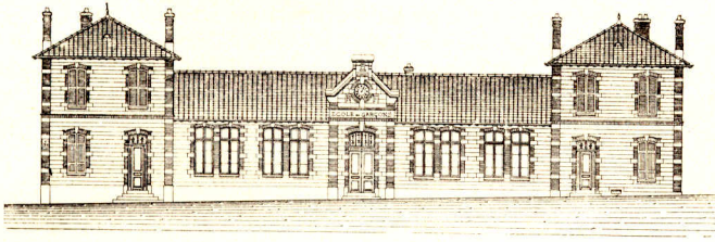
Hauptanicht.
