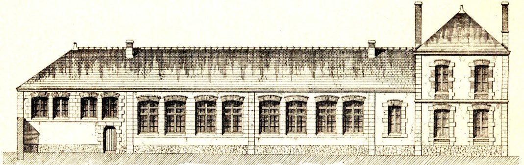
Ansicht gegen den Garten. — \frac{1}{300} w. Gr.
