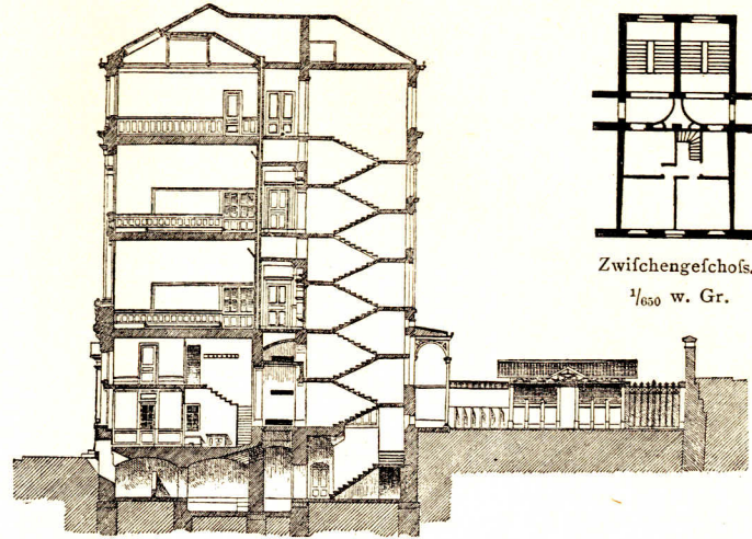
Querschnitt.
