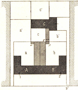
Lageplan der Schulhausgruppe zu Viroflay. 1/2000 w. Gr.
