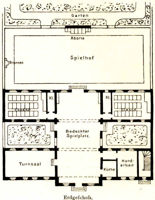
Musterplan einer zweiklaffigen Volksschule.
