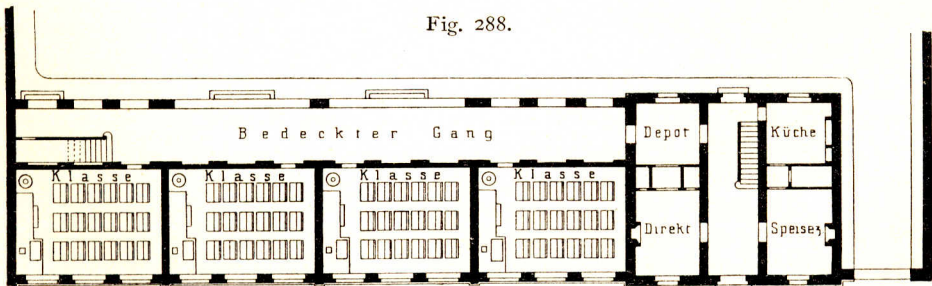
Obergeschoss.
