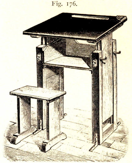
Gestühl nach Féret .
