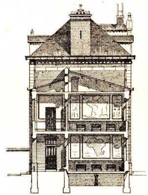
Querchnitt.
