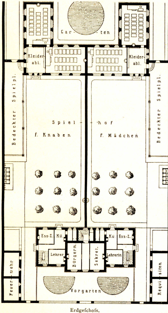
Vierklassige Knaben- und Mädchen-Schule nebst Gemeindeamt zu La Chapelle-St.-Mesmin (Loiret).
