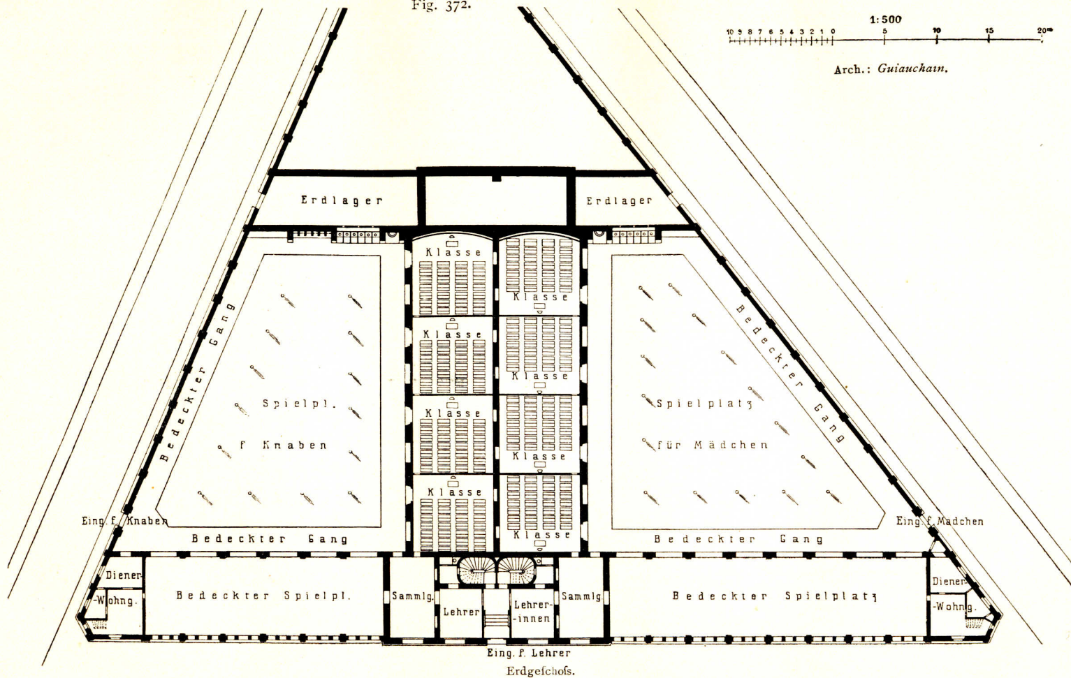
Schulhausgruppe zu Mustapha (Algier).
