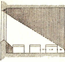
Einseitige Beleuchtung. 1/200 w. Gr.
