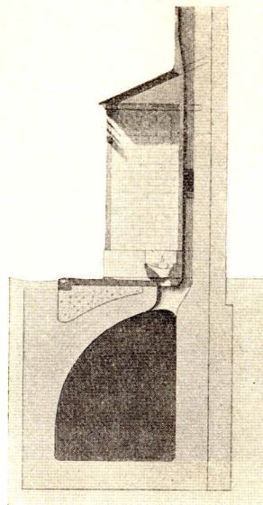
Querschnitt durch einen Abortraum.
