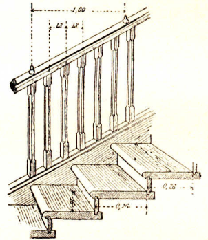
Treppengeländer.
