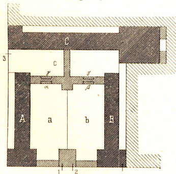
Lageplan der Schulhausgruppe zu Paris, Rue Lambert.
