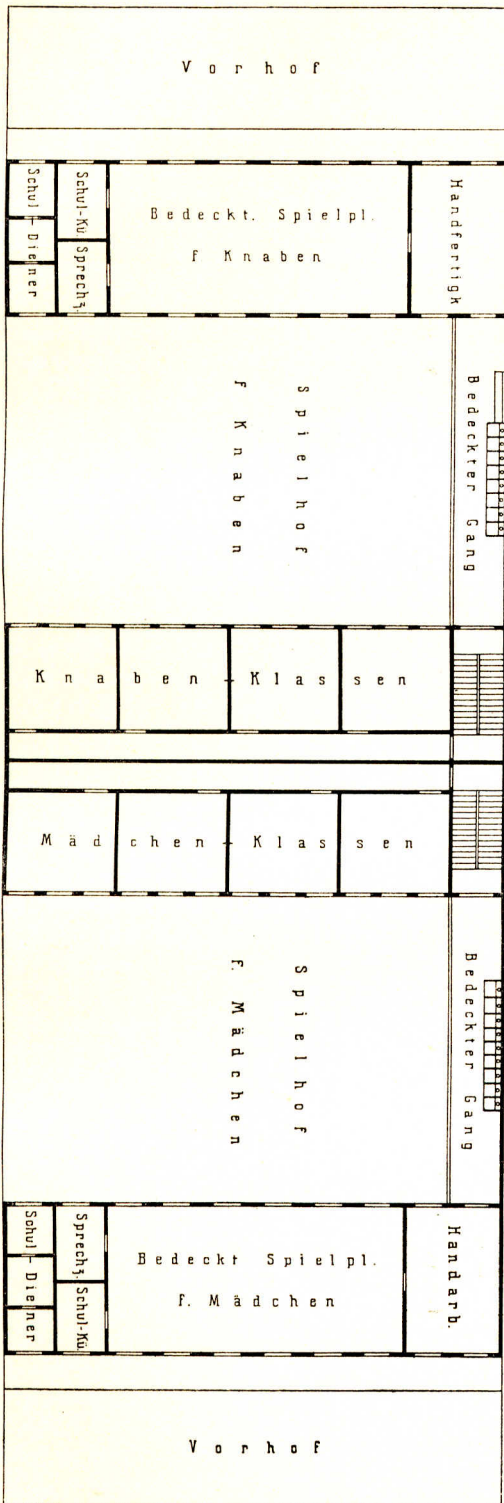
Grundriss der 14klassigen Schulbaracke zu Paris, Boulevard d'Enfer.
