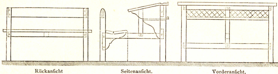
Gestühl nach Thiervoz . — \frac{1}{25} w. Gr.
