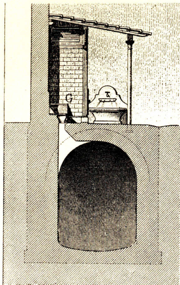
Querschnitt.
