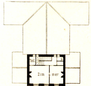
Obergeschoss.
