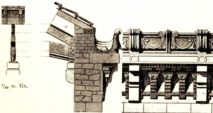
Querschnitt durch das Klassen-gebäude.
