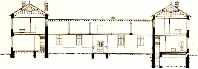
Längenschnitt.
