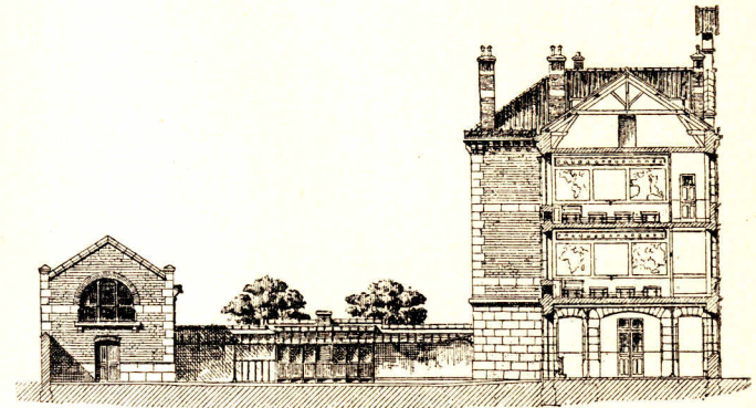
Querschnitt.
