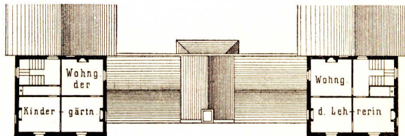
Obergeschoss.
