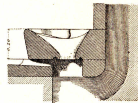
Einzelheit der Schüler-Hockaborte. — \frac{1}{25} w. Gr.
