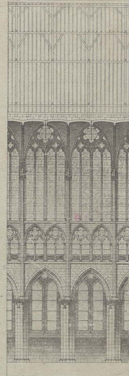
Elevation Intérieure
