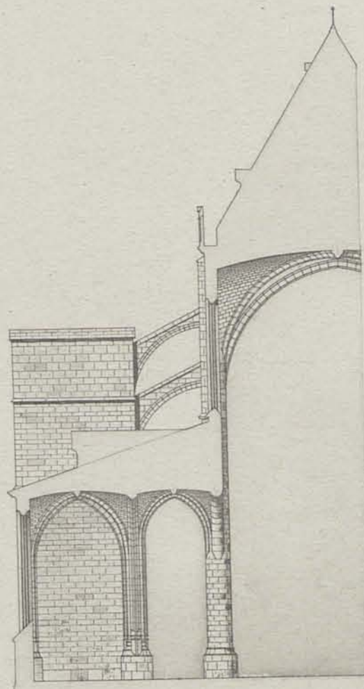
COUPE TRANSVERSALE
