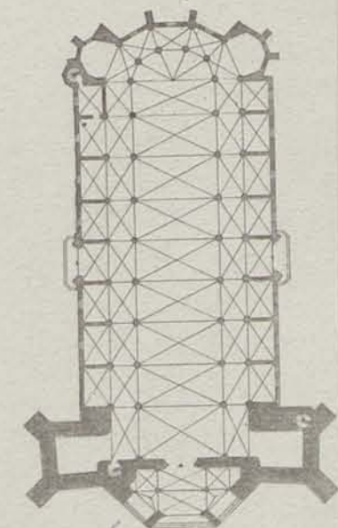
PLAN GÉNÉRAL
