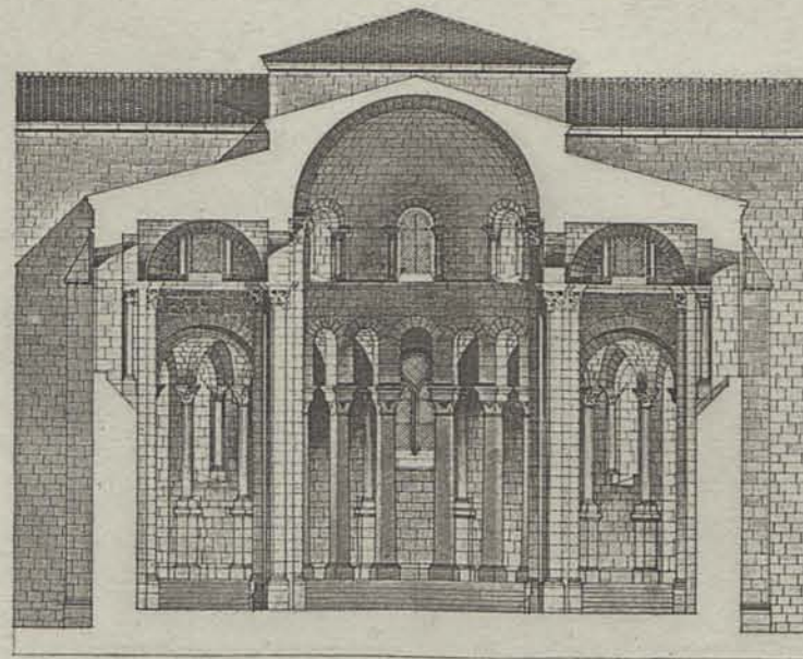
Coupe Transversale
