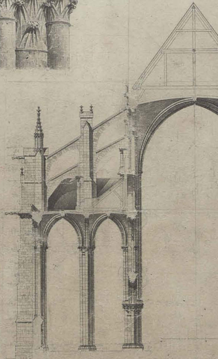
Coupe transversale
