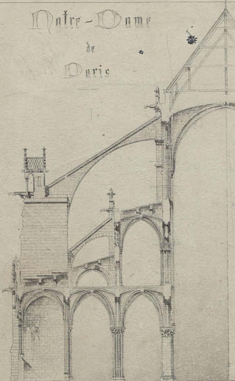
Coupe transversal
