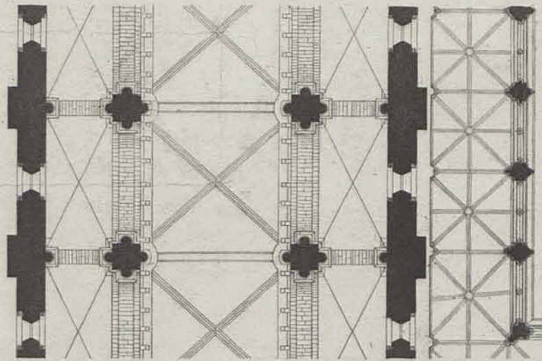
PLAN DU REZ-DE-CHAUSSEE
