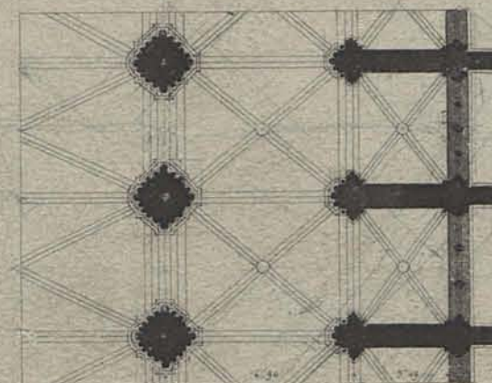
Plan intérieur
