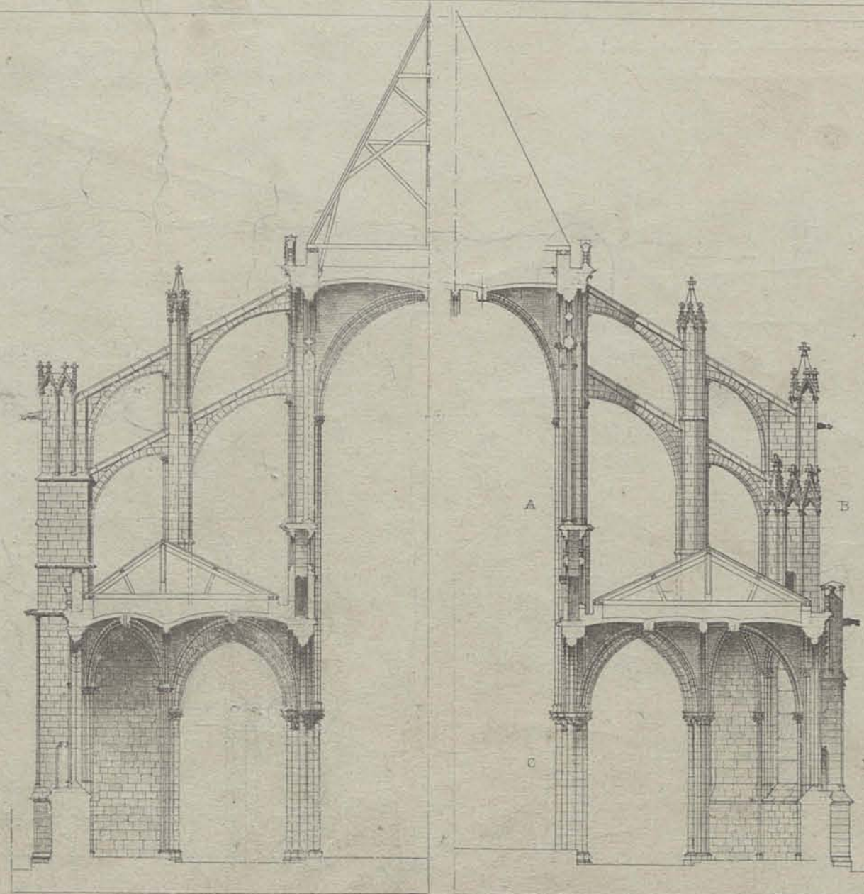
Coupe Transversale
