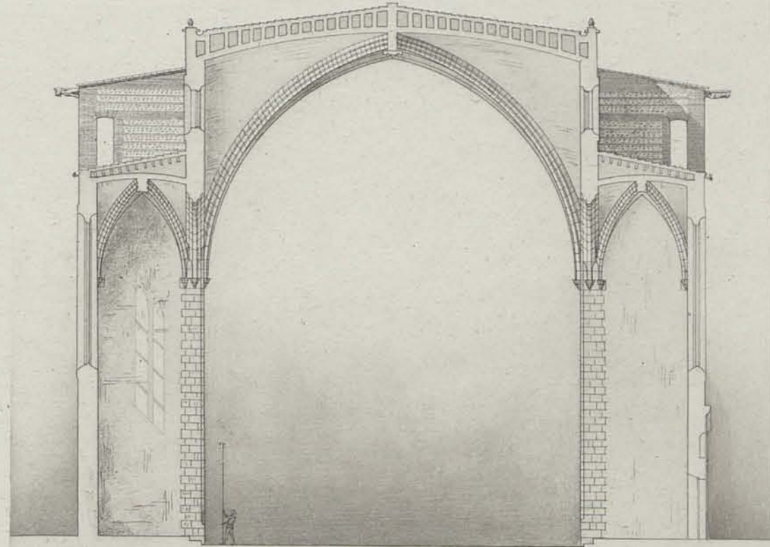
Coupe transversale
