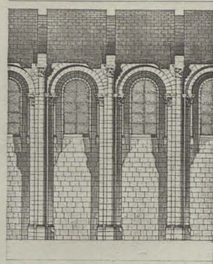
Coupe Longitudinale
