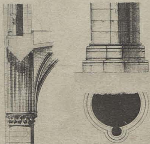
Bases des Piliers.
