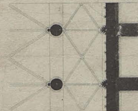
Plan d'une travée
