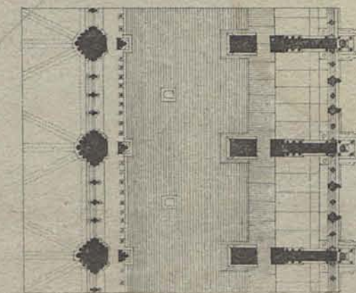
Plan sur le chœur de Rouen
