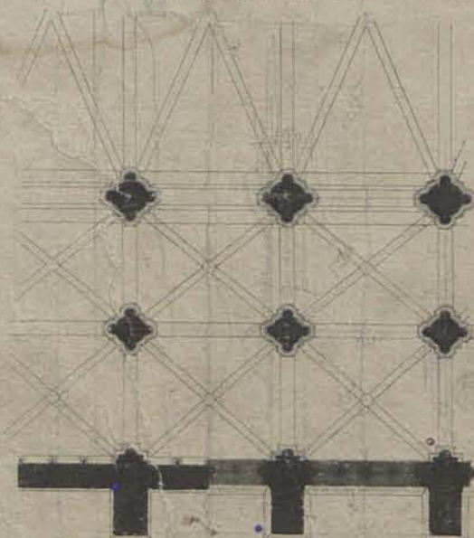
Plan d'une travée
