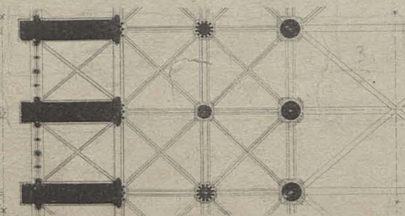
Plan au Rez de Chaussée
