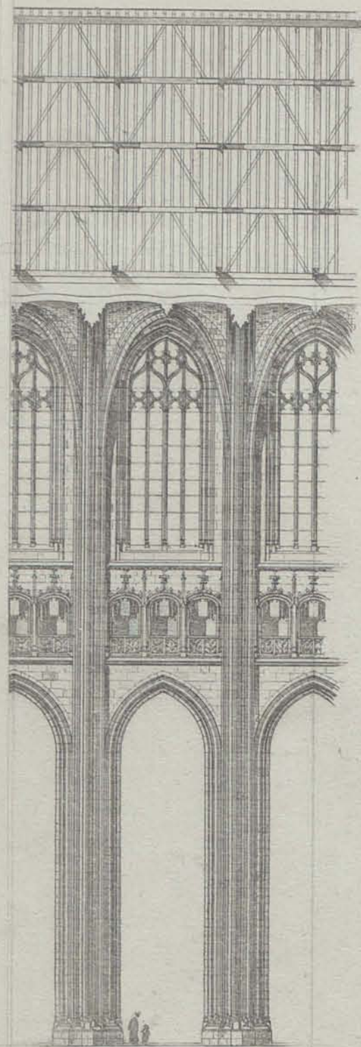
COUPE LONGITUDINALE
