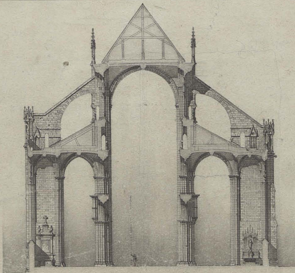
Coupe transversale sur la Nef
