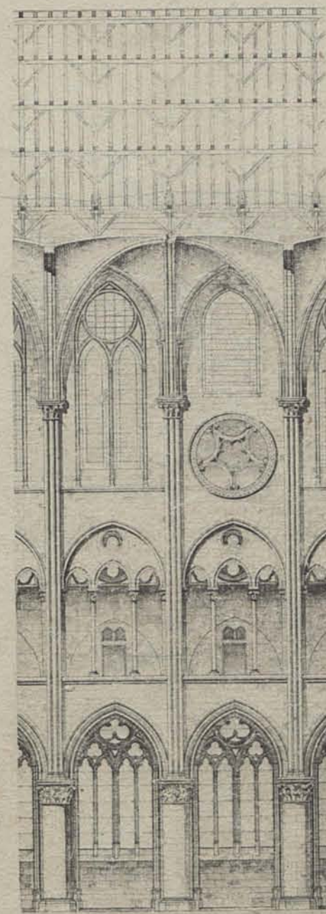
Coupe longitudinale
