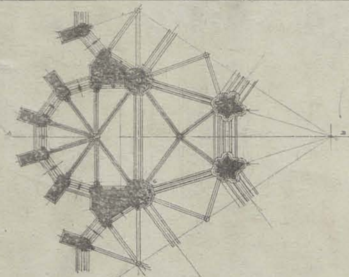
PLAN D'UNE CHAPELLE ABSIDALE
