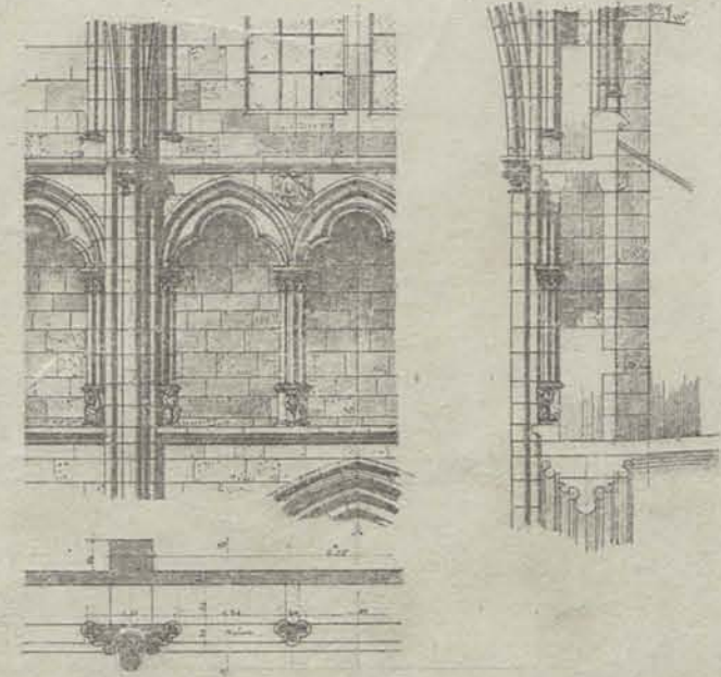
TRIPORIUM DE LA NEF
