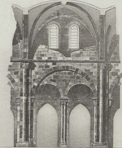
Elevation d'une Travee Nord
