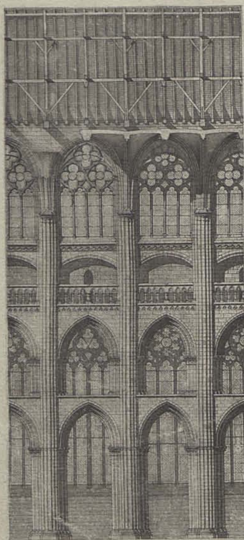
Face intérieure
