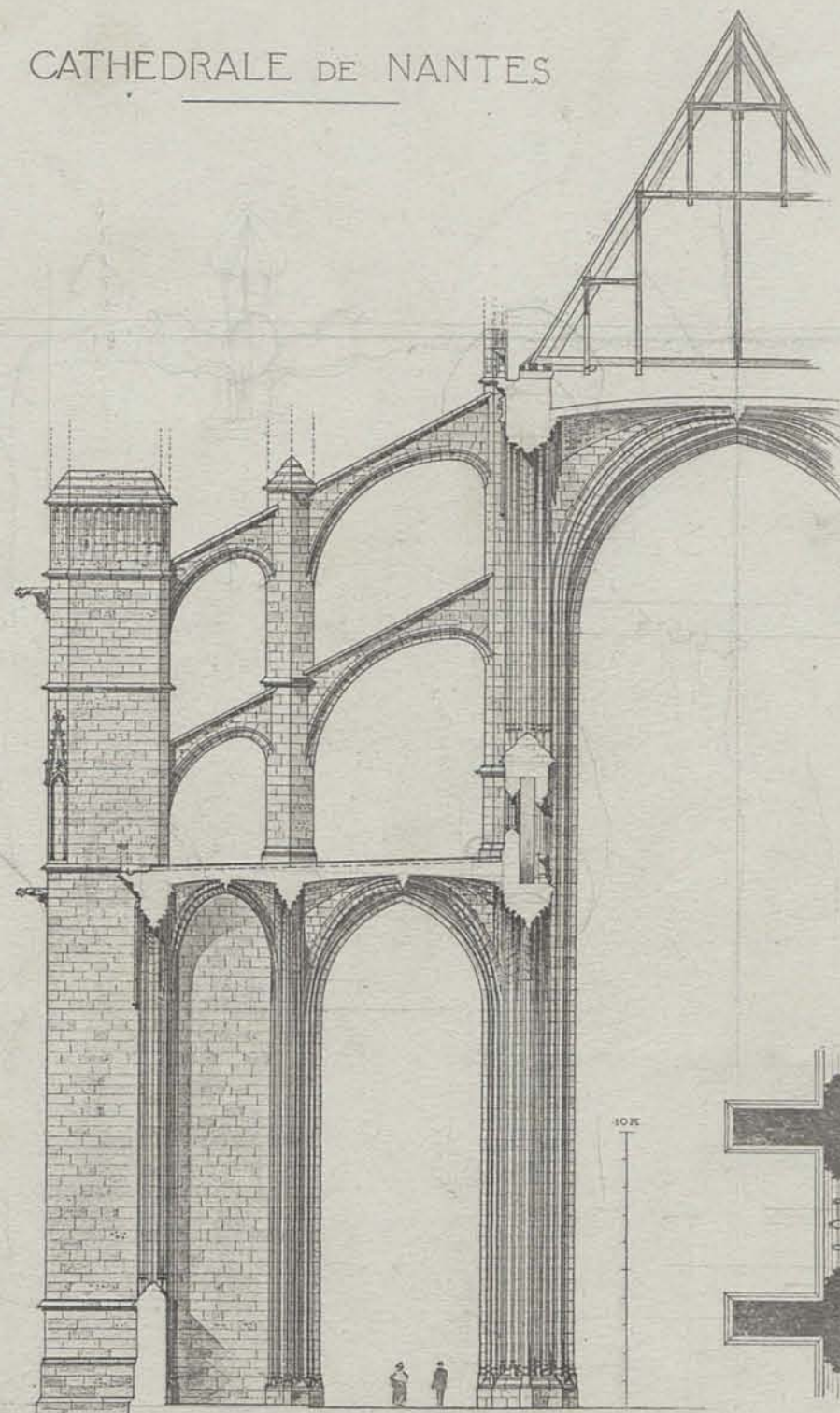
COUPE TRANSVERSALE
