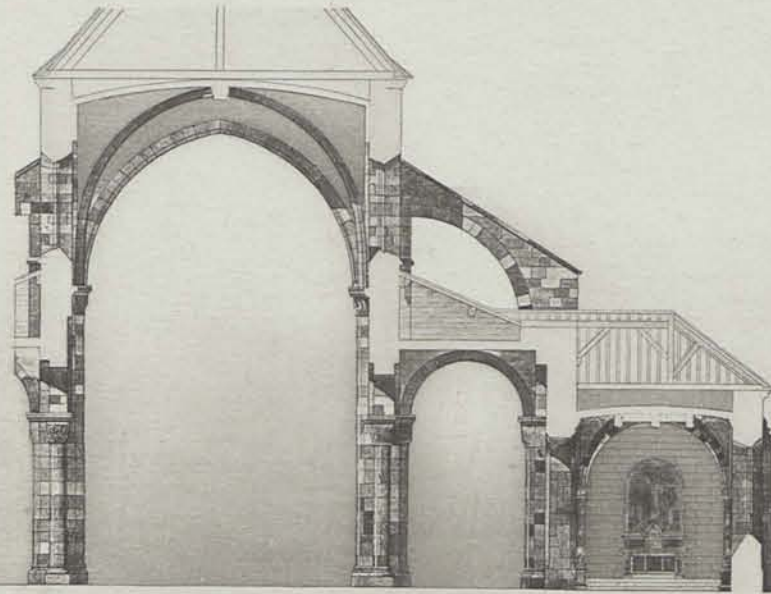
COUPE TRANSVERSALE
