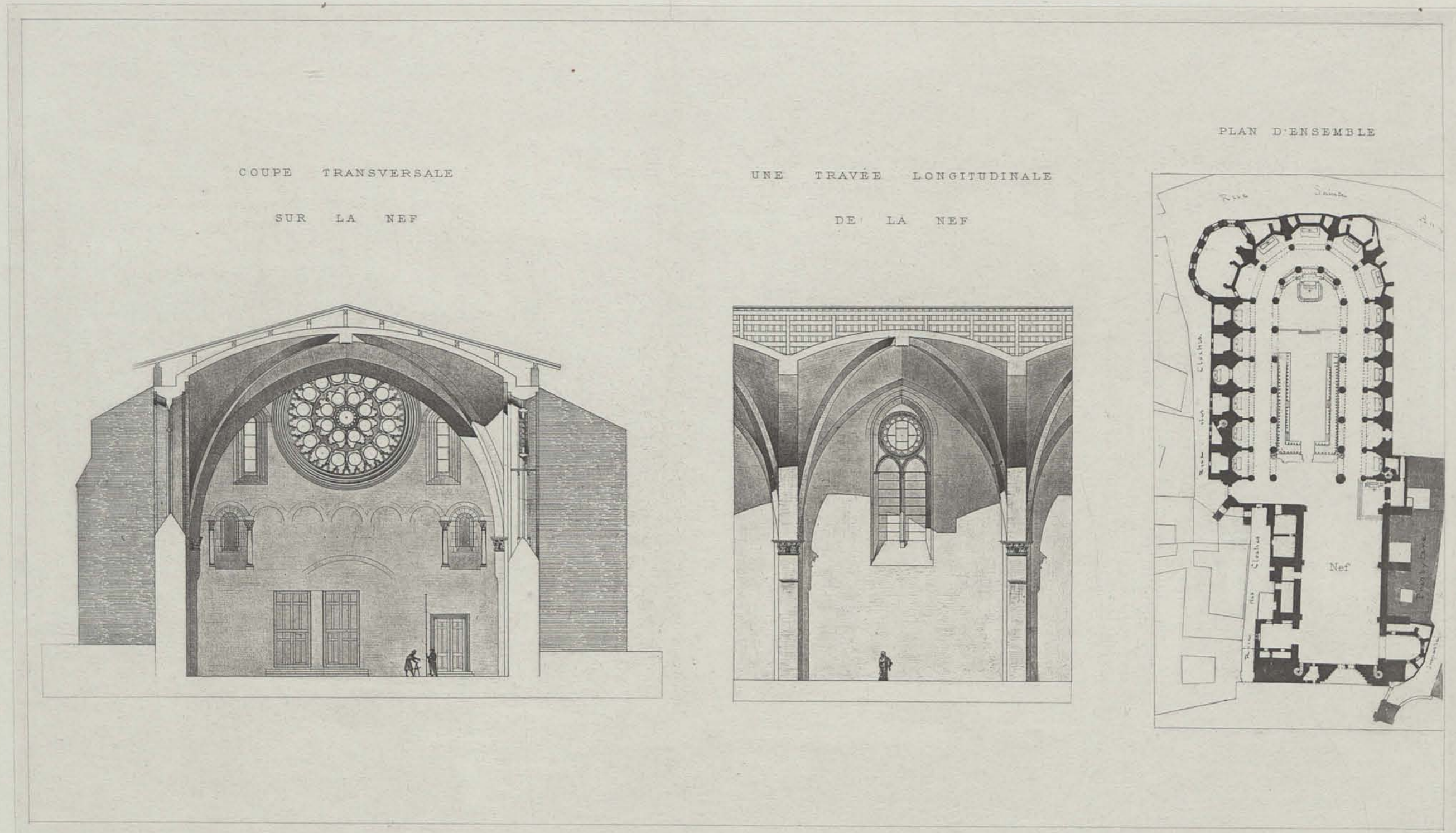
CATHEDRALE DE TOULOUSE (H TE GARONNE) (NEF)
