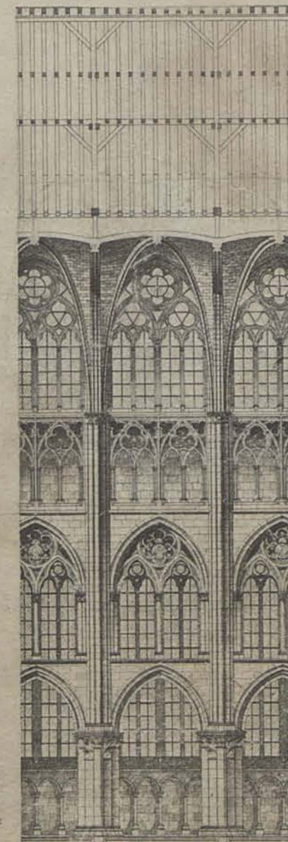
Coupe longitudinale
