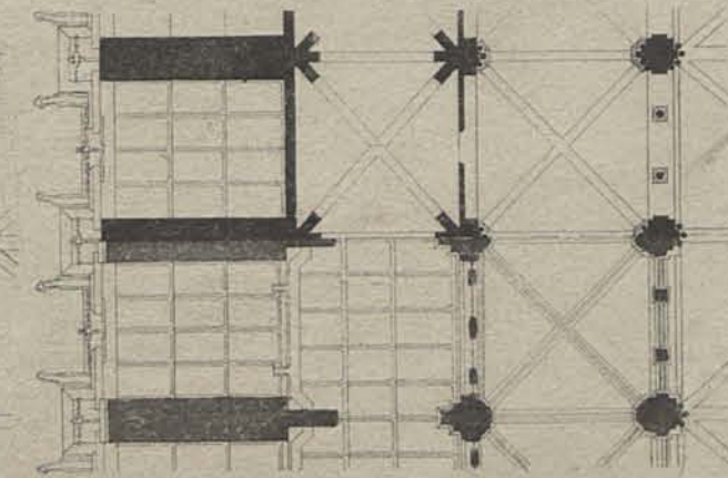
Plan au Sol et à la naissance du Triforium
