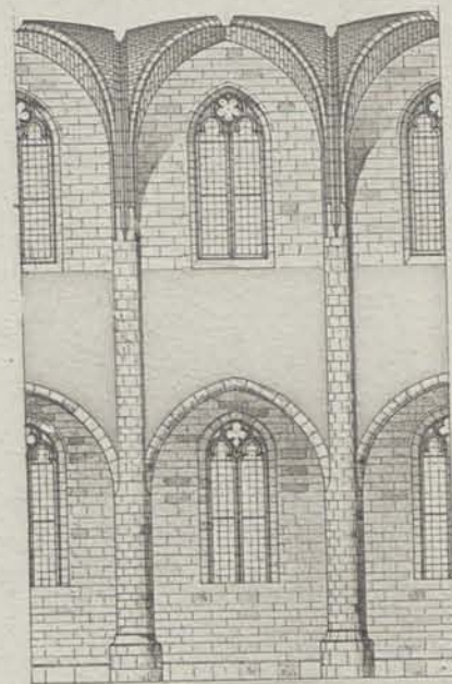
COUPE LONGITUDINALE
