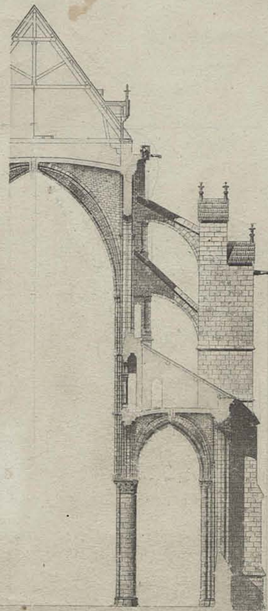
Plan, coupes transversale et longitudinale élévation extérieure et Détails d'une travée de la Nef
