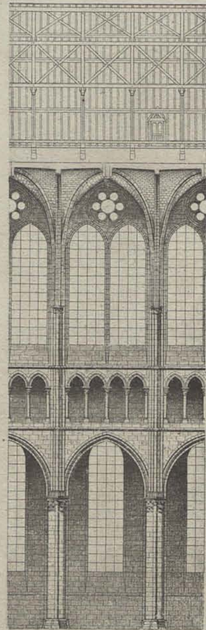
Plan, coupes transversale et longitudinale élévation extérieure et Détails d'une travée de la Nef
