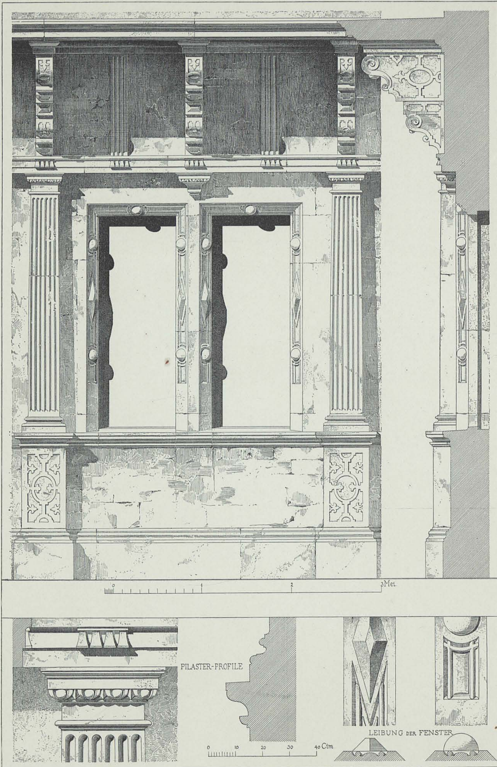
MOTIF DE LA FAÇADE DU CHÂTEAU DE BRACKE.
