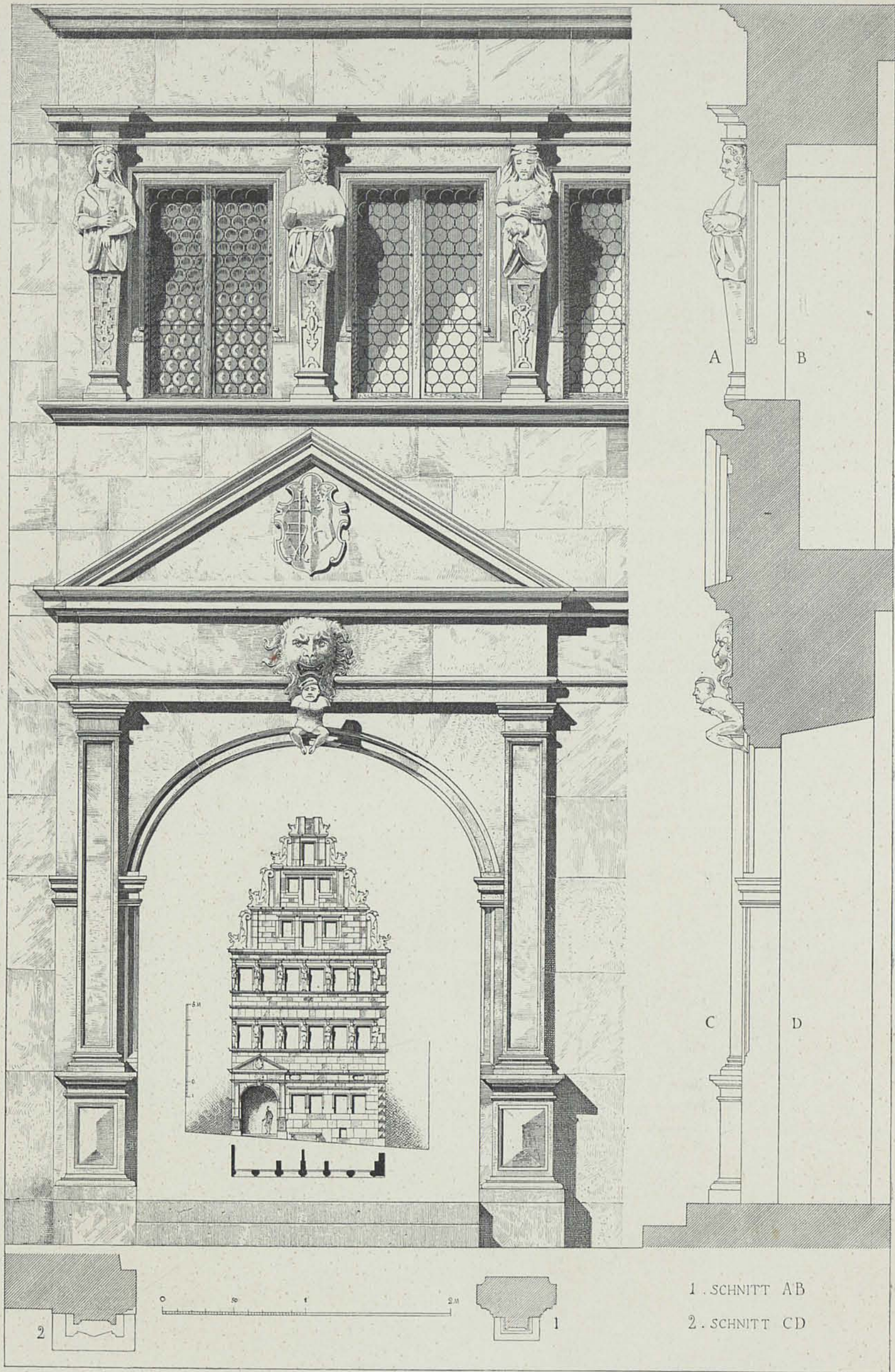
FASSADE DES BAUMEISTERHAUSES.
