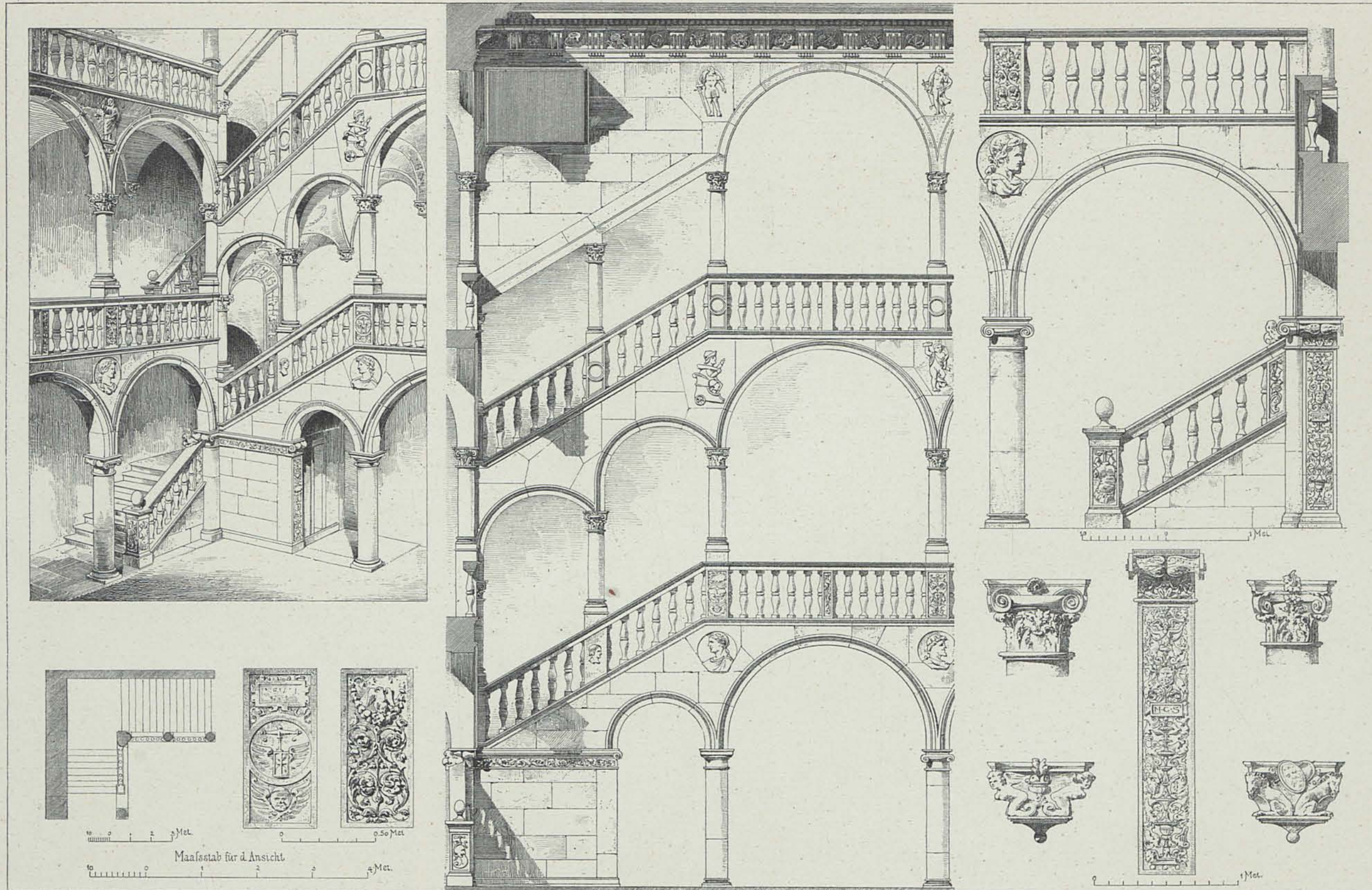
TREPPE IM HOFE VON SCHLOSS PORZIA.
