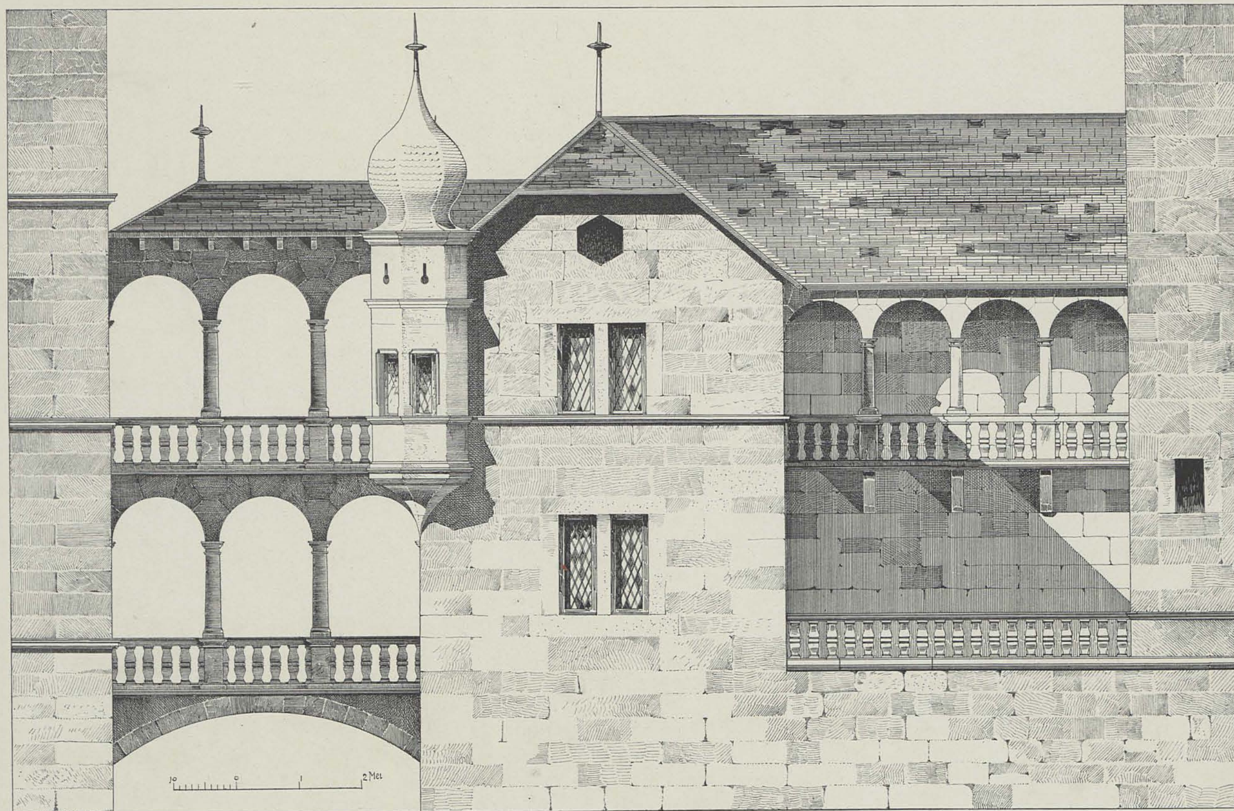
PARTIE DU PALAIS STOCKALPER.
