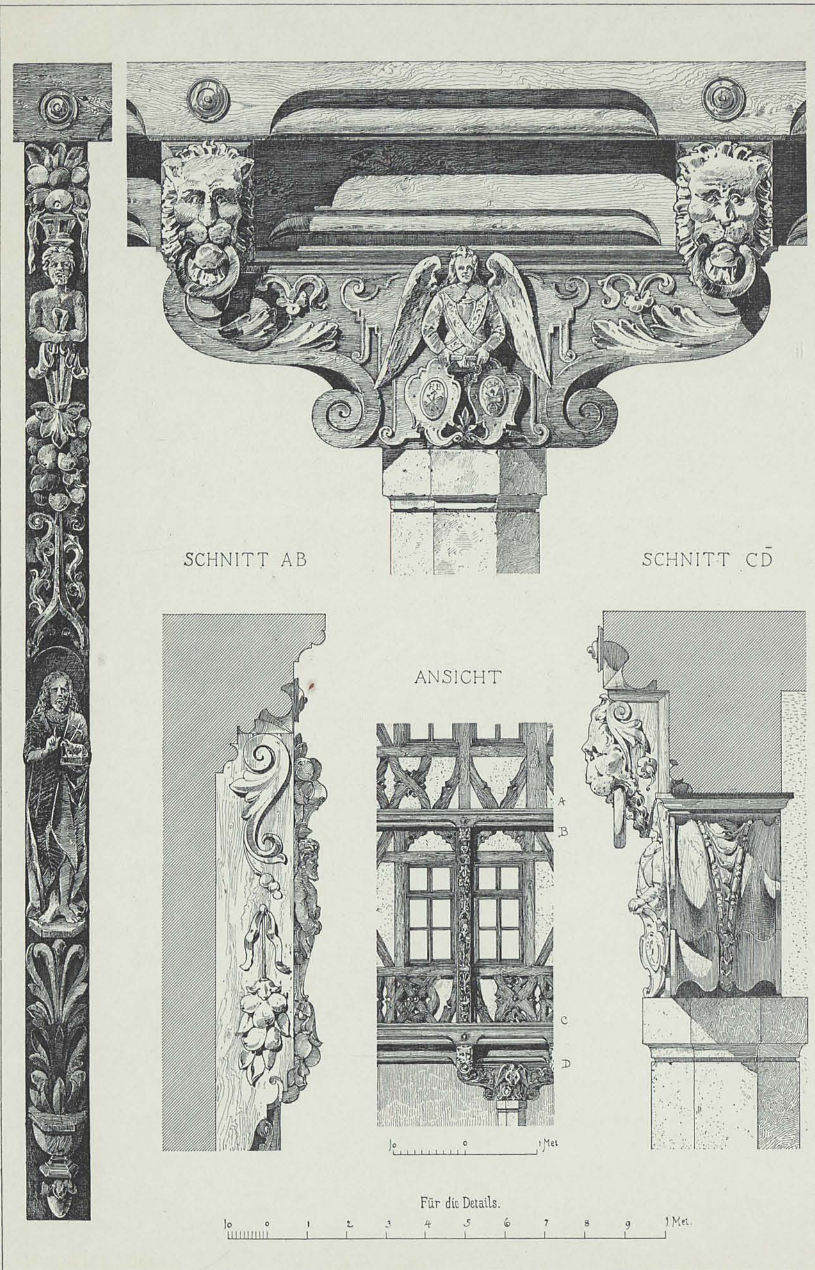
DÉTAILS D'UNE COUR.
