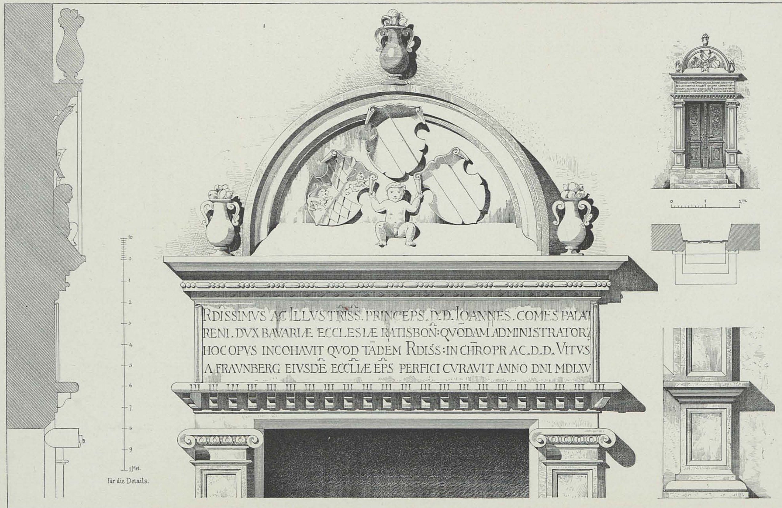
DETAIL EINER THÜRE (BISCHOFSHOF).
