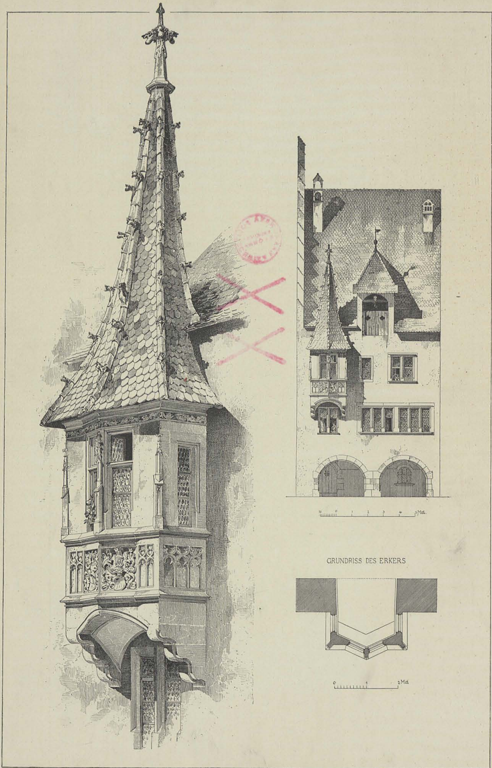
ERKER.
