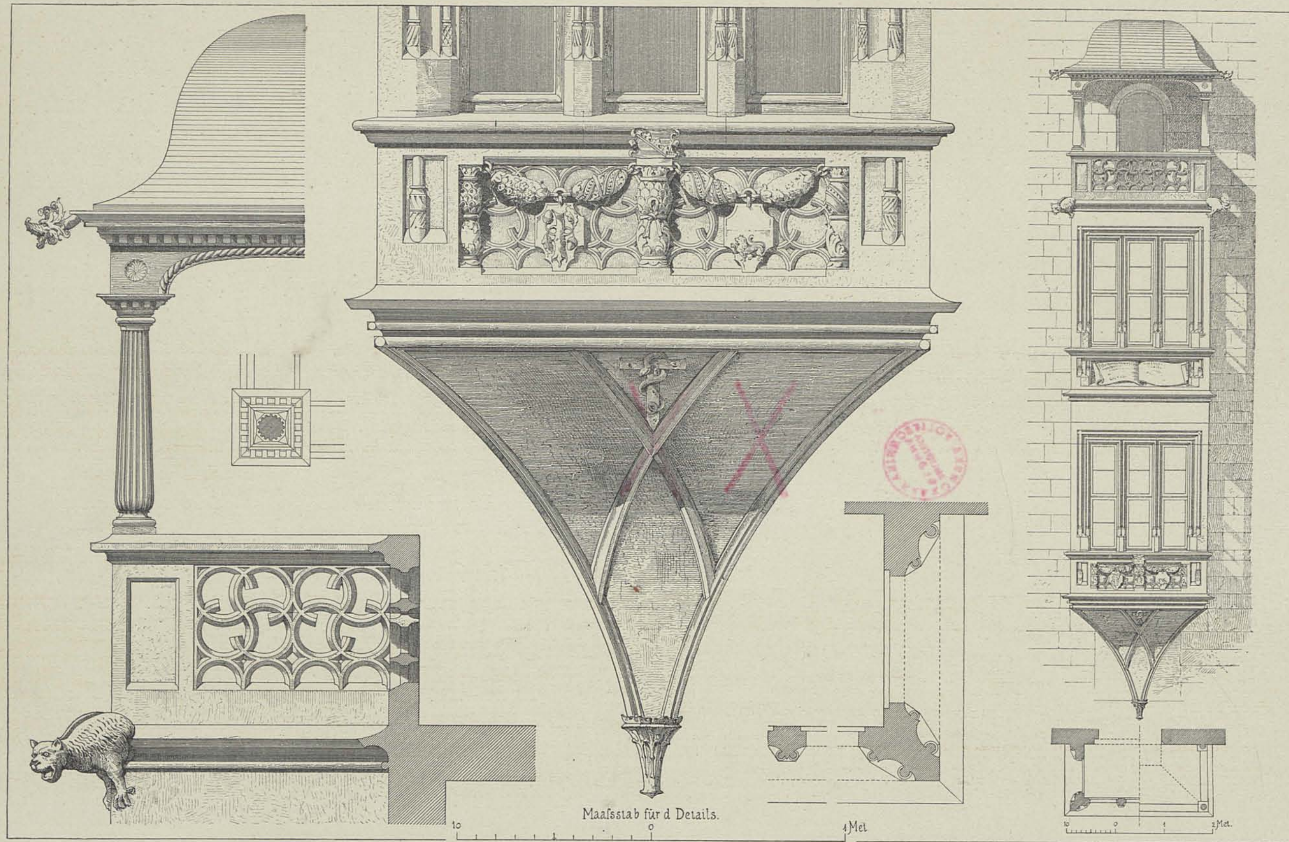
ERKER IM HOFE EINES HAUSES DER HAINSTRASSE.
