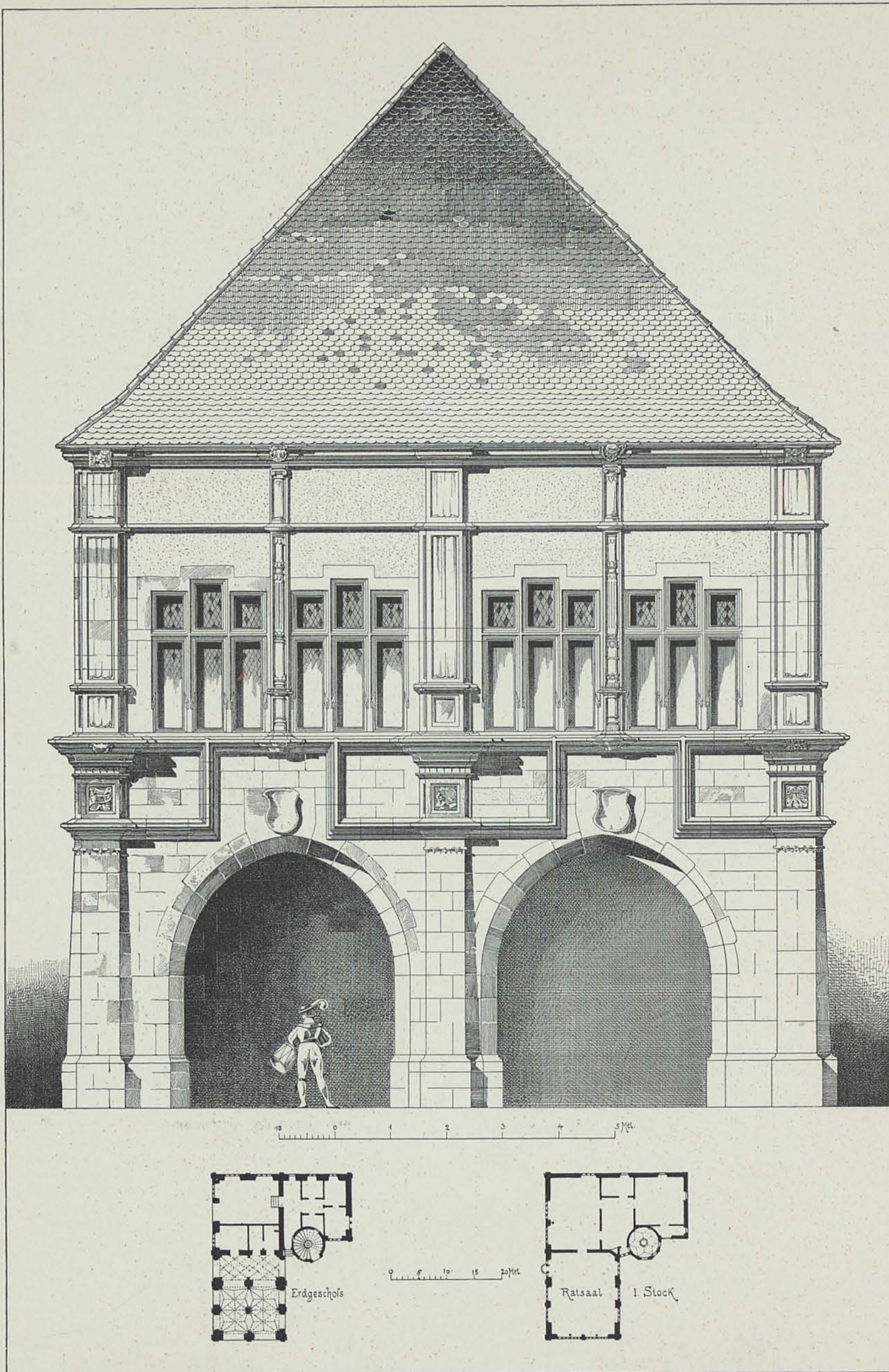
FAÇADE DE L'HÔTEL DE VILLE.
