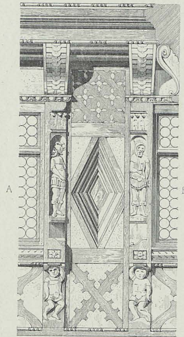
SCHNITT AB MITTELPFEILER DER FASSADE II. STOCK
