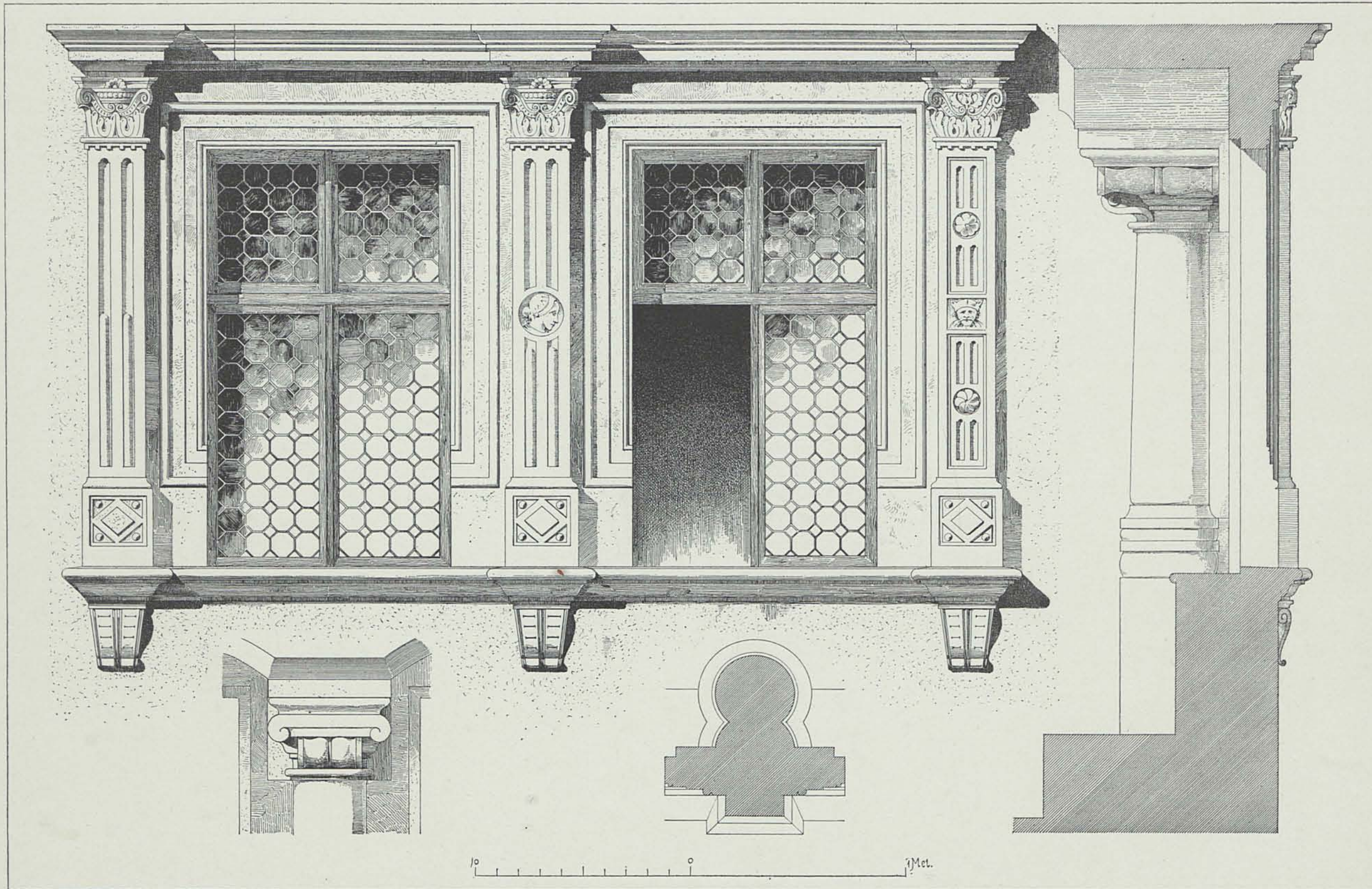
DOUBLE-FENÊTRE.
