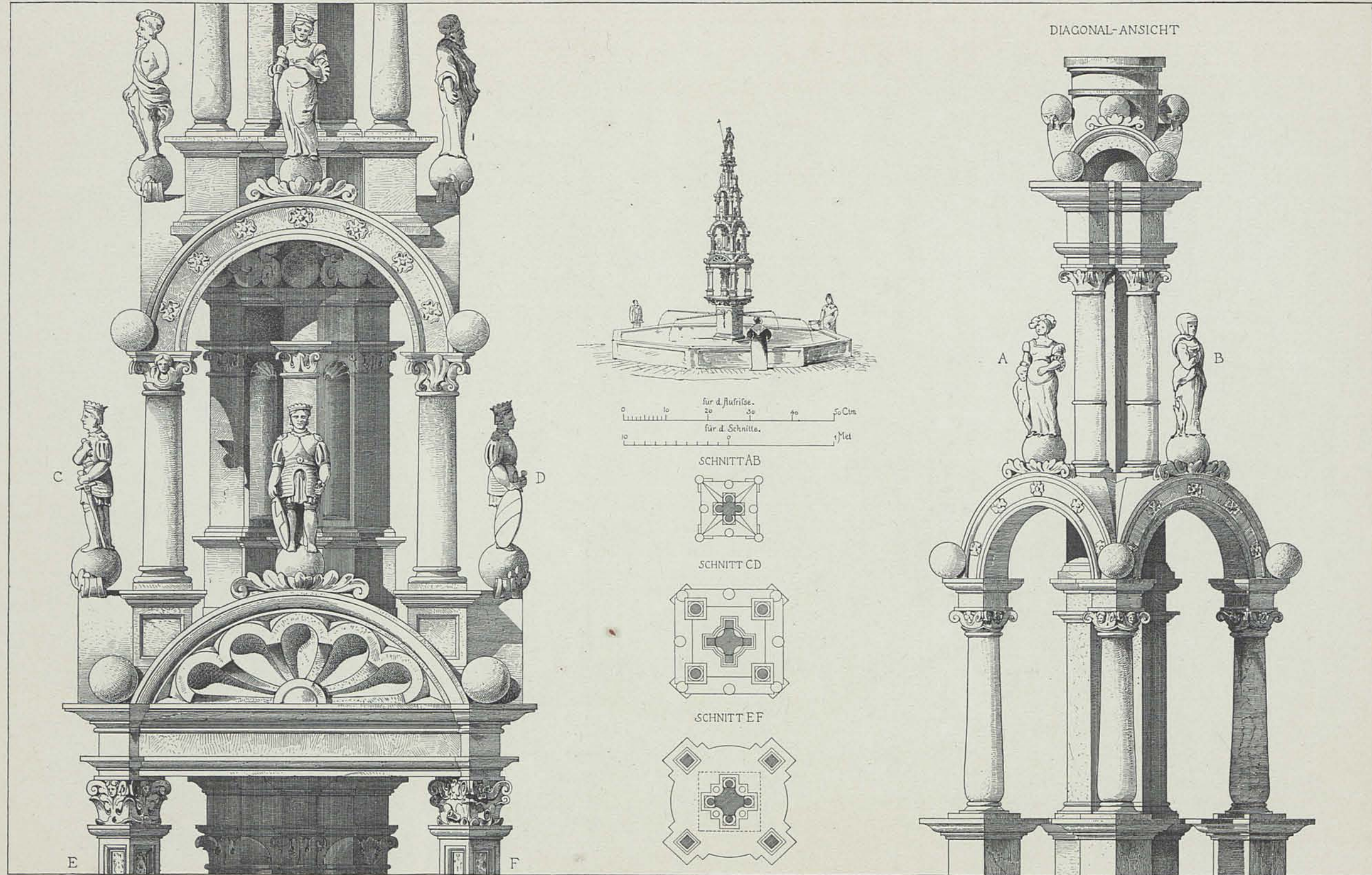
BRUNNEN AUF DEM MARKTPLATZE.
