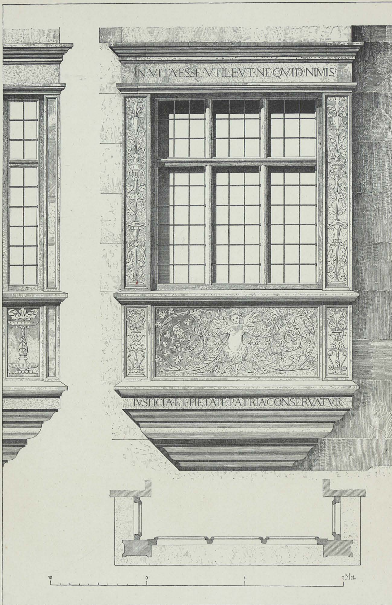
ERKER AM WELSERHAUS.
