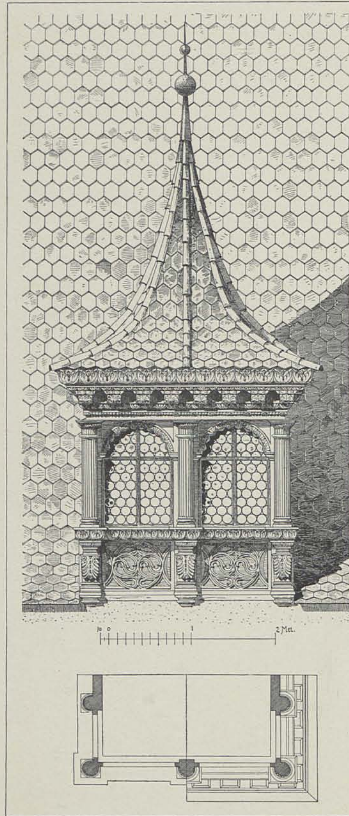
DACHFENSTER.
