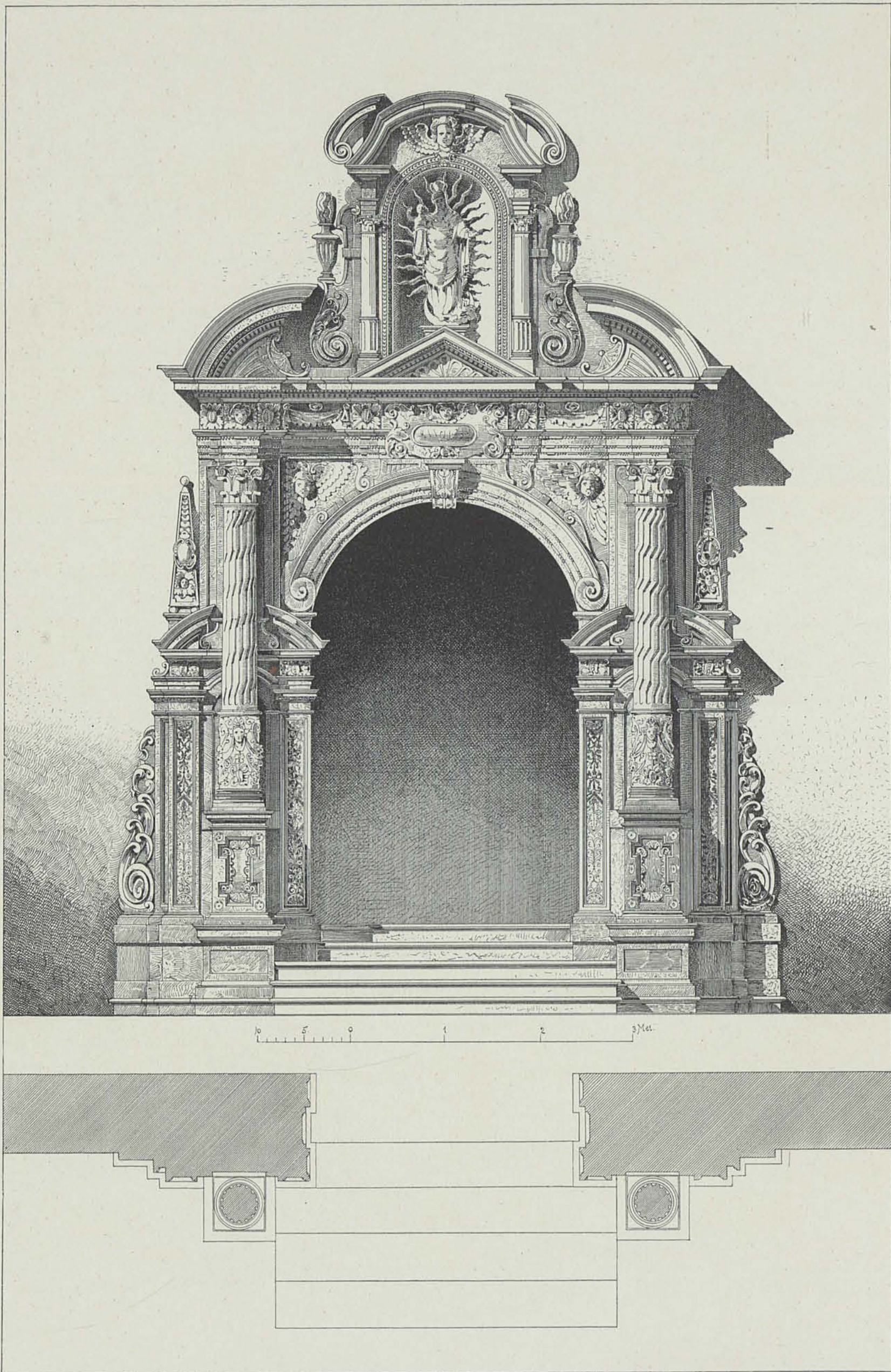
PORTAL VON ST. LEODOGAR.
