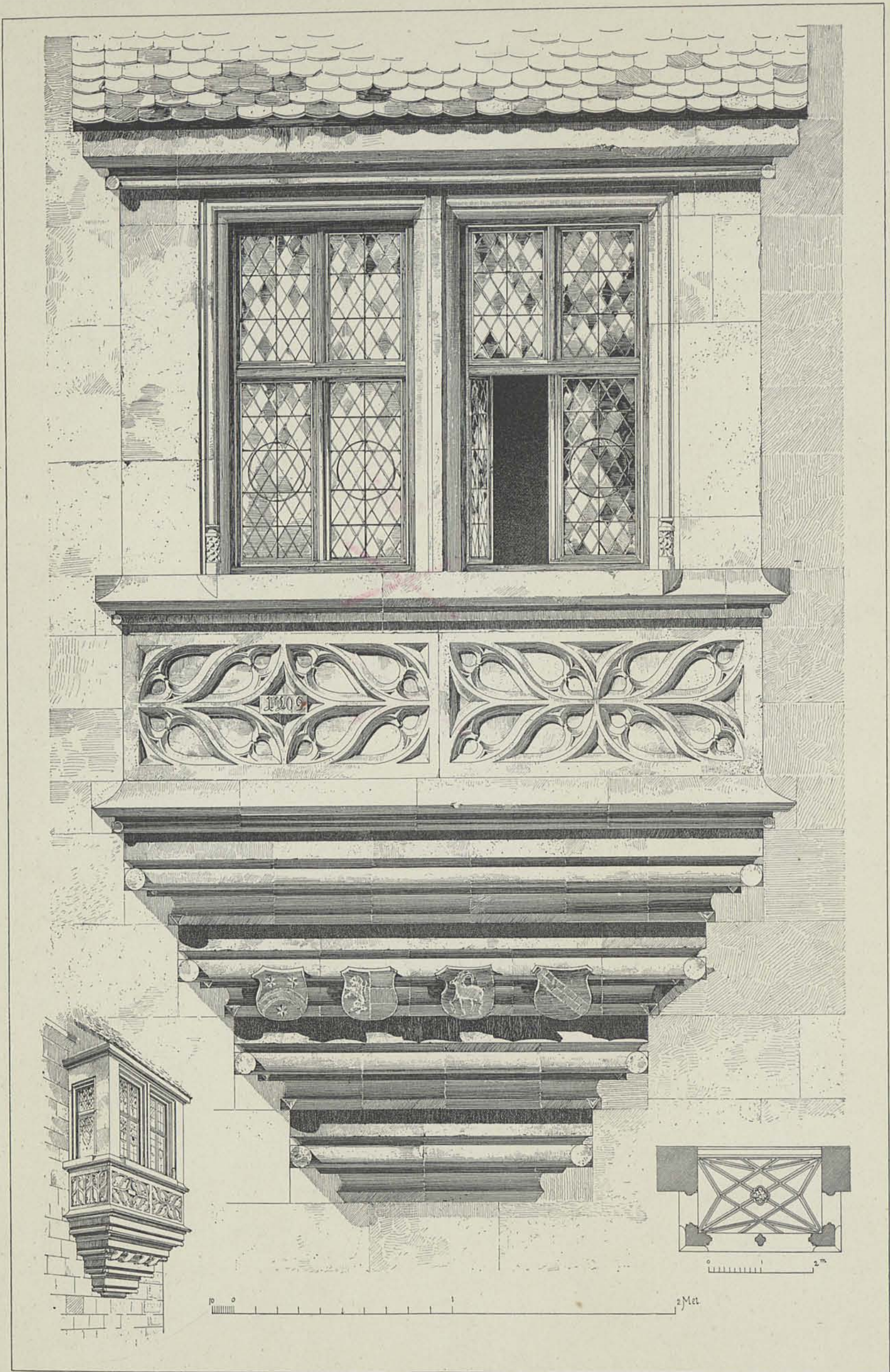
TOURELLE.
