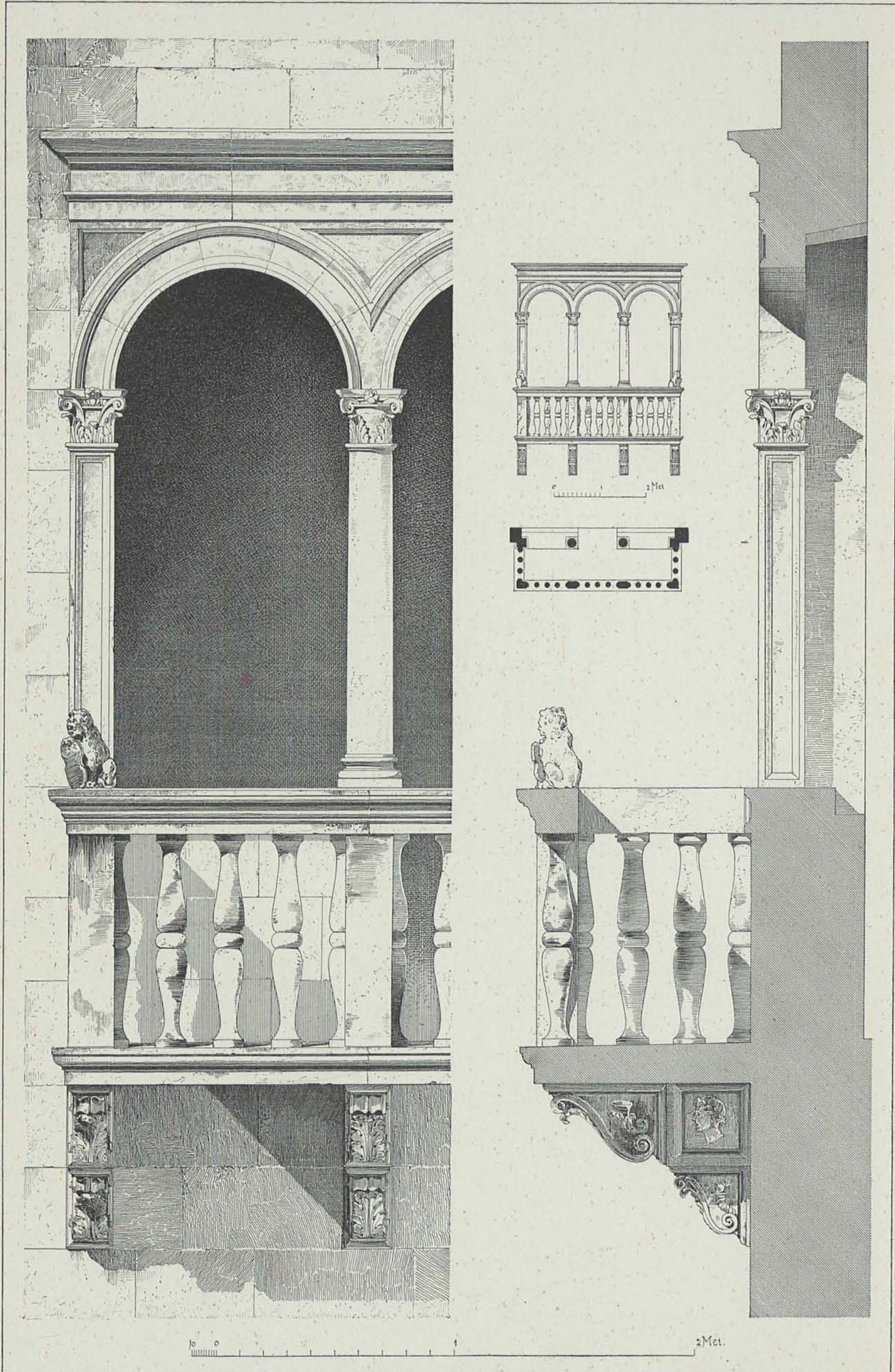
BALKON DES SCHLOSSES PORZIA.
