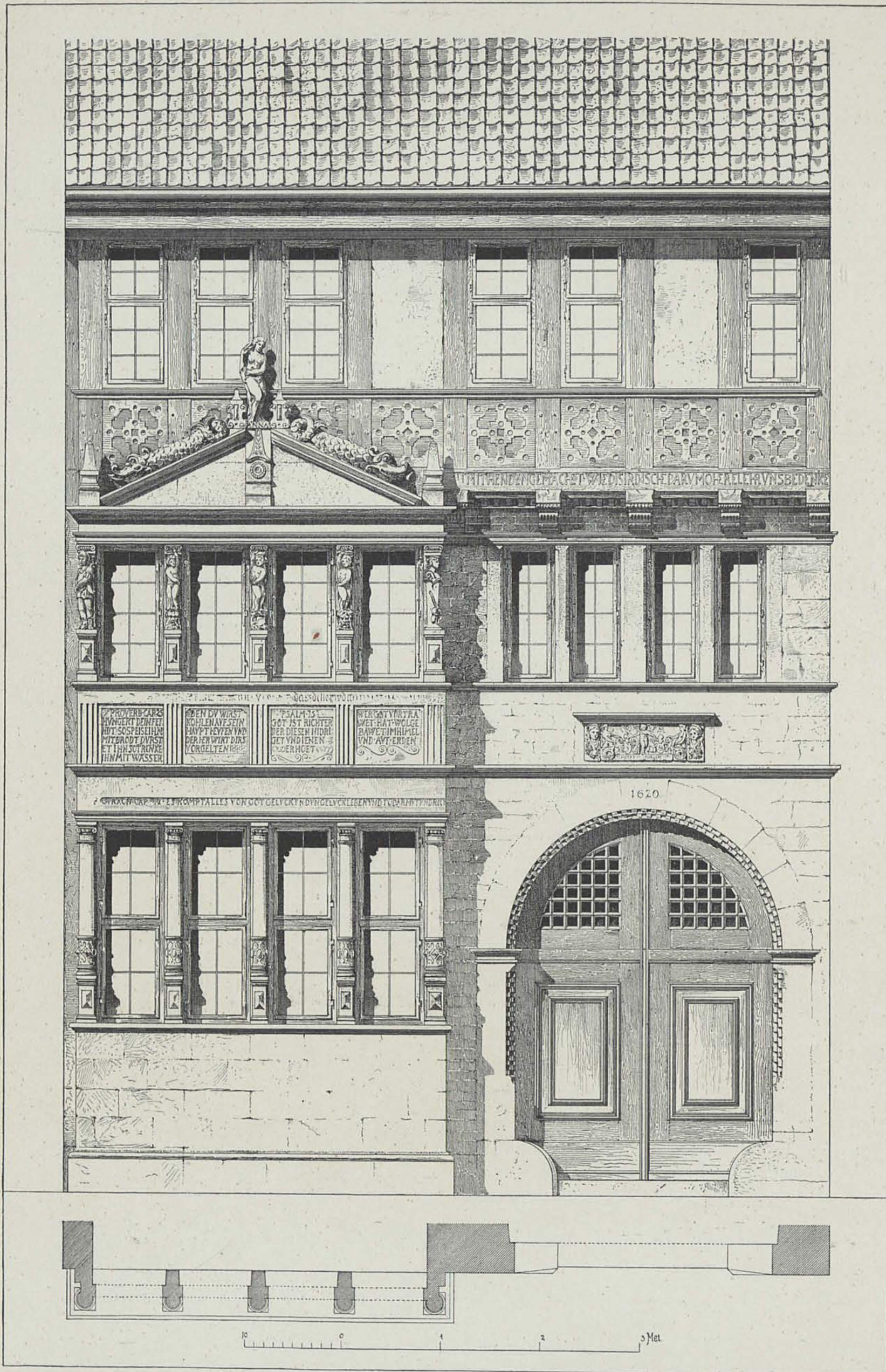
FASSADE BURGSTRASSE 23.
