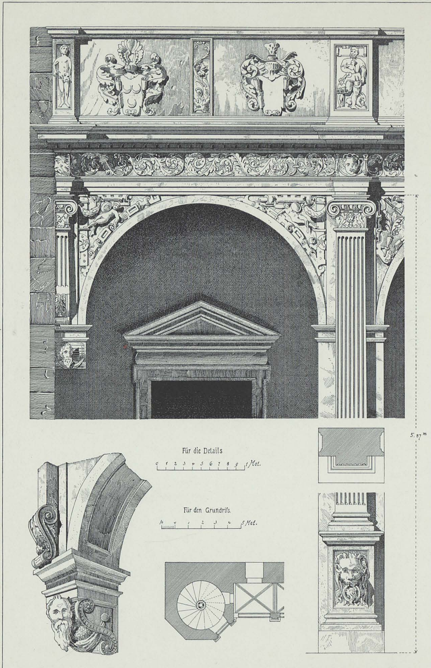
DETAILS VOM SCHLOSS.
