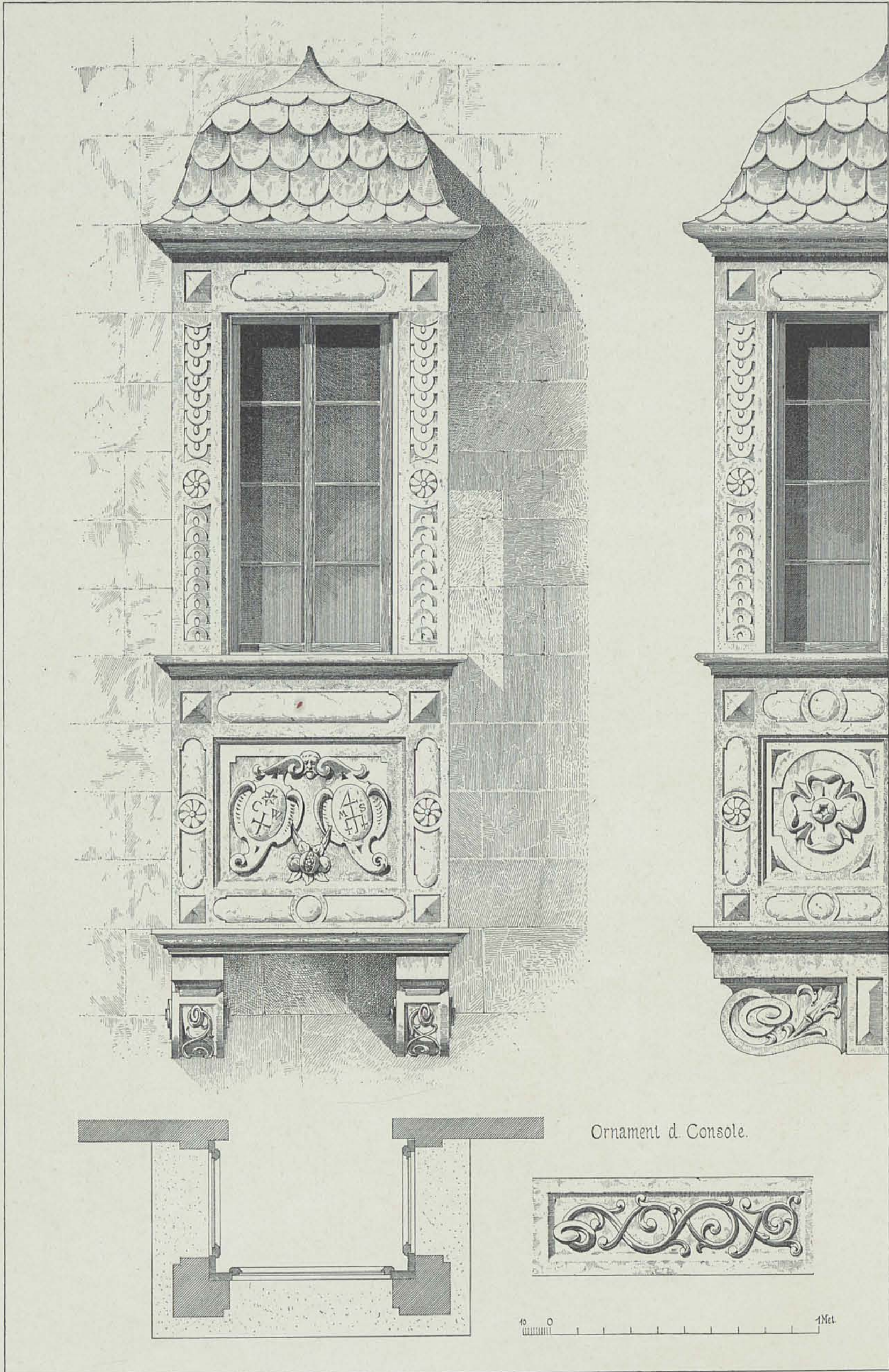
ERKER.
