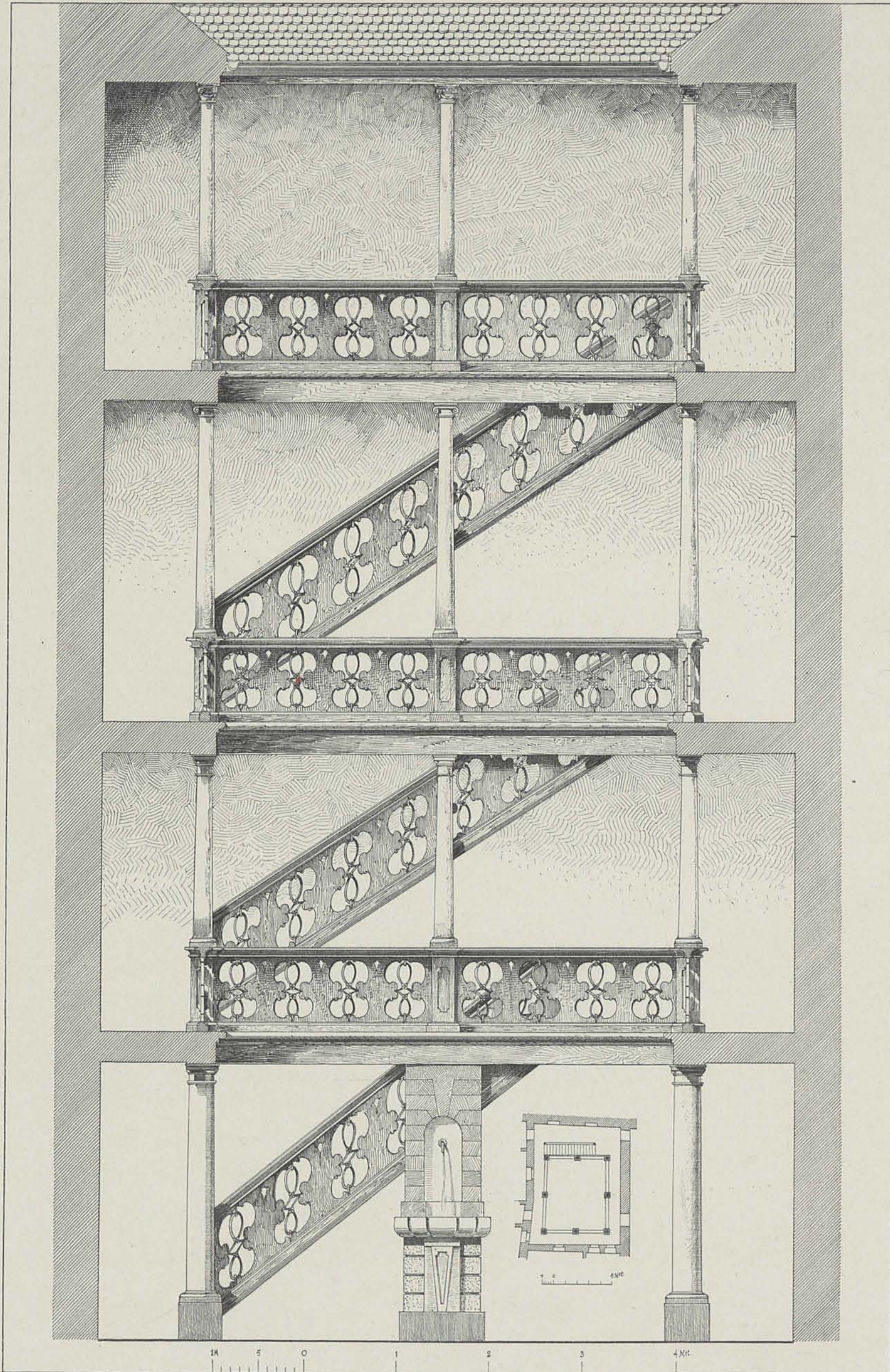
GALERIE UND TREPPE EINES HOFES.
