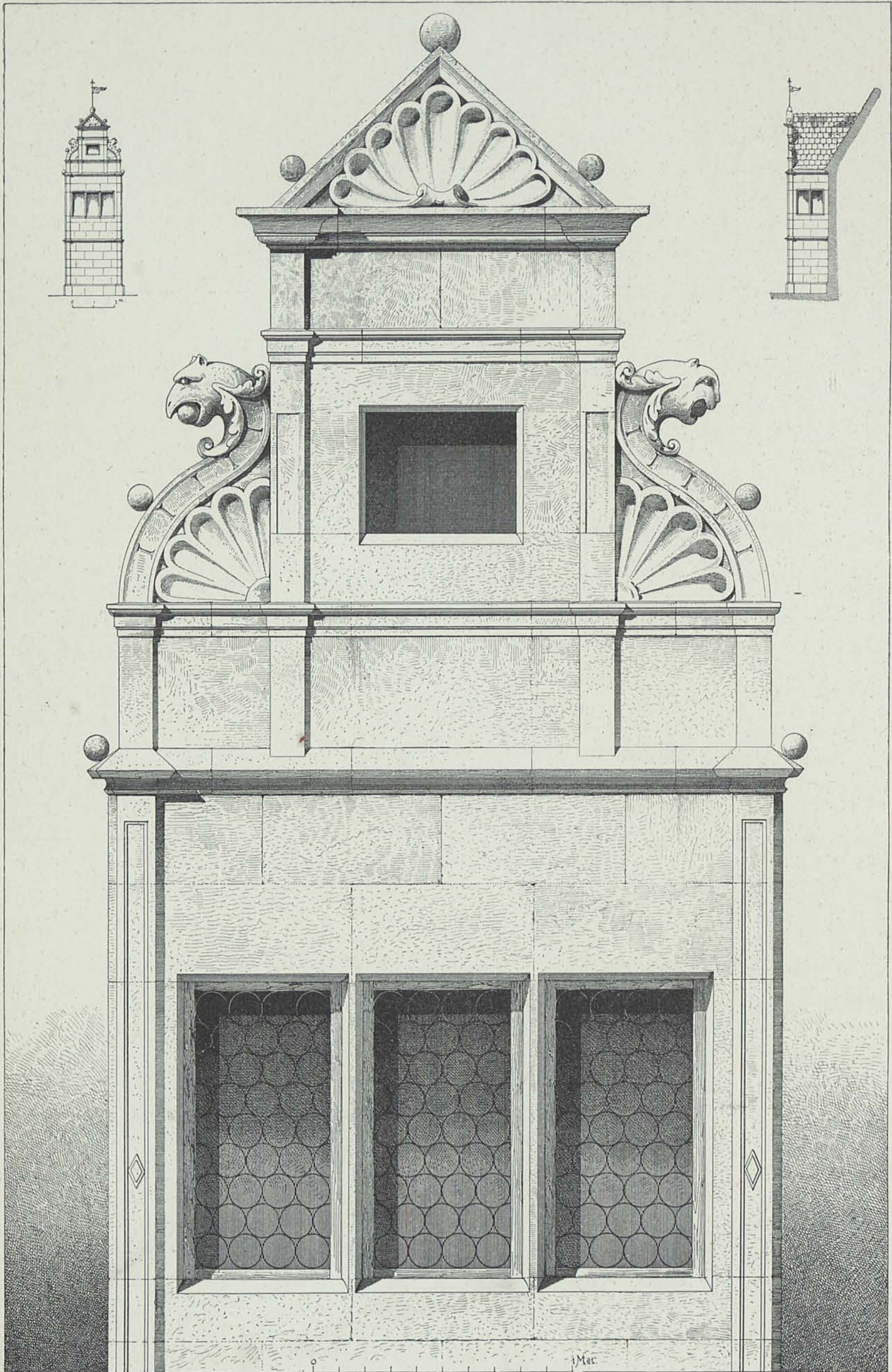
AVANT-CORPS D'UNE MAISON.
