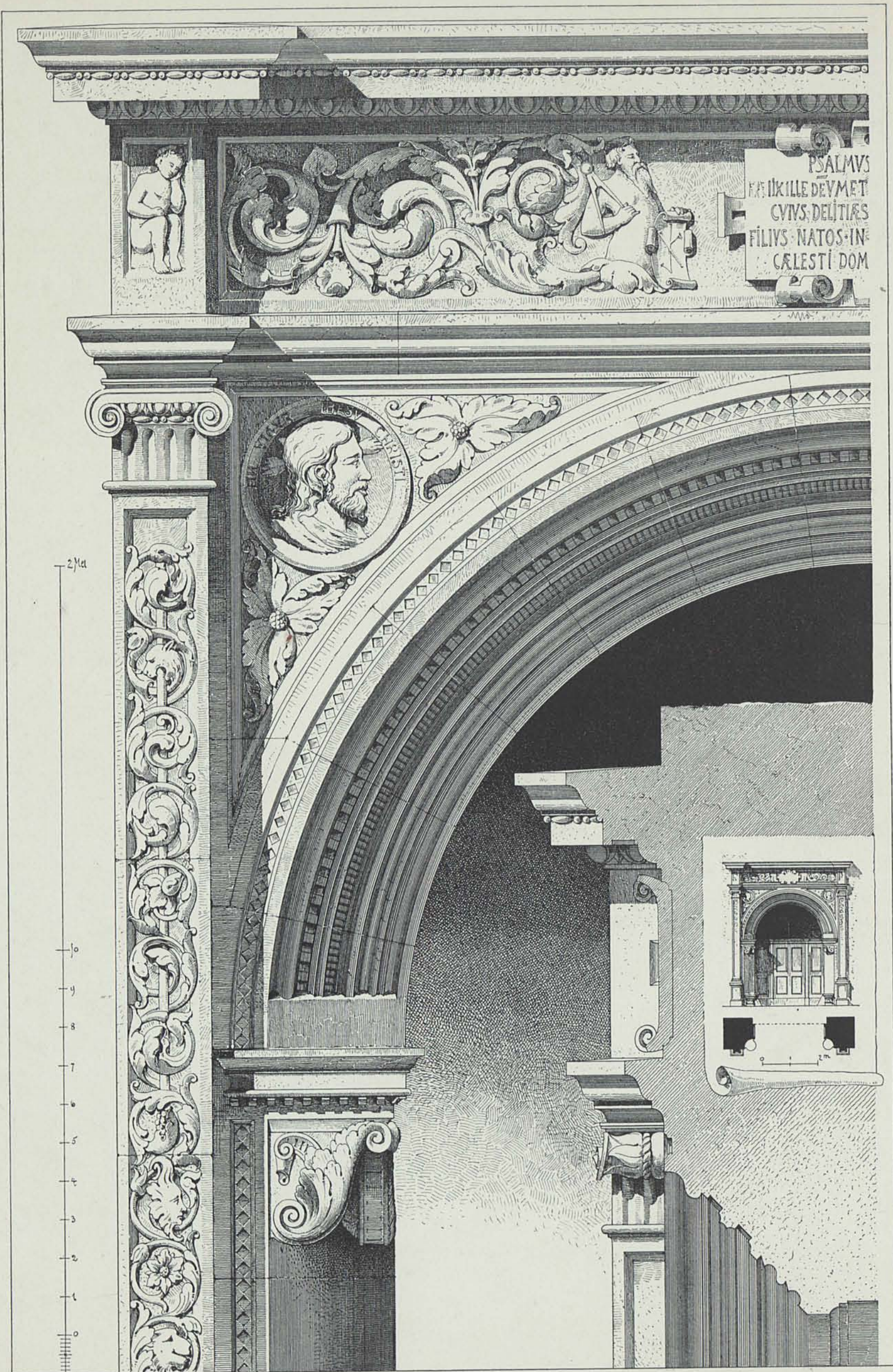
DÉTAIL D'UN PORTAIL.
