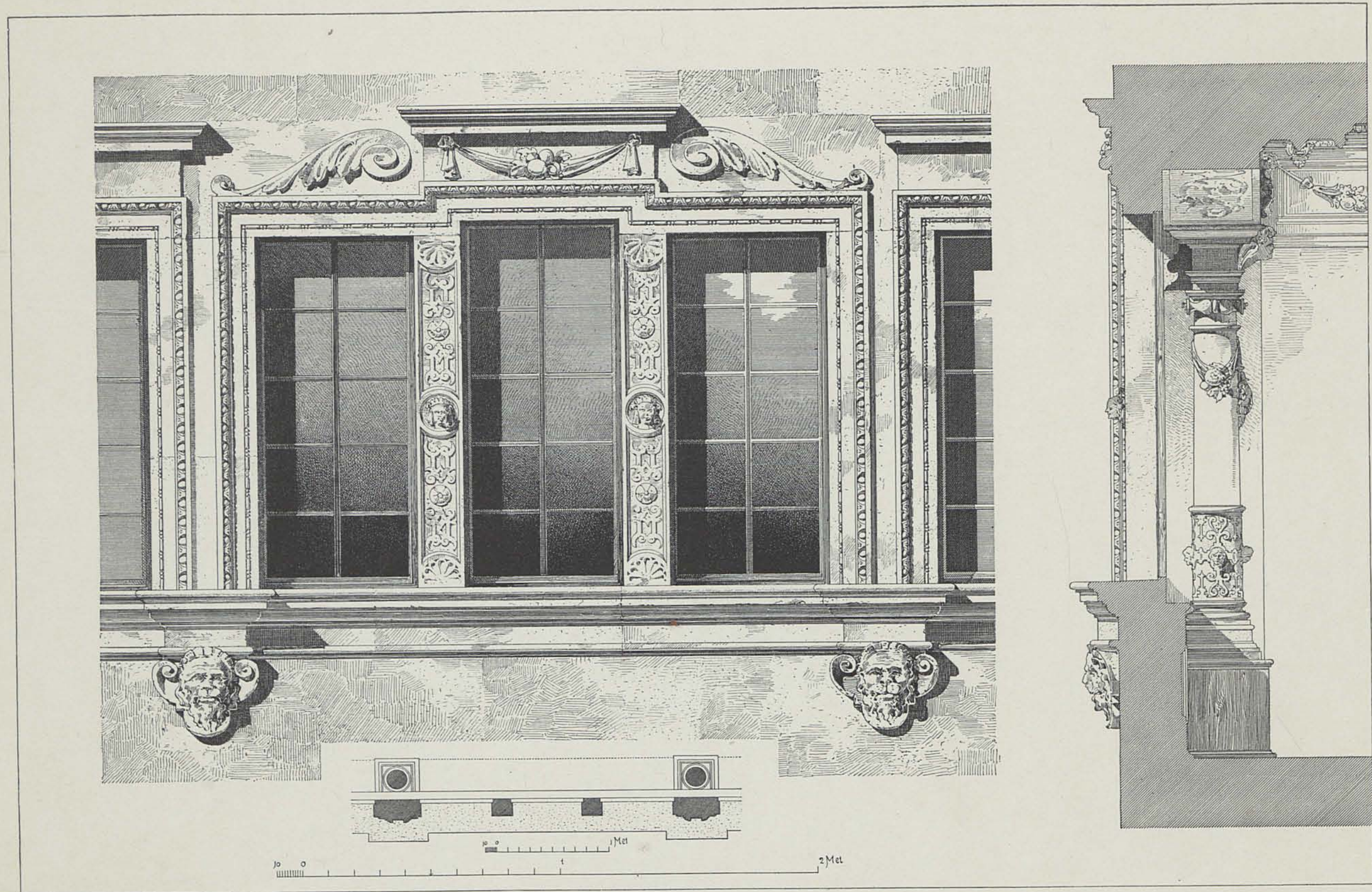
FENÊTRE.
