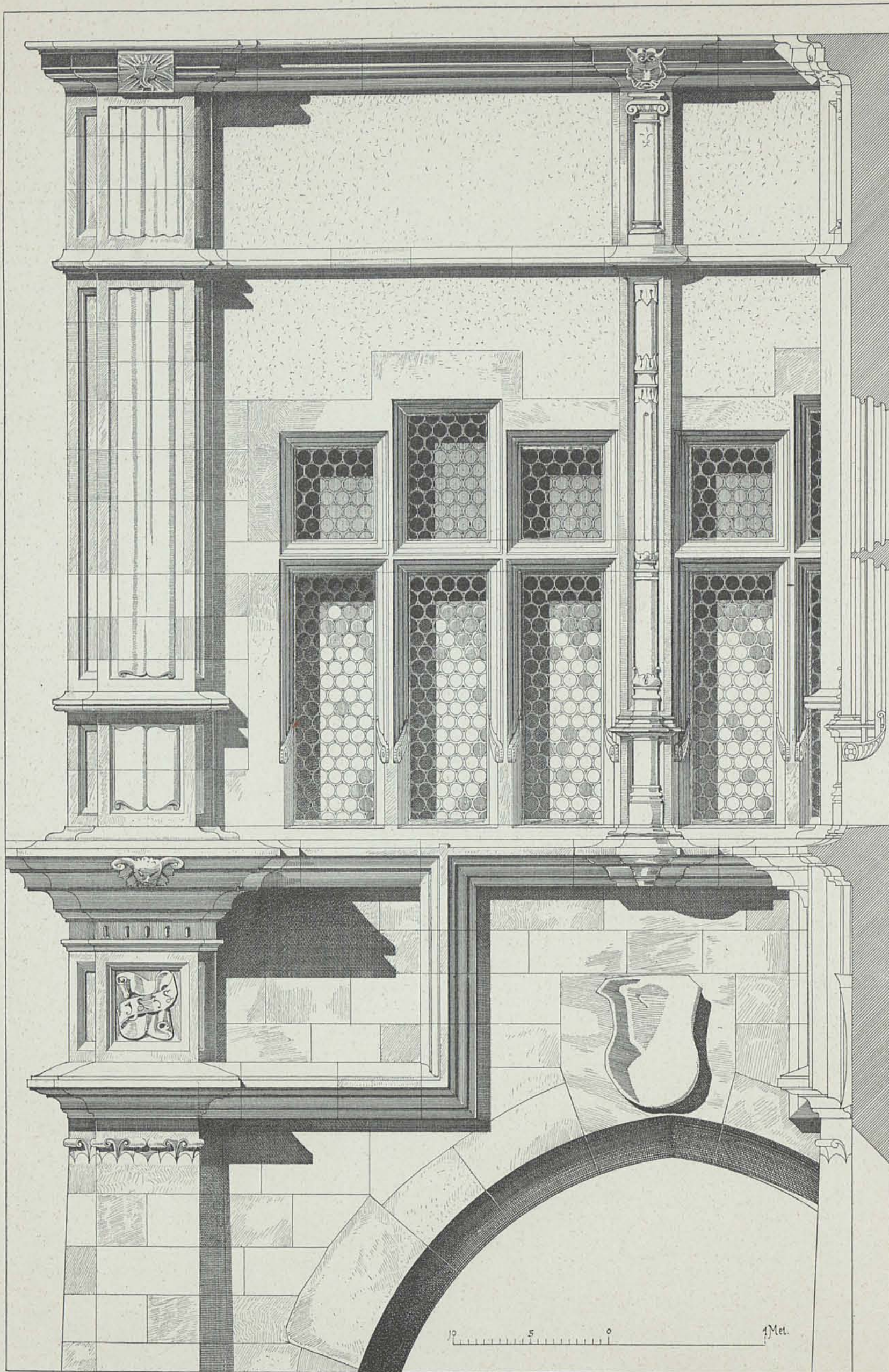
DETAIL DER FASSADE DES RATHAUSES.
