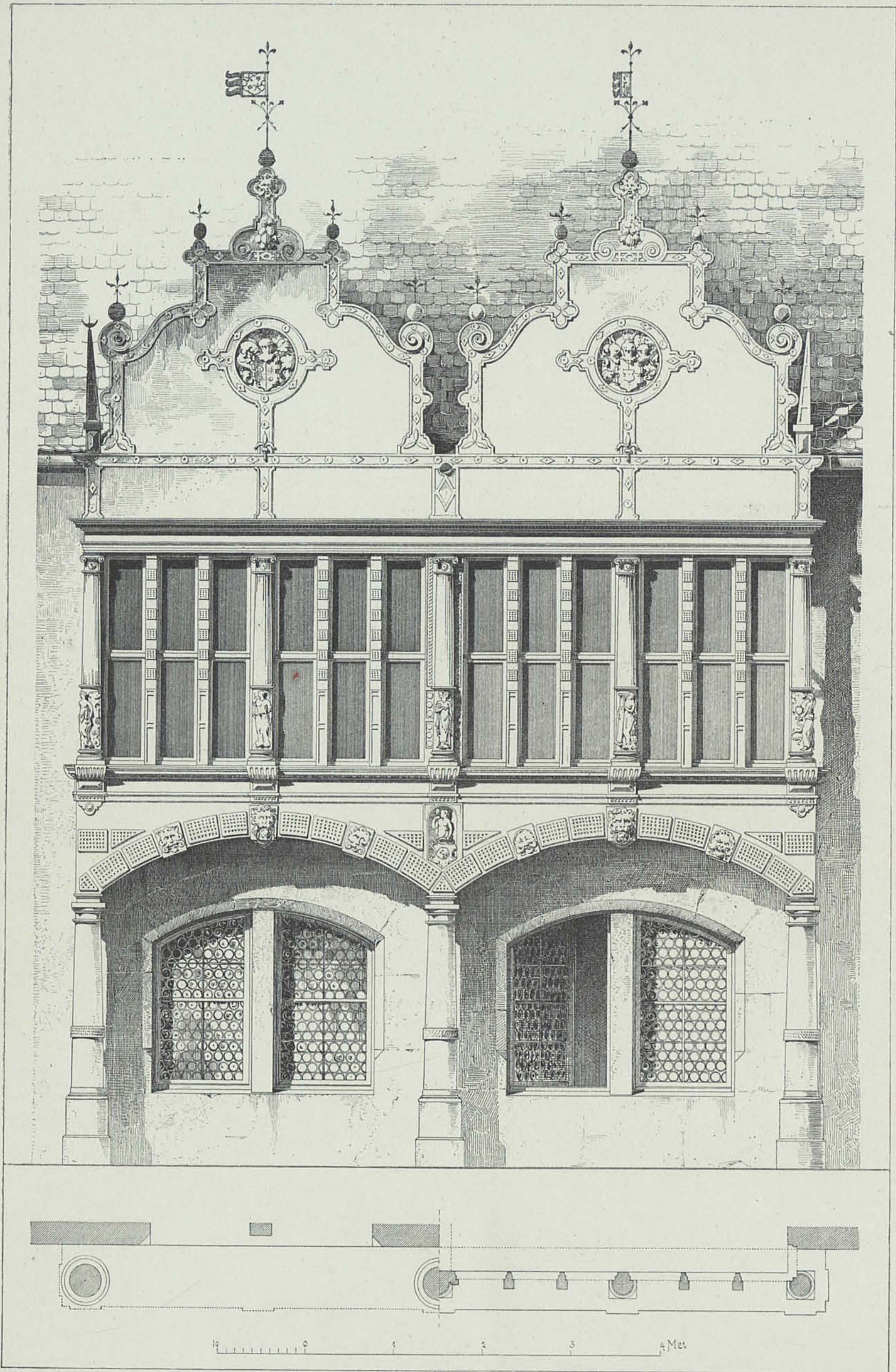
ERKER AM RATHAUS.
