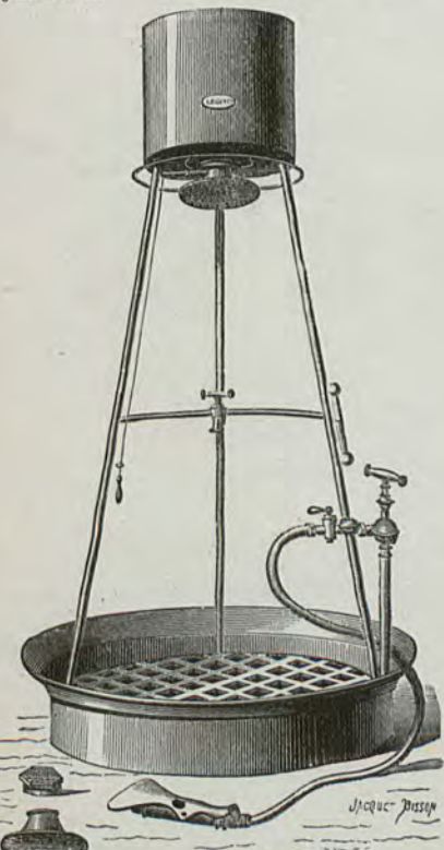
N° 5. Appareils pour Douches à pression d'air ayant 2 m 55 de hauteur sur 92 cent. de diamètre, contenant 40 litres d'eau sous pression de trois atmosphères, composé de la douche en pluie et d'une douche en jet mobile avec 2 pommes d'arrosoir, lance à 2 jets à spatule.
