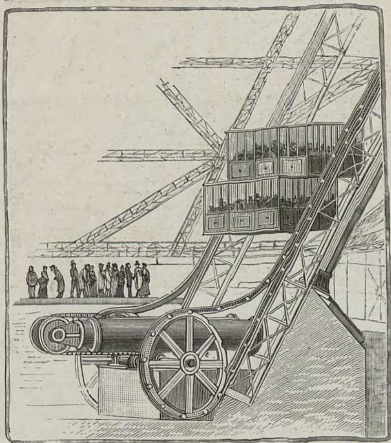
LA CAGE DE L'ASCENSEUR ROUX-COMBALUZIER.
