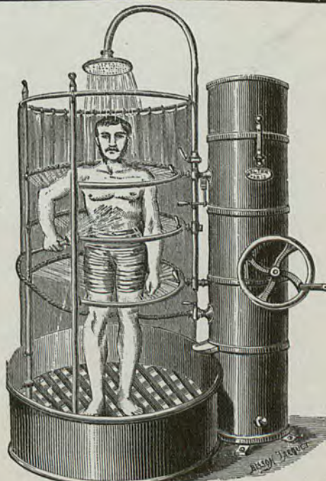
N° 8. Appareils pour Douches à pression d'air, de 2 m 40 de hauteur sur 1 m 50 de longueur et 82 cent. de largeur, contenant 150 litres d'eau sous pression de trois atmosphères, et composé de la douche en pluie, de trois douches en cercles à 3 rangées de trous chaque cercle, d'une douche locale mobile avec deux pommes d'arrosoir et lance à deux jets à spatule, de la pompe à double effet et d'un manomètre.
