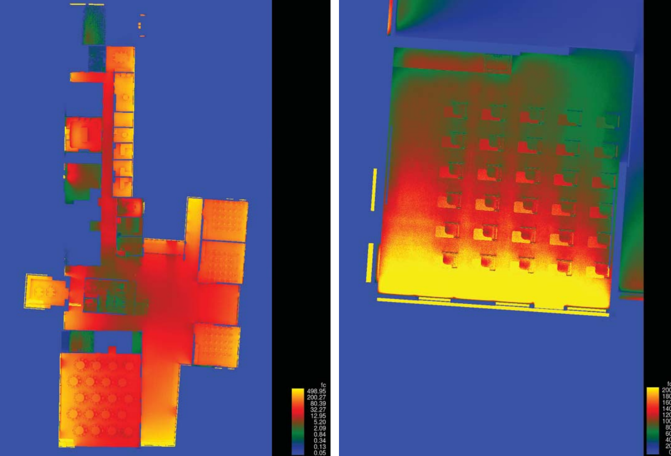
Il. 7. Analiza oświetlenia, Widok z góry pomieszczeń budynku i analiza ich naświetlenia światłem naturalnym. Autor: arch. Wojciech Cieplucha / Lighting analysis, View from the top of a building's rooms with analysis of their exposure to natural light. Author: Wojciech Cieplucha, MSc Eng.
