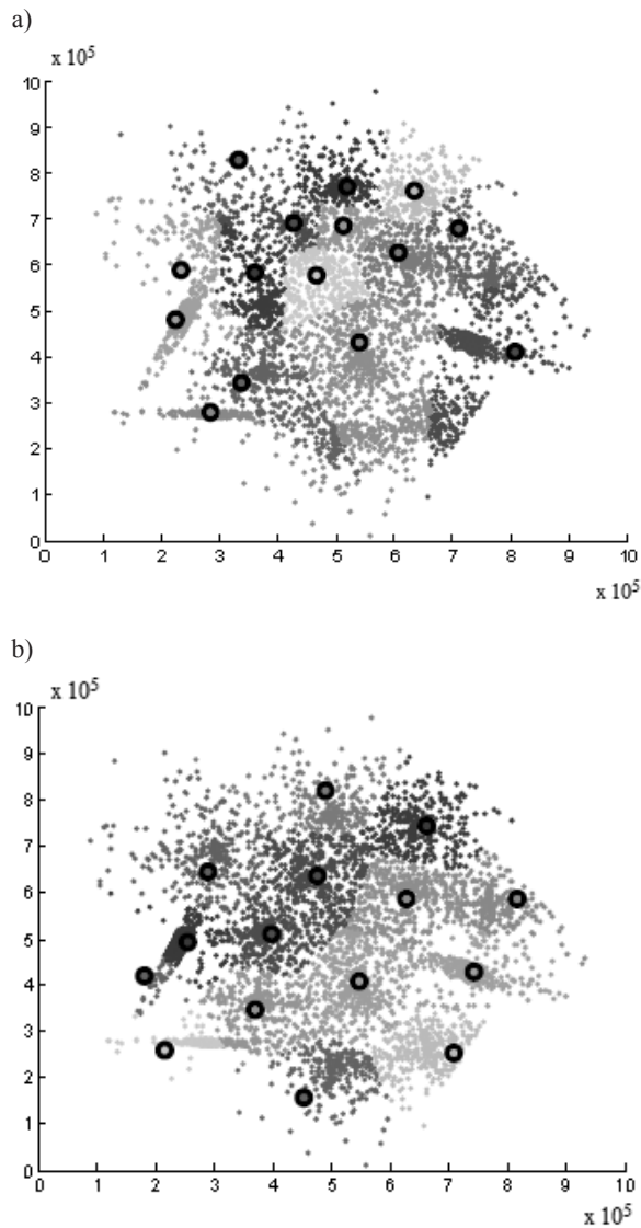
Rys. 3. Porównanie rozkładu środków klastrow dla pierwszej iteracji (a) i rozwiązania po 100 iteracjach (b) algorytmu PSO z liniową redukcją współczynnika inercji
