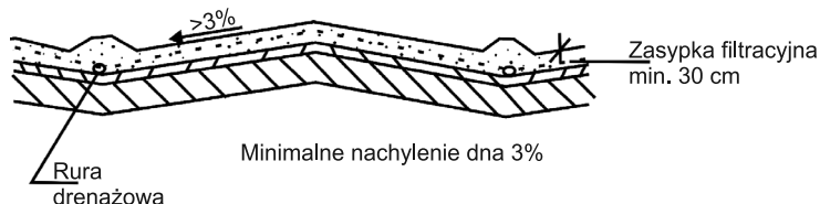
Rys. 3. Sposób układania drenażu odcieków [6]
