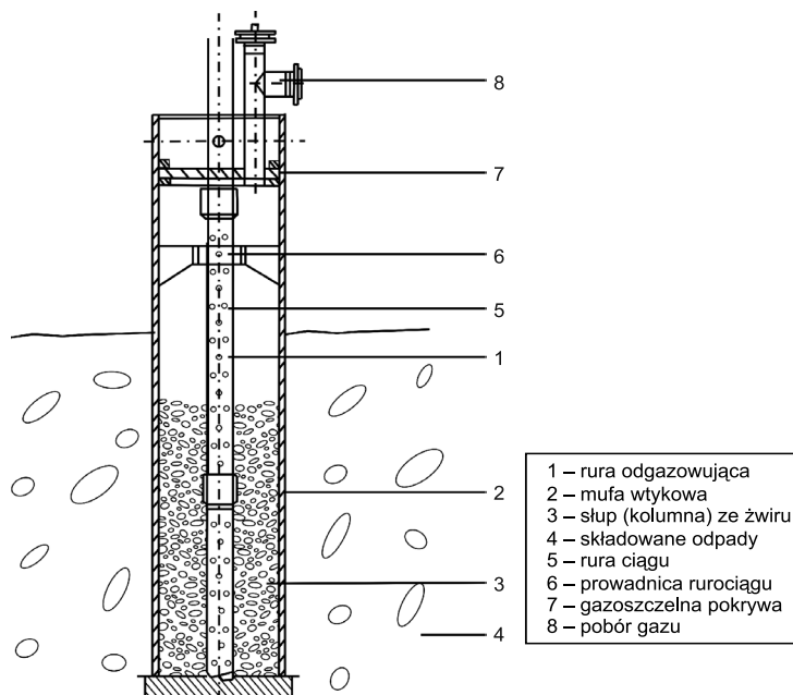
Rys. 7. Konstrukcja studni gazowej podwyższonej w miarę układania kolejnych warstw odpadów [11]
