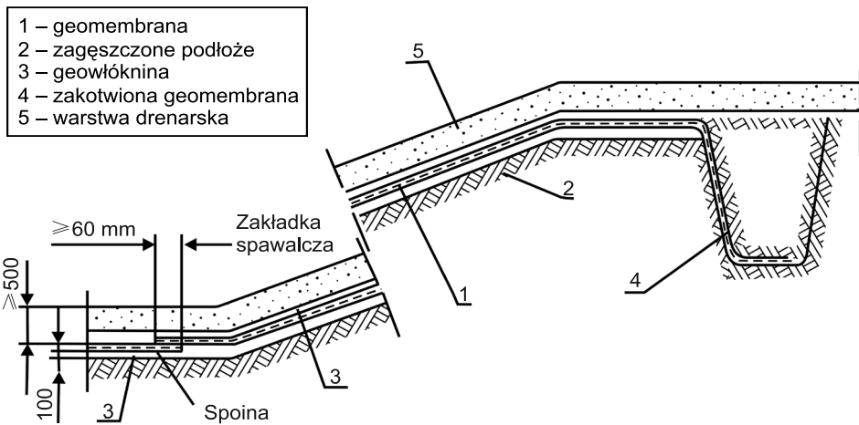
Rys. 2. Przekrój podłoża i skarpy składowiska – kotwienie [5]
