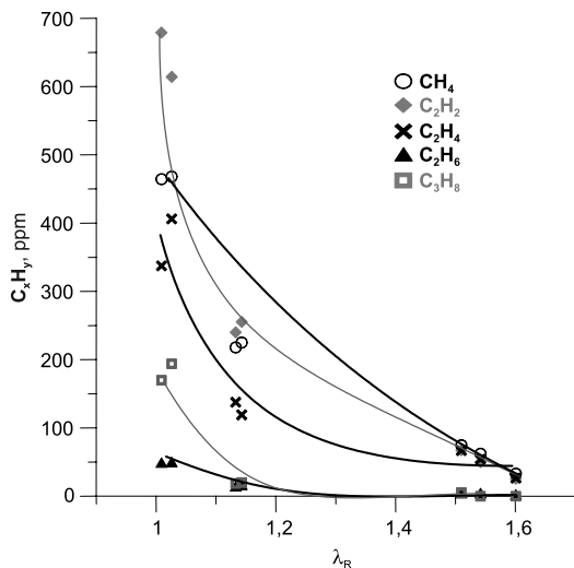
Rys. 5. Średnie stężenia związków organicznych typu \text{C}_x\text{H}_y w zależności od średniego współczynnika nadmiaru powietrza w strefie reburningu
