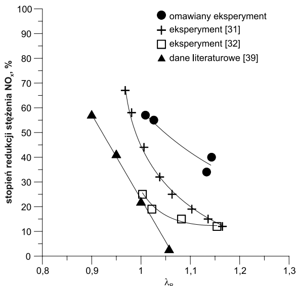
Rys. 7. Średni stopień redukcji stężenia \text{NO}_x jako funkcja średniego współczynnika nadmiaru powietrza w strefie reburningu odniesiony do porównywalnych warunków, unormowane na \text{O}_2 = 0\% w spalinach
