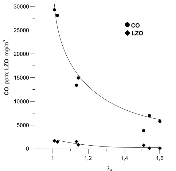
Rys. 3. Średnie stężenia tlenku węgla i lotnych związków organicznych w zależności od średnich współczynników nadmiaru powietrza w strefie reburningu
