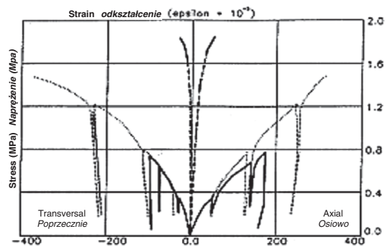
Fig. 10. Comparison of structural behaviour using injections and jacketing [7] Rys. 10. Porównanie zachowania się konstrukcji przy użyciu iniekcji i osłony płaszcza [7].
