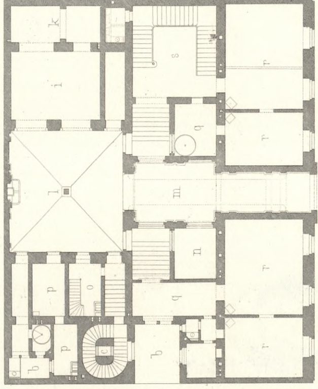
A. SOUS-SOL. B. REZ-DE-CHAUSSEE.
