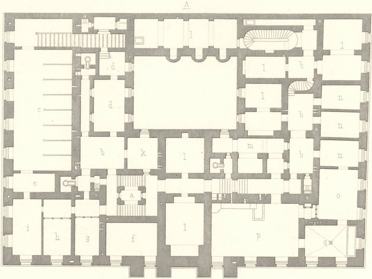
A. UNTERGESCHOSS.
