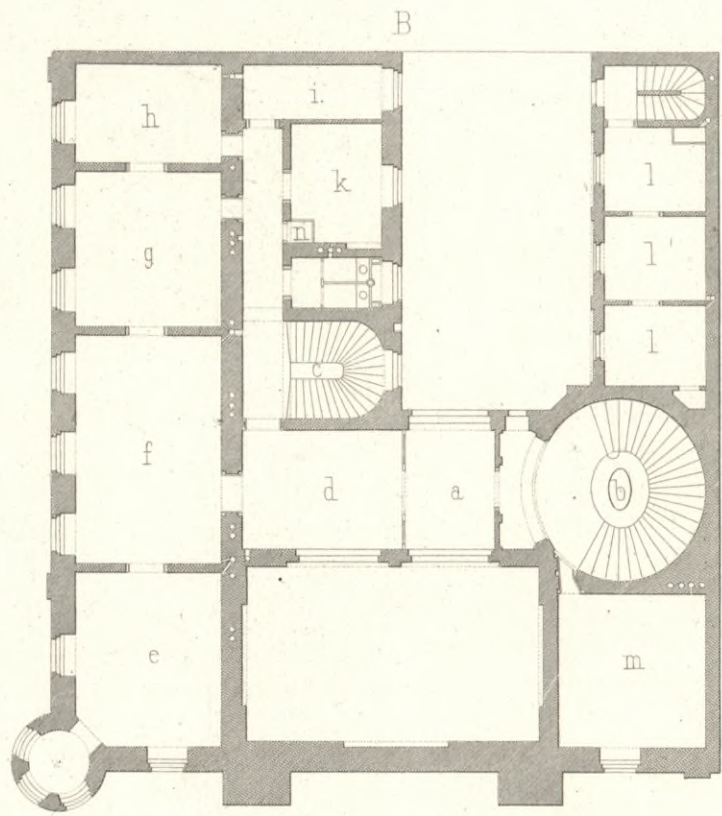
B. ZWISCHENGESCHOSS
