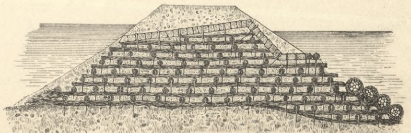
ABSCHLUSS EINES STROMARMES
