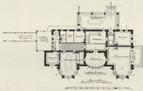
Проектъ загороднаго дома для графа А. Ф. Гейденъ (въ Подольск. губ.). П. А. ФОМИНЪ, Архитект.
