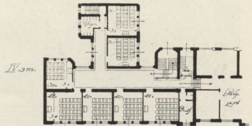
Конкурсъ на составленіе проекта училища при реформатской церкви въ С.П.Бургѣ. (Премія). С. В. БЪЛЯЕВЪ, Архитект.-Художн.
