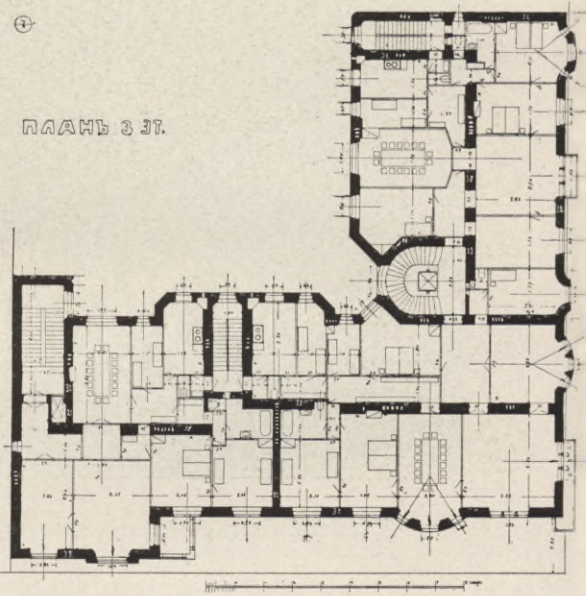
Доходн. домъ, Каменноостровскій пр., № 57-2, С.П.Бургъ. Ф. И. ЛИДВАЛЬ, Архитект.-Художн.
