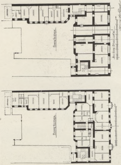
Домовый домъ, Вас. Остр., 2 линия, № 29, С.П.Бурго. Е. С. фонъ-ПОСЛЕДСЬ, Архитект.-Художн.
