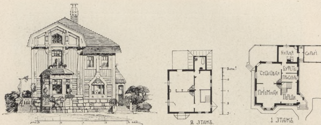
Проектъ деревяннаго особняка на Крестовскомъ Остр. въ С.П.Бургѣ. Э. А. ГУСТАВСОНЪ, Архитект.-Художн.
