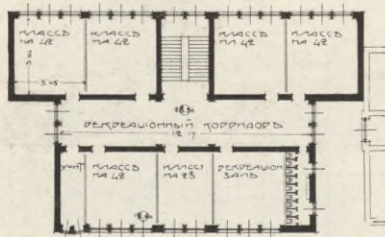
ПЛАНЪ 3 ЭТАЖА [начало и концы школы] площадь 1 классова
