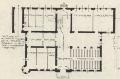
ПЛАНЪ 1 ЭТАЖА
