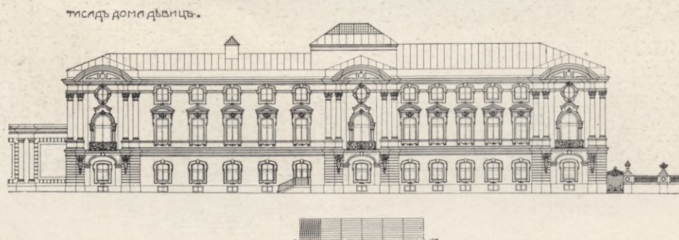
„Смоленый монастырь“, постр. граф. Растрелли въ 1758—1757 гг. Обмѣры съ натуры. Е. С. ПАВЛОВЪ, Архитект.-Художн.
