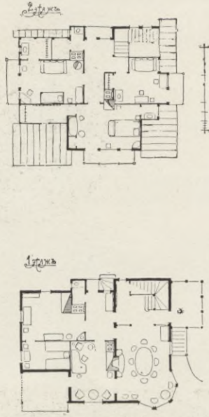
Дача на Дюнахъ, близъ Сестрорязки. Д. А. КРЫЖАНОВСКИ, Архитект.-Художн.
