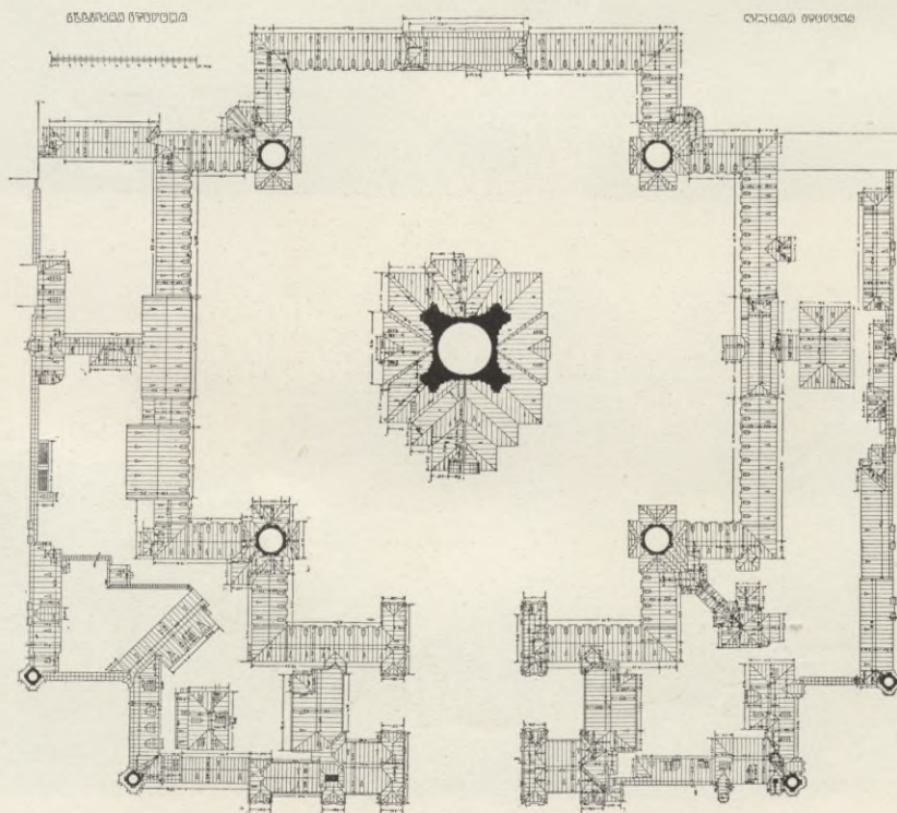
„Смоленый монастырь“, постр. гр. Растрелли въ 1748—1757 гг. Обмѣры съ натуры. Е. С. ПАВЛОВЪ, Архитект.-Художн.
