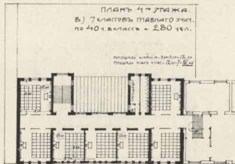
Конкурсъ на составленіе проекта училища при реформатской церкви въ С.П.Бурзъ. (Премія). М. М. ПЕРЕТЯКОВИЧЪ, Архитект.-Художн. и Гражд. Инжен.
