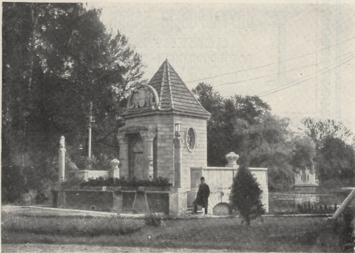
Лавильонъ фирмы Бодо Эгесторфъ на Художественно-Строительной Выставкѣ 1908 г., построенъ изъ бетонныхъ пустотѣлыхъ фасадныхъ камней.
