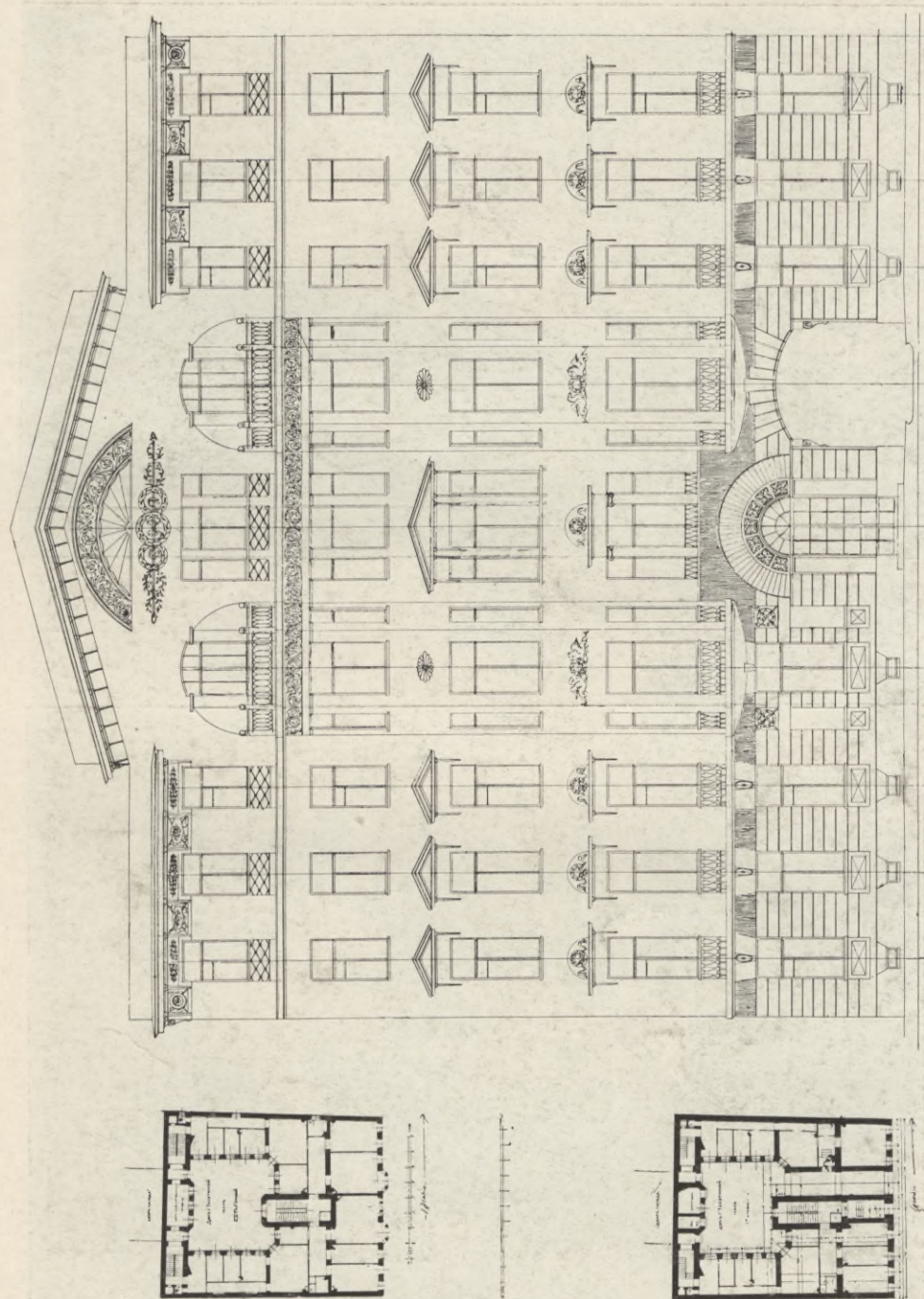
Проектъ дождяго дома Л. И. Чаломинной въ С.П.Бурге. Л. Л. ШРЕТТЕРЪ, Архитект.-Художн.
