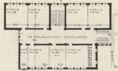
ПЛАНЪ 4 ЭТАЖА [училище] площадь 1 классова
