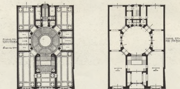
Проектъ торговаго дома въ С.-Петербургу. М. В. ЛЯЛЕВИЧЪ, Архитект.-Художн.
