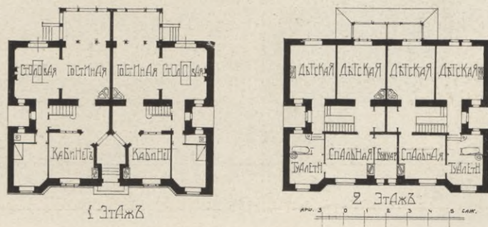
Проектъ дожднаго дома на Крестовскомъ Остр. въ С.П.Бургѣ. Э. А. ГУСТАВСОНЪ, Архитект.-Художн.
