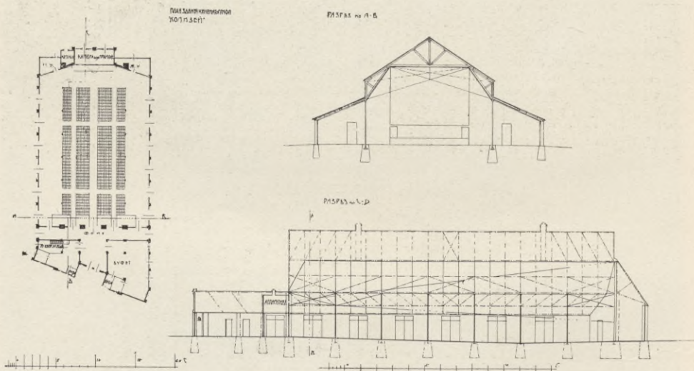
Зданіе для кинематографа „Коллизей“ въ С.П.Бургѣ. Я. Б. ГЕВИРЦЪ, Архитект.-Художн.
