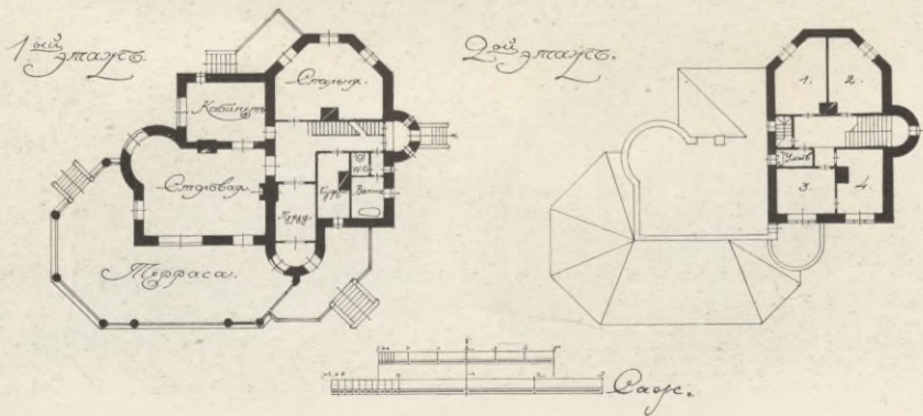
Особнякъ въ имѣніи Ф. А. Головина, Московск. губ. Ф. О. ШЕНТЕЛЬ, Академ. Архитект.
