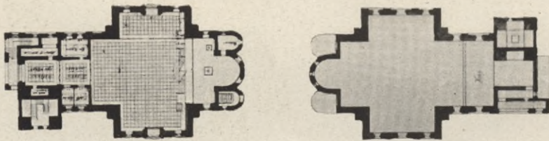
Проектъ старообрядческой церкви въ с. Балаковъ, Самарск. губ. Н. С. КУРДЮКОВЪ, Архитект.-Художн.
