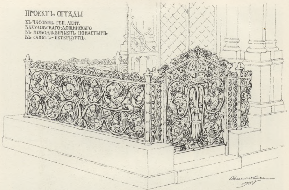
Проектъ рѣшетки къ надгробной часовнѣ. В. Ф. СОЛОМОВИЧЪ, Архитект.
