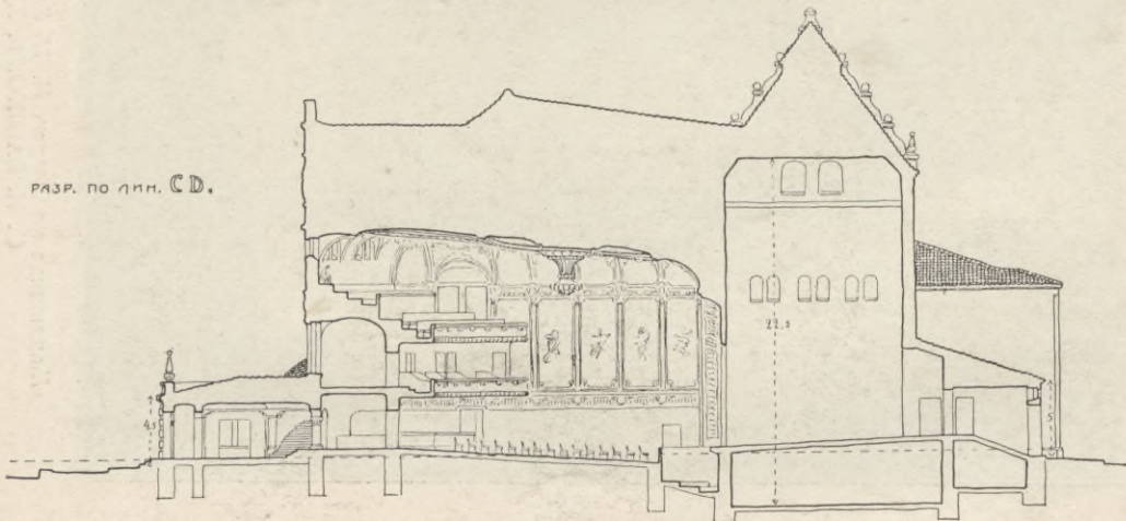
Проектъ театра для провинціального города въ Остзейскомъ краѣ. С. В. БЪЛЪЯЕВЪ, Архитект.-Художн.
