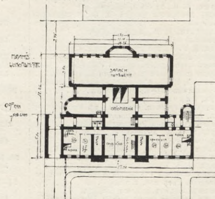
Конкурсъ на составленіе проекта училища при реформатской церкви въ С.П.Бурге. (Премія). П. П. СВѢТЛИЦКІЙ, Архитект.-Художн.
