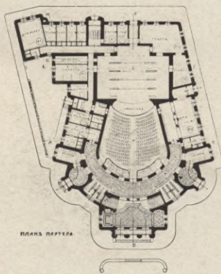
Проектъ театра для провинціального города въ Остзейскомъ краѣ. С. В. БЪЛЯЕВЪ, Архитект.-Художн.
