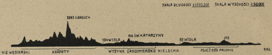
Rys. 1. Przekrój przez ziemię dawnej Polski z południa na północ na zachodzie obszaru. (Podług mapy O. Sosnowskiego).
