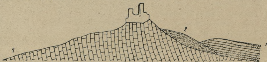
Rys. 45. Schemat budowy geologicznej góry Zamkowej w Chęcinach. (jedna część antyklinali, podług Sobolewa).
