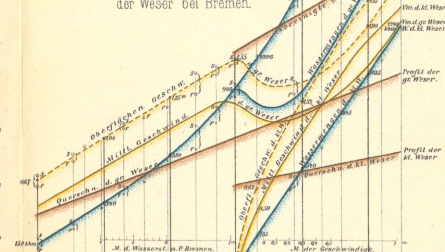
Fig. 14 b Graphische Darstellung der Geschwindigkeiten, Profile und Wassermengen der Weser bei Bremen.
