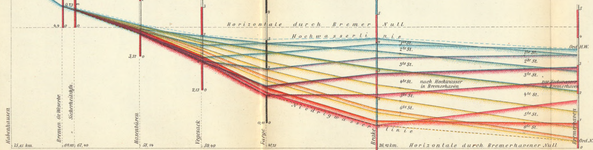
Fig. 3 Flutwellen der Weser nach der Korrektur bei normaler Flut und mittlerem Oberwasser von 0,73 m Br. P.
