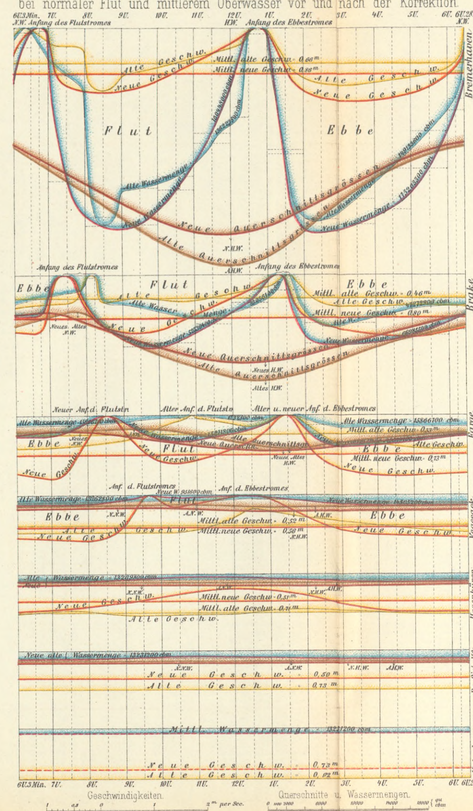
Fig. 5 Querschnitte Wassermengen und Geschwindigkeiten an den Pegelstationen bei normaler Flut und mittlerem Oberwasser vor und nach der Korrektur.
