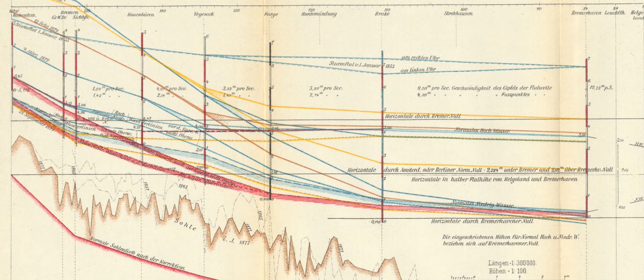
Fig. 2 Flutwellen der Weser vor der Korrektur bei normaler Flut und mittlerem Oberwasser von 0,73 m Br. P.
