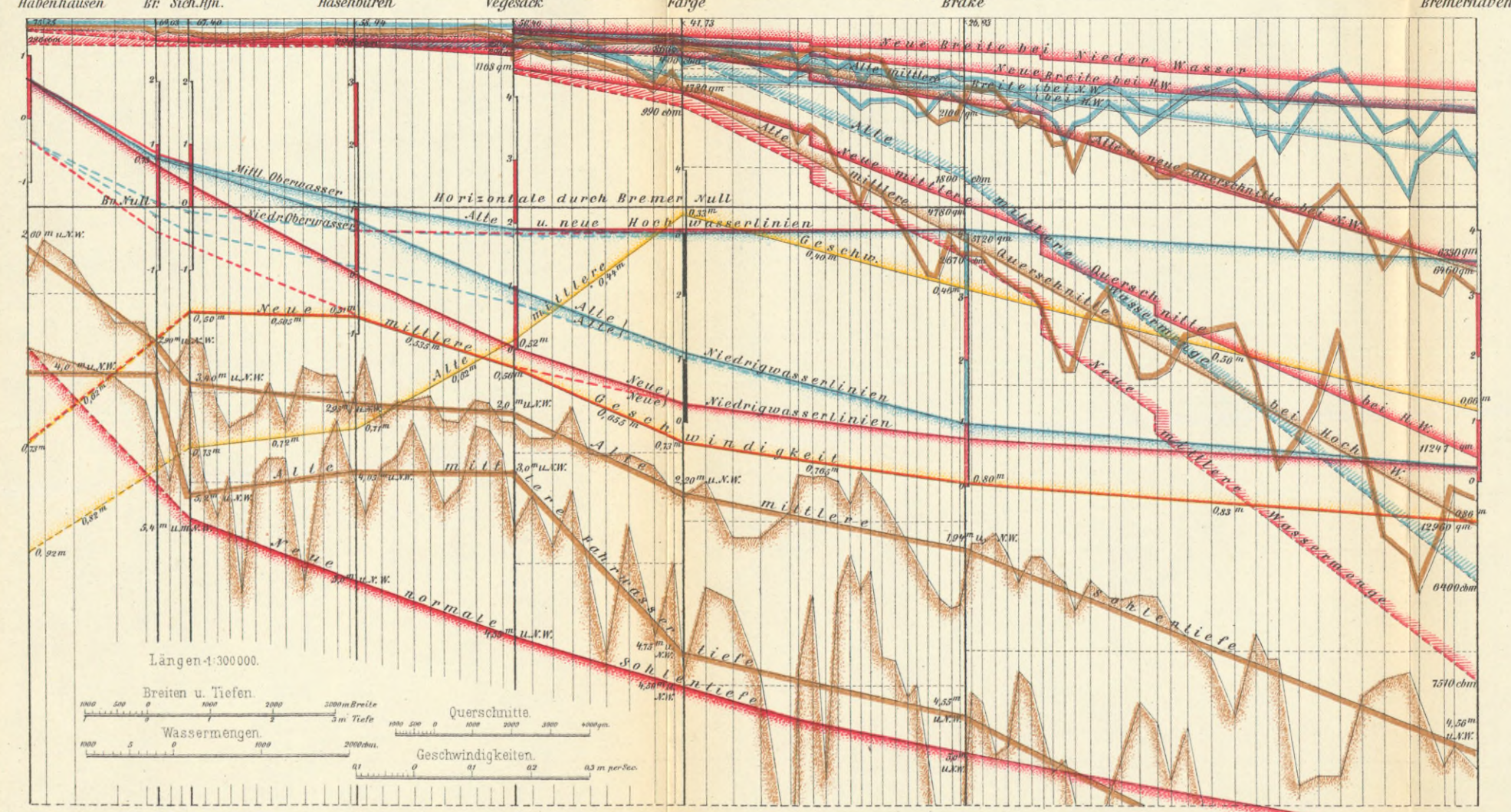
Fig. 4 Breiten, Tiefen, Querschnitte Wassermengen und Geschwindigkeiten der Unter-Weser vor und nach der Korrektur bei ordinarer Flut und mittlerem Oberwasser von 0,73 m am Pegel zu Bremen (Gr. Weserbr.)
