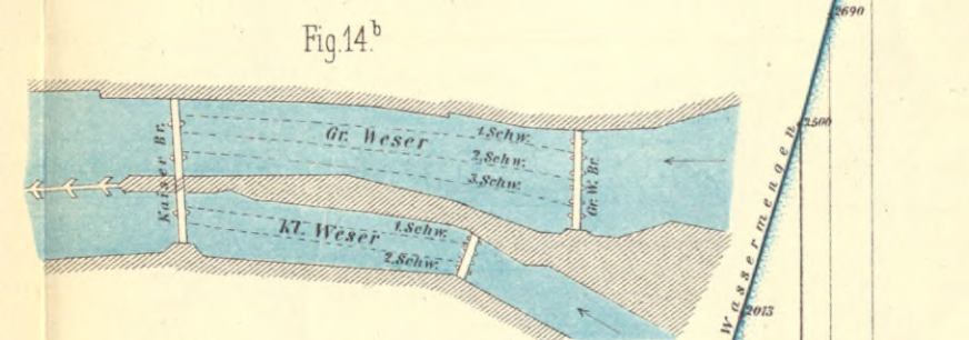
Fig. 14 b Graphische Darstellung der Geschwindigkeiten, Profile und Wassermengen der Weser bei Bremen.
