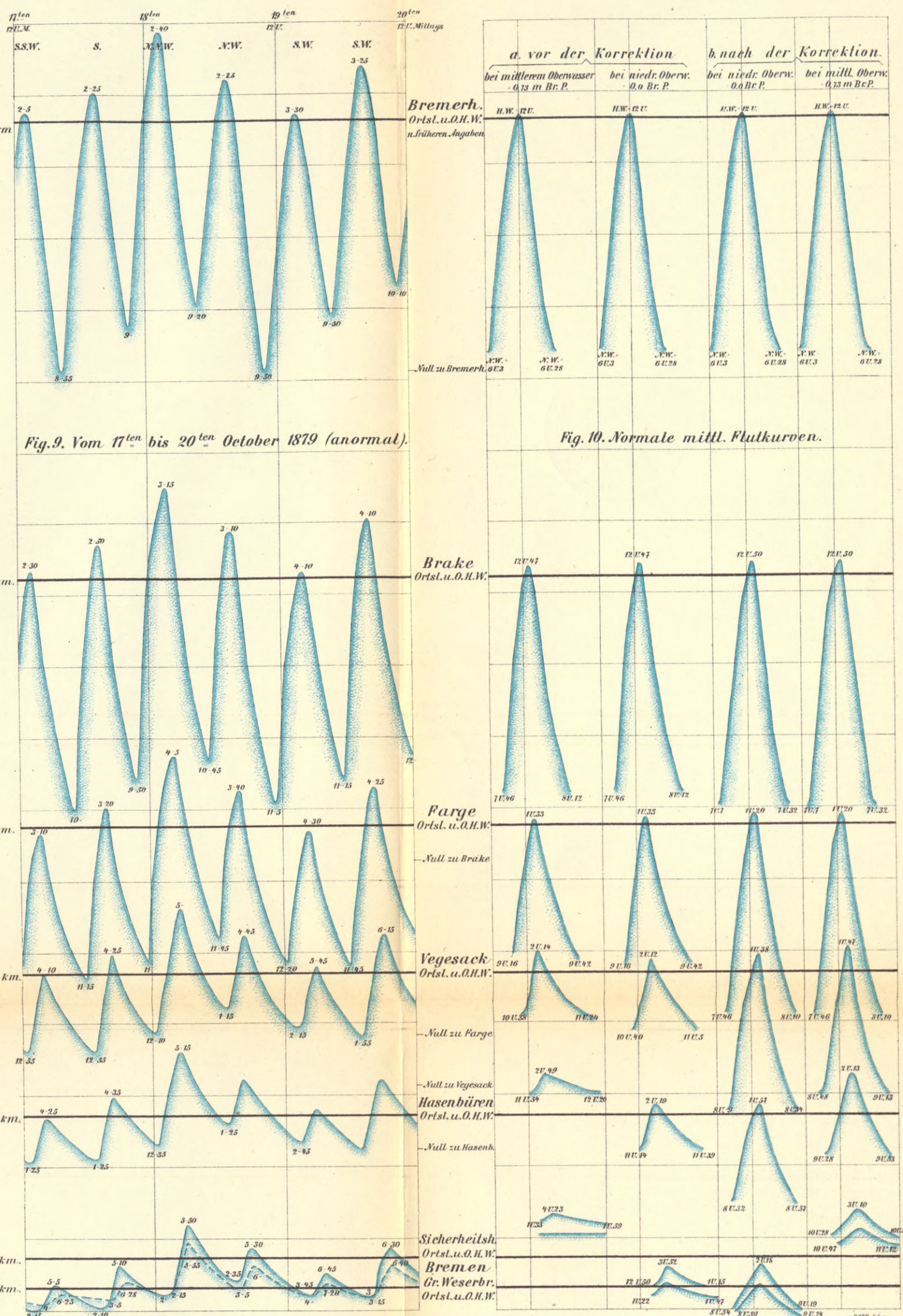
Flutkurven der Weser.
