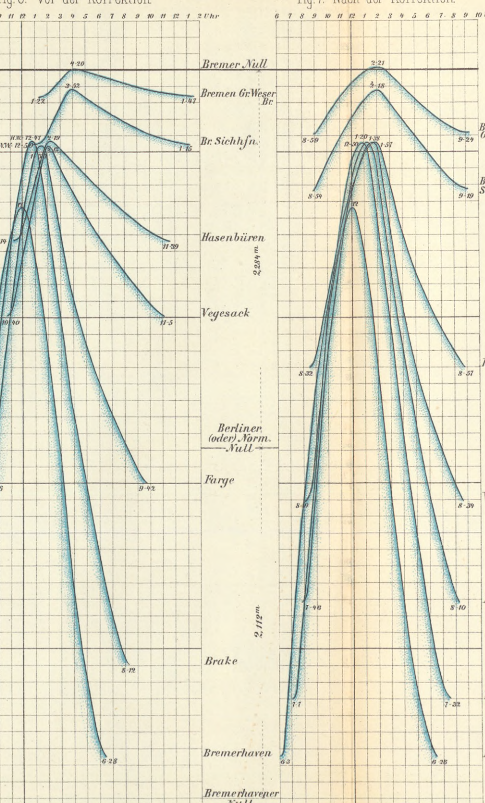
Normale Flutkurven der Weser bei niedrigem Oberwasser - 0 Br. P.
