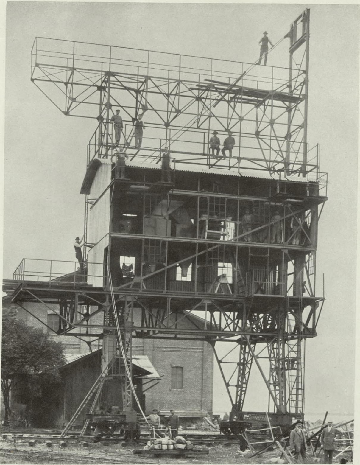
Schiffselevator während der Montierung.
