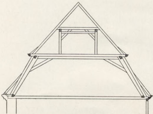
Abb. 30. Dachstuhl vom Gymnasium in Cottbus (vgl. Abb. 23)
