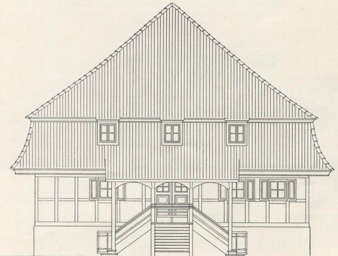
Abb. 32—33. Forsthaus vom Jagdschloß Stern bei Potsdam (vgl. Abb. 23)
