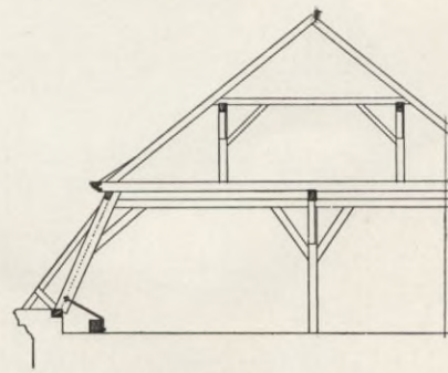
Abb. 31. Dachstuhl von der Stadtschule in Potsdam (vgl. Abb. 24)
