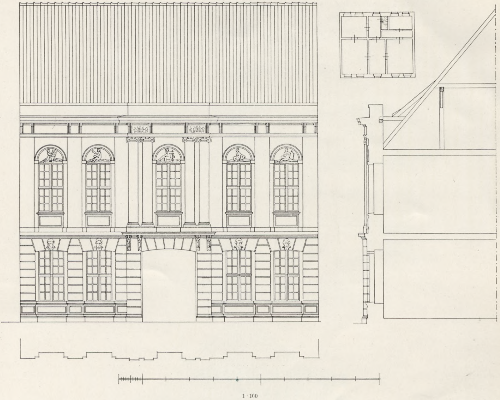
Abb. 27—29. Wohnhaus Berlin Taubenstraße (vgl. Abb. 25)
