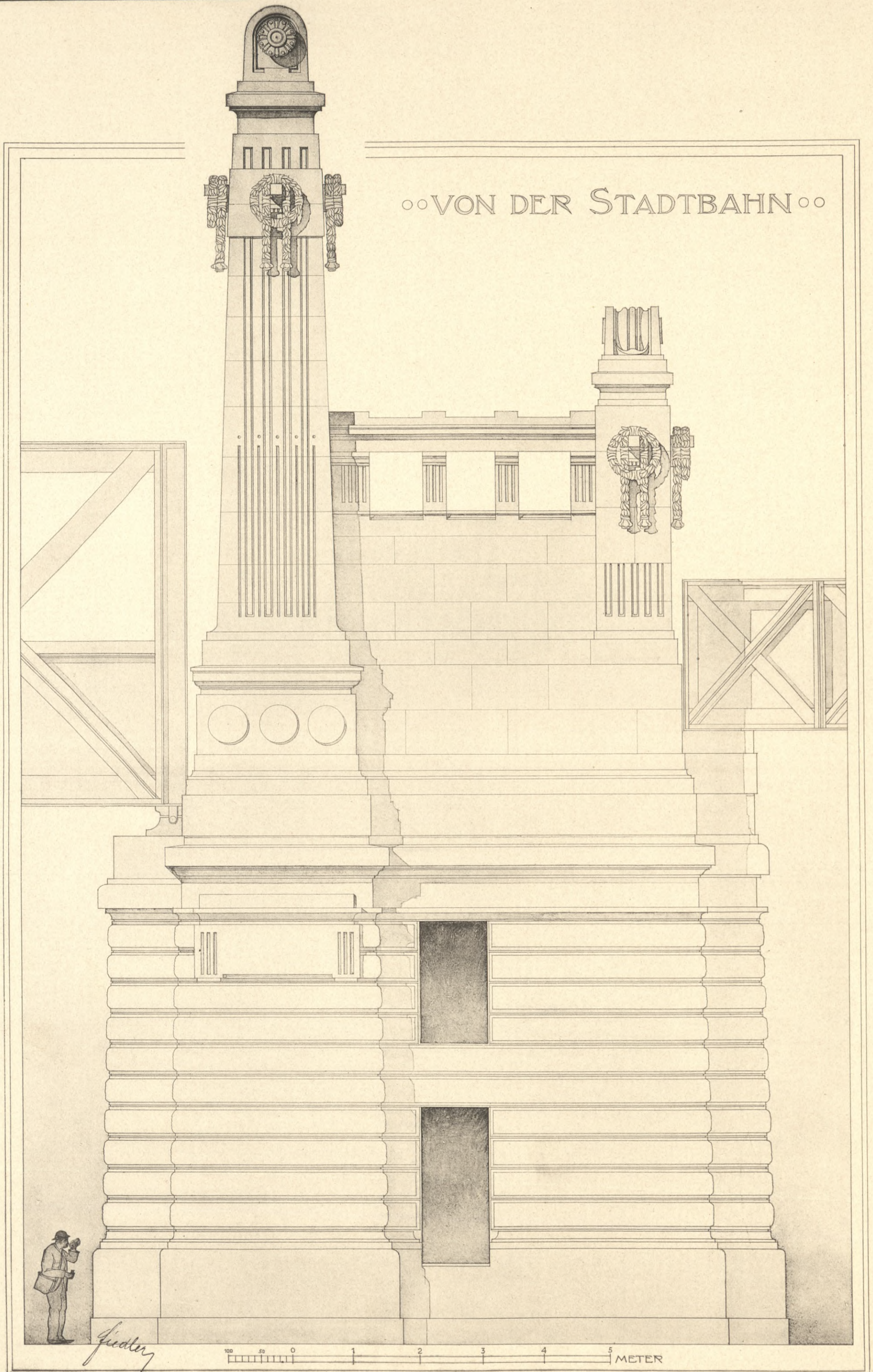
OBELISK DER MEIDLINGER STADTBAHNBRÜCKE. ≡≡≡
