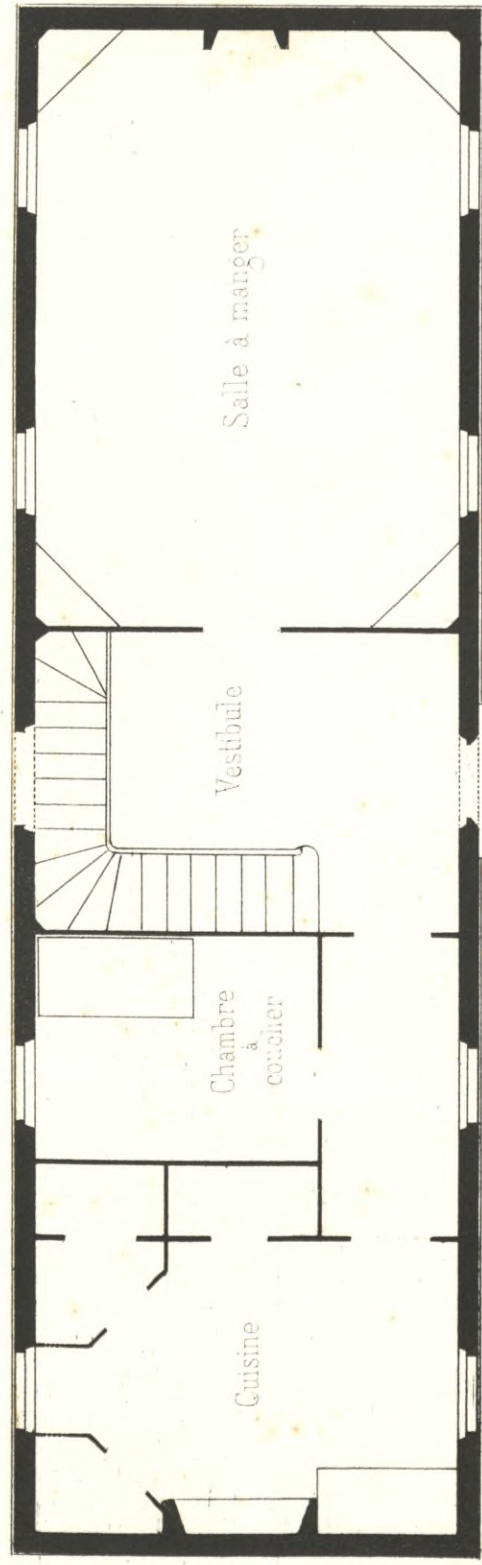
Plan du rez-de-chaussée.
