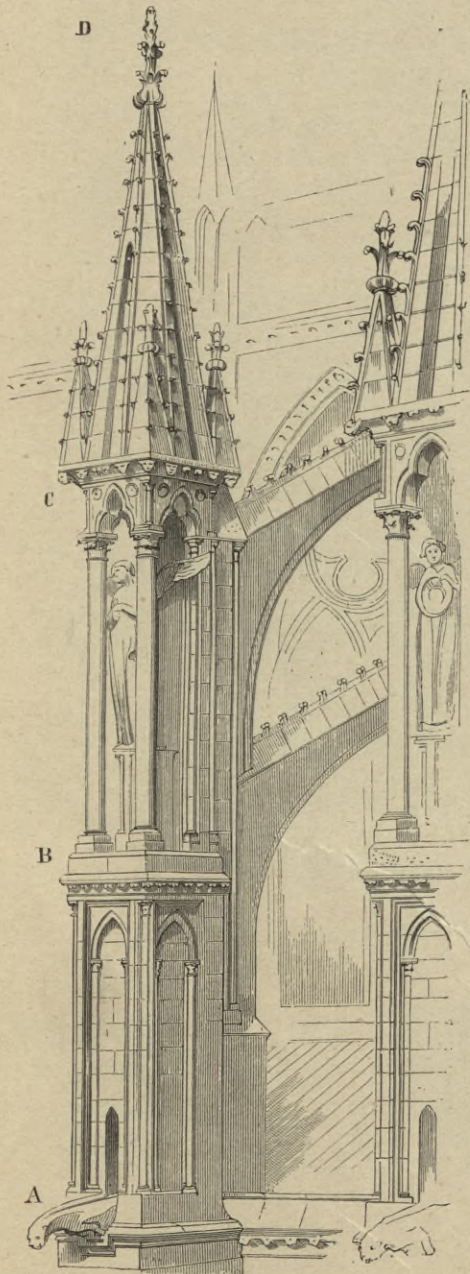
7. Strebepfeiler. (Rheims, Kathedrale.)
