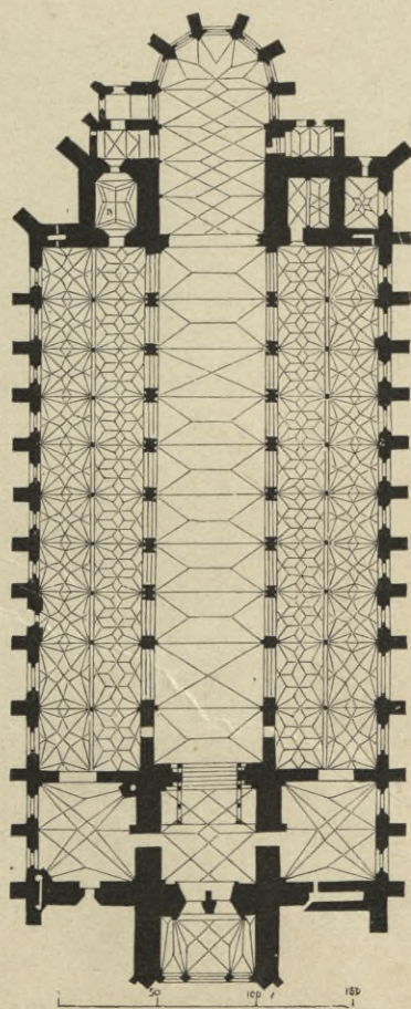
4. Münster zu Ulm. Grundriss.
