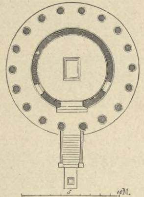
11. Rundtempel zu Tivoli.
