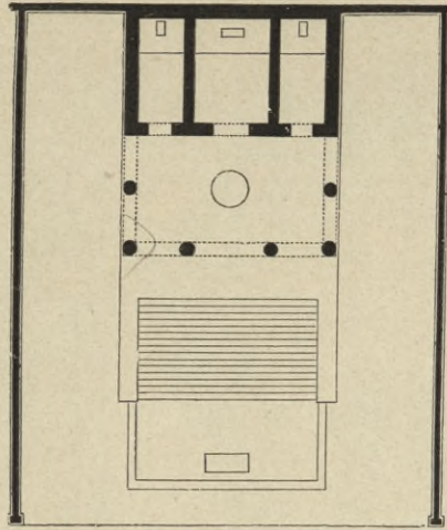
5. Grundriss des etruskischen Tempels.
