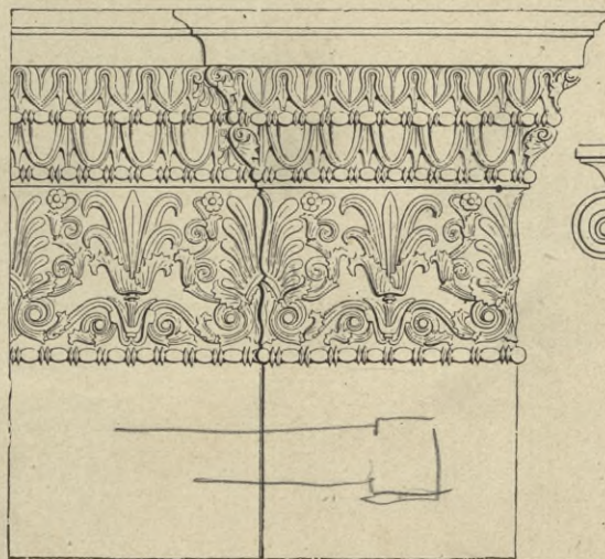
10. Kapitäl der Ante und der Wand, Erechtheion.
