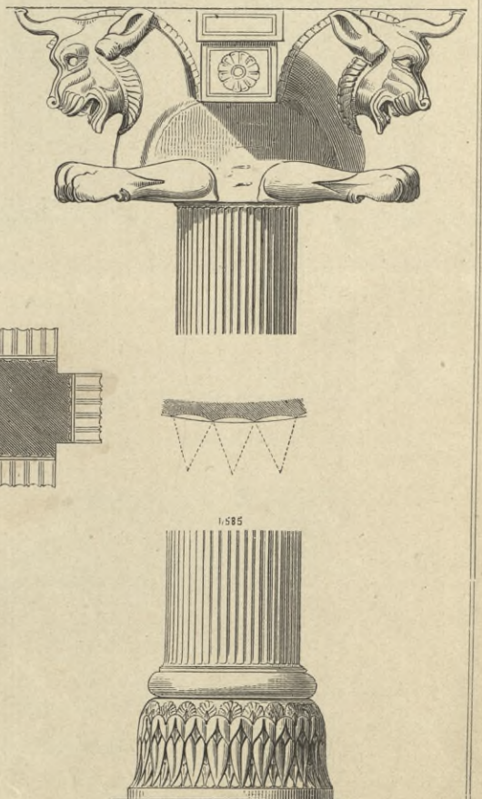
9. Säulen von der Halle des Xerxes zu Persepolis.
