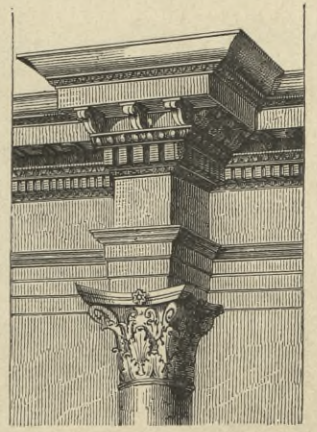
9. Verkröpftes Gebälk.
