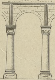
3. Arkaden der Kirche zu Paulinzelle.
