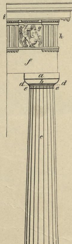
4. Aufriss der dorischen Säule samt Gebälk.
