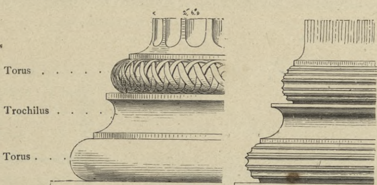
4. Säulenbasis. Von der Nordhalle des Erechtheion.
