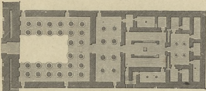
6. Tempel des Chunsu zu Karnak (Längendurchschnitt und Grundriss). 0 10 20 30 40 M.
