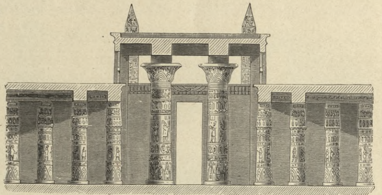
5. Tempel von Karnak. Säulensaal.
