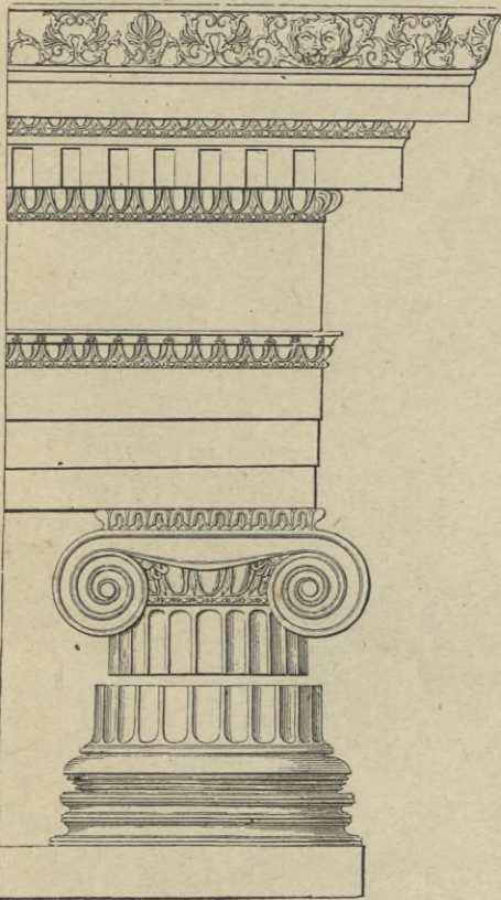
4. Ionische Ordnung. Athenetempel zu Priene.
