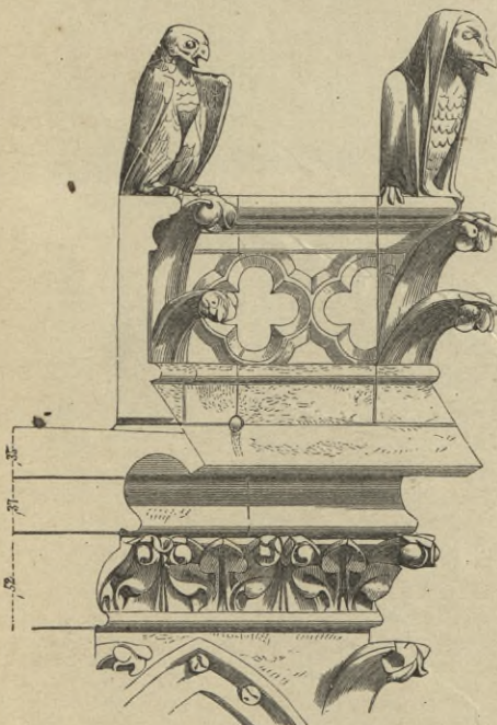
4. Sims und Balustrade. (Paris, Notre Dame.)
