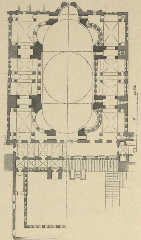
2. Grundriss der Sophienkirche.
