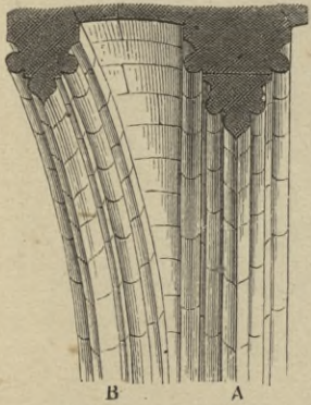
8. Gewölbeprofil. (Paris, Ste. Chapelle.)
