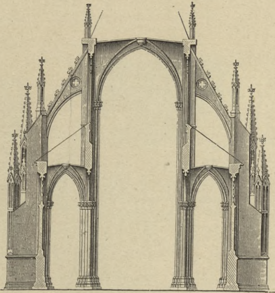
4. Querschnitt des Doms zu Halberstadt.
