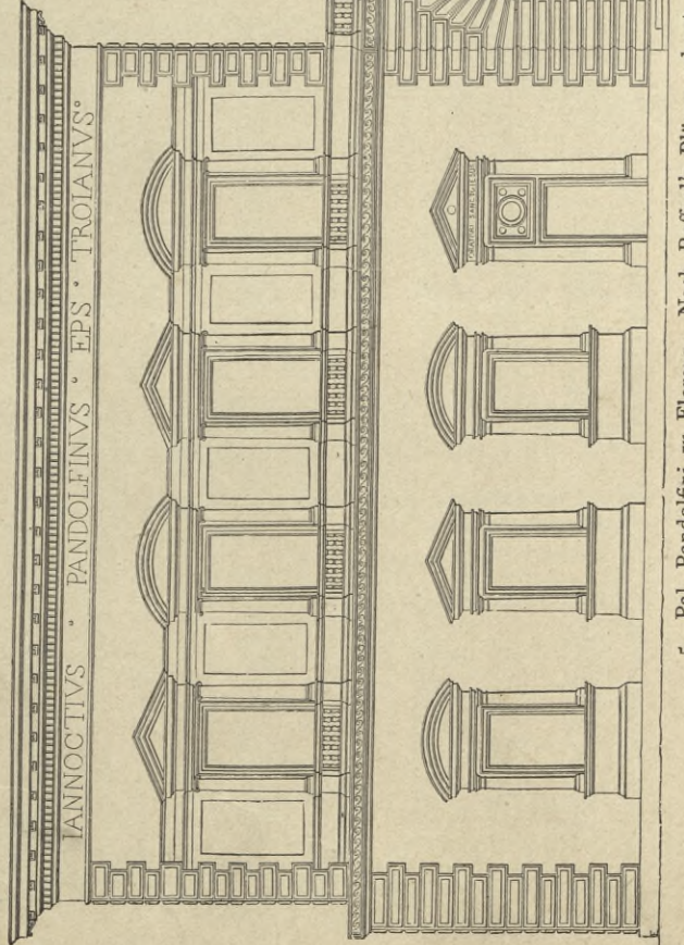
5. Pal. Pandolfini zu Florenz. Nach Raffael's Plänen erbaut. (ca. 1530.)
