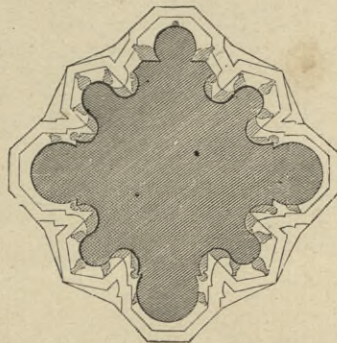
5. Grundriss eines Pfeilers vom Kölner Dom.
