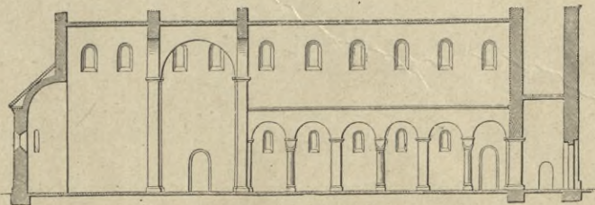
1. Längenschnitt einer romanischen Basilika.
