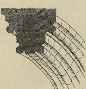
12. Gewölbeprofil. Notre Dame zu Paris.
