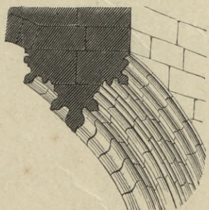
13. Gewölbeprofil. Kathedrale zu Narbonne.
