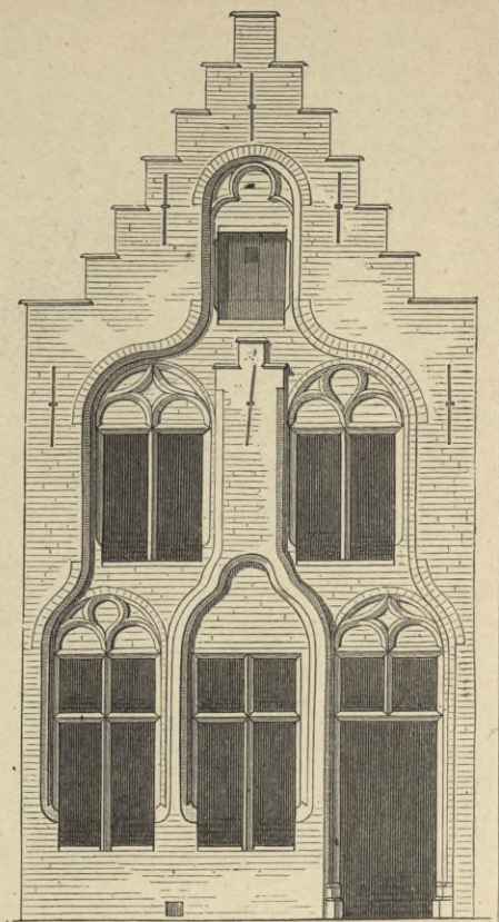
6. Haus in Brügge.
