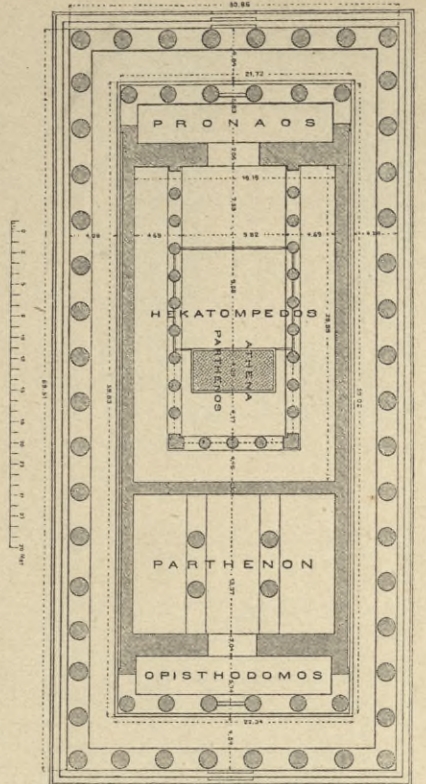
2. Grundriss des Parthenon. (Nach Dörpfeld.)
