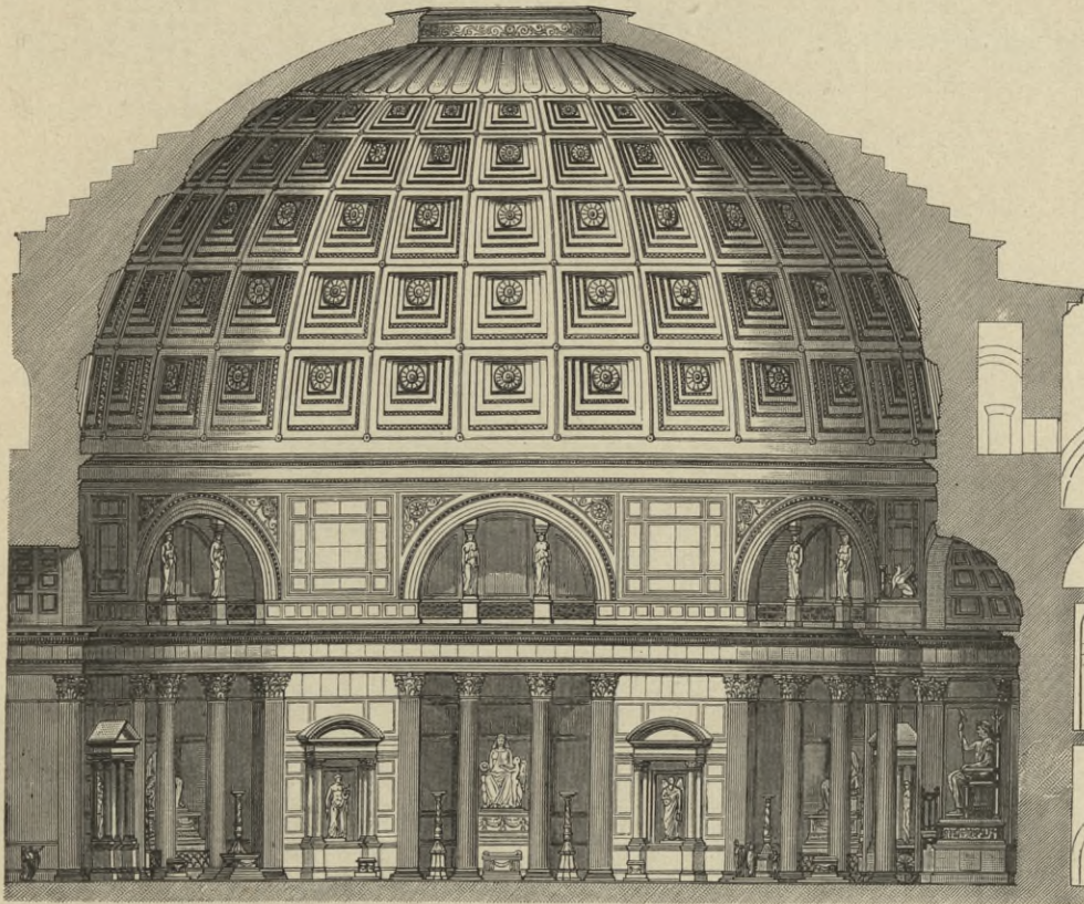
13. Durchschnitt des Pantheon, Ursprüngliche Anlage. (Nach Adler.)
