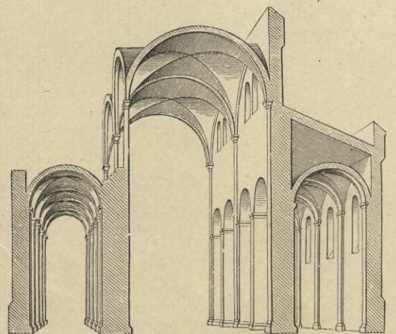
2. Romanisches Gewölbesystem.
