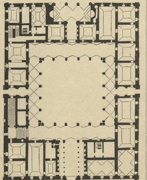
7. Pal. Farnese, Rom. (Arch.: Antonio da Sangallo j., † 1546.)
