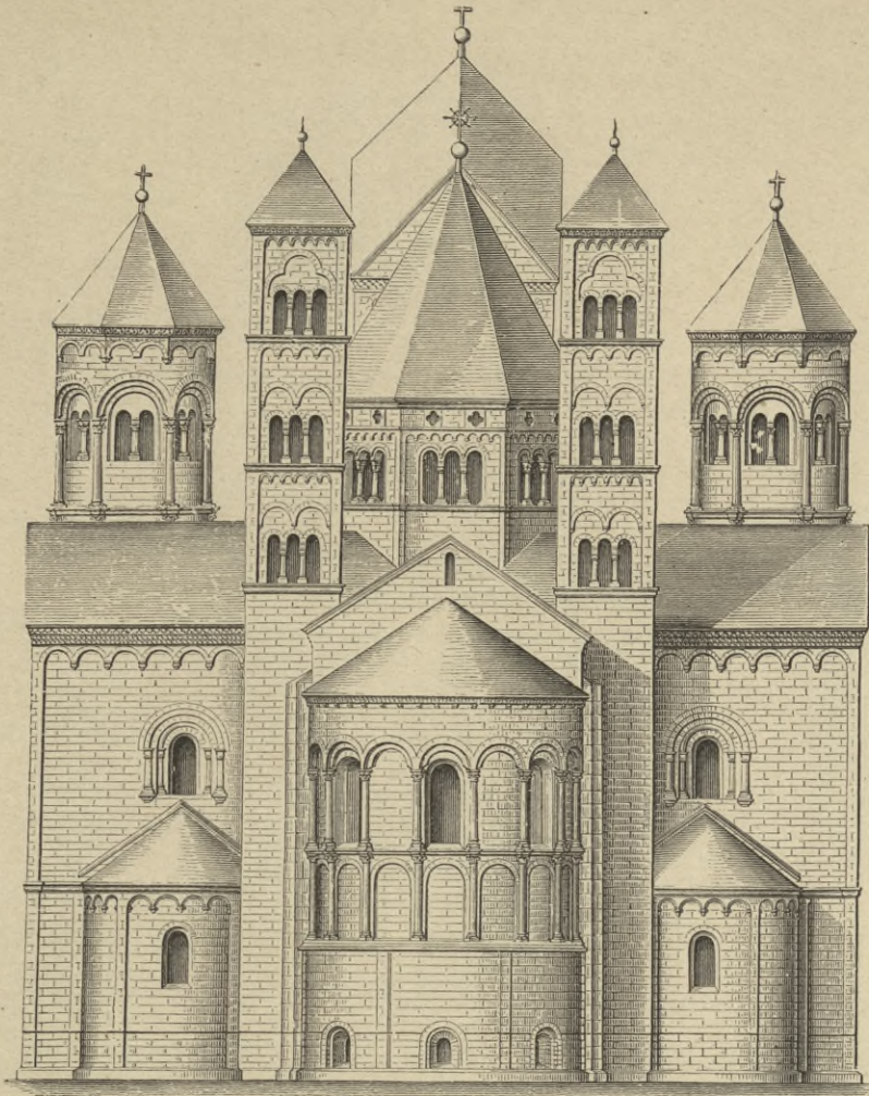
5. Abteikirche zu Laach. Oestlicher Aufriss.
