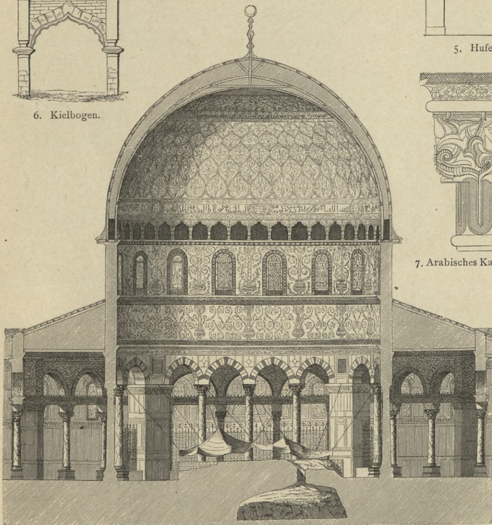
3. Durchschnitt der Sachrah-Moschee (Felsendom) zu Jerusalem. 688 n. Chr.
