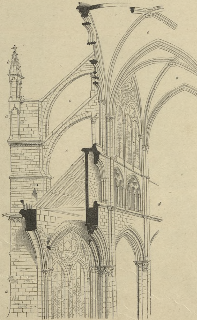
8. Kathedrale zu Amiens.
