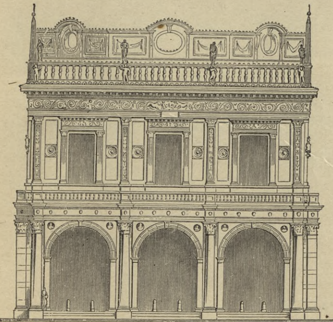
6. Pal. Comunale zu Brescia. (ca. 1508; Arch.: Formentone.)
