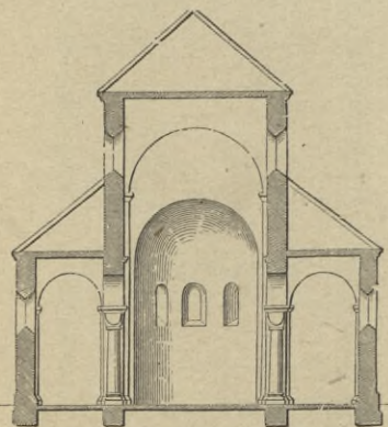
4. Querschnitt einer romanischen Basilika.
