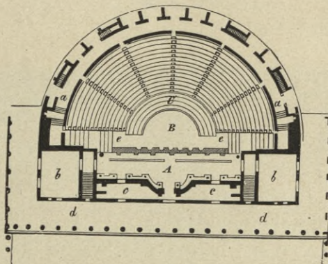
6. Theater zu Herculaneum. A. Scena. B. Orchestra. C. Sitzplätze. aa. Eingang. bb. Ankleidezimmer. c. Raum hinter der Scene. d. Arkaden. ee. Treppen.
