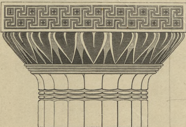
6. Bemaltes dorisches Kapitäl.
