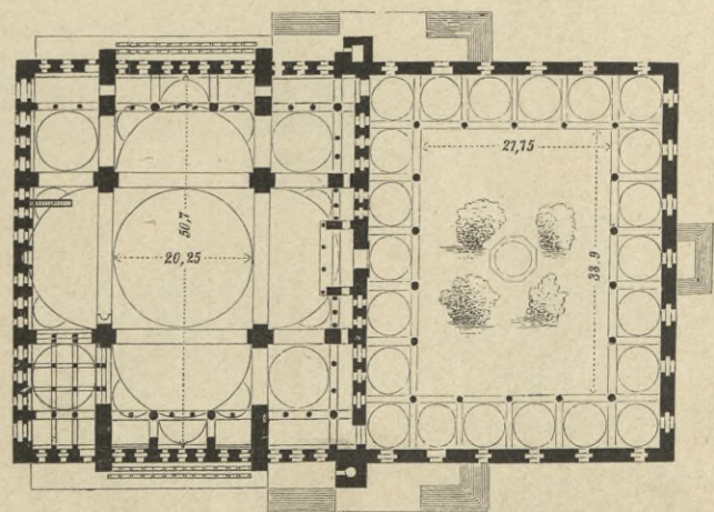
4. Mahmud's II. Moschee. Grundriss. (Constantinopel.)
