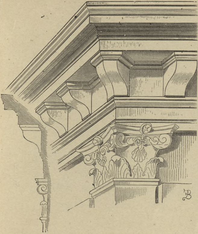
1. Kranzgesims von der Cancelleria in Rom. (Arch.: Bramante; ca. 1445-1514.)
