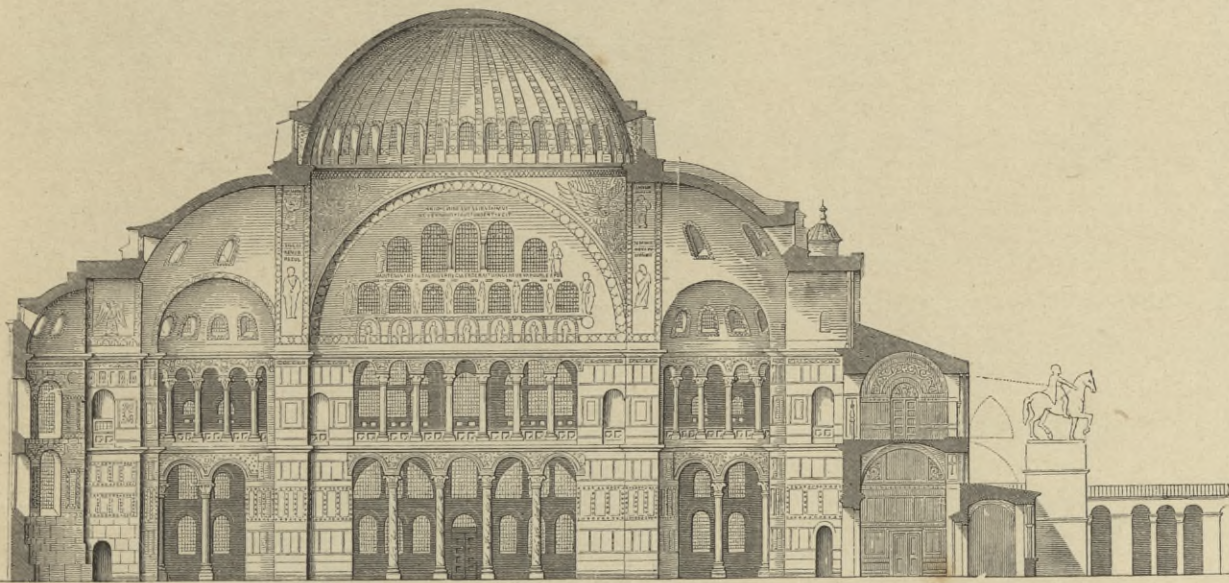
3. Längendurchschnitt der Sophienkirche.
