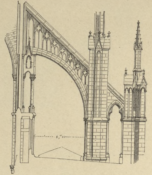
6. Strebesystem am Chor der Kathedrale zu Amiens.
