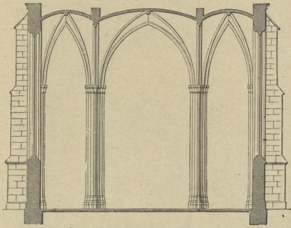
5. Querdurchschnitt einer Hallenkirche.
