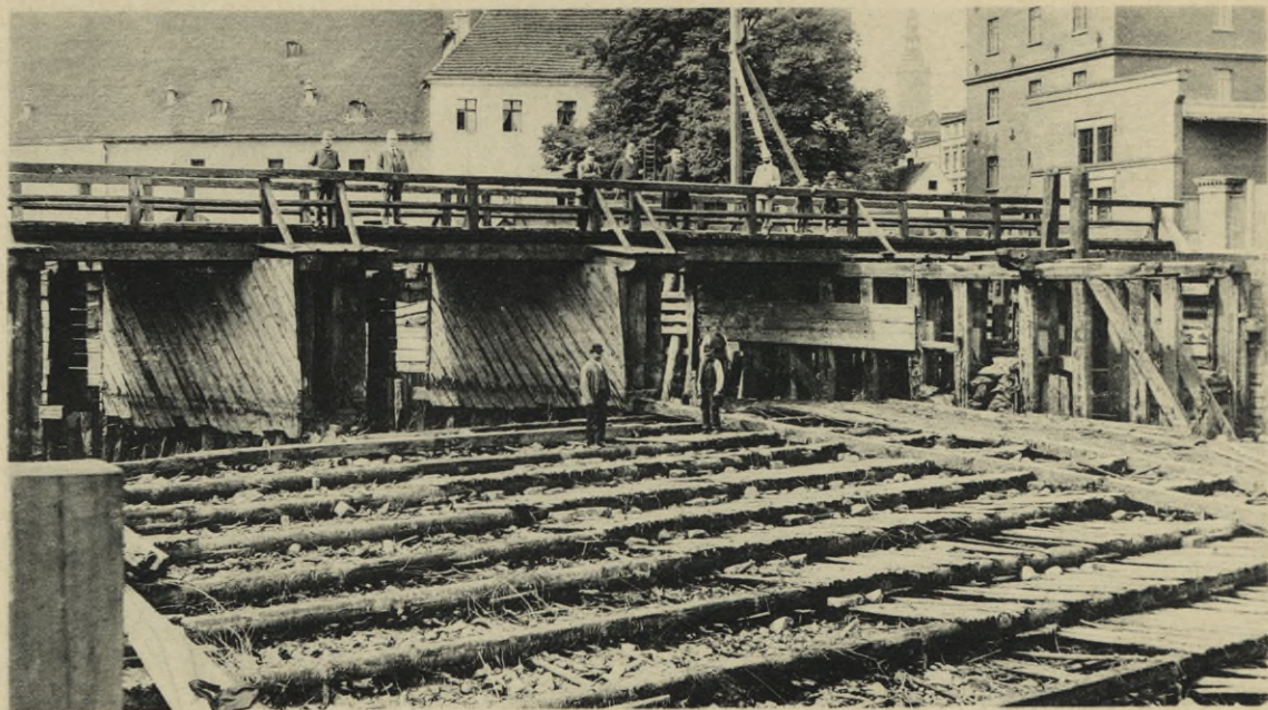
Brieg. Niederwehr vor dem Bau.
