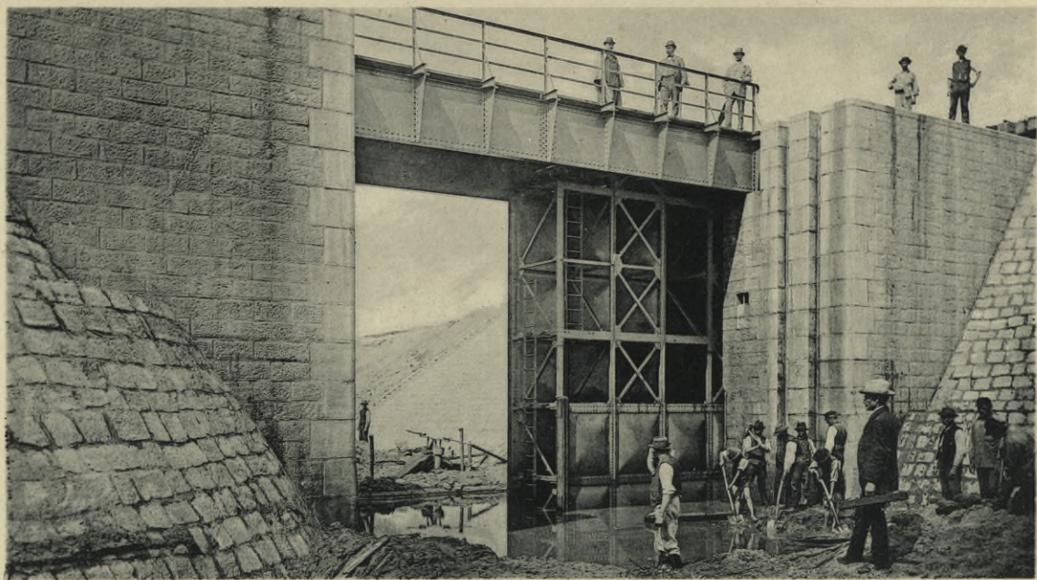
Breslau, Grossschiffahrtsweg. Fluthschleuse.
