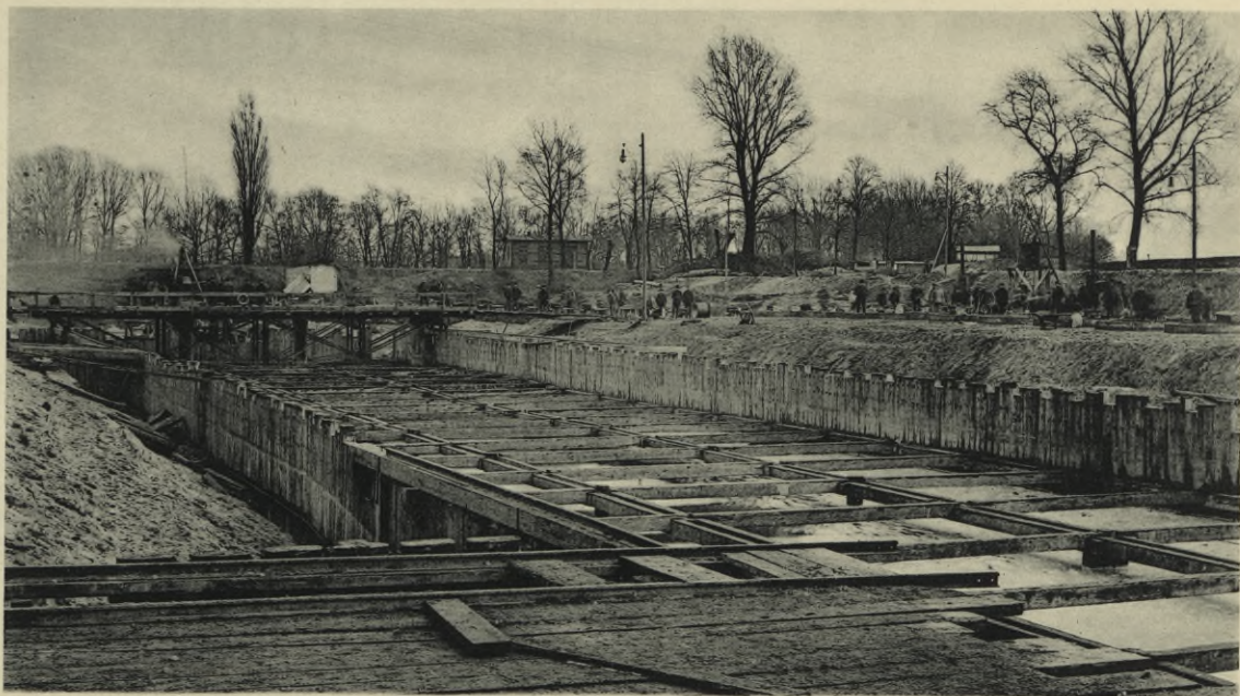
Breslau. Grossschiffahrtsweg. Betonierung der Scheitniger Schleuse.
