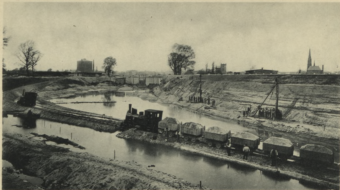
Breslau. Grossschiffahrtsweg. Scheitniger Schleuse bei Beginn des Baues.
