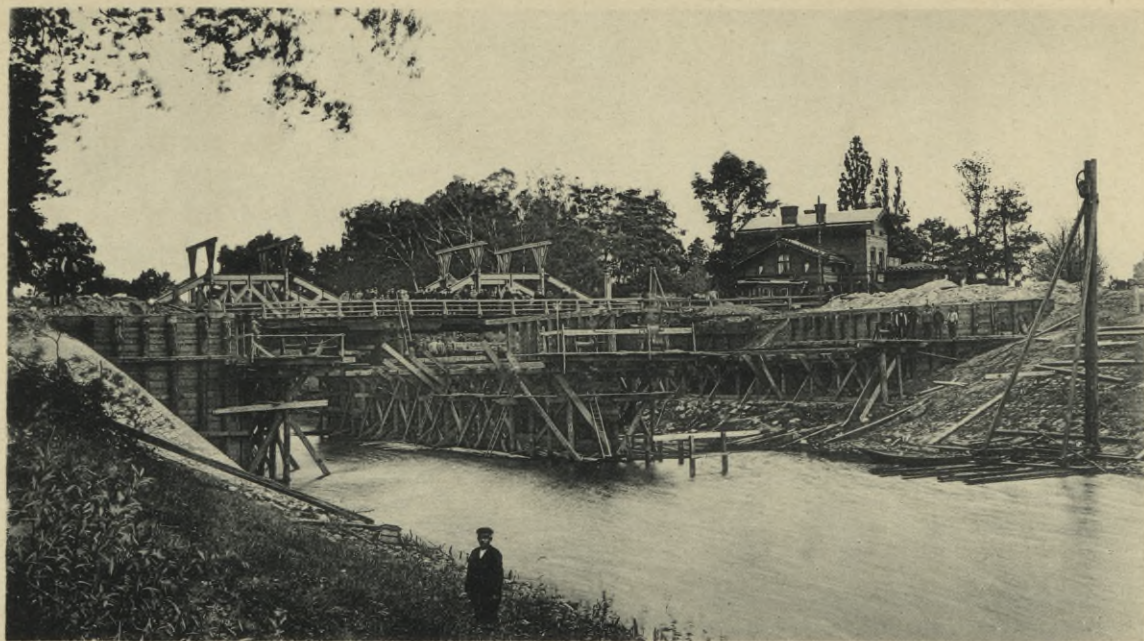
Breslau, Grossschiffahrtsweg, Alte Passbrücke mit Verschiebungsgerüst.
