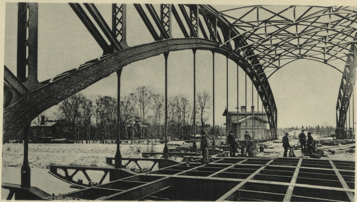
Breslau, Grossschiffahrtsweg, Passbrücke. Blick in die Construction.
