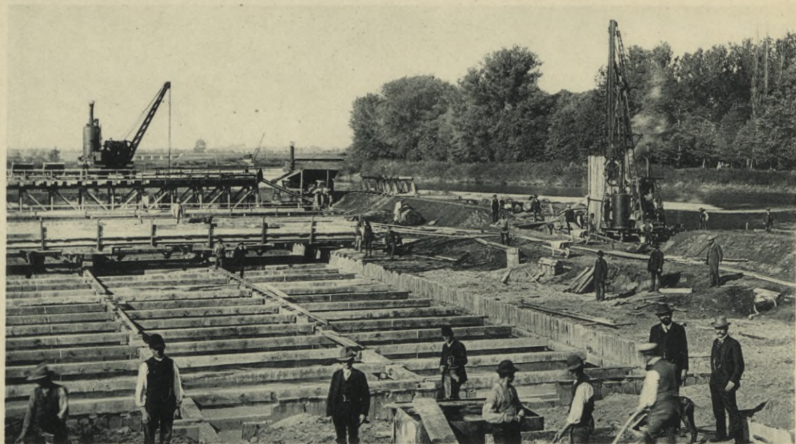
Oppeln. Neue Schleuse.
