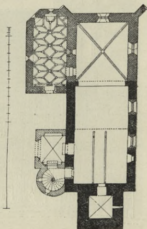
Obr. 9. Boletice. Půdorys kostela se sakristií.
