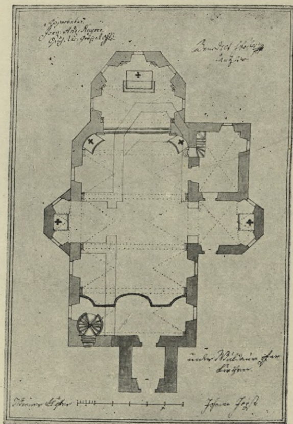
Obr. 359a. Vltavice Dolní. Půdorys kostela J. Jopsta z r. 1769.
