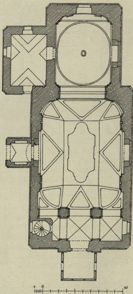
Obr. 260. Ondřejov. Pádorys nynějšího kostela.
