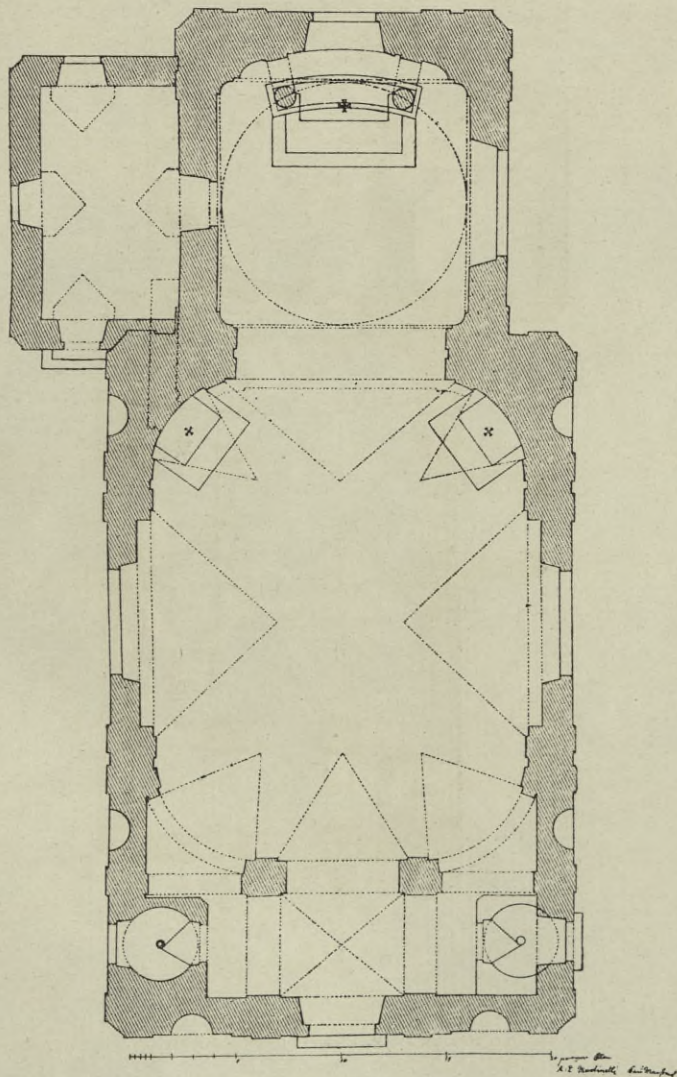
Obr. 259. Ondřejov. Půdorys kostela od Martinelliho.
