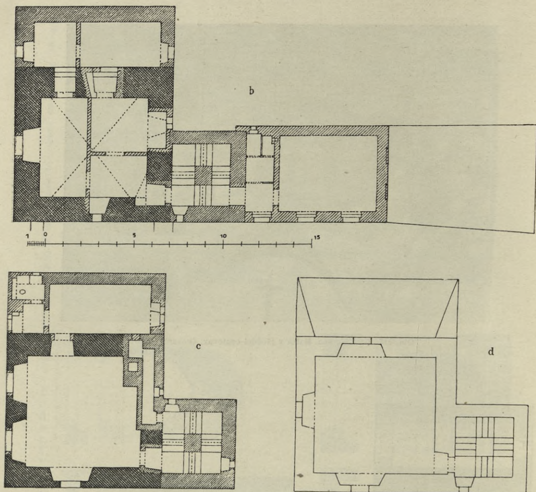
Obr. 219. Zlatá Koruna. Bašta, nyní fara: b), c), d) půdorysy přízemí 1., 2. a 3. sneseného patra.
