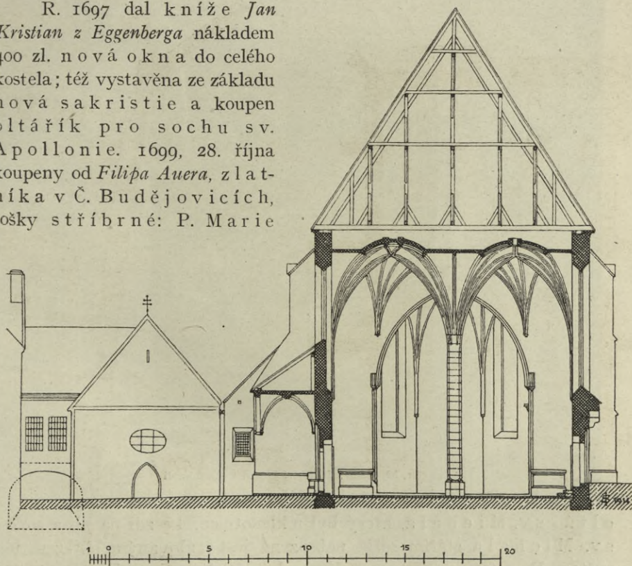
Obr. 87. Kájov. Průřez kostela.
