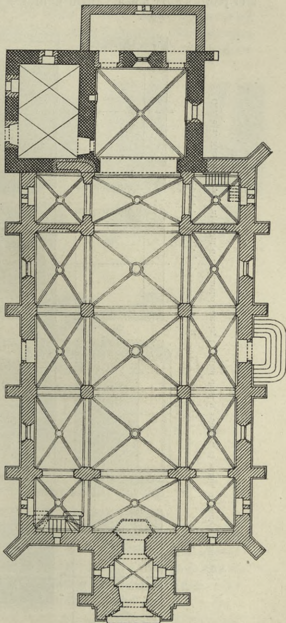
Obr. 240. Křemže. Dnešní půdorys kostela.
