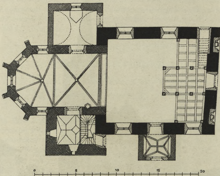
Obr. 290. Příklad. Půdorys kostela.
