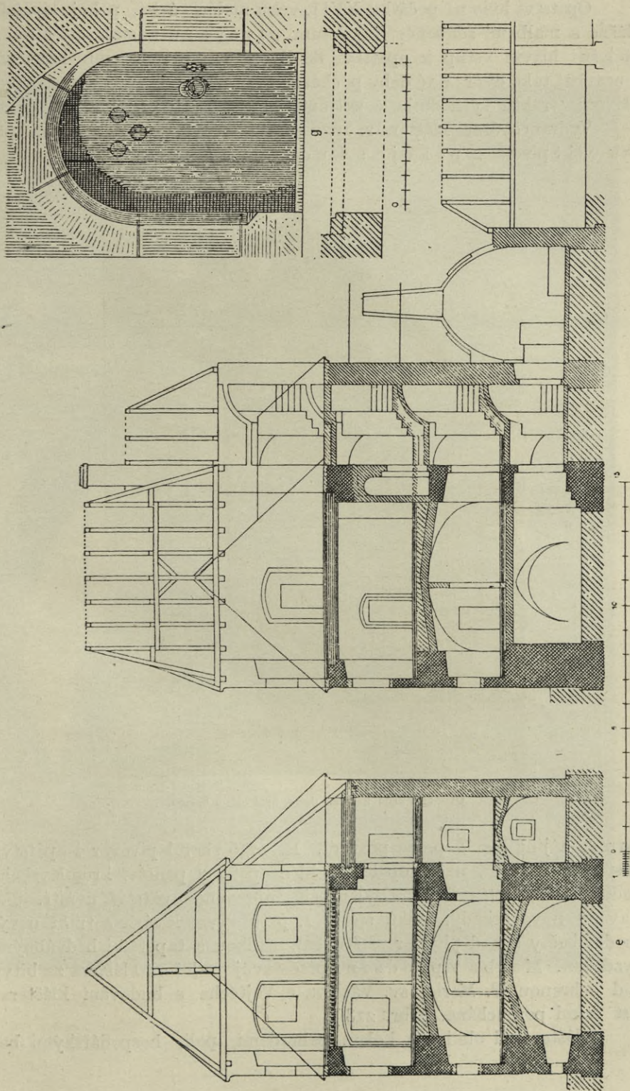
Obr. 219. Zlatá Koruna. Bašta, nyní fara: e) f) průřezy, g) ostění u sklepu.
