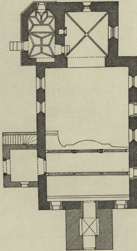
Obr. 280. Polná. Půdorys kostela.
