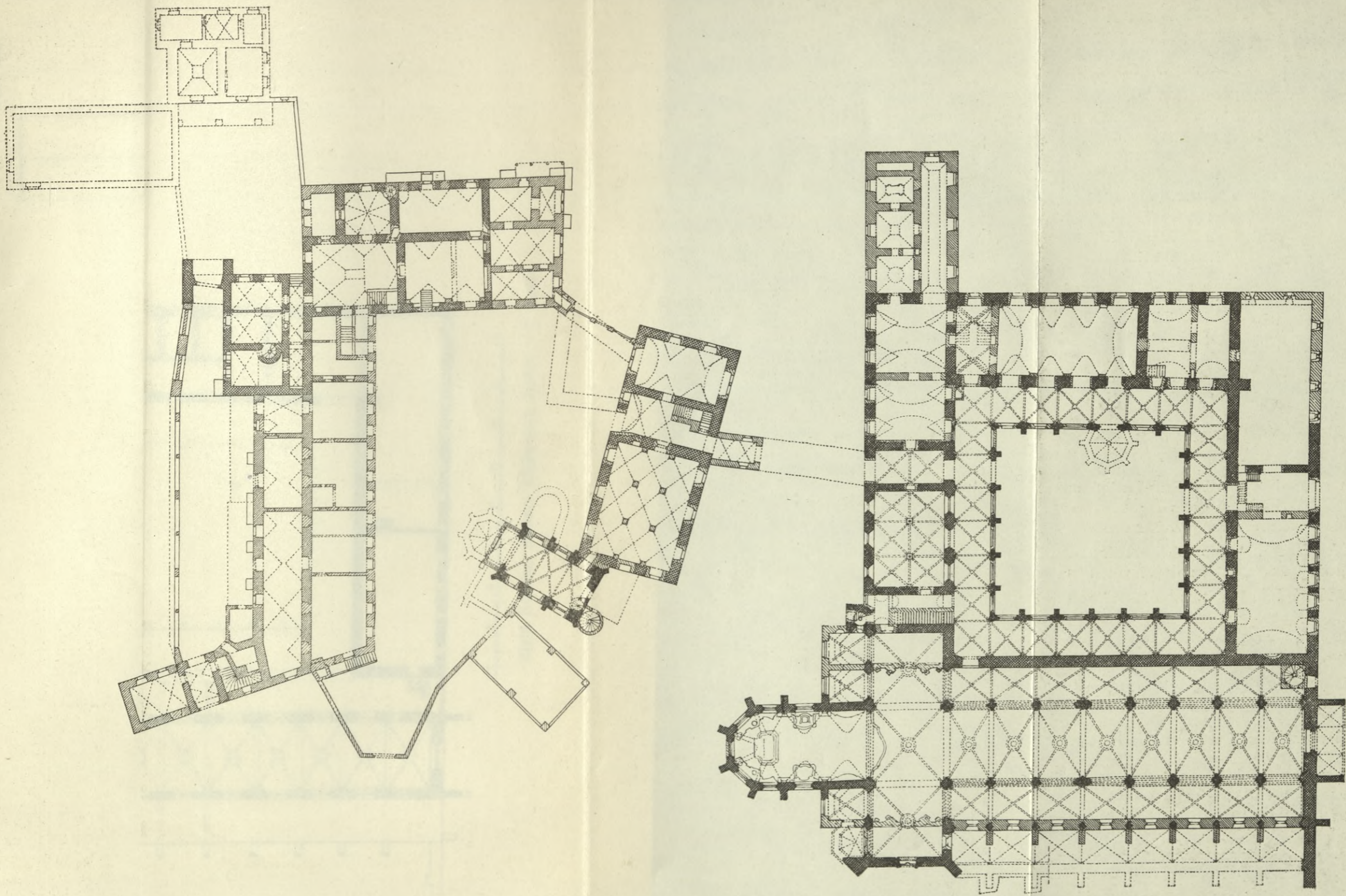
Zlatá Koruna. Situace klášterních budov v přízemí.
