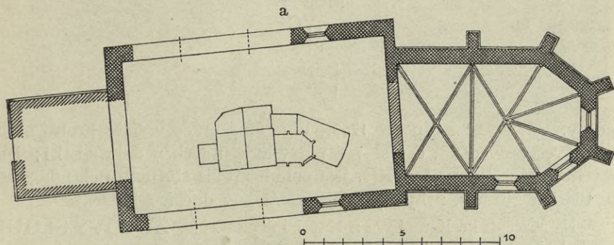
Obr. 348a. Velešín. Kostel sv. Filipa a Jakuba. Půdorys.
