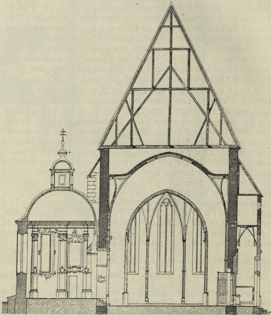
Obr. 70. Chvalšín, Průřez kostela.
