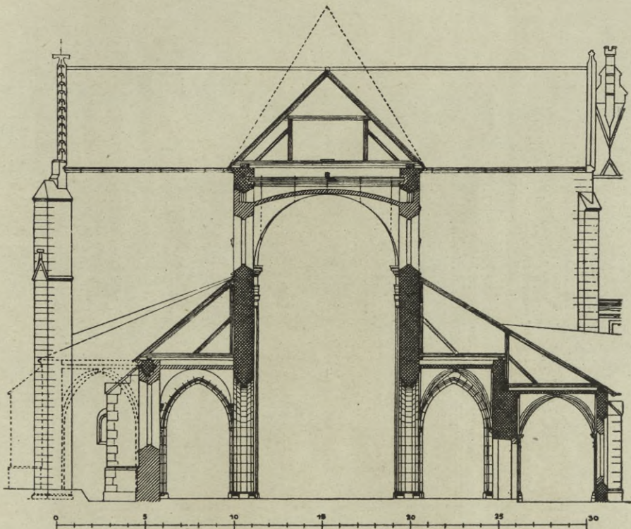
Obr. 147. Zlatá Koruna. Průřez chrámový.
