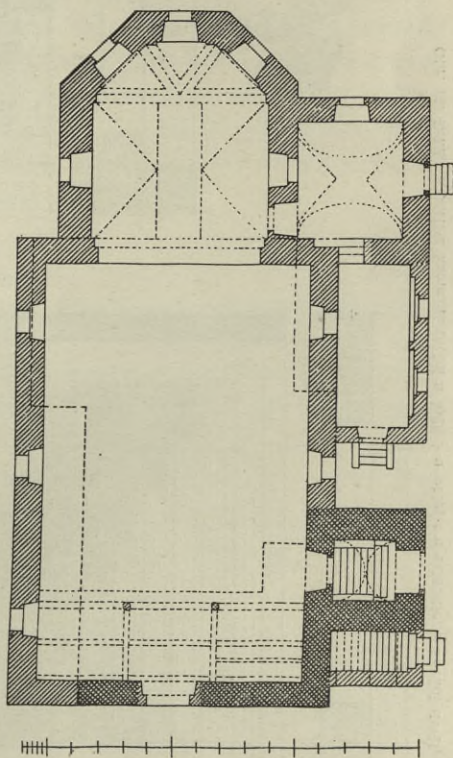
Obr. 17. Brloh. Půdorys dnešního kostela.
