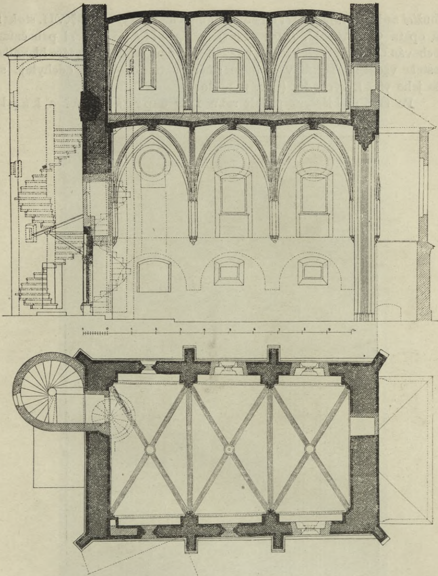
Obr. 204. Zlatá Koruna. Půdorys horního patra a průřez kaple Andělů Strážných.
