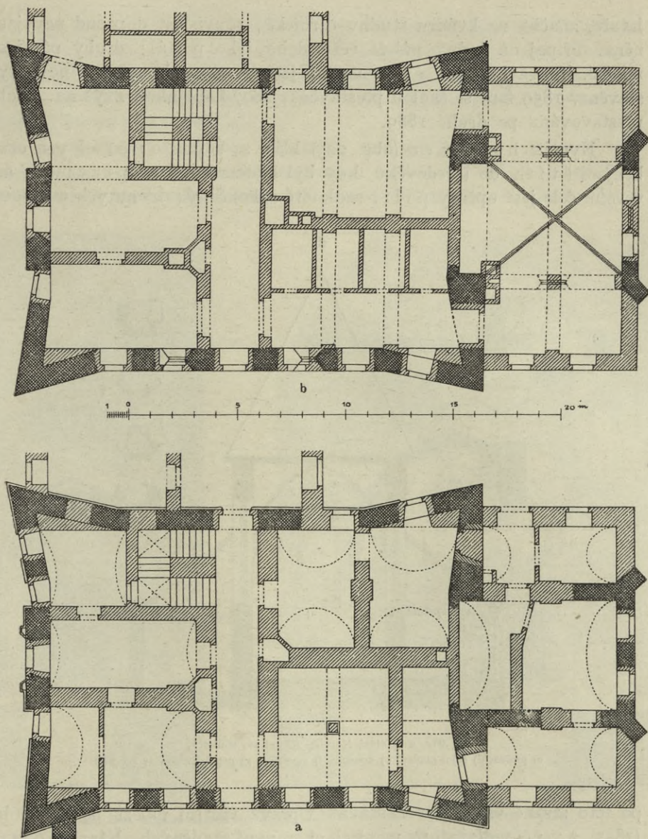
Obr. 225. Zlatá Koruna. Kostel sv. Markety: a), b) půdorys přizemí a I. patra.
