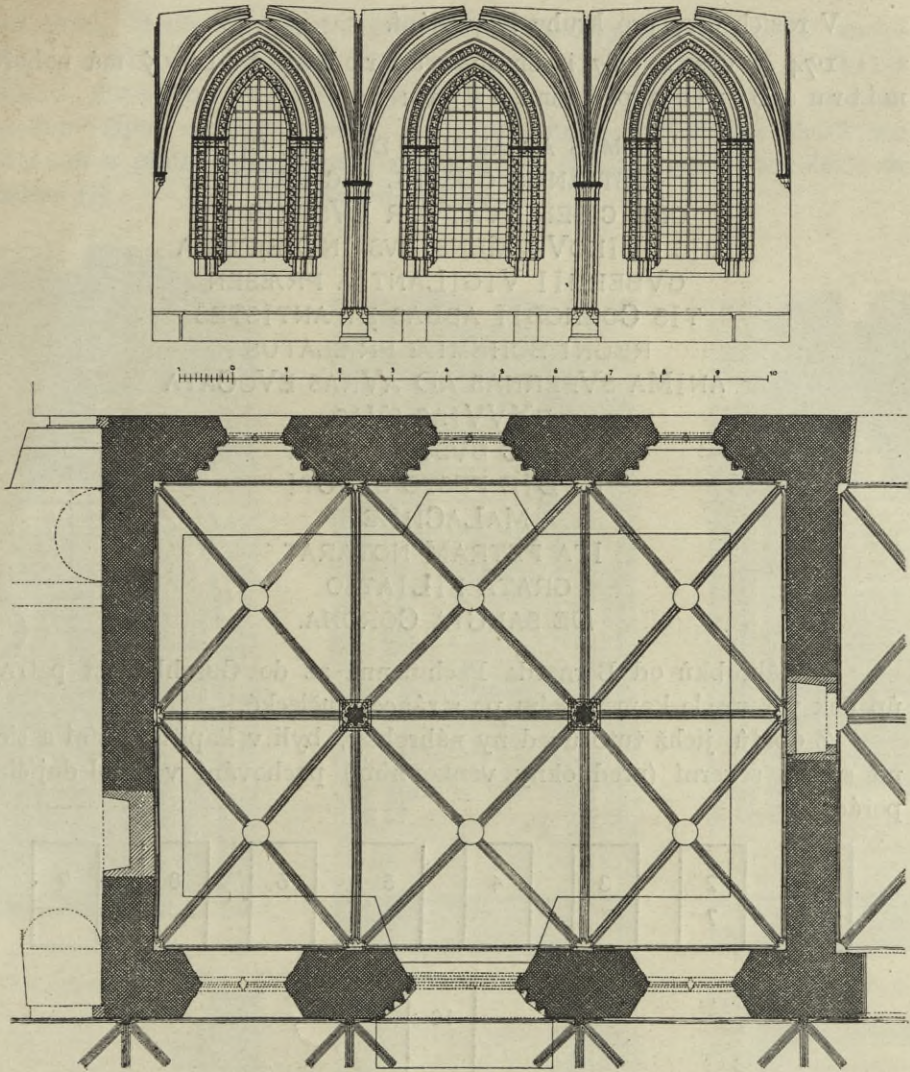
Obr. 188. Zlatá Koruna. Pádorys a profil kapitulní síně.
