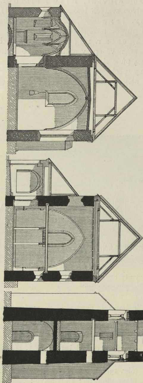
Obr. 10. Boletice. Průřez kostela, věže, presbytáře a sakristie.
