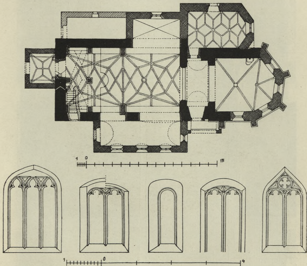
Obr. 29. Černice. Půdorys a okna kostel..
