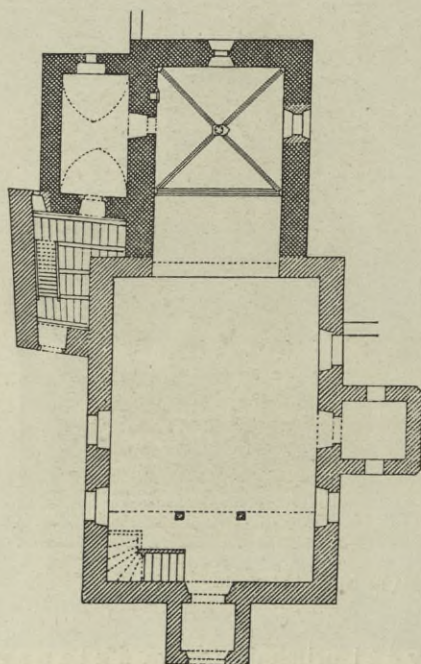
Obr. 303. Slavkov. Půdorys kostela.
