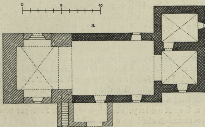
Obr. 316a. Sveraz. Půdorys kostela z r. 1687.
