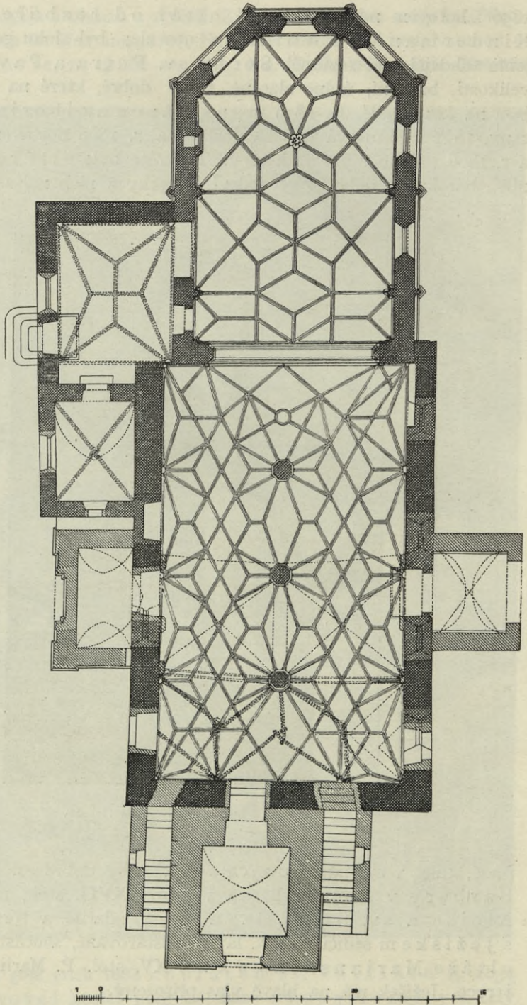
Obr. 56. Hořice. Kostel: půdorys.
