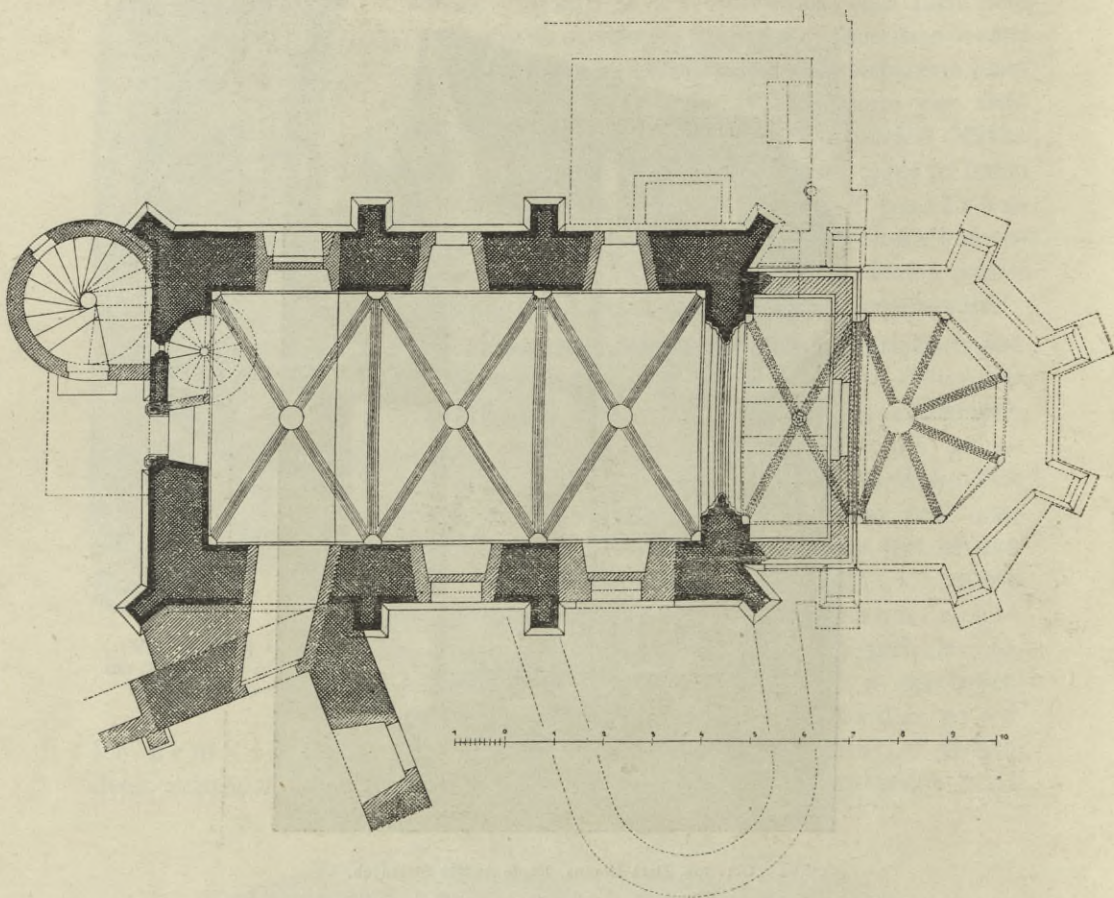
Obr. 203. Zlatá Koruna. Půdorys kaple Andělů Strážných.
