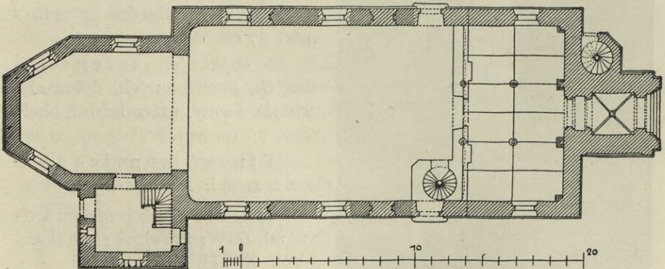
Obr. 22. Černá. Půdorys kostela.
