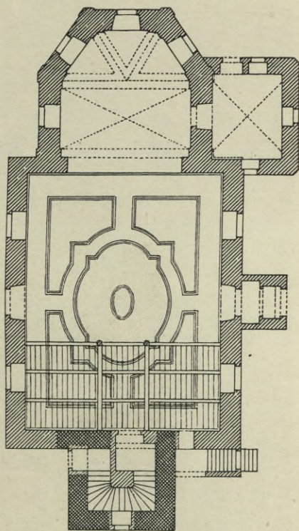
Obr. 377. Želnavá. Půdorys kostela.
