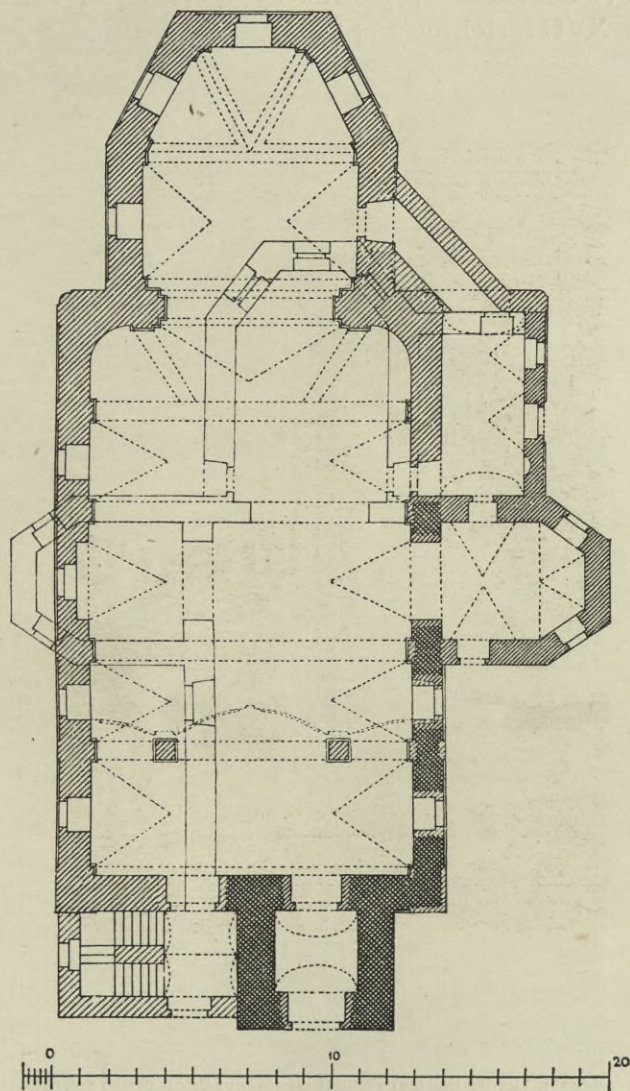
Obr. 360b. Vltavice Dolní. Dnešní půdorys kostela.
