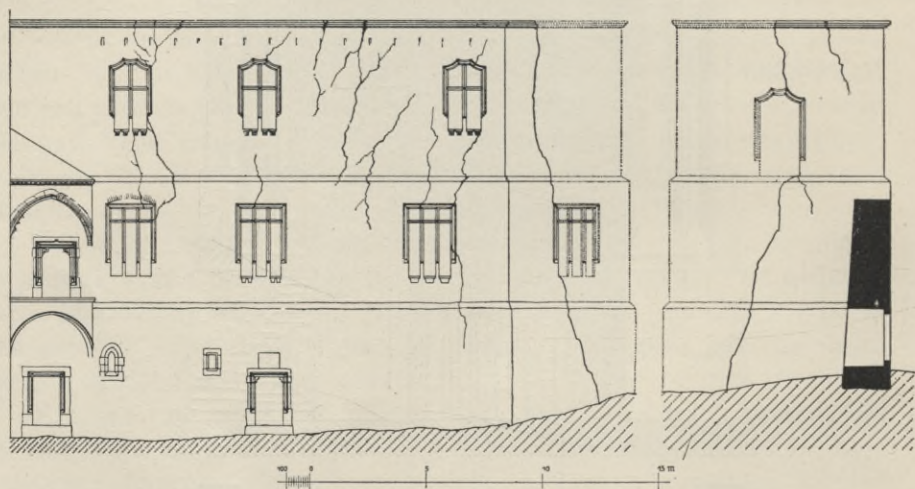
Obr. 42. Vladislavská stavba v zadním dvoře hradním. Průčelí jižní a východní před sřícením r. 1876.
