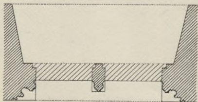
Obr. 32. Tvar okna z XV. st. paláce v II. patře.
