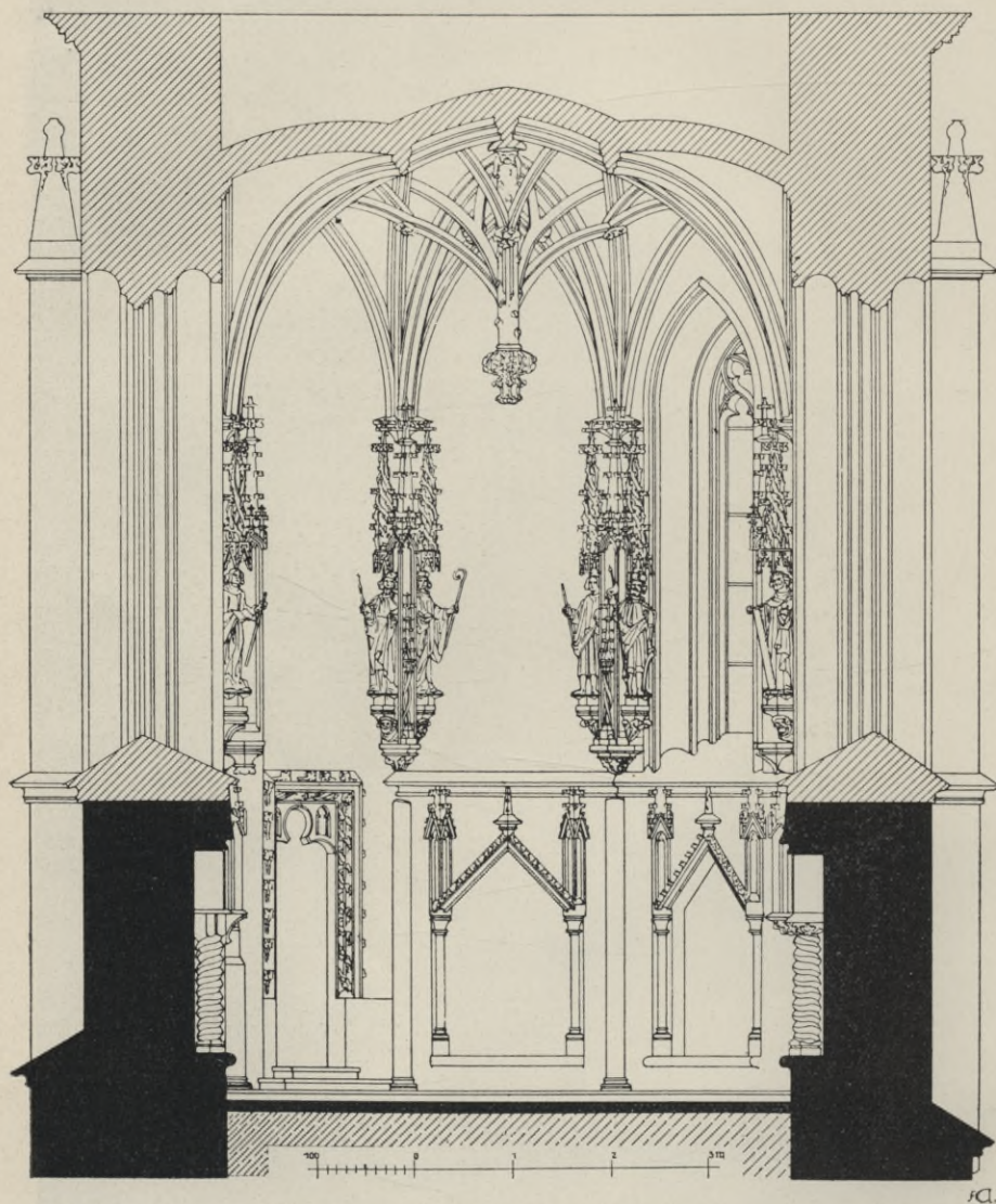
Obr. 71. Hradní kaple: Příčný řez. Pohled do presbytáře.
