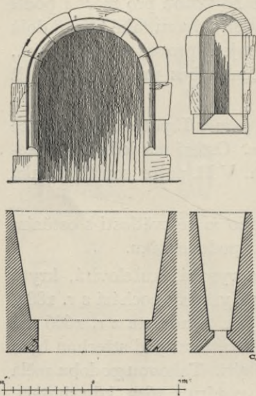
Obr. 43. Ostění vchodu a okénka z XIII. stol. v přízemí zadního dvora pod kaplí.
