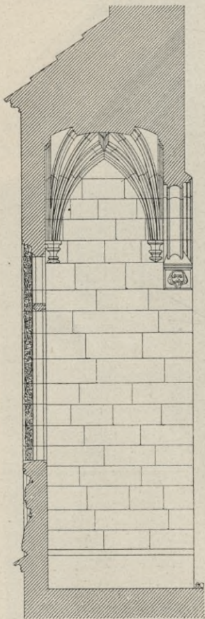
Obr. 53. Rytířský sál: Příčný řez arkýřem.
