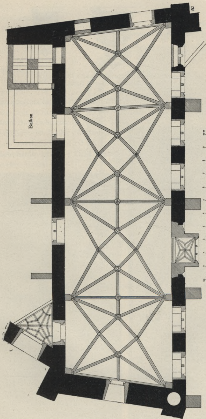
Obr. 47. Půdorys rytířského sálu, přiléhajícího schodiště a přechodu do Václavského křídla.
