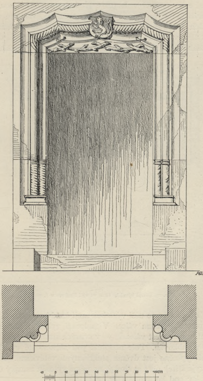
Obr. 22. Ostění dveří v I. patře věže Huderky.
