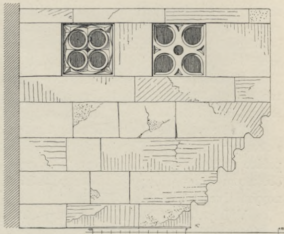
Obr. 35. Postranní pohled na balkon v zadním dvoře hradním.
