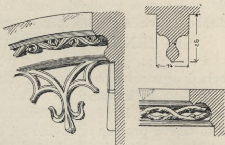
Obr. 39. Detaily přechodu z paláce do Vladislavské stavby: Nástěnná arkatura, průsek žebra klenbičky nad přechodem a hlavní římsa přechodu.
