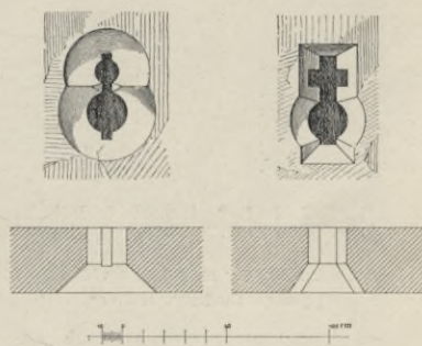
Obr. 15. Střílny (nyní v „hodinové“ věži).
