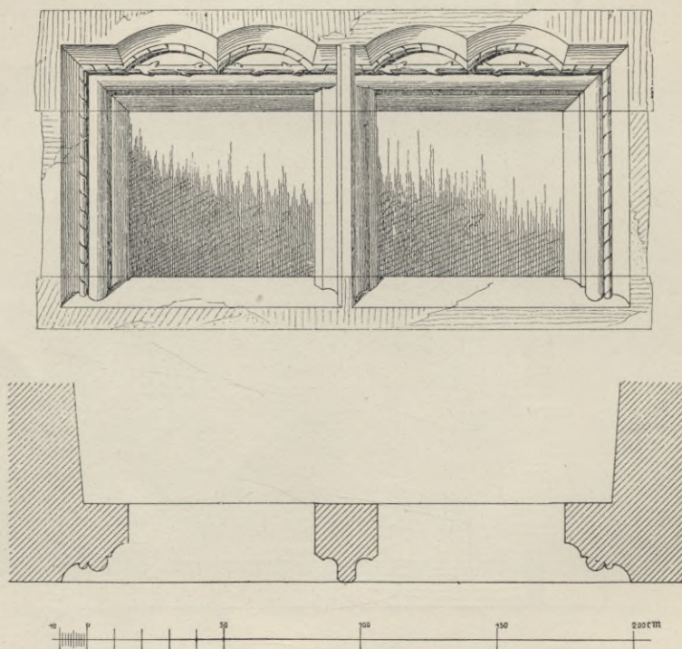
Obr. 23. Ostění bývalého okna ve věži Huderce v I. patře.
