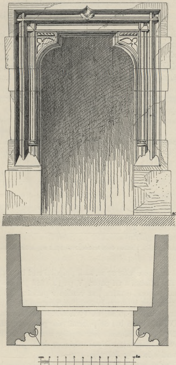
Obr. 41. Ostění vchodu do Vladislavské stavby z přechodu z paláce v I. patře.
