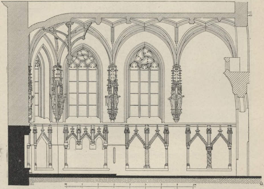
Obr. 67. Hradní kaple. Podélný řez.
