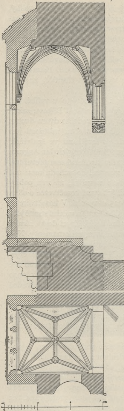
Obr. 62. Arkýř v předsíni kaple. Půdorys a řez.
