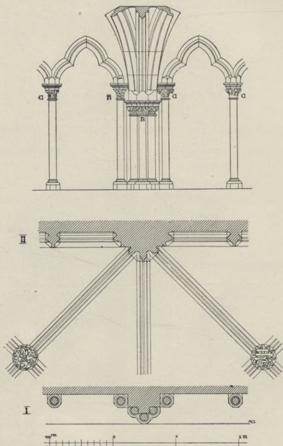
Obr. 28. Detail stěny a klenby průjezdu v paláci.
