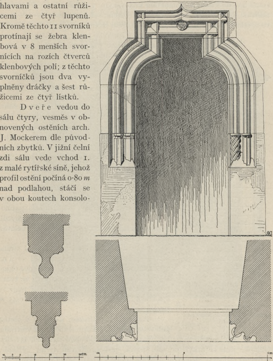
Obr. 51. Průsek žebra klenbového v rytířském sále (dole) a v kapli (nahore).
