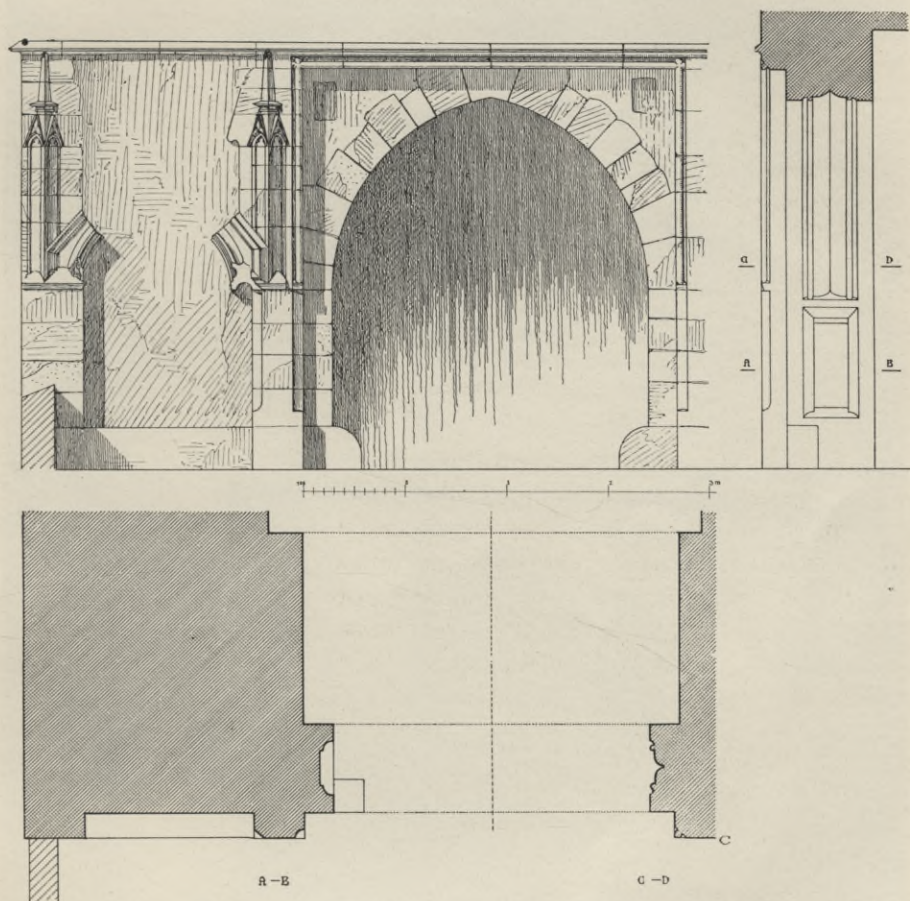
Obr. 12. Půdorys, pohled a řez první (původně druhé) hradní brány.
