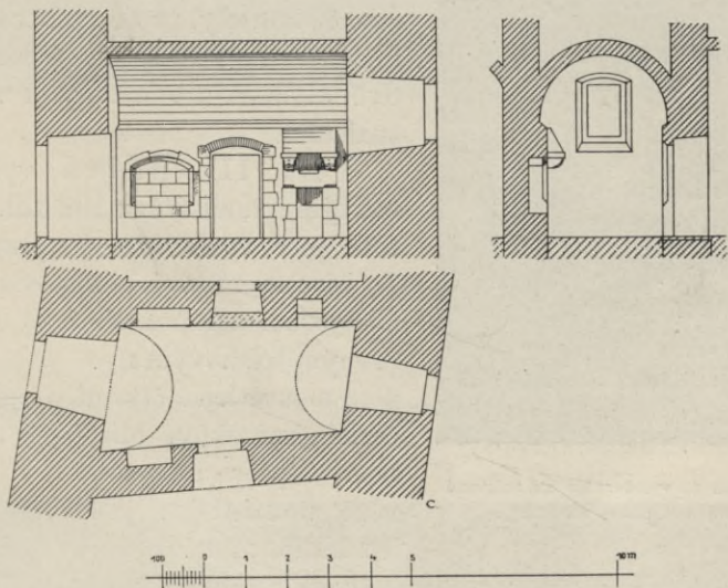
Obr. 56. Přízemí Vladislavského křídla v zadním dvoře: Půdorys a řez příčný i podélný bývalé t. zv. krčmy hradní.
