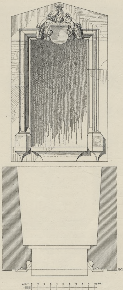
Obr. 29. Ostění okna do „stříbrnice“ v přízemí paláce.
