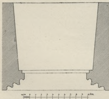
Obr. 36. Průsek ostění dveří do stříbrnice v přízemí paláce v zadním dvoře.
