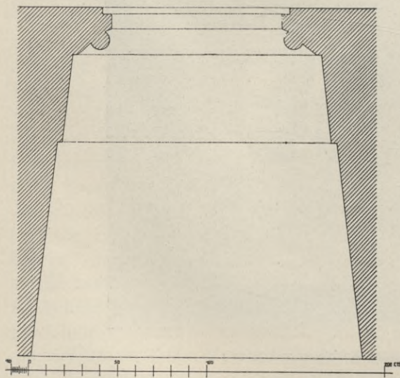
Obr. 85. Věž prochoditá. Ostění dveří v I. patře, na záp. straně.
