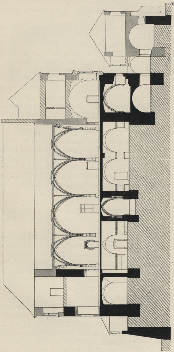
Obr. 46. Podélný řez palácem.
