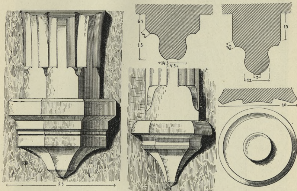
Obr. 210. Písek. Hrad. Žebra, svorník a konsoly v arkádách.
