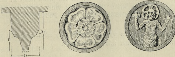
Obr. 70. Dobeš. Kostel sv. Brikcí. Profil žebra a svorníky.
