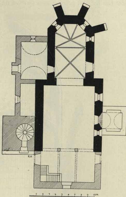
Obr. 343. Strunkovice. Půdorys kostela.
