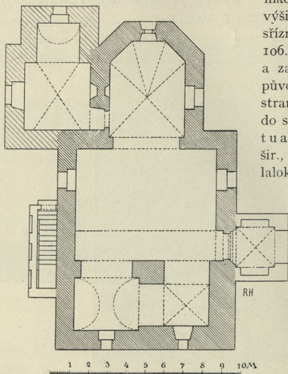
Obr. 105. Krč. Půdorys kostela.
