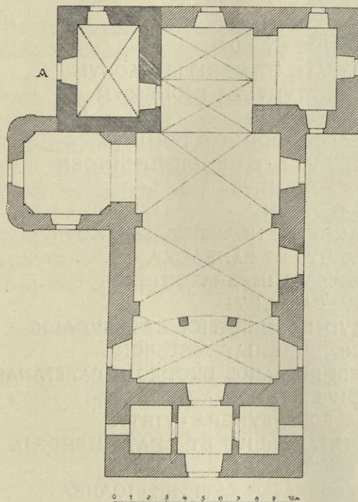
Obr. 43. Čimelice. Kostel sv. Trojice. Půdorys.
