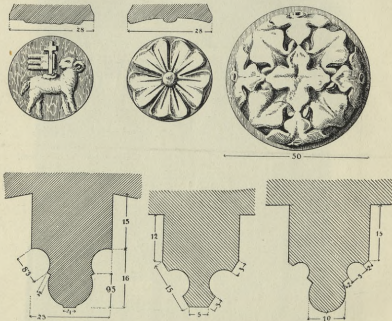
Obr. 239. Písek. Děk. kostel. Svorníky v sakristii (v levo) a presbytáři (v pravo); profil žebra v hlav. lodi a v presbytáři.
