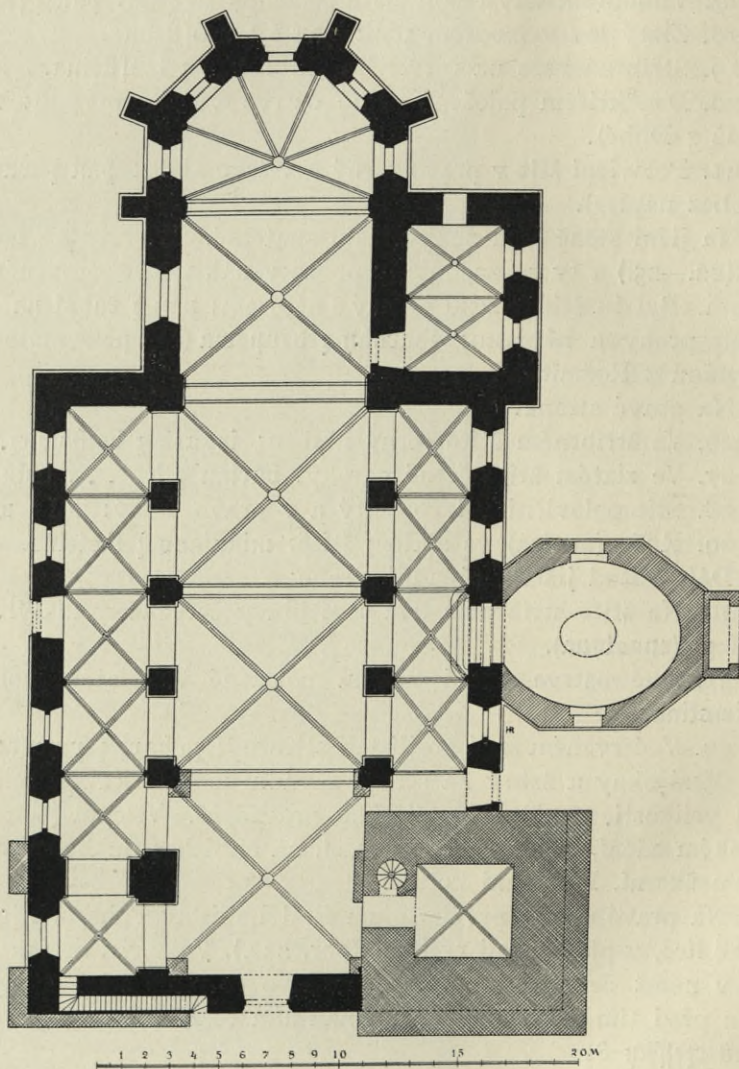
Obr. 221. Písek. Děk. kostel. Půdorys.
