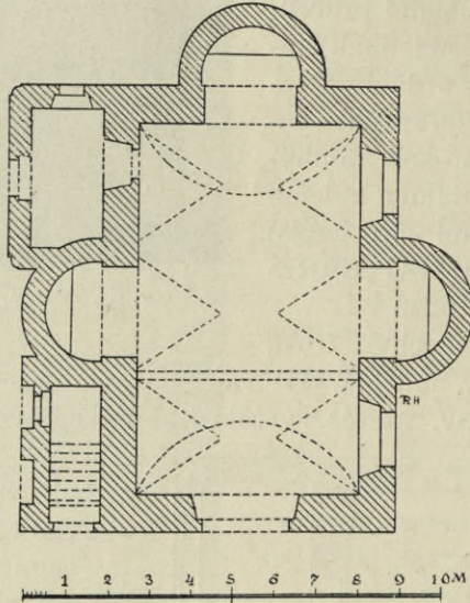
Obr. 320. Protivín. Hřbitovní kaple sv. Anny. Pádorys.
