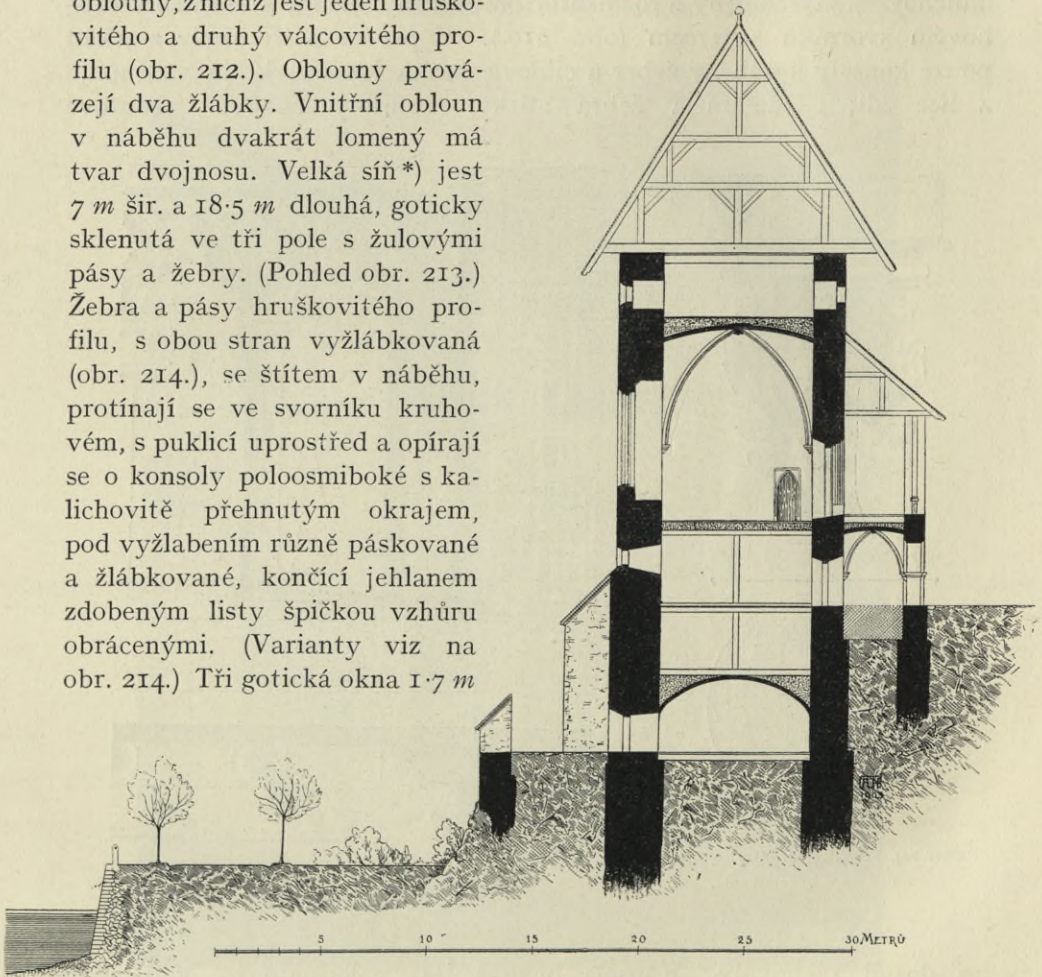
Obr. 206. Písek. Hrad. Řez zachovaným křídlem západním.
