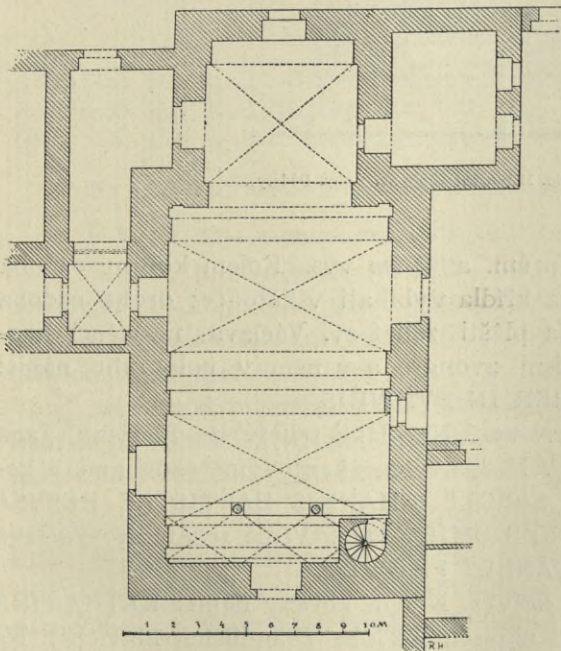
Obr. 319. Protivín. Kostel sv. Alžběty. Půdorys.
