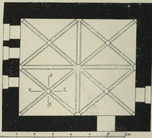
Obr. 28r. Písek. Dům čp. 26., tak zv. modlitebna Čes. Bratří. Síň v přízemí. 1. Pohled, půdorys a žebro.
