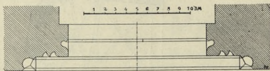
Obr. 135. Myšelec. Kostel. Profil ostění portálu v lodi.
