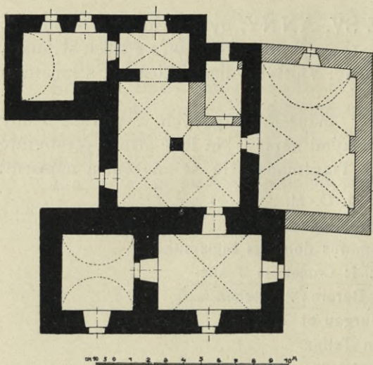
Obr. 321. Putim. Púdorys fary (bývalé tvrze).
