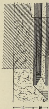
Obr. 26. Bavorov. Kostel P. Marie. Profil portálu do Božího hrobu.
