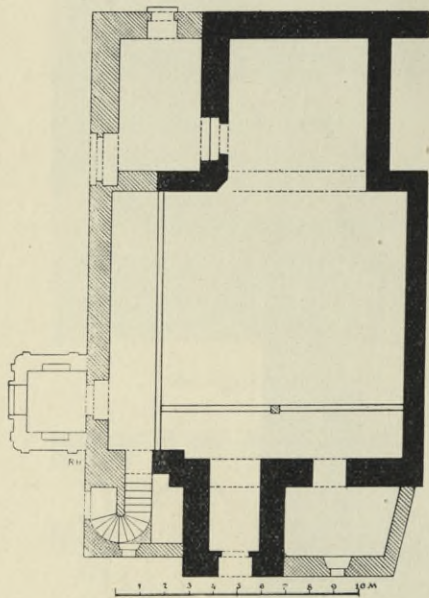
Obr. 116. Mirovice. Půdorys kostela.
