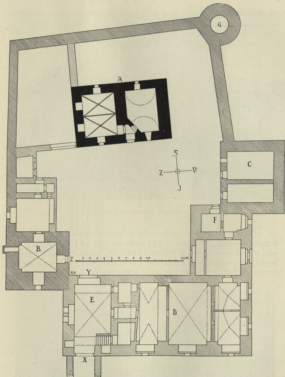
Obr. 90. Kestřany. Horní tvrz. Půdorys.
