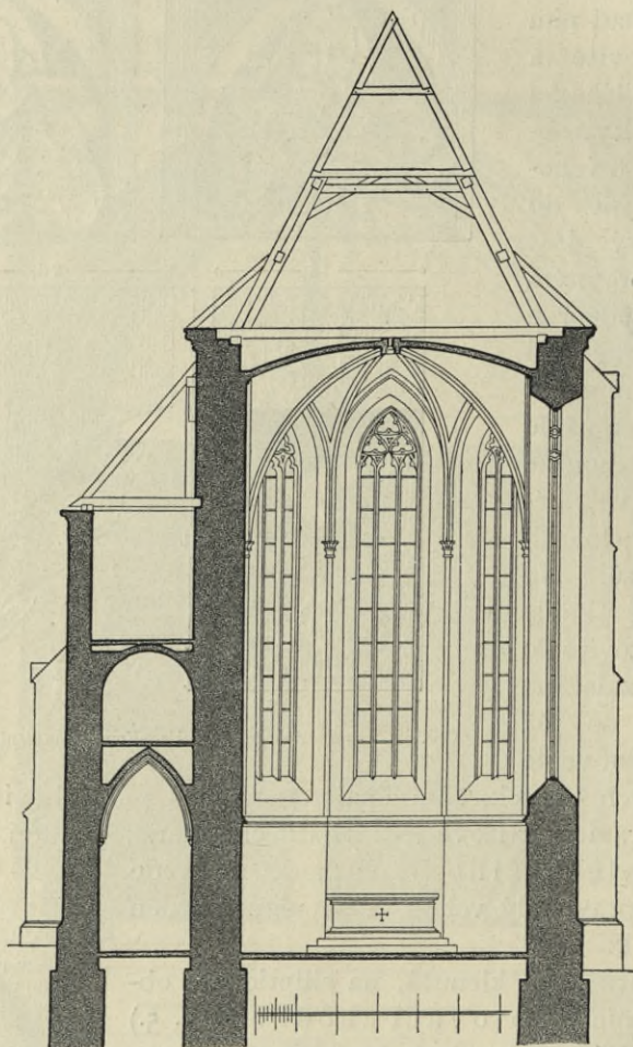
Obr. 15. Bavorov. Kostel P. Marie. Řez presbytářem a sakristií.
