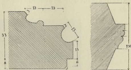
Obr. 224. Písek. Děk. kostel. Profil okna ve velké věži a presbytáři.
