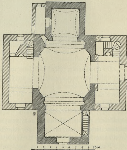
Obr. 98. Kestřany. Kostel sv. Kateřiny. Půdorys.
