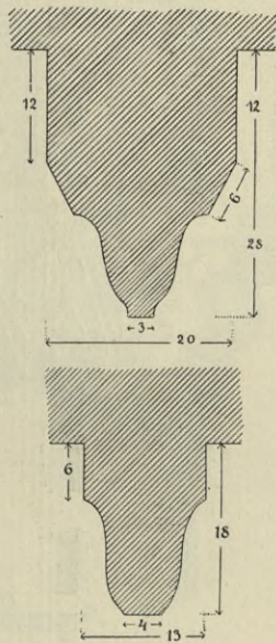
Obr. 18. Bavorov. Kostel P. Marie. Profil žebra v sakristii (nahore) a v presbytáři a transeptu (dole).
