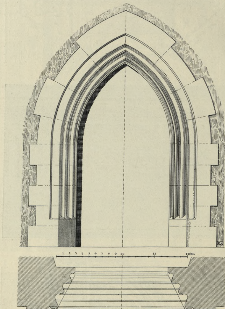
Obr. 25. Bavorov. Kostel P. Marie. Portál kaple Anděla Strážce.
