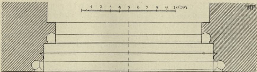
Obr. 81. Heřmaň. Kostel sv. Jiljí. Profil záp. portálu.
