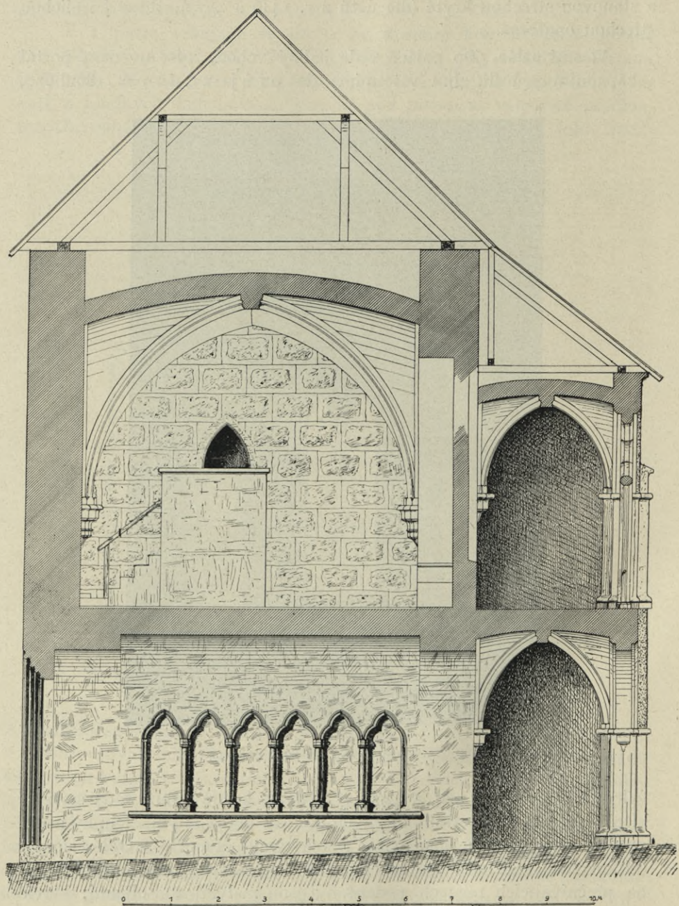
Obr. 428. Zvíkov, Vlastní palác, Řez průřezem, t. zv. svatební síní a oběma úrovněmi nádvořních arkád. ] (omylem při reprodukci obráceno).
