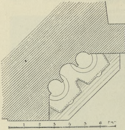
Obr. 233. Písek. Děč. kostel. Profil ostění sev. portálu.
