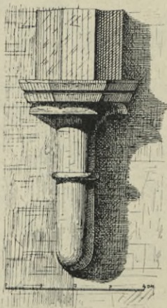
Obr. 426. Zvíkov, Hlízová věž, Konsola a žebro klenby v korunní síni.
