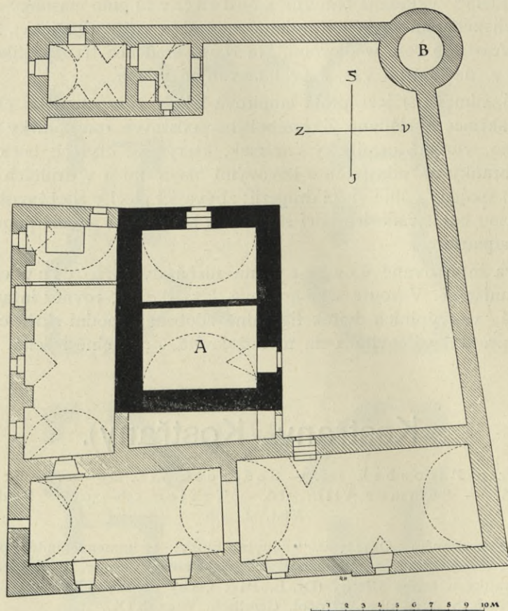
Obr. 87. Kestřany. Dolní tvrz. Půdorys.
