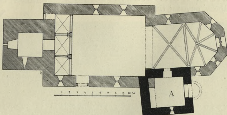
Obr. 133. Myšelec. Půdorys kostela.
