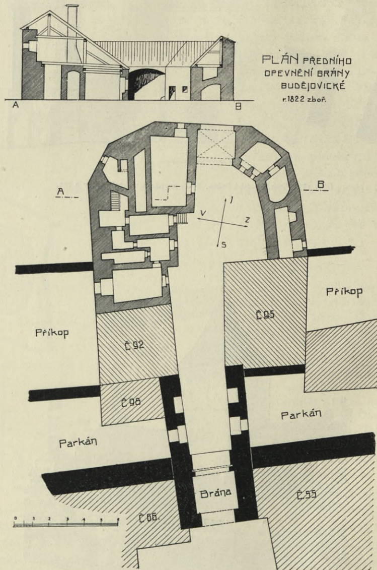
Obr. 189. Písek. Plán předního opevnění brány Budějovické, r. 1822 zbořeně.
