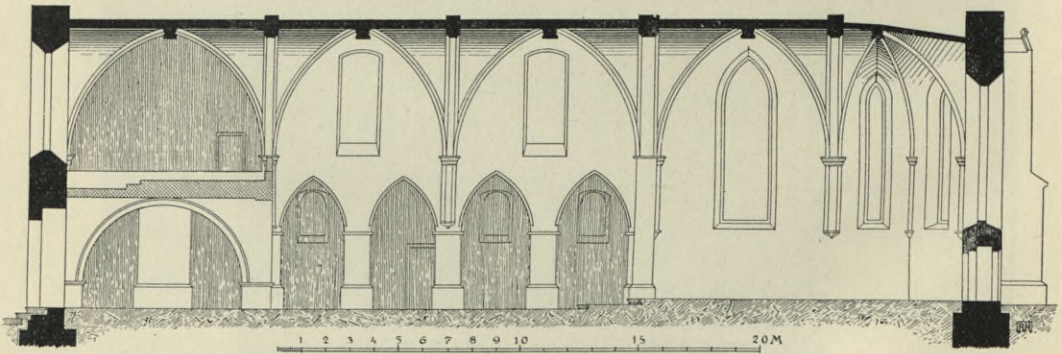
Obr. 234. Písek. Děč. kostel. Řez podélný hlavní lodi a presbytářem.
