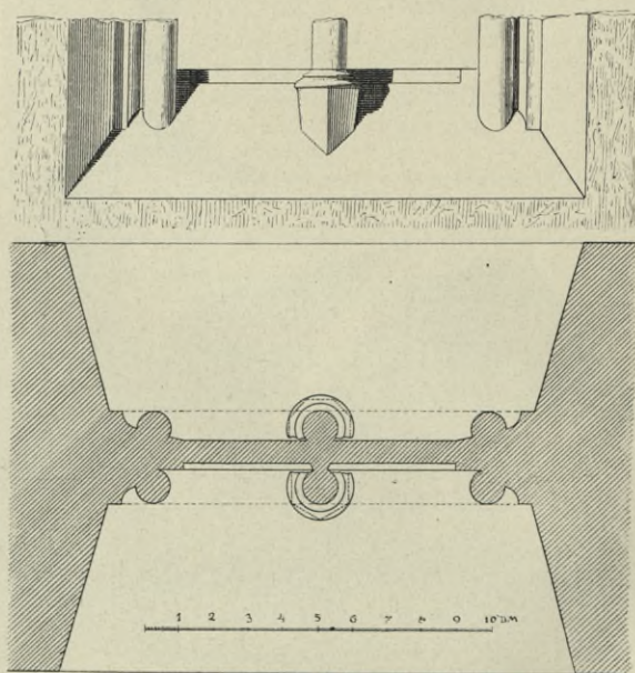
Obr. 137. Myšelec. Kostel. Nárys a řez okna v presbytáři.
