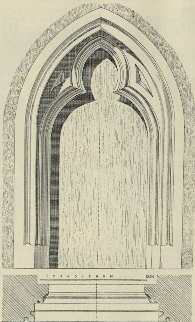
Obr. 212. Písek. Hrad. Portál z arkád do velké síně.
