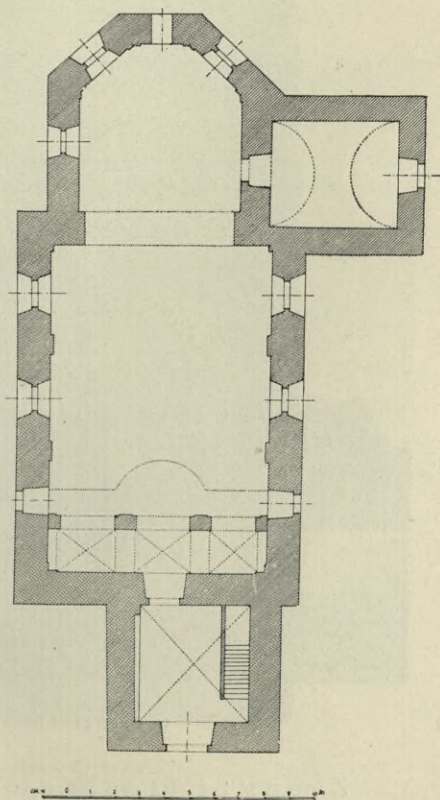
Obr. 333. Staré Sedlo. Půdorys kostela.
