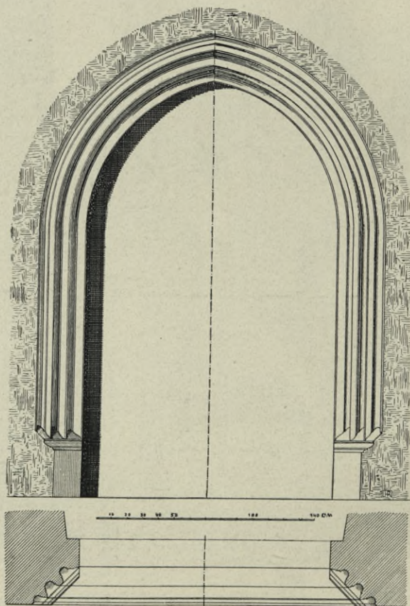
Obr. 379. Vodňany. Děk. kostel. Portál v hlavní lodi na severu.
