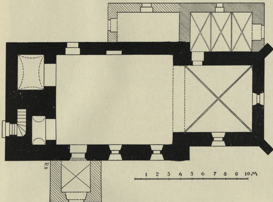
Obr. 34. Blsko. Kostel. Půdorys.
