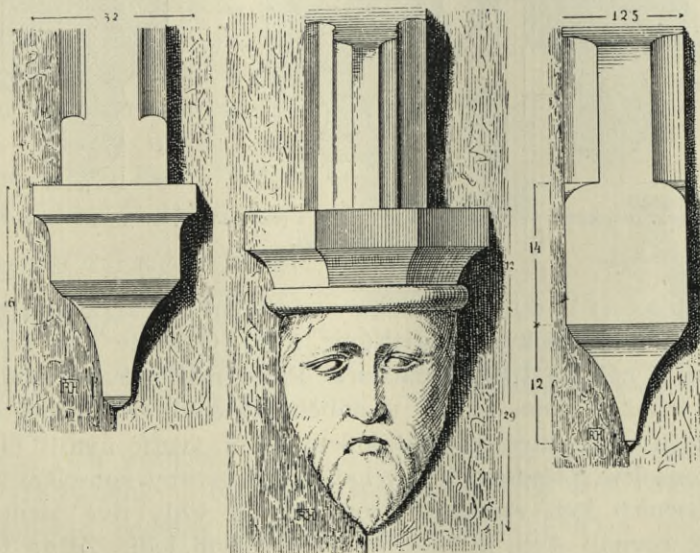
Obr. 238. Písek. Děk. kostel. Konsoly v záp. travée hlav. lodi (uprostřed) a koutové konsoly bočních lodí (po stranách).
