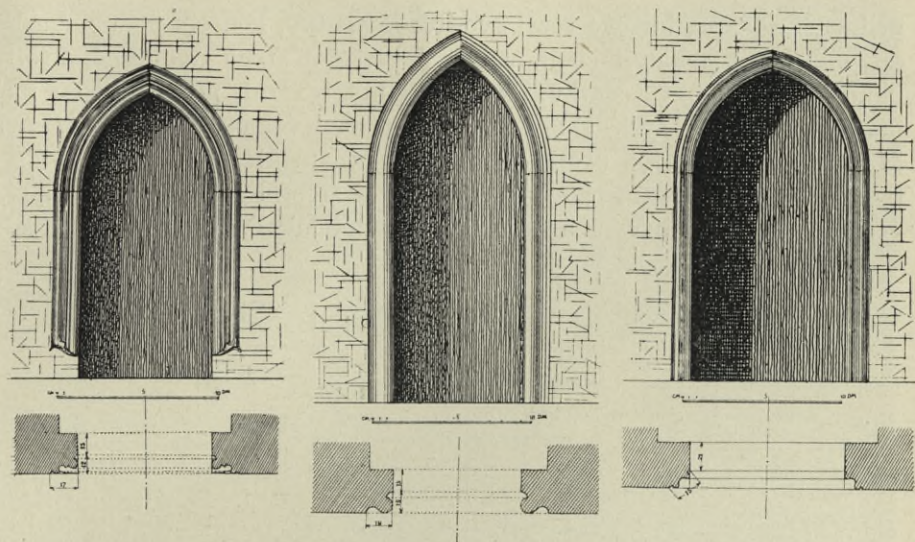
Obr. 439. Zvíkov, Vlastní palác. Portálky do sakristie v přízemních i horních arkádách (typ.).
