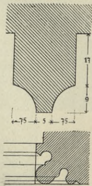
Obr. 106. Krč. Kostel. Profil žebra a ostění portálu v lodi.
