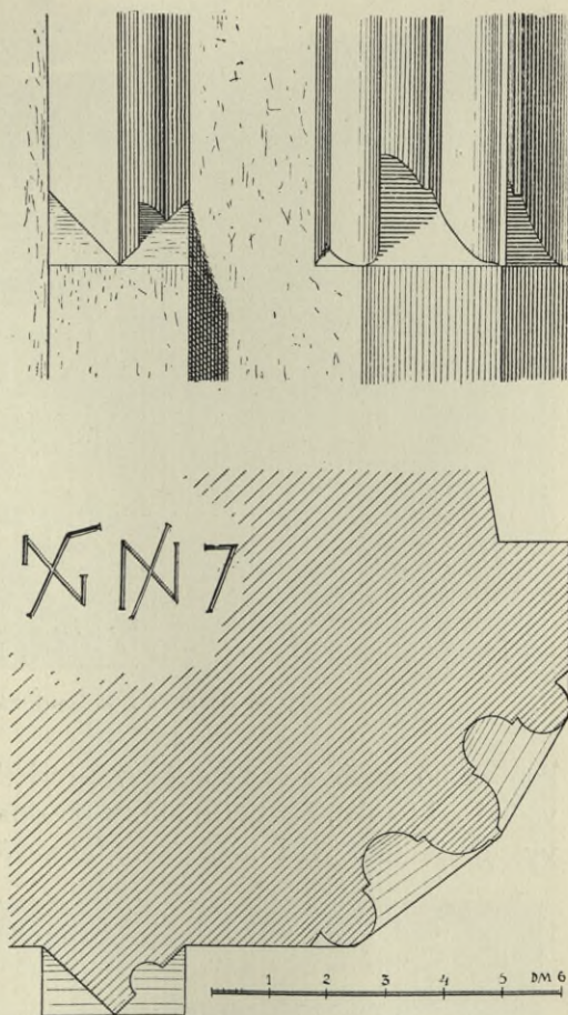
Obr. 227. Písek. Děk. kostel. Profil ostění záp. portálu a značky na něm.
