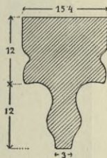
Obr. 278. Písek. Dům čp. 119. „U tří korun“. Tvárnice žebrová.
