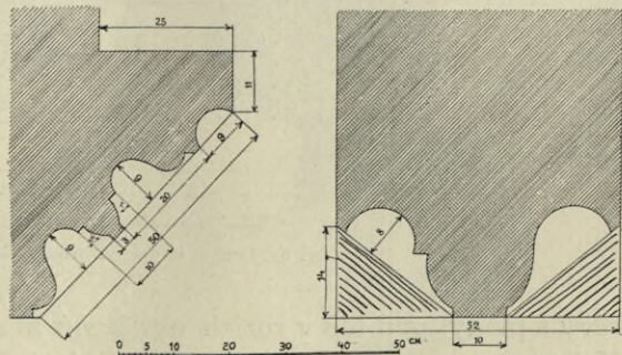
Obr. 65. Dobeň. Kostel sv. Bricej. Profil portálu a triumf. oblouku.
