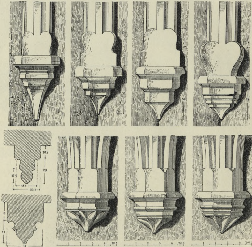
Obr. 214. Písek. Hrad. Profil žeber a varianty konsol ve velké síni.
