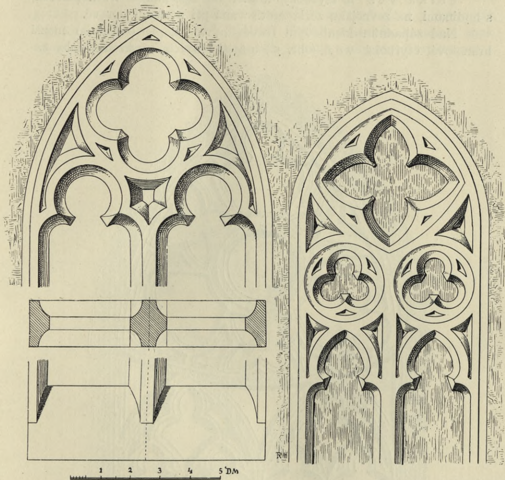
Obr. 7. Bavorov. Kostel P. Marie. Kružby okenní v sakristii (v levo) a v záp. průčelí (v pravo).
