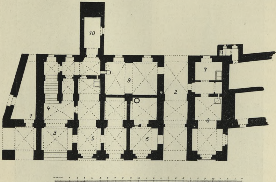
Obr. 266. Písek. Radnice. Půdorys.
