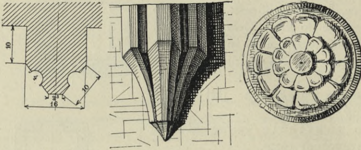
Obr. 399. Záhoří, Kostel. Profil a pata žebra, svorník,
