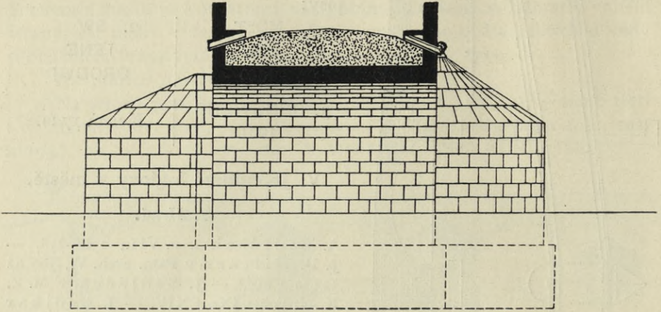
Obr. 196. Písek, Most. Řez příčný středem oblouku (nynější stav).
