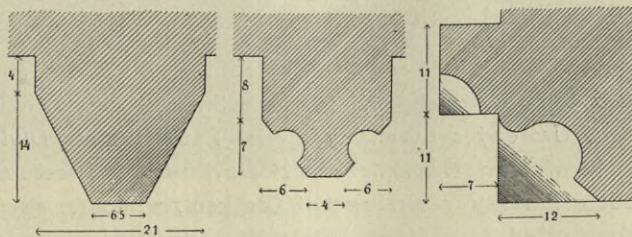
Obr. 35. Blsko. Kostel. Profil žeber v presbytáři, sakristii a ostění již. portálu.
