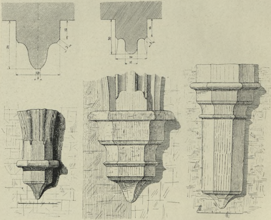
Obr. 436. Zvíkov. Vlastní palác. Konsoly a žebra v arkádách, v t. zv. svatební síni a královské síni.
