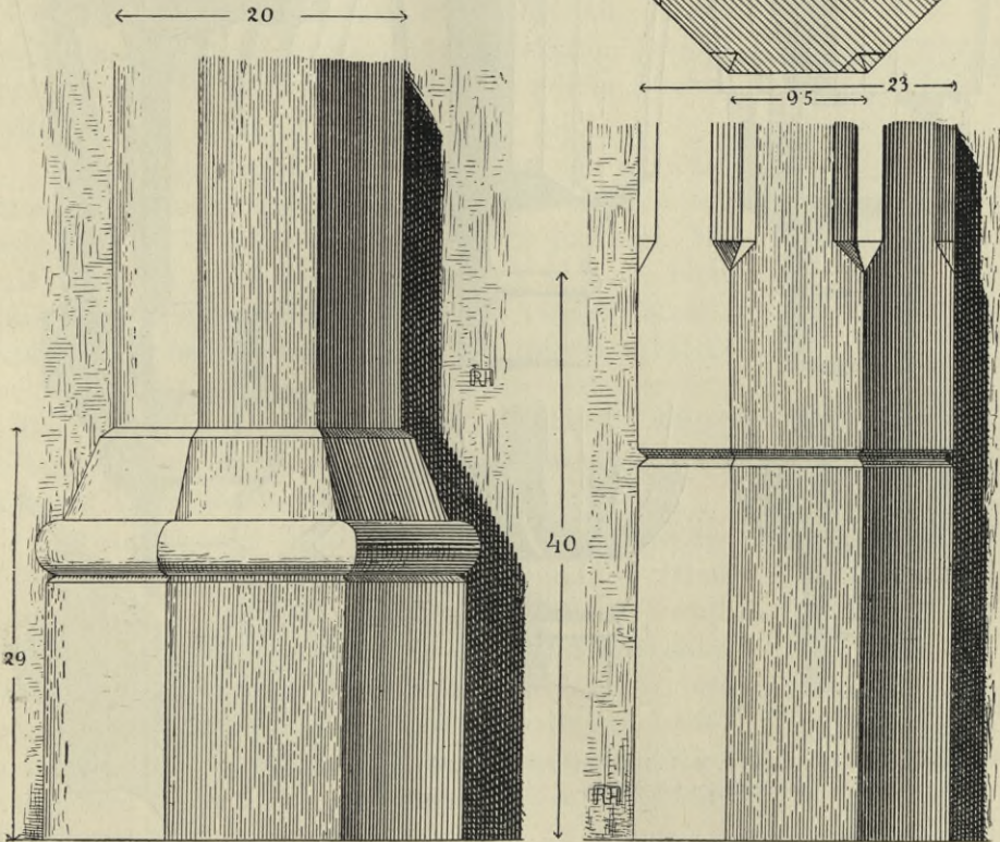
Obr. 16. Bavorov. Kostel P. Marie. Přípory původní klenby v lodi.
