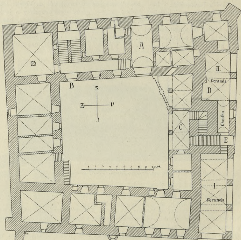
Obr. 310. Protivín. Zámek. Půdorys.
