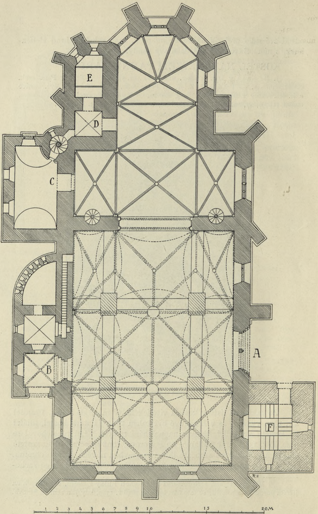
Obr. 4. Bavorov. Kostel P. Marie. Půdorys.
