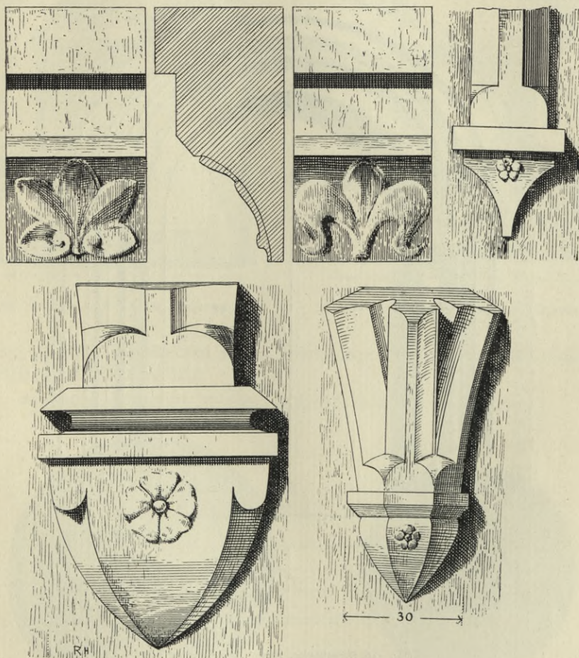
Obr. 345. Strunkovice. Kostel. Podřímší lodí a konsoly v presbytáři.
