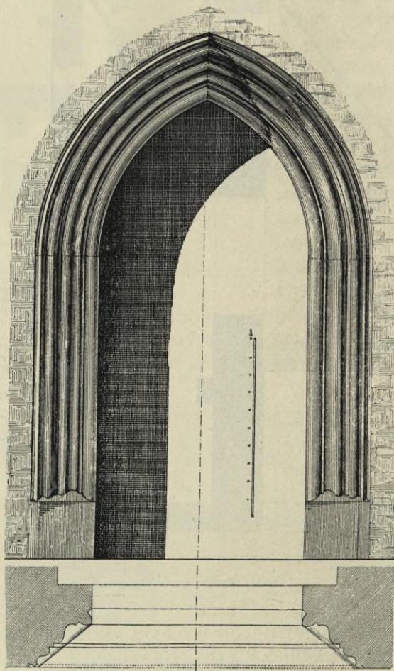
Obr. 325. Putim. Kostel. Portál v jižní lodi.
