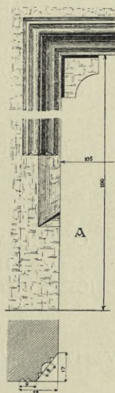
Obr. 44. Čimelice. Kostel sv. Trojice. Portál sakristie.
