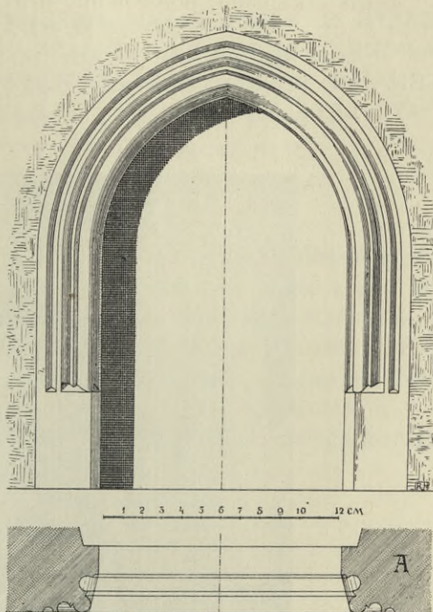
Obr. 303. Poholí. Kostel. Portál do věže.
