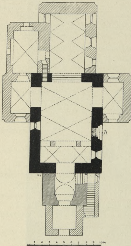
Obr. 84. Chelčice. Kostel sv. Martina. Půdorys.
