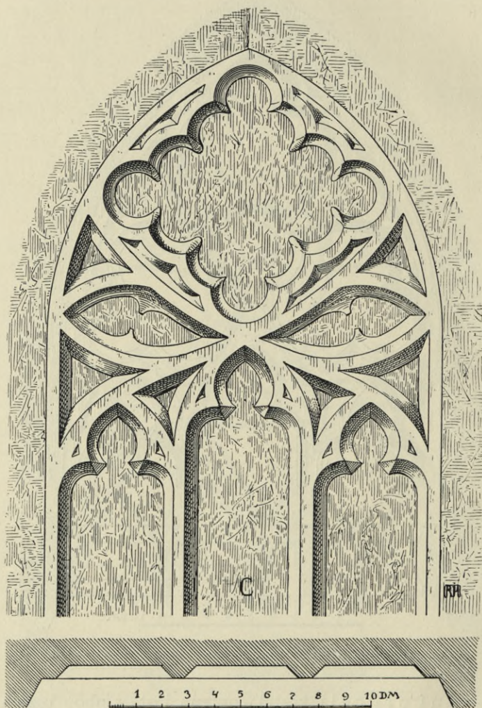
Obr. 10. Bavorov. Kostel P. Marie. Kružba v okně posledního travée lodi na již. straně (zazděná).
