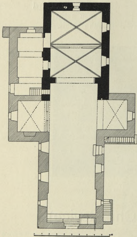
Obr. 112. Křešovice. Kostel. Půdorys.
