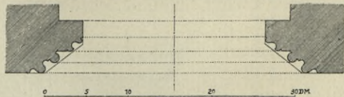
Obr. 422. Zvíkov, Vlastní palác. Portál v záp. průčelí a řez jeho ostěním.
