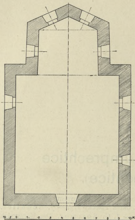
Obr. 1. Sv. Anna. Püdorys kaple sv. Anny.
