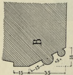
Obr. 304. Poholí. Kostel. Profil druhého vchodu věžního.
