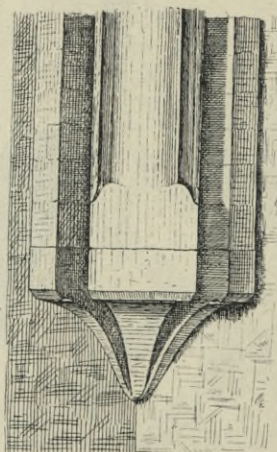
Obr. 425. Zvíkov, Hlízová věž, Konsola a žebro klenby v přízemí.
