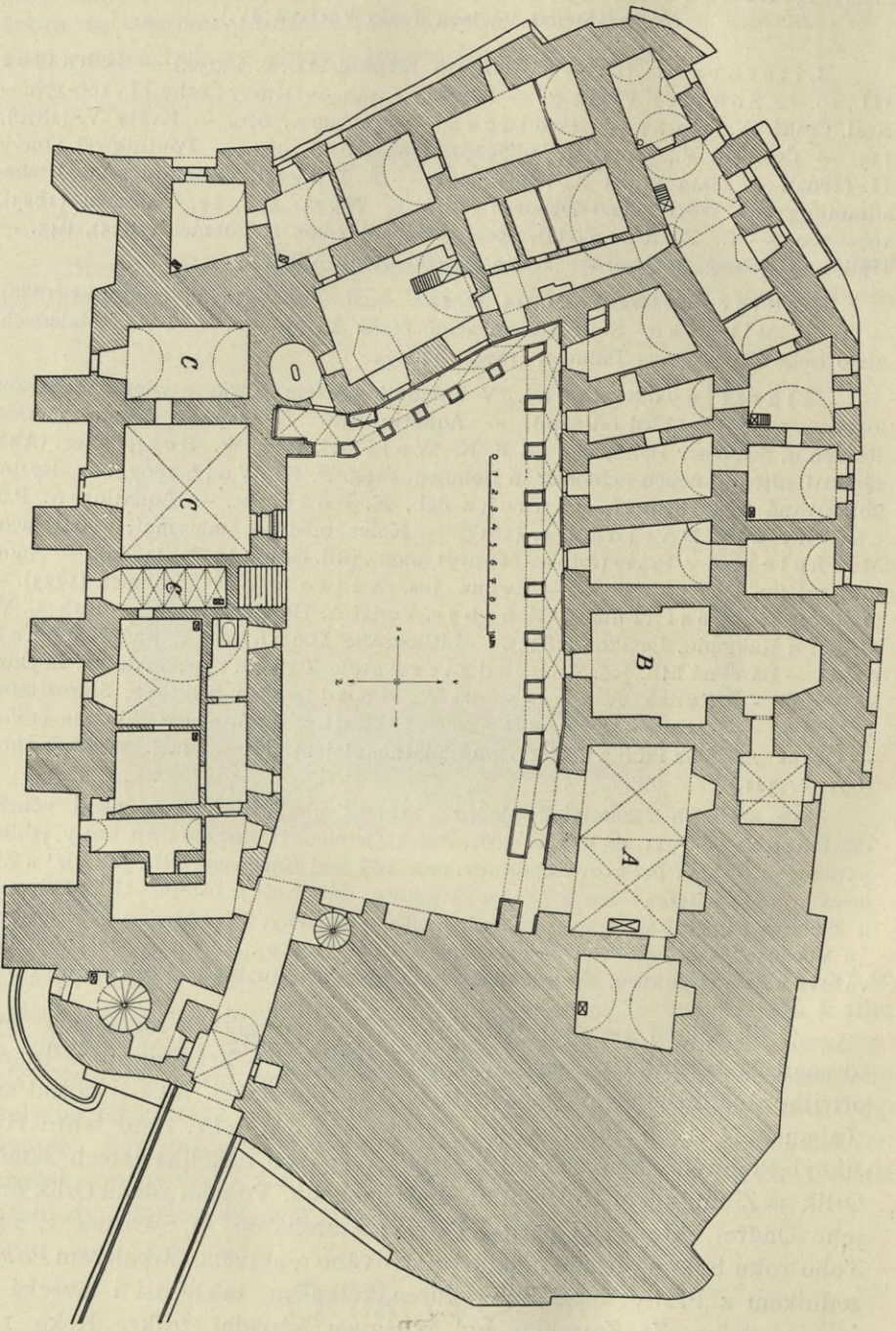
Obr. 148. Orisk. Páduys zámku.
