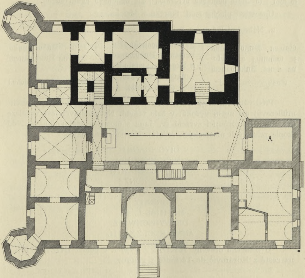
Obr 41. Bukovany. Půdorys zámku.
