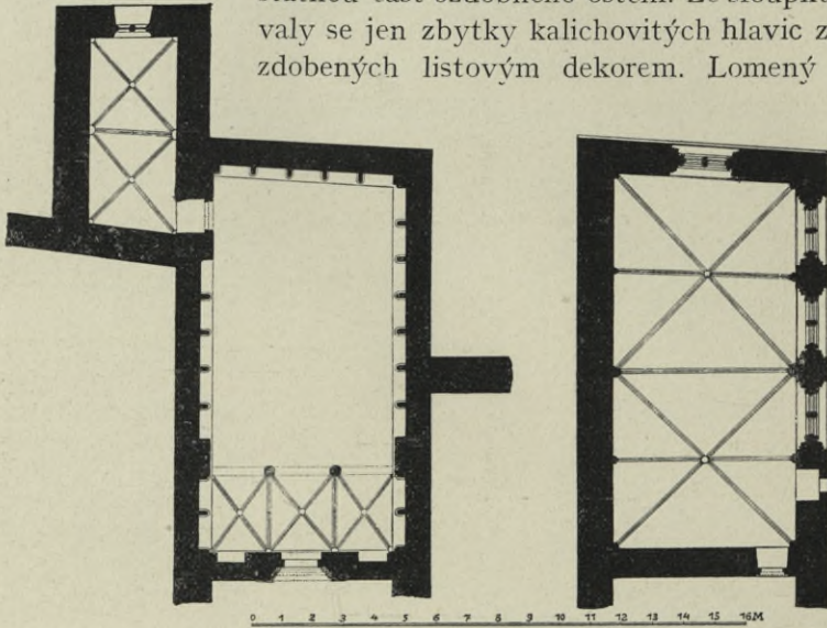
Obr. 449. Zvíkov, Hradní kaple. Půdorys v úrovni podlahy (se sakristií) a klenby.
