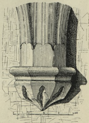
Obr. 451. Zvíkov. Hradní kaple. Nahoře konsoly v sakristii, dole konsoly a žebra v kapli, v koberce pod kaplí a v podempfoři.
