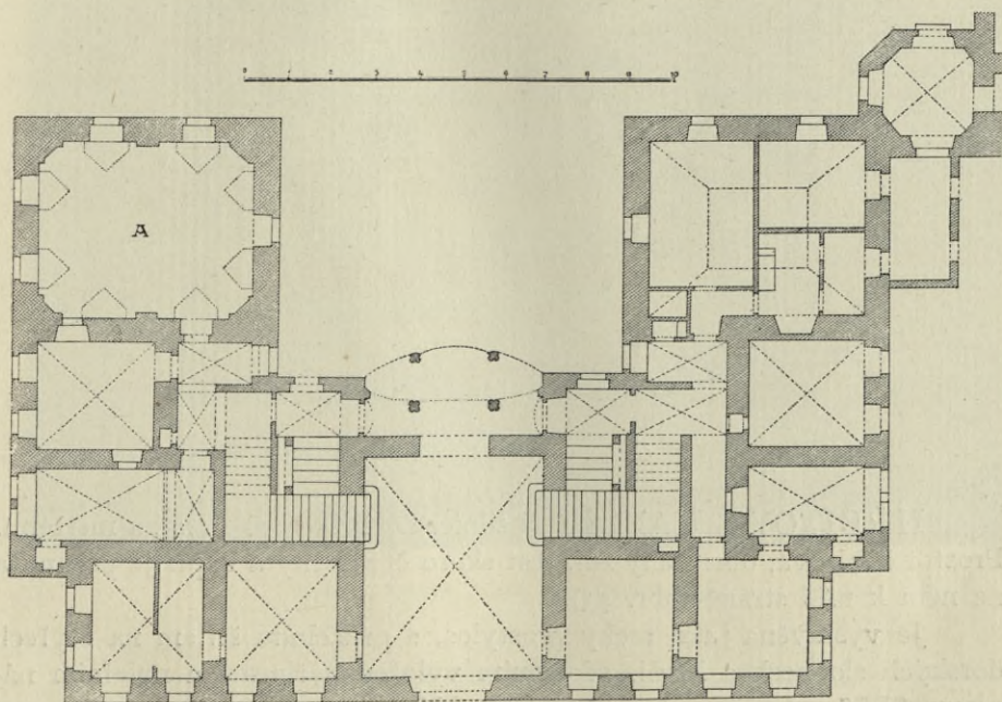
Obr. 50. Čimelice. Zámek. Půdorys.
