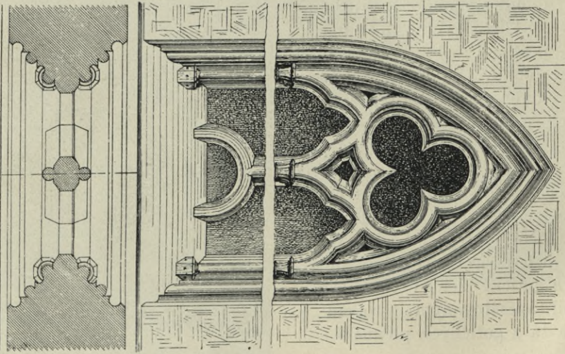
Obr. 423. Zvlkov. Kružby okenní v sluchách záp. traktu, v kapti (vých. strana) a v předstíni.
