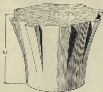
Obr. 361. Velká Blánice. Kostel. Náběhy žeber na vrcholu klenebního sloupu.
