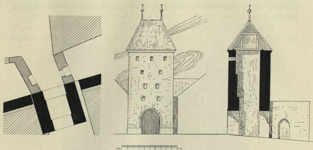
Obr. 187. Písek. Pražská brána. Půdorys, nárys vnitřní strany a řez.
