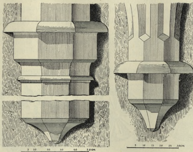
Obr. 237. Písek. Děk. kostel. Přípora v hlavní (v levo) a konsola v boční (v pravo) lodi.
