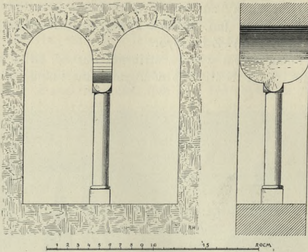
Obr. 118. Mírotice. Románské okénko ve věži.
