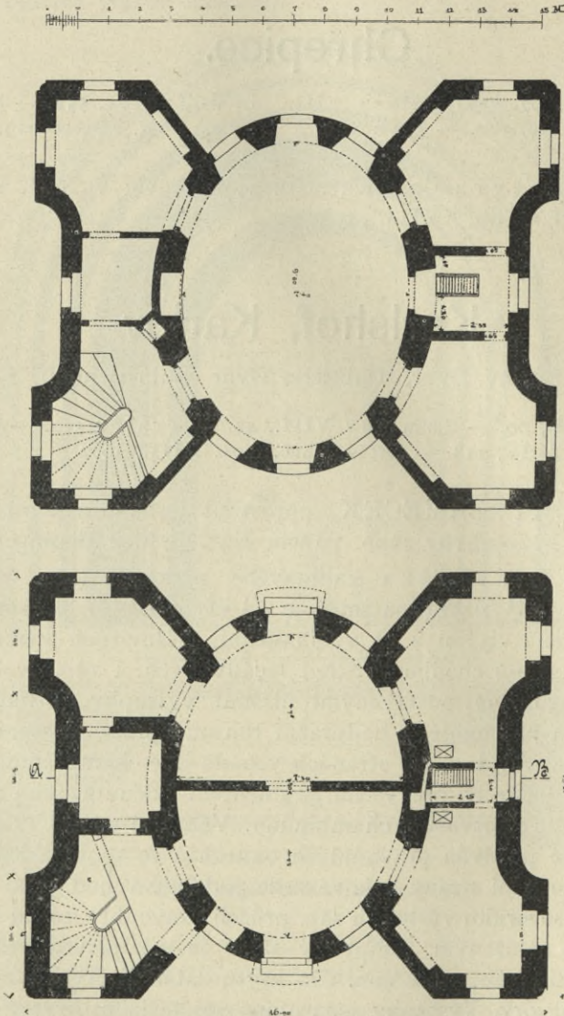
Obr. 86. Karlov. Půdorys přízemí a 1. patra zámku.
