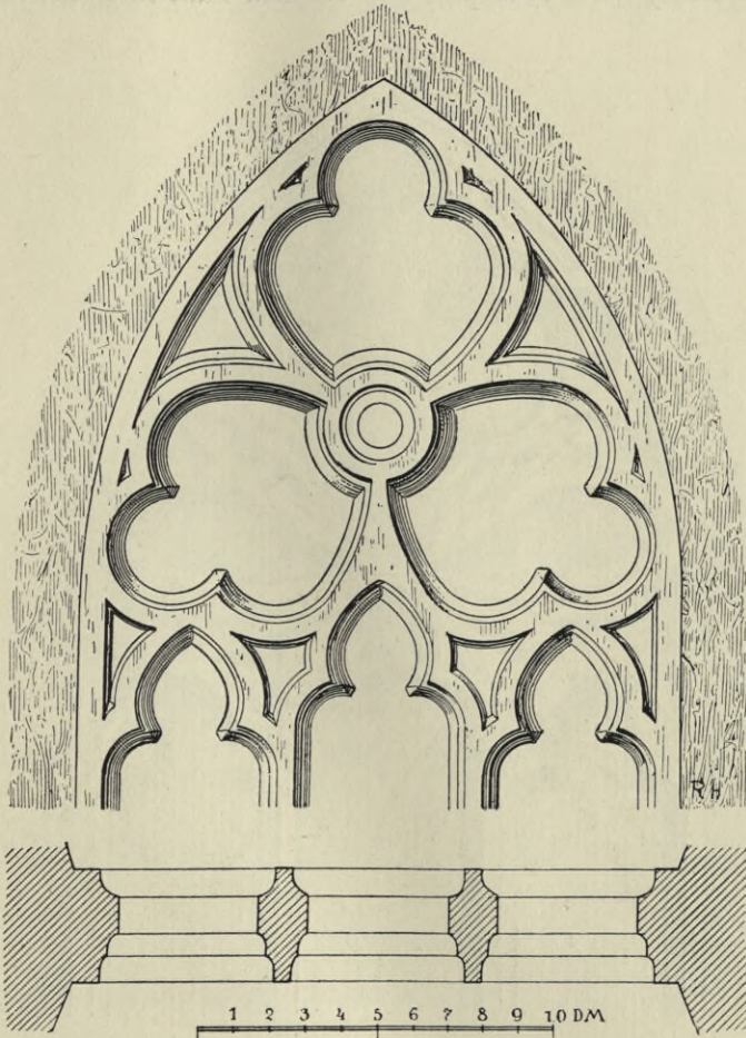
Obr. 9. Bavorov. Kostel P. Marie. Kružba v okně na jižní straně loďi.
