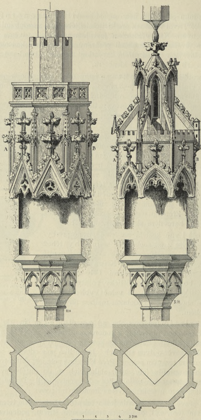
Obr. 19. Bavorov. Kostel P. Marie. Výklenky s baldachýny na triumfálním oblouku.
