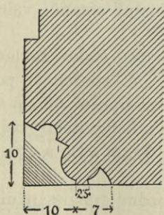
Obr. 363. Velká Blánice. Kostel. Profil žebra v presbytáři a ostění portálu do sakristie.
