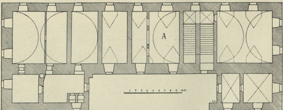
Obr. 96. Kestřany. Zámek. Půdorys.
