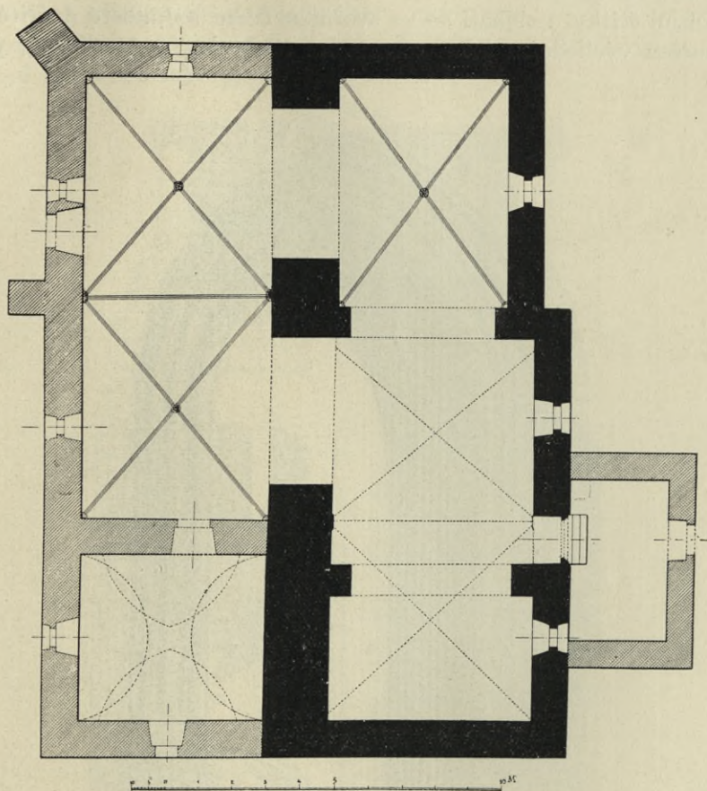
Obr. 323. Putim. Kostel. Půdorys.
