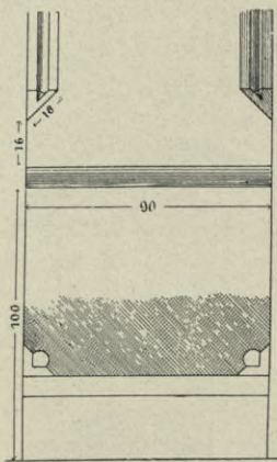
Obr. 383. Vodňany. Děk. kostel. Profil triumfálního oblouku.
