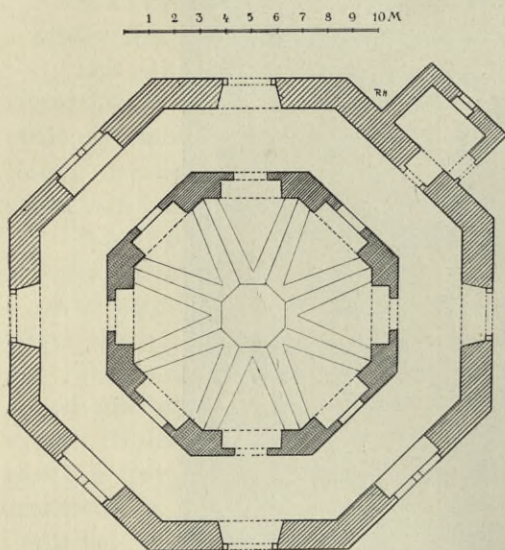
Obr. 331. Skočice. Půdorys kostela.
