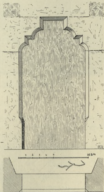
Obr. 274. Písek. Dům „U páva“. Portálek v průjezdě.
