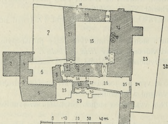
Obr. 7 Bystřice Nová. Situace záuku.
