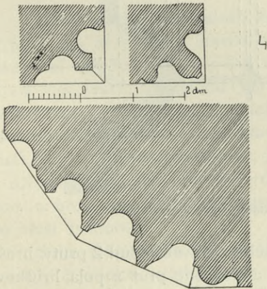
Obr. 147. Hradec J. Kostel proboštský : Profily obložení portálů, menších, jižního a severního a hlavního jižního.
