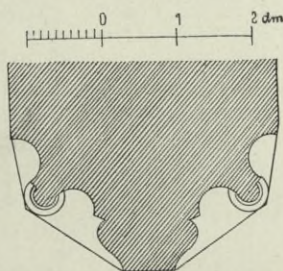
Obr. 158. Hradec J. Probošský kostel: Profil vchodu do kaple Špulfřské.
