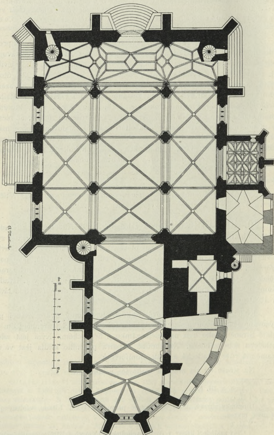
Obr. 146. Hradec J. Pádorys proboskitého kostela.
