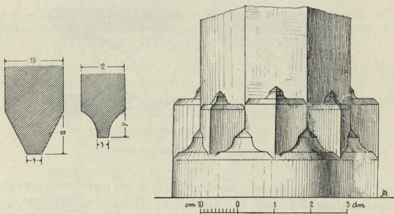
Obr. 235. Pěna Horní. Profil žeber v presbyteři a pod kúrem. Patka sloupu pod kruchtou farního kostela.
