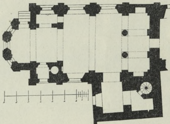
Obr. 142. Hradec J. Půdorys kostela sv. Maří Magdaleny.
