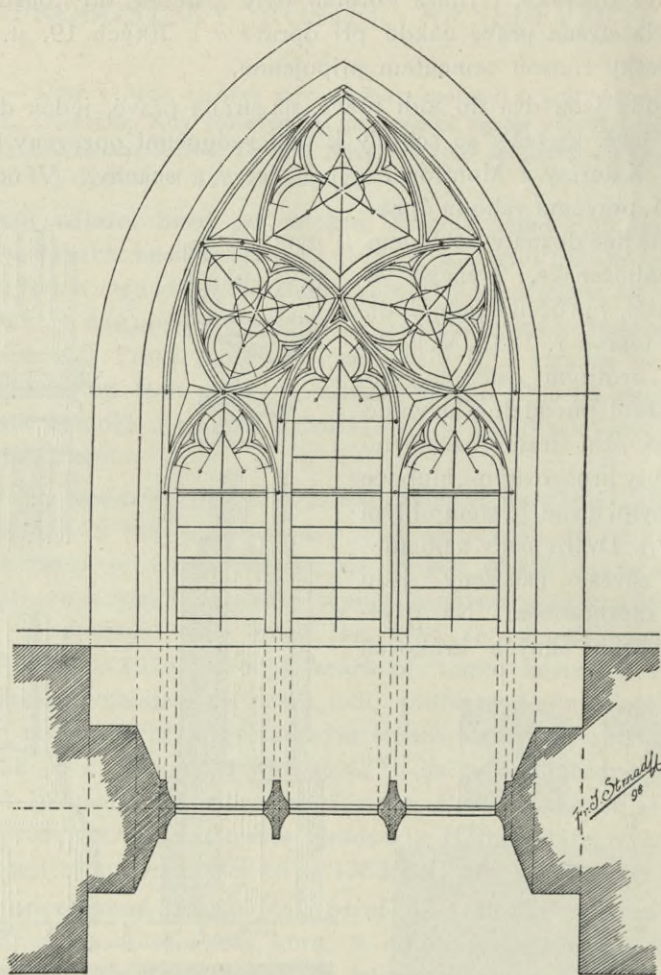
Obr. 149. Hradec J. Proboštský kostel: Okno v pravé lodi.
