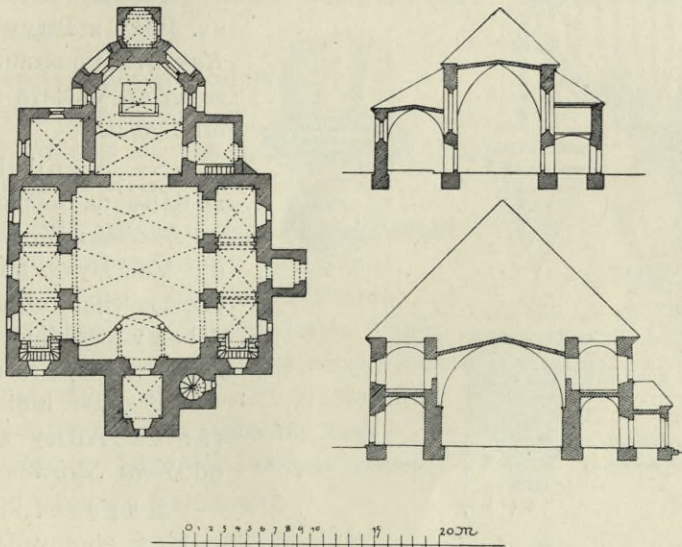
Obr. 229. Lohéřov. Kostel farní. Půdorys kostela, kolmý průřez presbytere a lodi.
