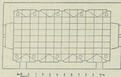
Obr. 9. Bystřice Nová. Obrazec klenutí tabulnice.
