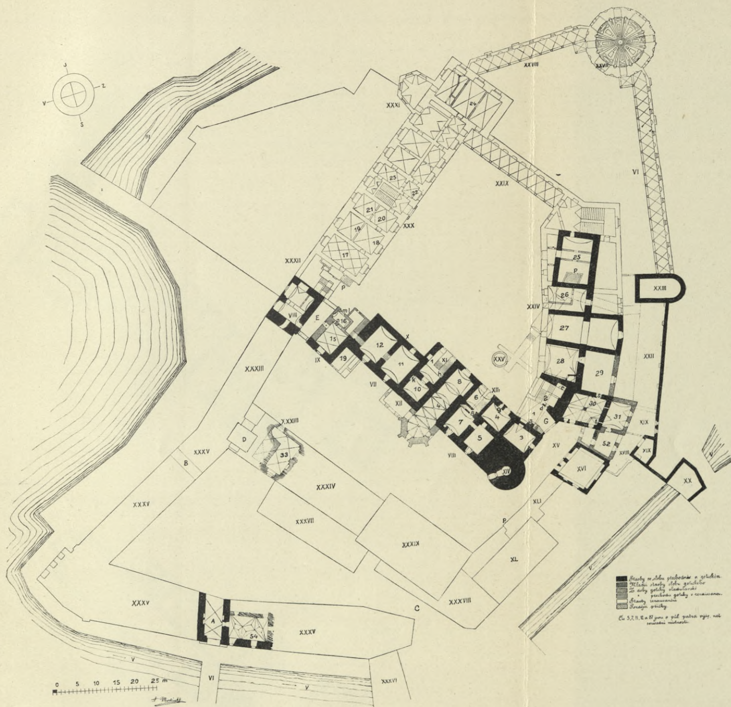
Obr. 11. Hradec J. Zámek. Půdorys přízemí.
