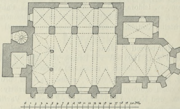
Obr. 233. Pěna Horní. Půdorys kostela.
