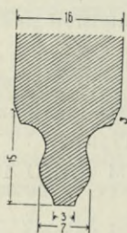
Obr. 224. Kumžak. Konsola, profil římsy a žebra v presbyteři.
