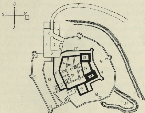
Obr. 227. Landštejn. Situace hradu dle Sedláčka.
