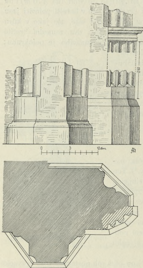
Obr. 151. Hradec J. Probošský kostel: Levý pilíř vítězného oblouku.
