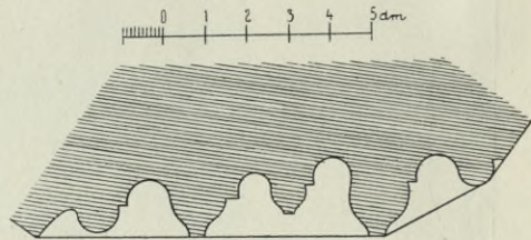
Obr. 99. Hradec J. Kostel sv. Jana. Profil portálu.
