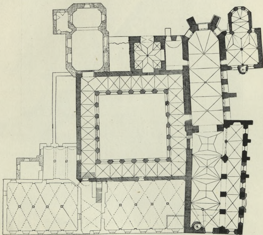
Obr. 95. Hradec J. Půdorys kostela sv. Jana Křtitele, křížové chodby, kaple a špitálu.
