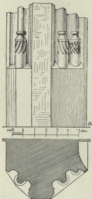
Obr. 156. Hradec J. Probošský kostel: Pilíř pod kruchtou.
