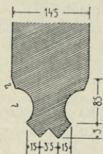
Obr. 166. Hradec J. Proboštský kostel. Profil žeber pod mladší částí kruchty.
