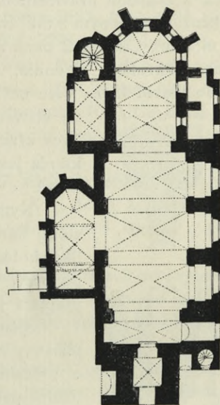
Obr. 4 Bystřice Nová. Půdorys děk kostela.
