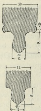
Obr. 86. Hradec J. Zámek. Profily žebér v kapli sv. Ducha v starší a mladší části.
