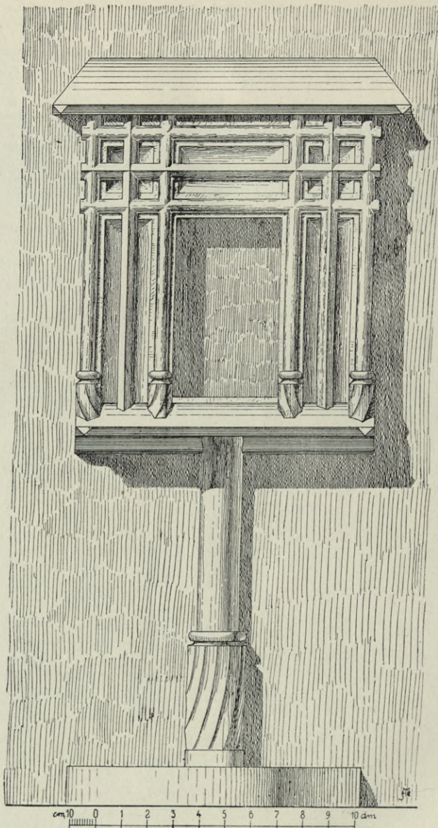
Obr. 246. Staré město. Sanktuarium farního kostela.
