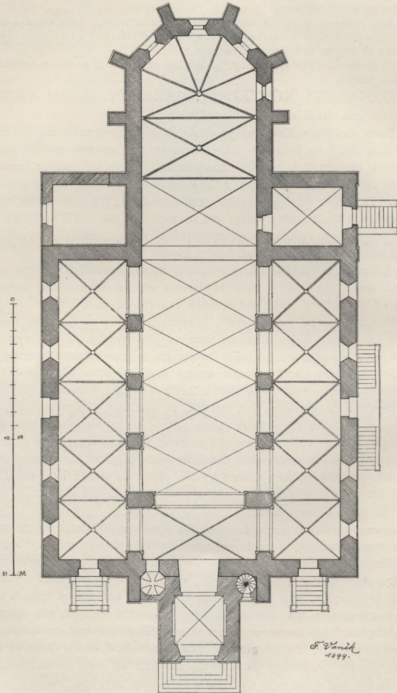
Obr. 19. Hory Kašperské, Půdorys děkanského kostela.
