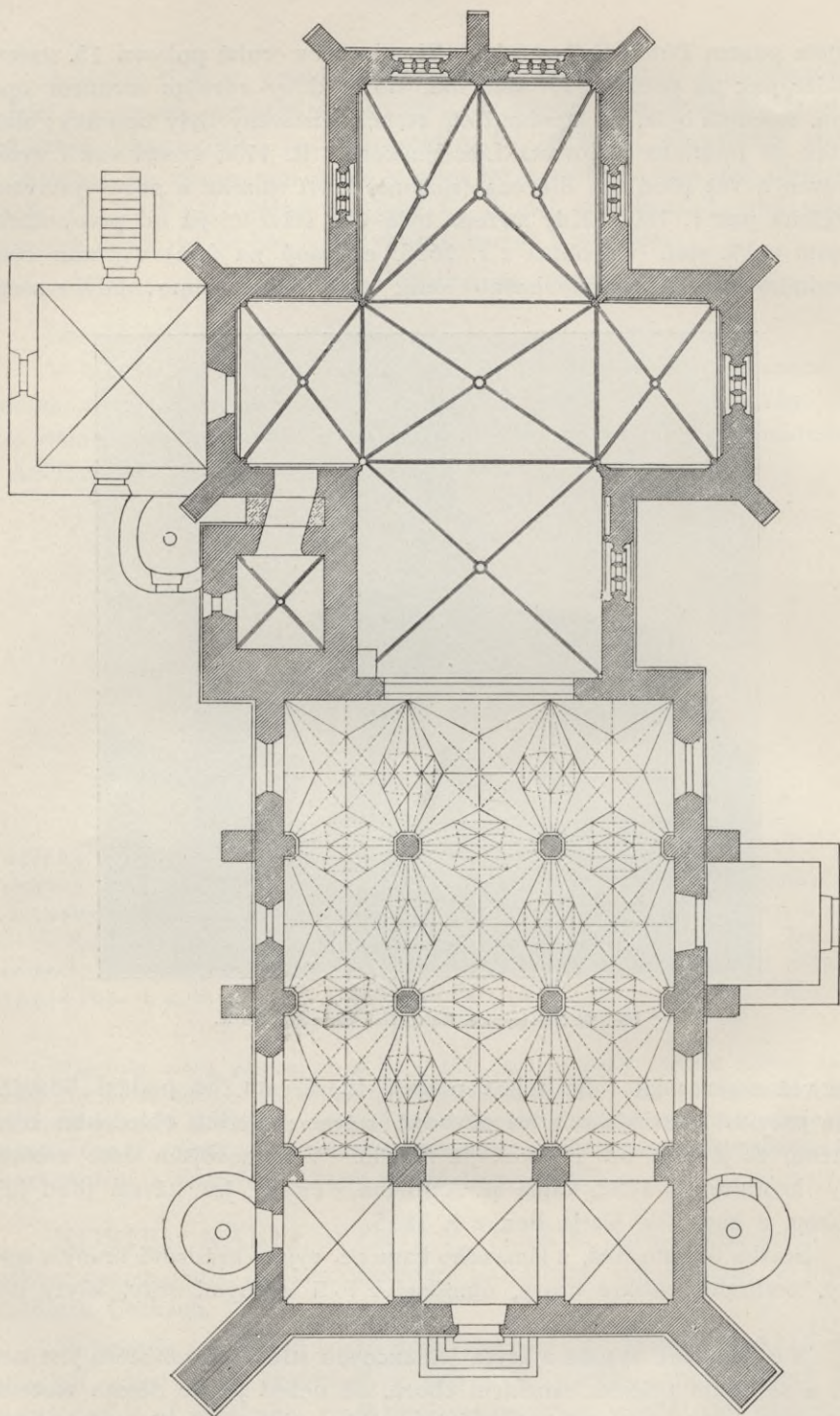
Obr. 51. Nezamyslice. Půdorys kostela.
