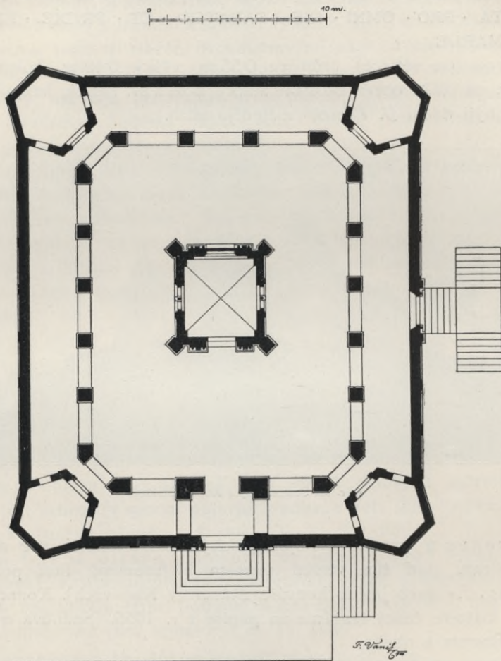
Obr. 93. Sušice. Půdorys kaple Anděla Strážce.
