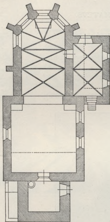
Obr. 137. Zbynice. Půdorys kostela.
