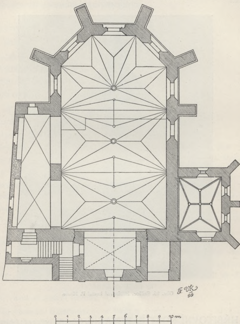
Obr. 87. Sušice. Půdorys hřbitovního kostela.
