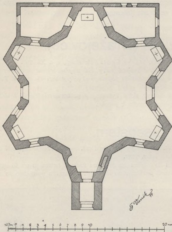
Obr. 15. Eisenstein. Půdorys kostela.
