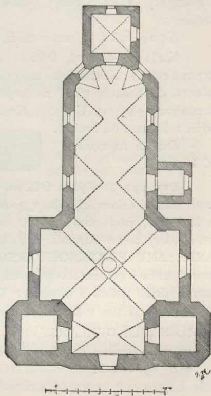
Obr. 77. Seewiesen. Půdorys kostela.
