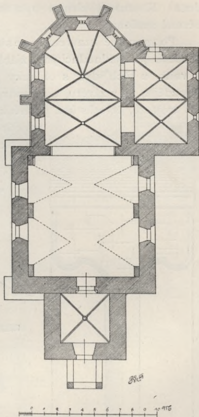
Obr. 124. Vzduny. Půdorys kostela.
