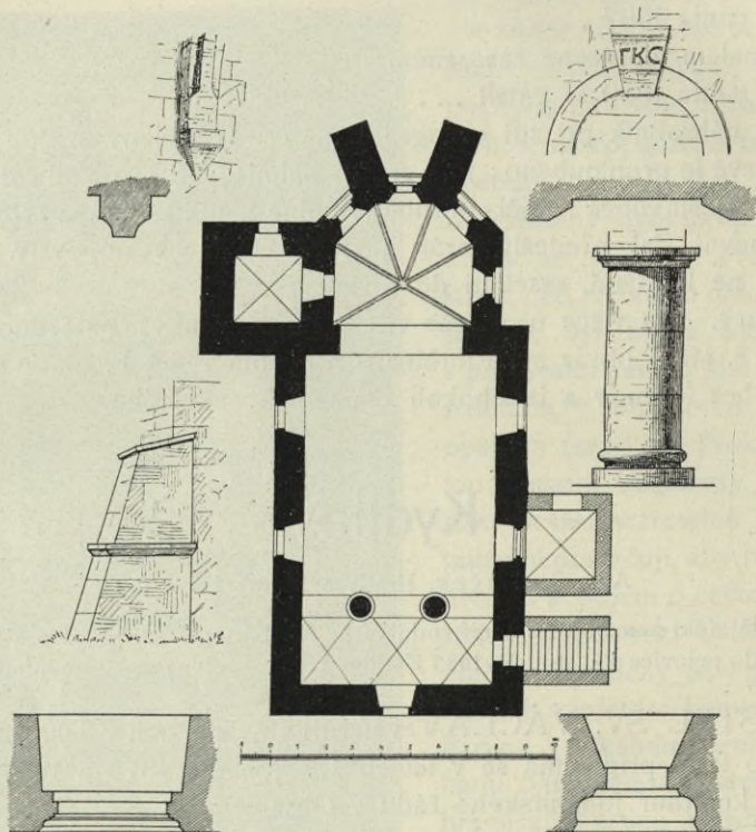
78. Kydliny. Půdorys kostela sv. Václava.
