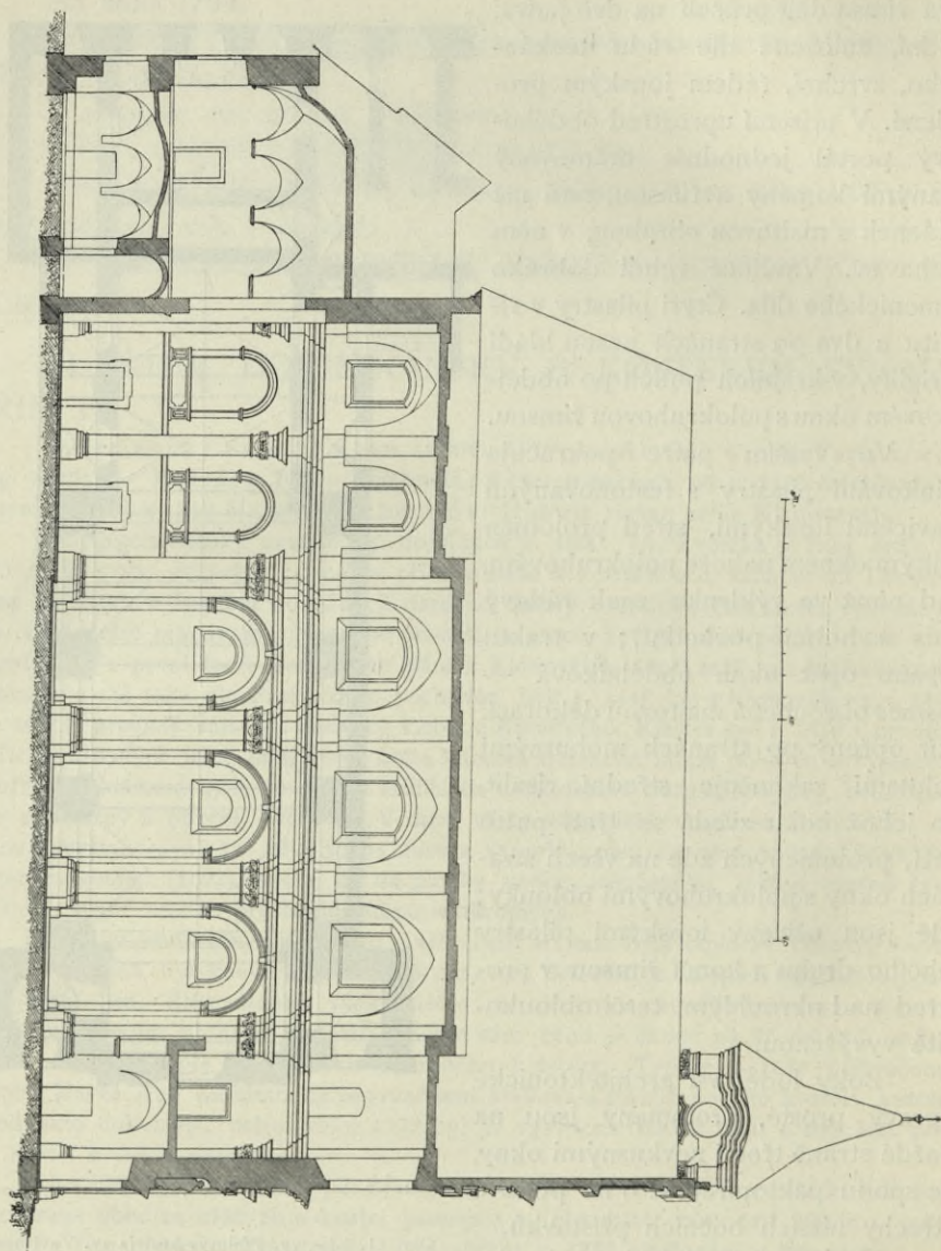
Obr. 52. Klášter. Podélný řez chrámu sv. Vavřince.
