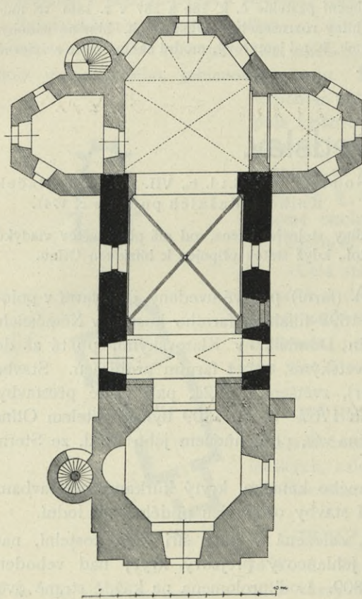
Obr. 101. Předslav. Půdorys kostela sv. Jakuba.
