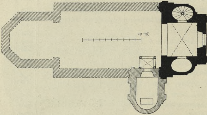
Obr. 17. Chudějnice. Věž bývalého kostela sv. Volfganga a kaple.
