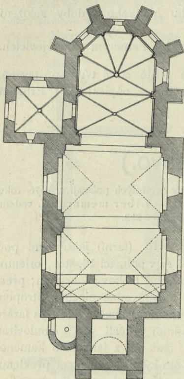
Obr. 84. Myslív. Půdorys kostela.
