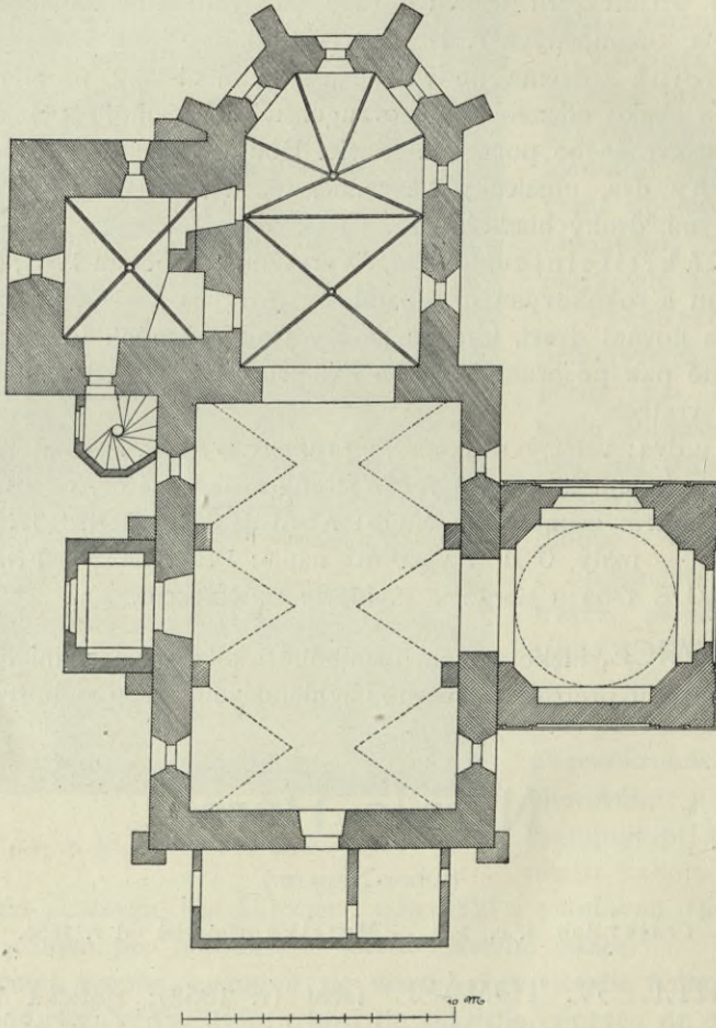
Obr. 93. Nýrsko Horní. Půdorys farního kostela.
