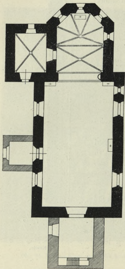
Obr. 96. Poleň. Pádorys farního kostela.
