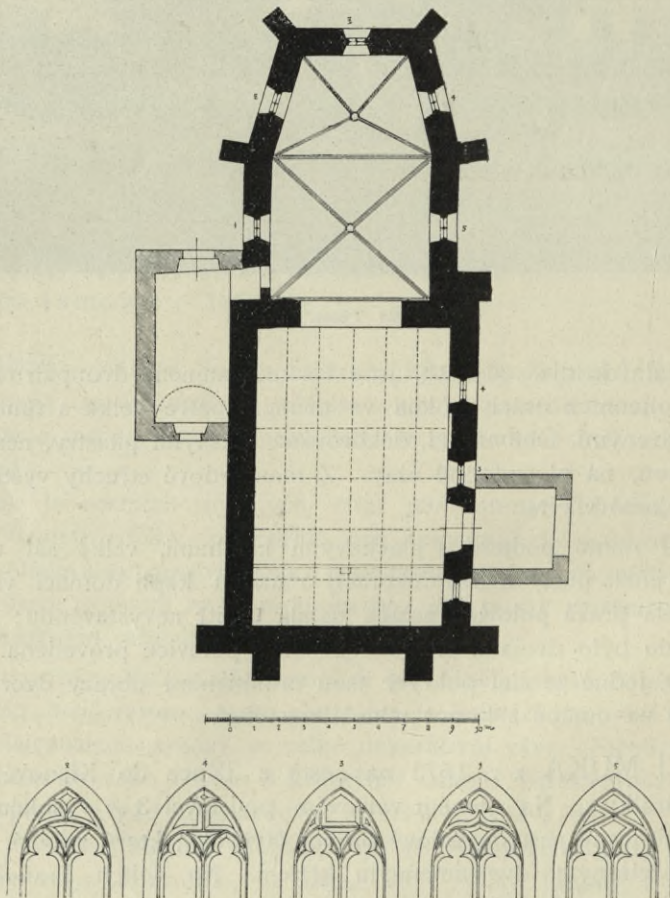
Obr. 124. Uhlíště. Půdorys kostela a kružby okenní.
