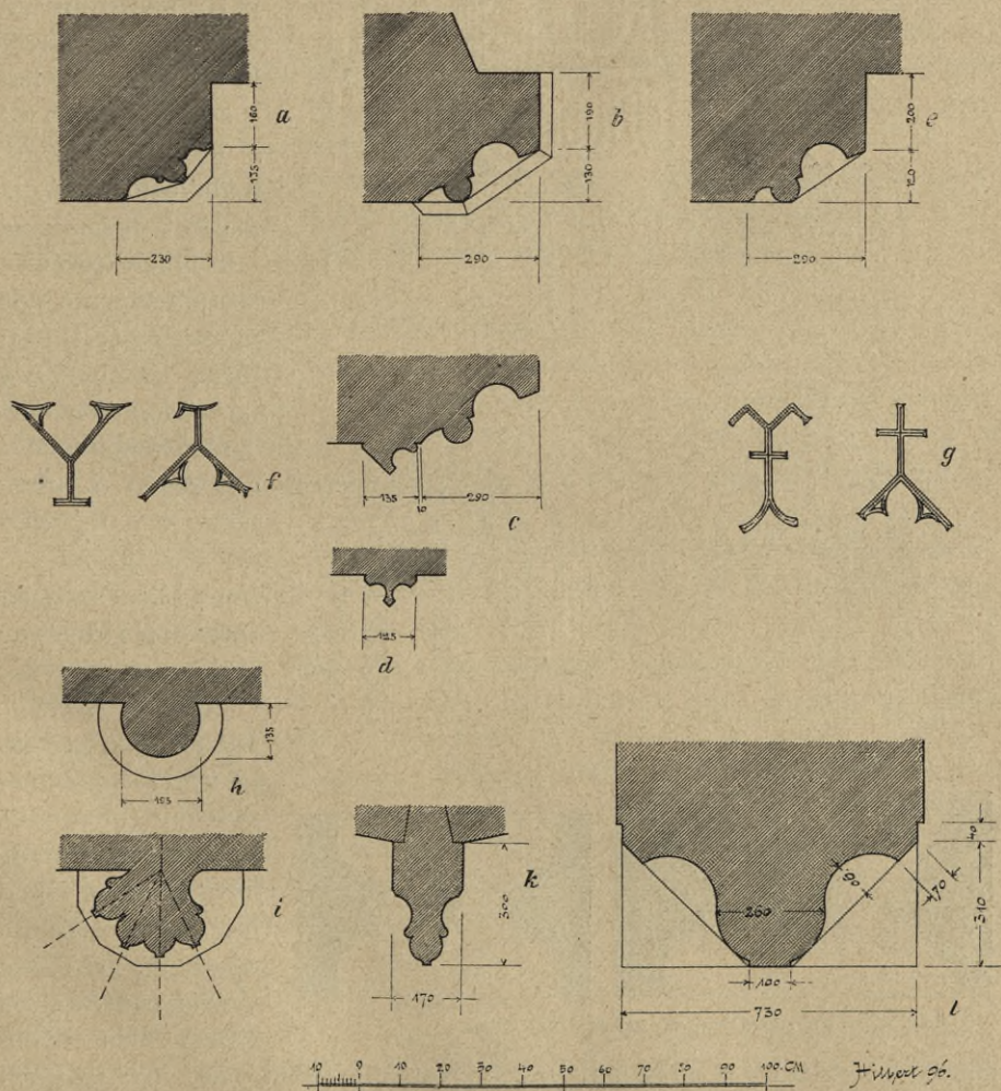
Obr. 39. Louny. Profily z kostela sv. Petra. a, portál severní; b, c, d, portál západní; e, portál jižní; f, g, kamenické značky; h, přípory; i, k, žebra; l, vítězný oblouk.
