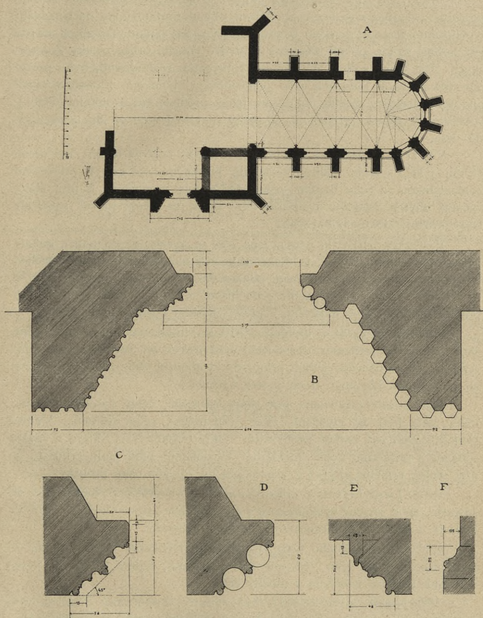
Obr. 34. Týnec Panenský. Klášterní kostel: A , půdorys kostela; B , C , D , portál; E , pažení výklenku pro křeslo biskupské; F , trnož.
