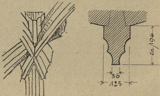
Obr. 27 a 28. Louny. Žebra klenbová v kostele sv. Mikuláše.
