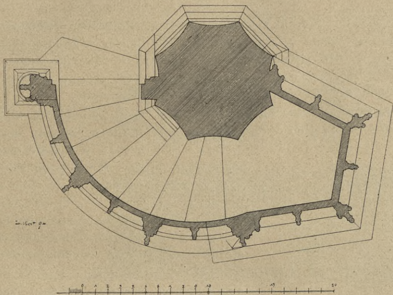
Obr. 31. Louny. Vodorovný řez kazatelnou v kostele sv. Mikuláše.
