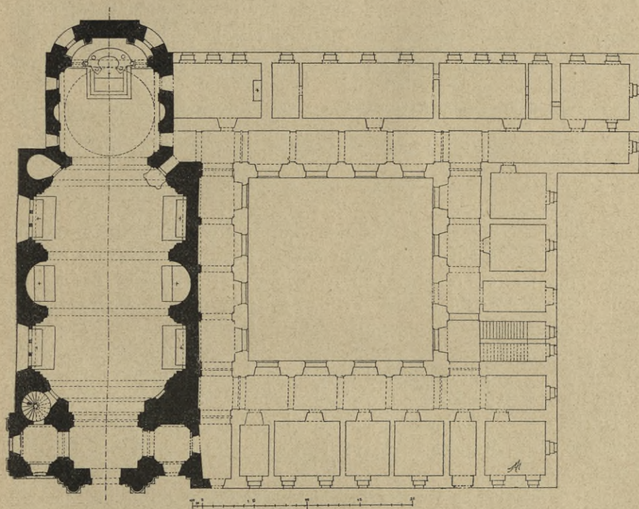
Obr. 64. Ročov dolní. Půdorys kostela a kláštera.
