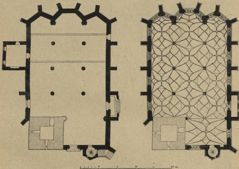
Obr. 19. Louňany. Půdorys a klenba kostela sv. Mikuláše. Kreslil arch. J. Mockrer.
