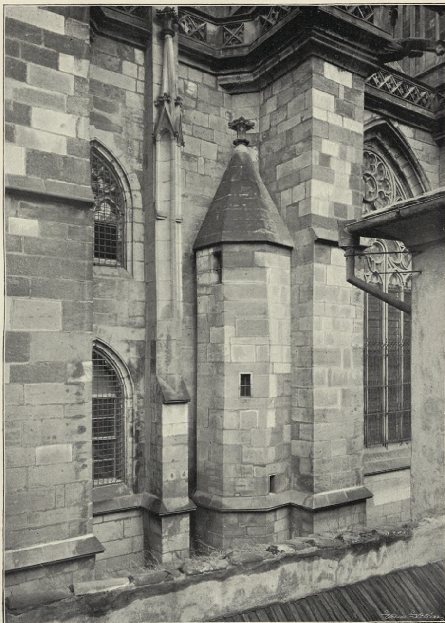
Obr. 32. Schodová vížka u sakristie.
