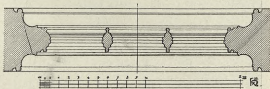
Obr. 14. Ostění a kružby v kaplích polygonálního ochozu.
