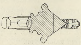
Obr. 73. Profil vrchního opěrného oblouku.
