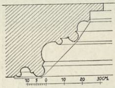
Obr. 50 a. Profil vchodu sakristie.
