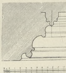
Obr. 111. Ostění oken první zvonice. A jižní, B západní a severní.
