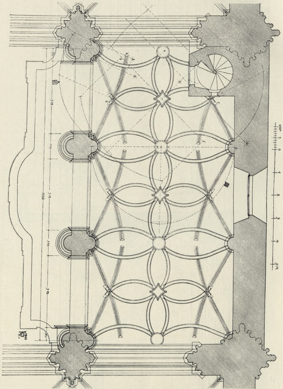
Obr. 125. Hudobny hudební kručky ; prvé patro.
