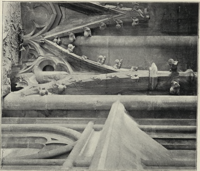
Obr. 115. Výzdoba opěrných piliřů věže: a ve výši hlavních římsy lodi křížové, b nad křížovou lodí (před opravou).
