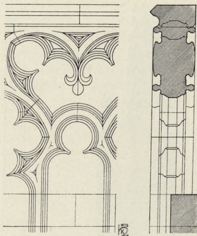
Obr. 76. Zábradlí nadokenní vysoké lodi a chóru.
