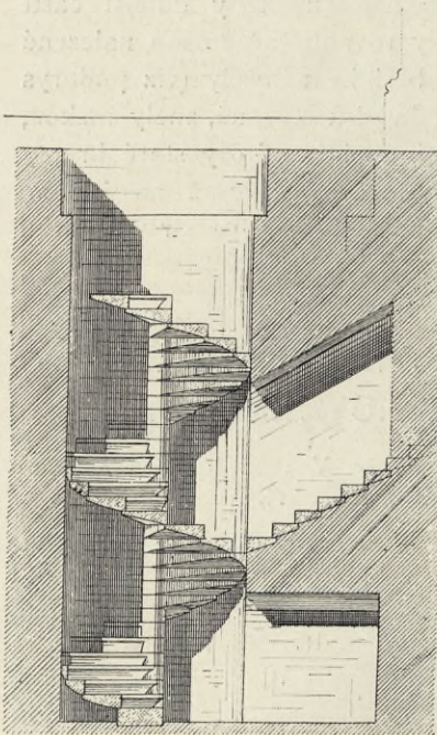
Obr. 6. Vřetenové schodiště objevené při kopání základů pro novou stavbu.
