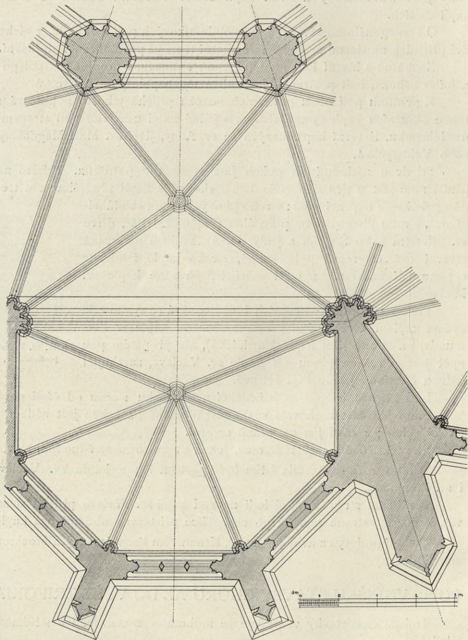
Obr. 13. Púdorys kaplí Matyáše z Arrasu.
