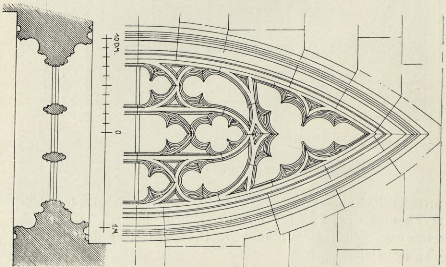
Obr. 55. Kružba oken v jižní stěně kaple sv. Václava.
