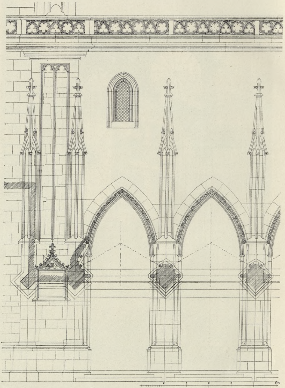
Obr. 83. Průčelí jižní předsíně.
