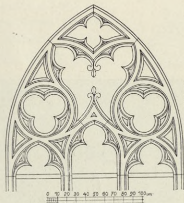
Obr. 22. Kružba okna kaple sv. Maří Magd.
