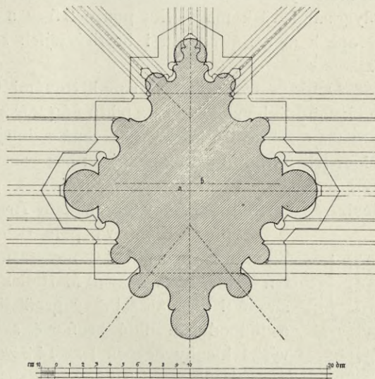
Obr. 38. Pilíře Petra Parléře.
