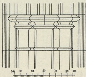
Obr. 63. Hlavice pilířů pod hlavní klenbou.
