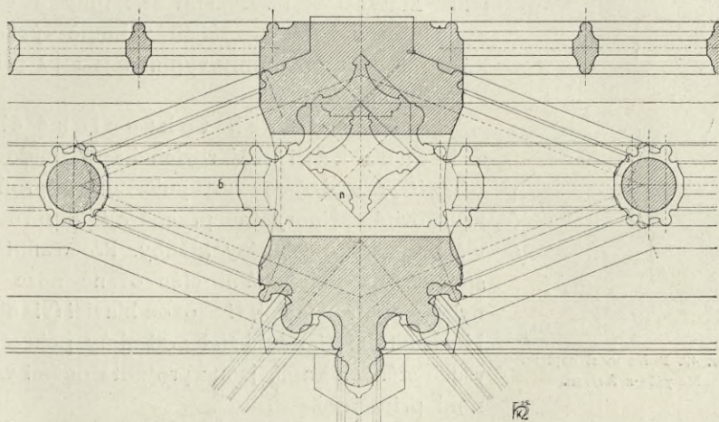
Obr. 39. Pilíř Petra Parléře v triforiích se zakresleným vyvinutím až ku galerii.
