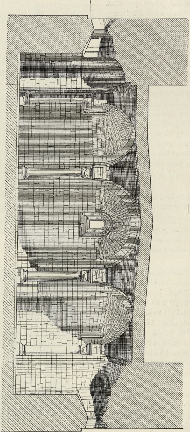
Obr. 3. Přičný řez bývalé románské krypty.
