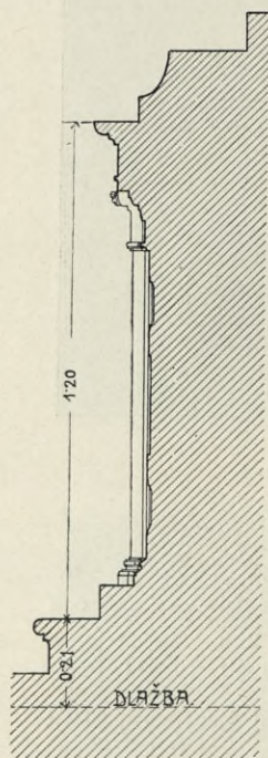
Obr. 230. Řez postranní stěnou král. mauzolea. 1/30 skut. velikosti.
