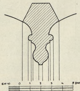
Obr. 64. Průsek žebra klenby chóru.
