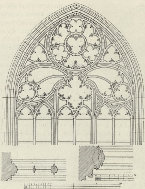
Obr. 28. Kružba oken kaple Martinické.
