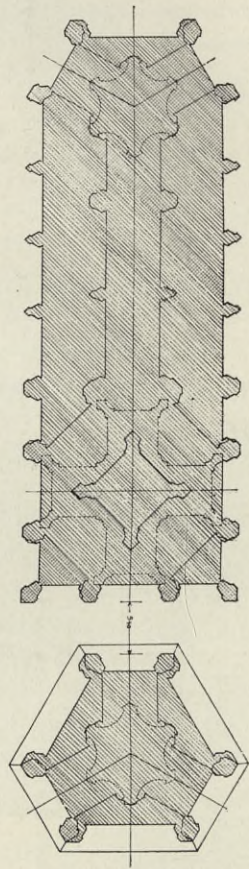
Obr. 72 a. Púdorys opěrného pilíře nad kapli sv. Kříže.
