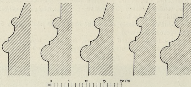
Obr. 101. Článkování trnože severního portálu kaple sv. Václava, vnitřku téže kaple, jižní předsíně, západního portálu a opěrných pilířů kaple sv. Václava.
