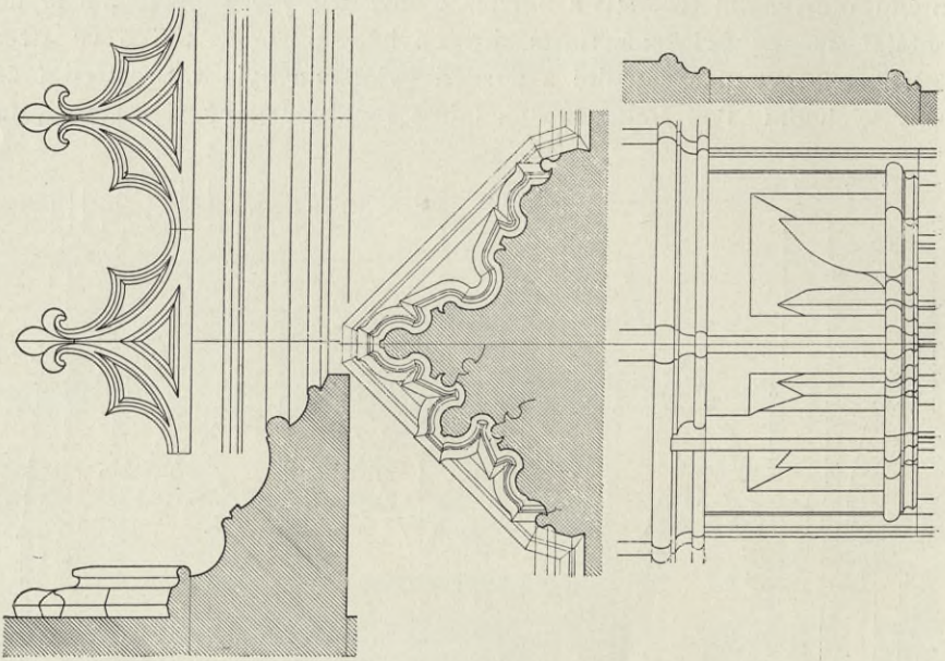
Obr. 54. Přezední pilř a římsa v kapli sv. Václava.
