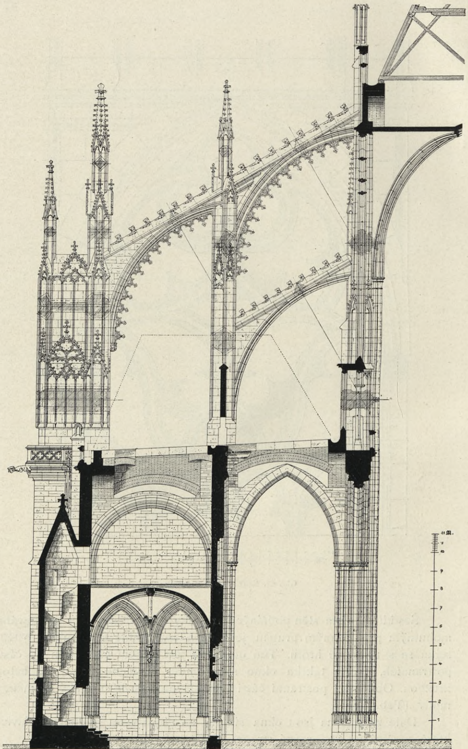
Obr. 68. Vzpěrný systém (řez sakristií, pokladní komorou, boční lodí, triforiem a vysokou lodí).
