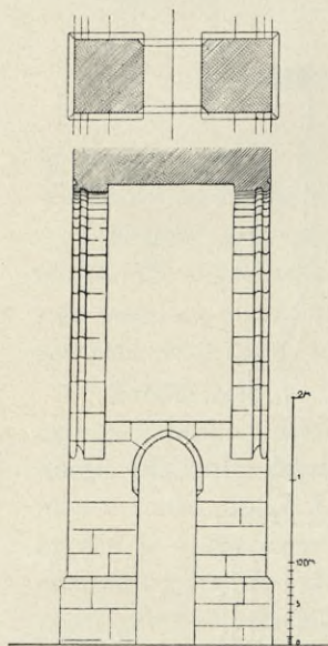
Obr. 119. Střední pilíř spojovacího mostu mezi oratoří a král. hradem. (Půdorys a příčný řez.)
