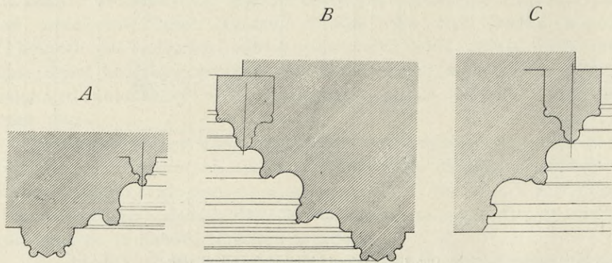
Obr. 112. Ostění oken druhé zvonice, A západní, B jižní a severní, C východní.
