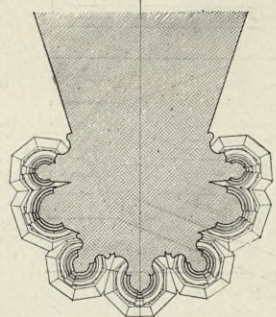
Obr. 42. Pilíře mezi kaplemi Matyáše z Arrasu.
