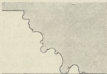
Obr. 99. Ostění portálu západního.
