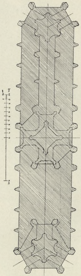
Obr. 72 b. Púdorys opěrných pilířů nad kaplemi polygonu.
