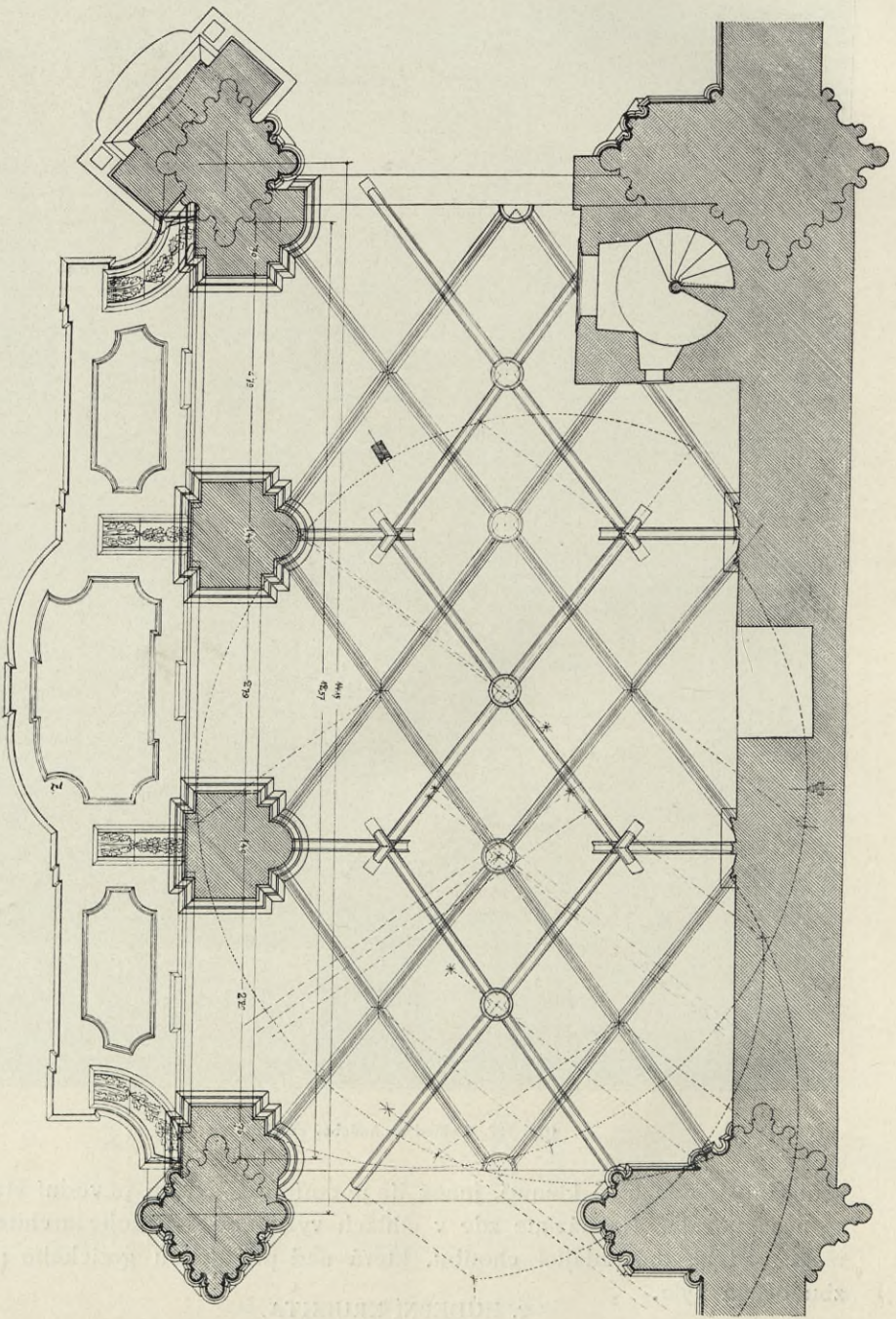
Obr. 123. Půdorys hudební křehy; přizemí.
