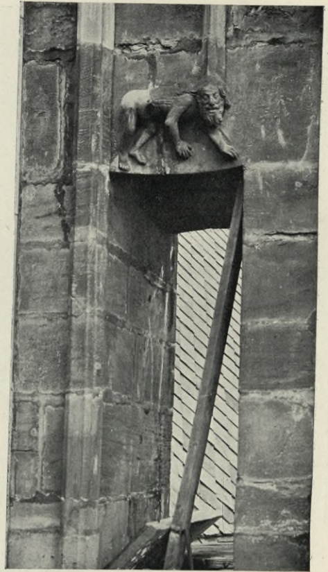
Obr. 164. a 165. Průchody v opěrných pilířích nad kaplemi.
