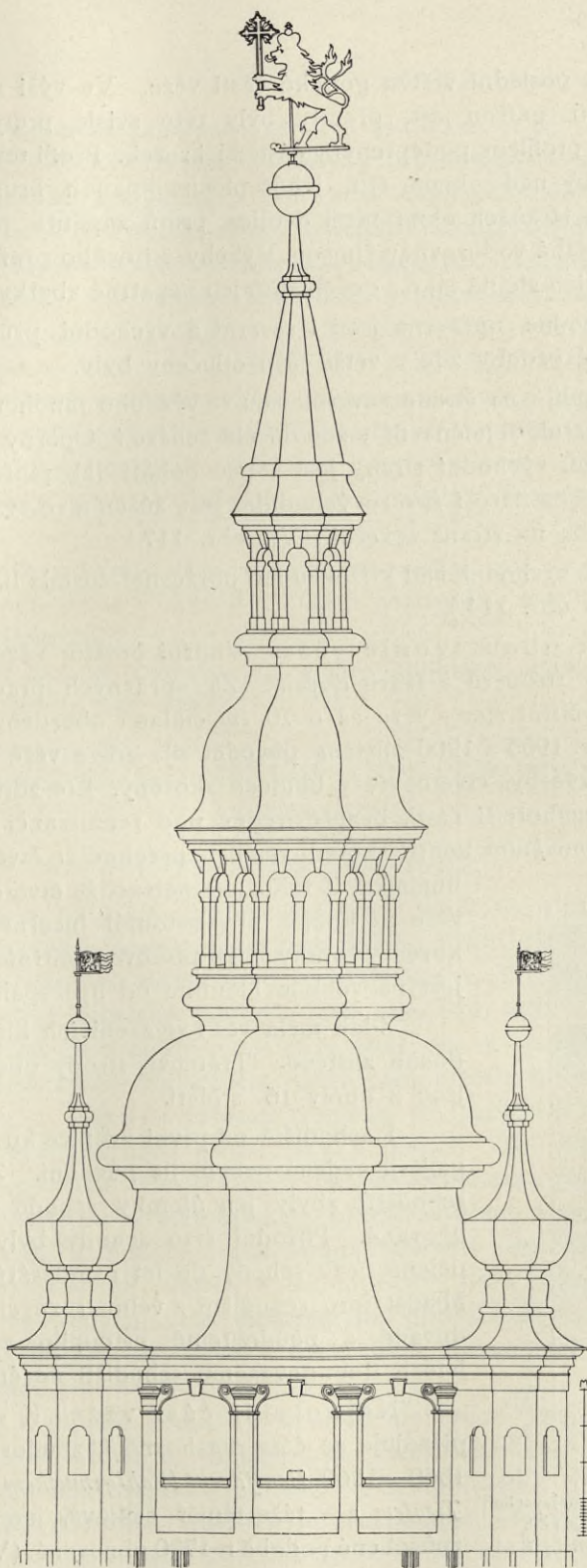
Obr. 118. Nárys helmice věže v pohledu z jihu.
