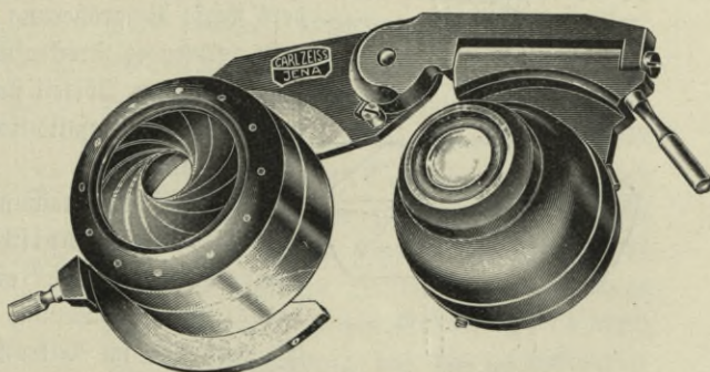
Abb. 229. Ausklappbarer Kondensor, links die Friszylinderblende.
