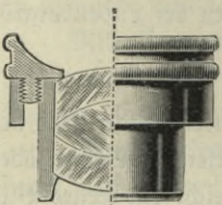
Abb. 247. Aplanatische Lupe nach Steinheil.
