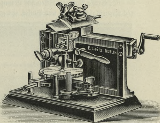
Abb. 22. Schanze-Mikrotom mit Kurbelführung, automatischer Schnittdickeneinstellung und Feinübertragung für 1-5\mu -Schnitte.
