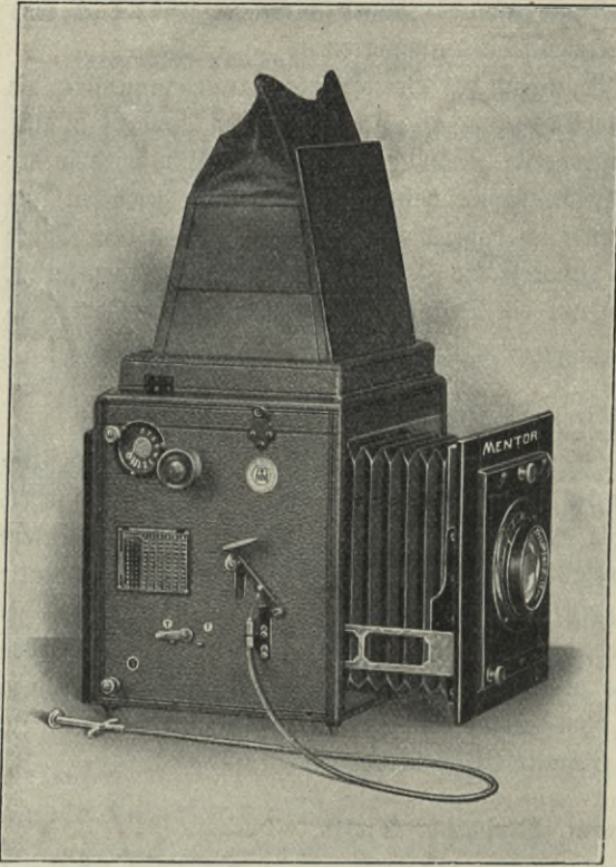
Abb. 255. Spiegelreflexkamera von Goltz und Breitmann, Dresden.
