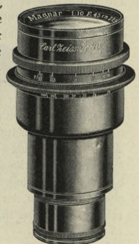
Abb. 263. Zeiß-Magnar.
