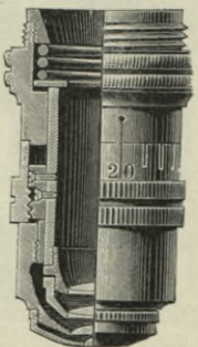
Abb. 224. Starkes Objektiv mit Korrekzionsfassung.
