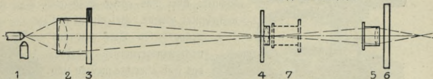
Abb. 275. Beleuchtung (Strahlengang) mit starker Lichtquelle (Bogenlicht) und Brillenglaskondensor. 1 Lichtquelle, 2 Kollektor, 3 Kollektorblende, 4 Sammellinse, 5 Brillenglaskondensor, 6 Tisch des Mikrostops, 7 Polarifator oder Filter.
