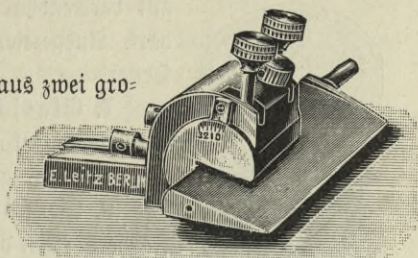
Abb. 27. Verstellbarer Messerhalter.
