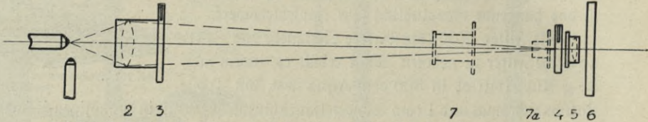
Abb. 277. Beleuchtung (Strahlengang) mit Bogenlicht und Abbeschem Beleuchtungsapparat.
