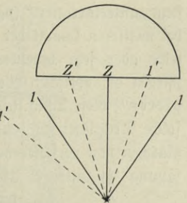
Abb. 214. Schema für schiefe Beleuchtung; oben die Frontlinse.
