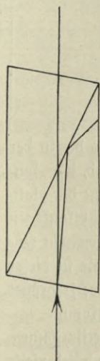
Abb. 196. Nicol'sches Prisma.
