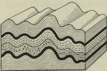
Abb. 336. Blockdiagramm: Gefaltete Gesteinschichten.
