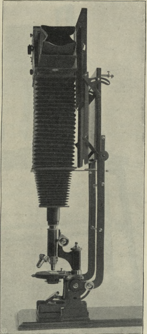
Abb. 281. Wie Abb. 280, doch Zwischenschaltung eines Balgen, um stärkere Vergrößerungen zu erhalten.
