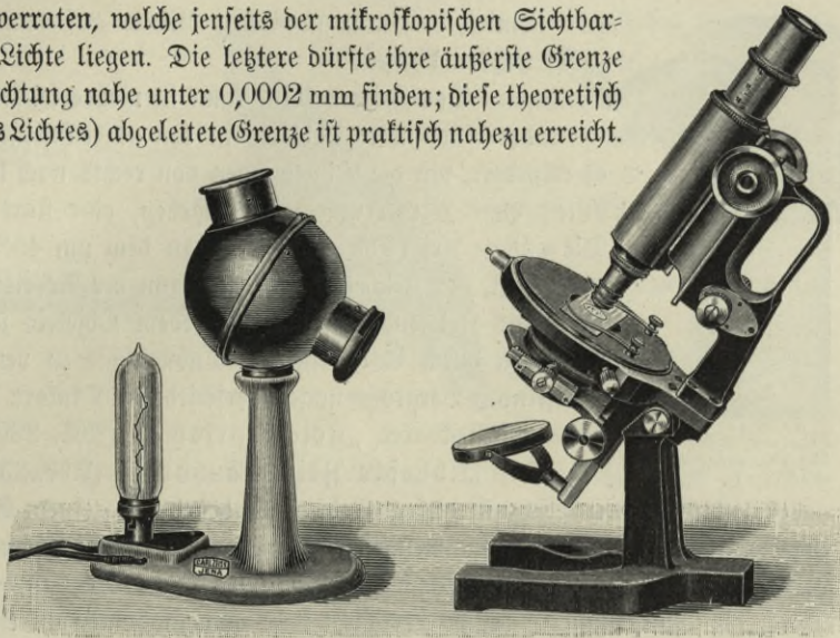
Abb. 233. Mikroskop mit Kernlampe, für Dunkelfeldbeleuchtung.
