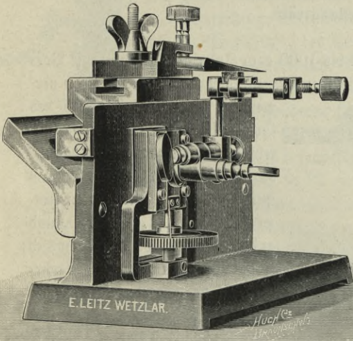
Abb. 21. Schanze-Mikrotom für Handführung.
