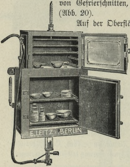
Abb. 19. Thermostat mit Aufsatz. Modell des anatomisch-biologischen Instituts in Berlin.
