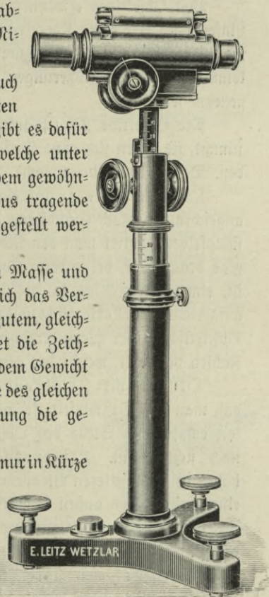
Abb. 239. Ablesemikroskop.
