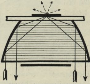
Abb. 230. Paraboloidkondensfor.
