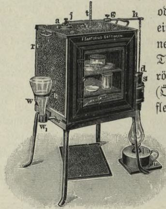
Abb. 18. Einfacher Thermostat mit Lampenheizung.
