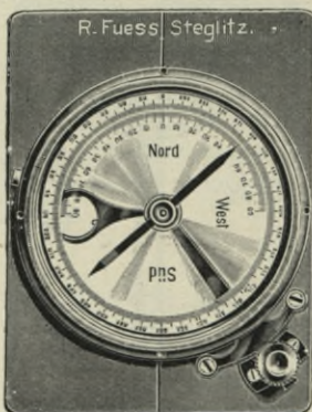
Abb. 307. Bergkompaß mit Klinometer der Firma R. Fueß.
