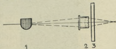
Abb. 274. Beleuchtung (Strahlengang) mit Gasglühlicht und Brillenglaskondensor. 1 Lichtquelle, 2 Brillenglaskondensor, 3 Tisch des Mikrostops.
