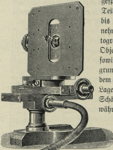
Abb. 278. Objektisch für Mikrophotographie mit auffallendem Licht nach Wandollef.
