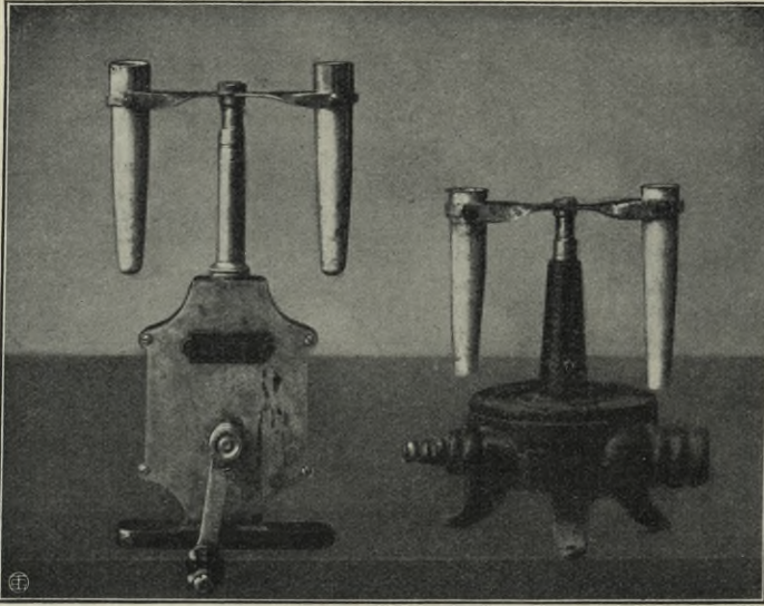
Abb. 86. Planktonzentrifugen.
