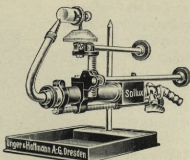
Abb. 273. Solluxbrenner von Unger & Hoffmann, Dresden.
