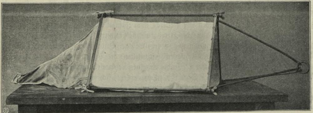
Abb. 85. Even Ekmanns „Doppelrahmige Netzredge“.
