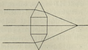
Abb. 198. Schema der Bikonverglinse.
