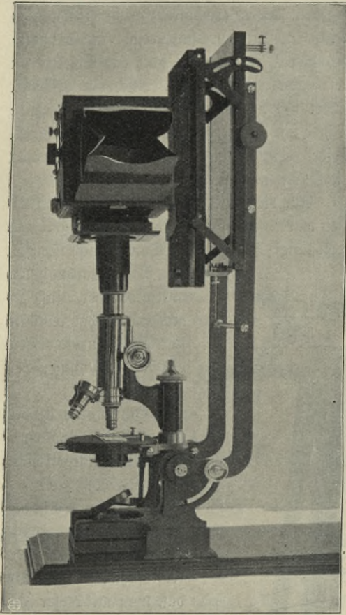
Abb. 280. Spiegelreflexkamera von Goltz-Breutmann in Verbindung mit Mikroskop. Geringe Vergrößerung.
