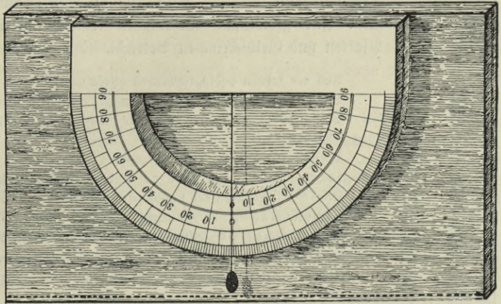
Abb. 308. Selbstverfertigtes Alinometer (Neigungsmesser).
