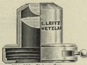
Abb. 228. Kleiner Kondensor mit feststehender Frisblende.
