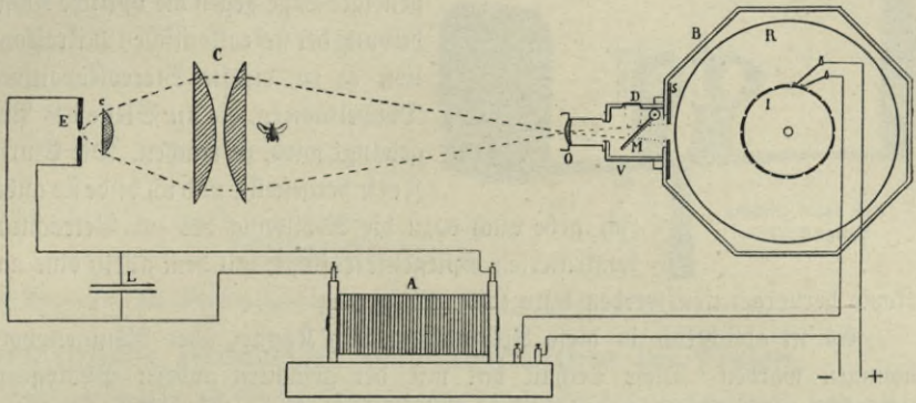
Abb. 283. Einrichtung nach Lucien Bull zur Kinematographie des Insektenflügelchlags.
