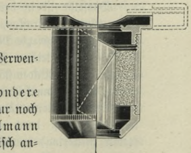
Abb. 243. Polarisator.
