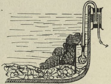
Abb. 172. Selbstregulierende Ablaufvorrichtung.
