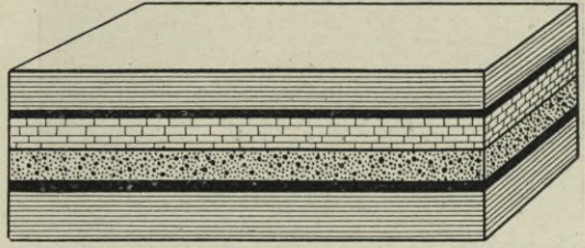
Abb. 335. Blockdiagramm: Wagerichte Gesteinschichten.
