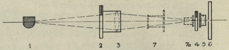
Abb. 276. Beleuchtung (Strahlengang) mit Gasglühlicht und Abbeschem Beleuchtungsapparat. 1, 2, 3 wie in Abb. 275 7 oder 7a Polarisor auf Meier im Abbe, oder Filter, 4 Zris des Abbe, 5 Abbe, 6 Tisch des Mikroskops.
