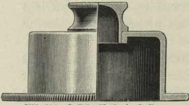
Abb. 225. Zylinderblende in Fassung.
