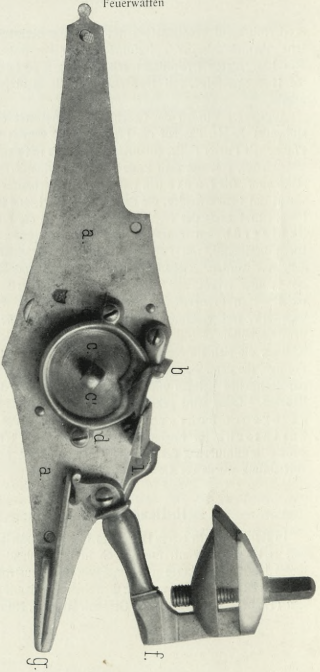
Fig. 69. Deutsches Radschloß, Vorderseite.
