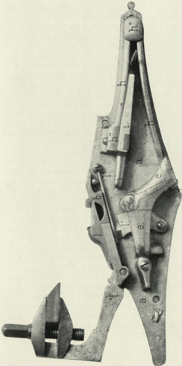
Fig. 70. Deutsches Radschloß, Innenseite.
