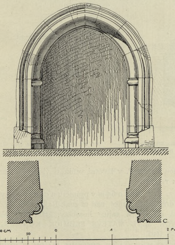
Obr. 286. Veliz. Far. kostel sv. Jana Křt. Portál v západní zdi.
