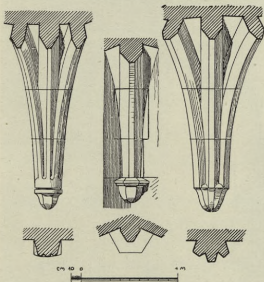
Obr. 245. Senomaty. Farní kostel sv. Vavřince. Patky klenbové s konsolkami. V levo a uprostřed z kněžiště, v pravo z lodi.
