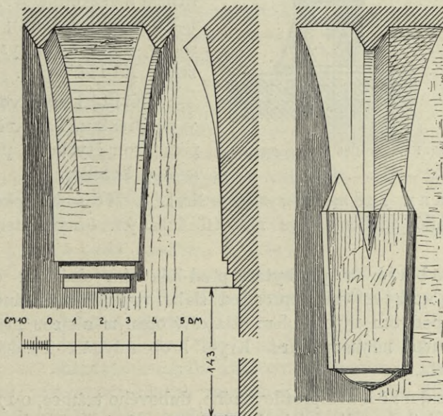
Obr. 183. Rakovník. Kostel sv. Jiljí. Patky klenbové v kněžišti.
