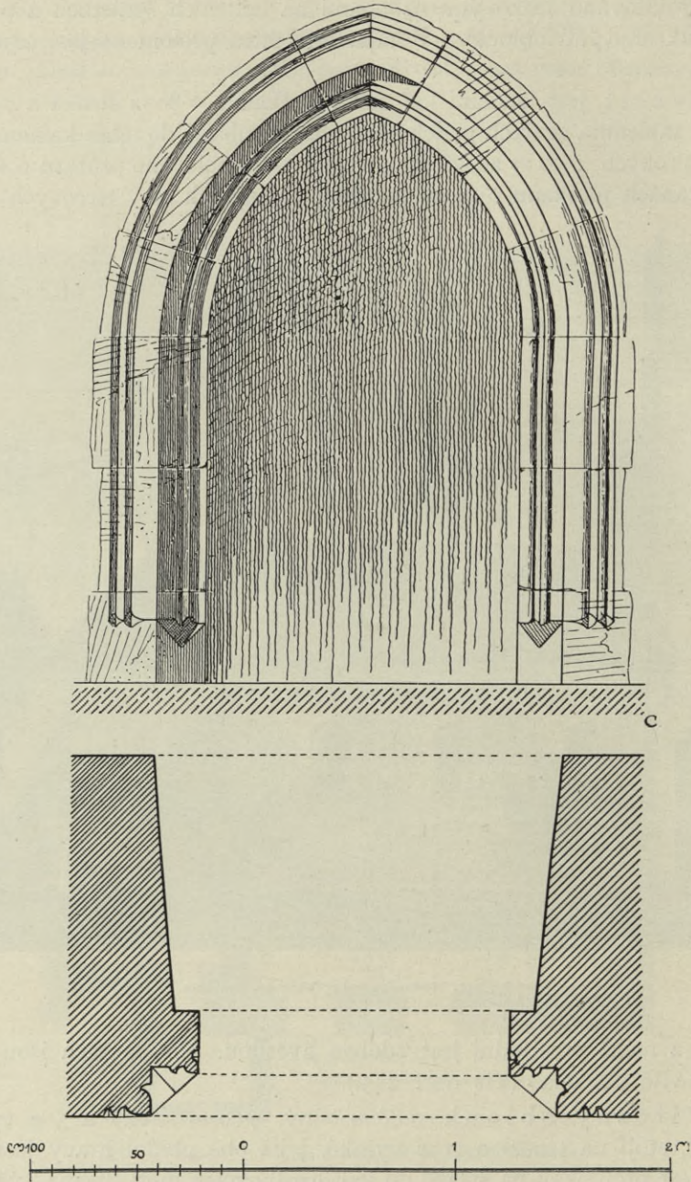
Obr. 244. Senomaty. Farní kostel sv. Vavřince. Západní vchod.
