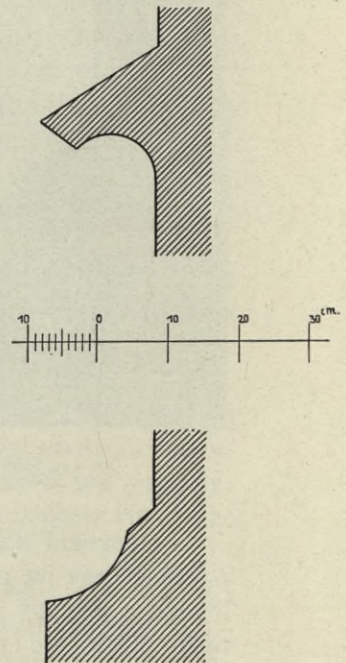
Obr. 136. Rakovník. Chrám sv. Bartoloměje. Průsek římsou trnožní a pasovou.
