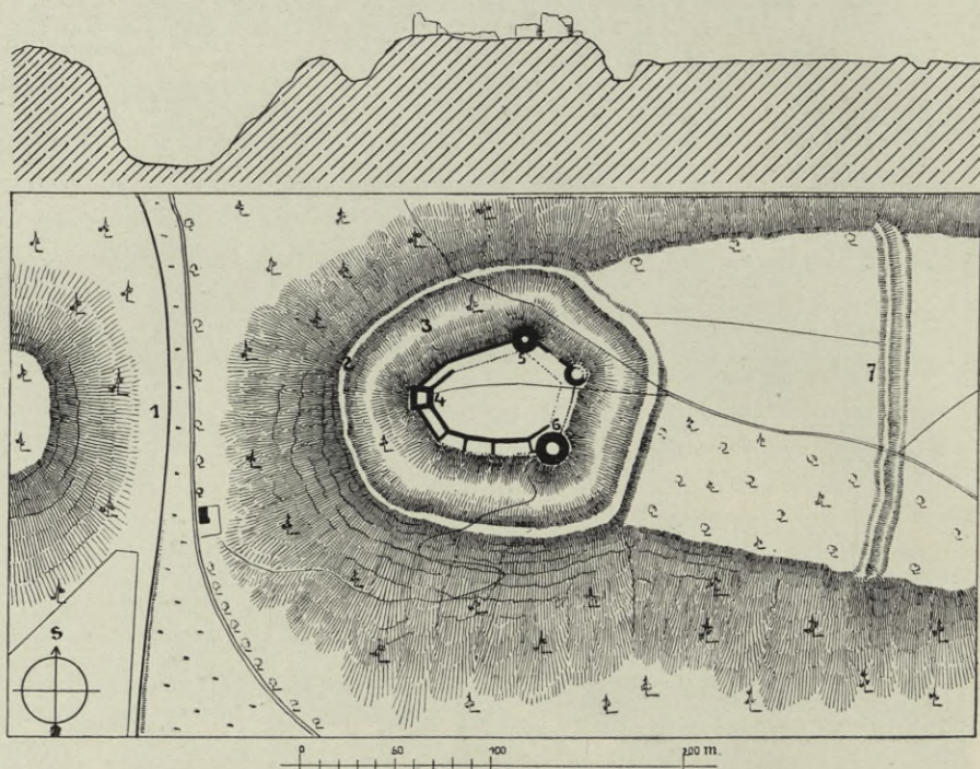
Obr. 300. Žbán. Hrad. Situace a řez.
