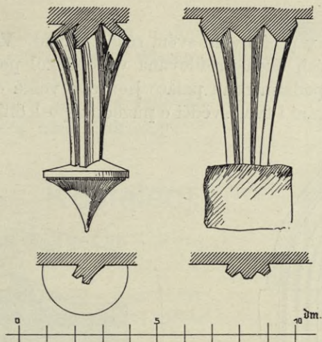
Obr. 31. Krakovec. Hrad. Náběhy kleneb v západ. křídle: ve sklepe z XIII. stol. (na pravo) a v přízemí z XV. stol. (na levo).
