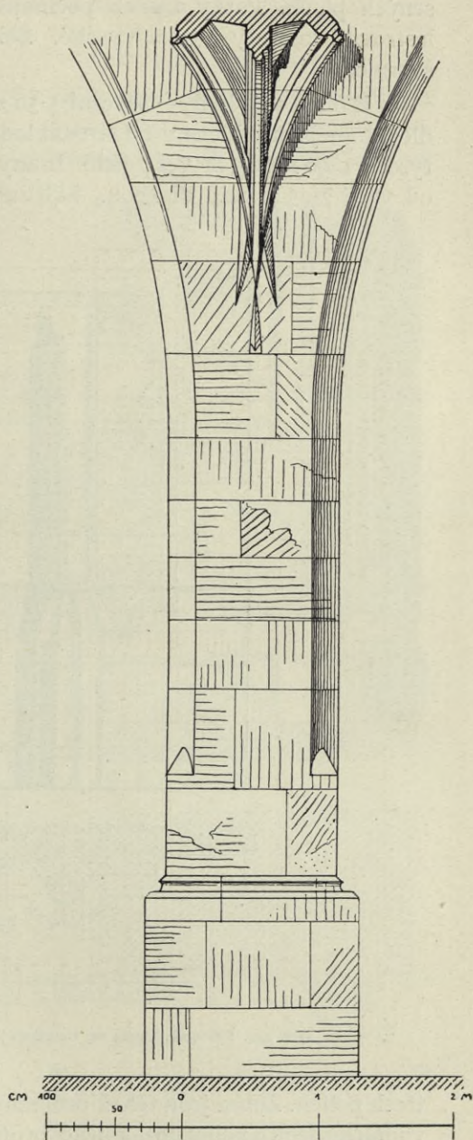
Obr. 143. Rakovník. Chrám sv. Bartoloměje. Patka klenby na pilíři mezi střední a jižní lodí.
