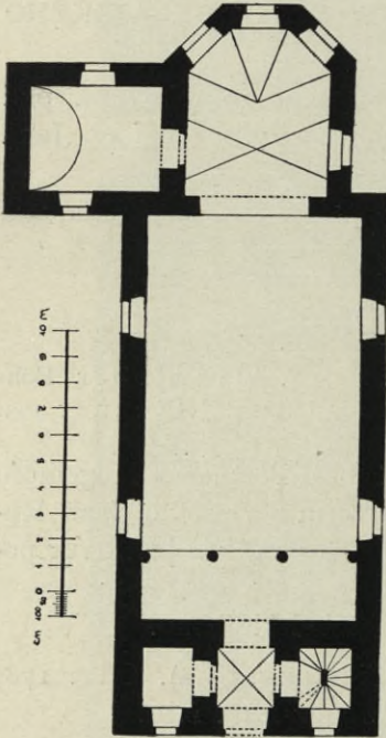
Obr. 69. Nezabudice. Púdorys far. kostela sv. Vavřince.
