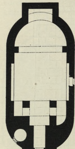
Obr. 37. Krupá. Půdorys filiálního kostela sv. Gotharda.
