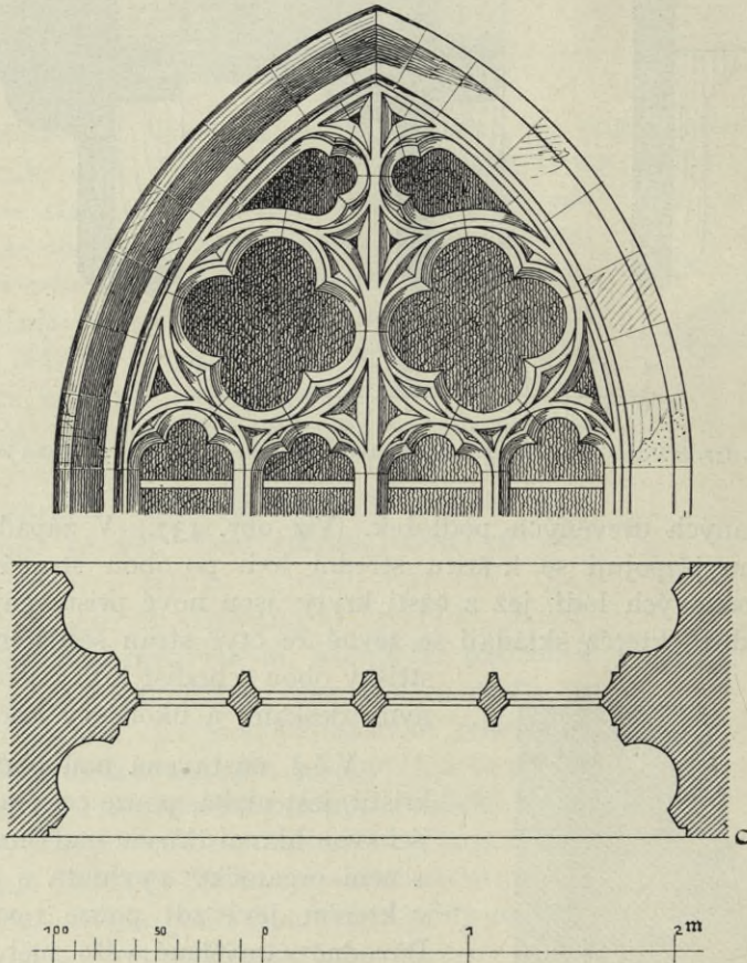
Obr. 139. Rakovník. Chrám sv. Bartoloměje. Pádrcys a kružba západního okna.
