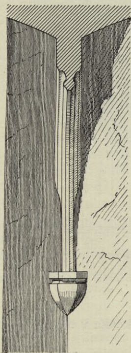
Obr. 31. Krakovec. Hrad. Náběhy kleneb v západ. křídle: ve sklepe z XIII. stol. (na pravo) a v přízemí z XV. stol. (na levo).
