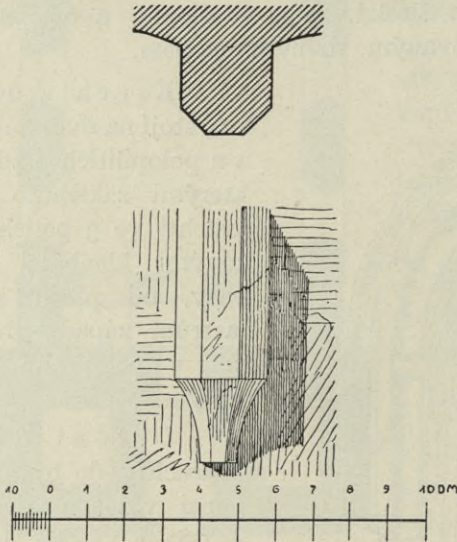
Obr. 287. Veliz. Far. kostel sv. Jana Křt. Průsek žebra a konsola pod klenbou presbytáře.
