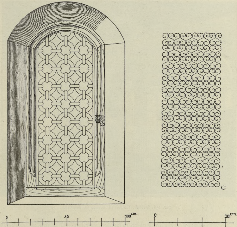
Obr. 257. Skřiváň. Fil. kostel sv. Štěpána. Okno a vzorec sítě před okny.
