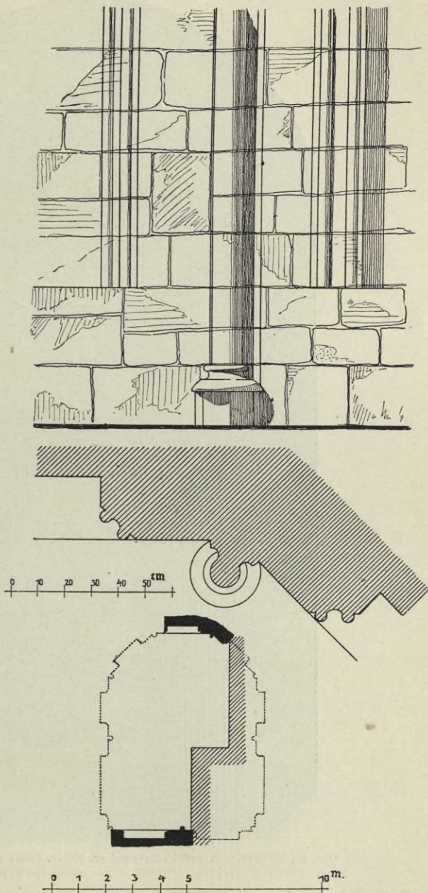
Obr. 74. Nižburk. Hrad. Zbytky původní kaple. Půdorys a detail ostění výklenků a koutové přípory.
