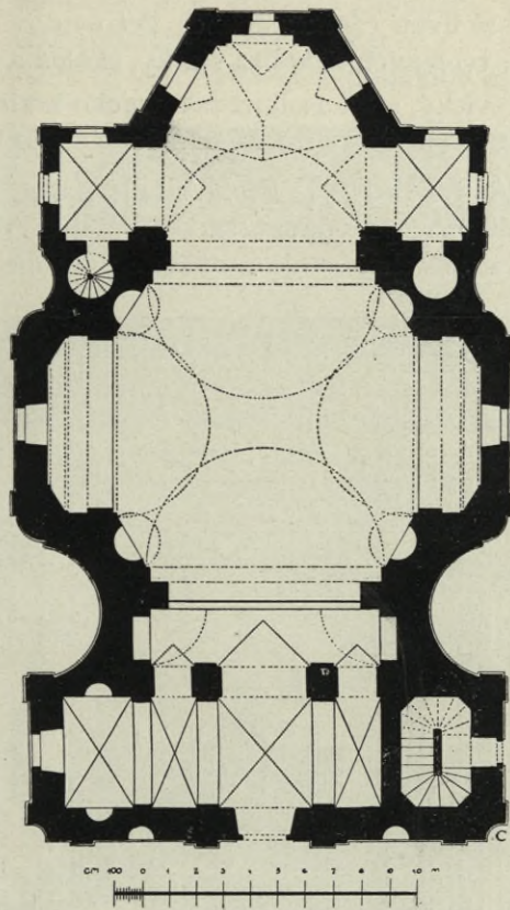
Obr. 108. Petrovice. Púdorys far. kostela Navšt. P. Marie.
