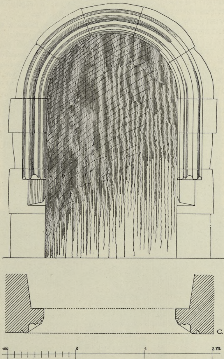
Obr. 236. Rousínov. Farní kostel P. Marie. Západní portálek. Pohled a půdorys.
