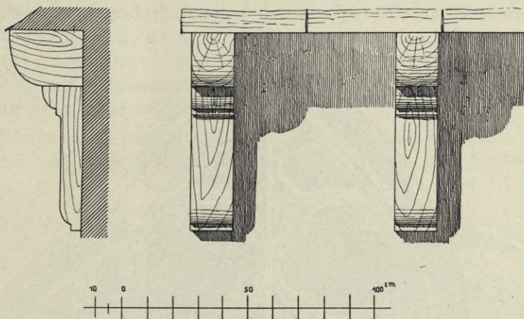
Obr. 137. Rakovník. Chrám sv. Bartoloměje. Dřevěné konsoly hlavní římsy na střední lodi.
