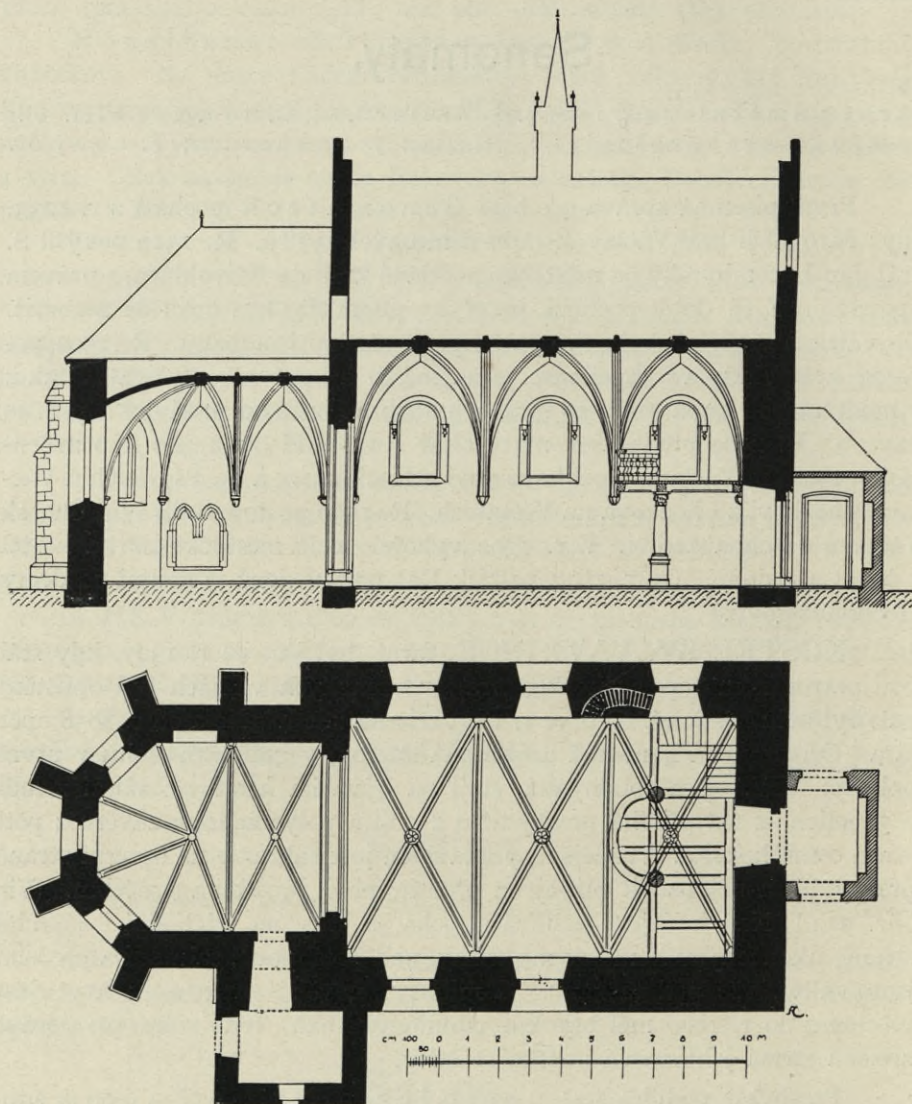
Obr. 242. Senomaty. Půdorys a podél. řez. far. kostela sv. Vavřince.
