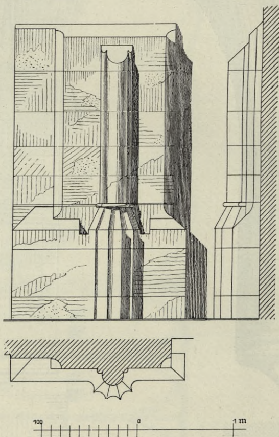
Obr. 144. Rakovník. Chrám sv. Bartoloměje. Zbytky přípory v severní boční lodi.
