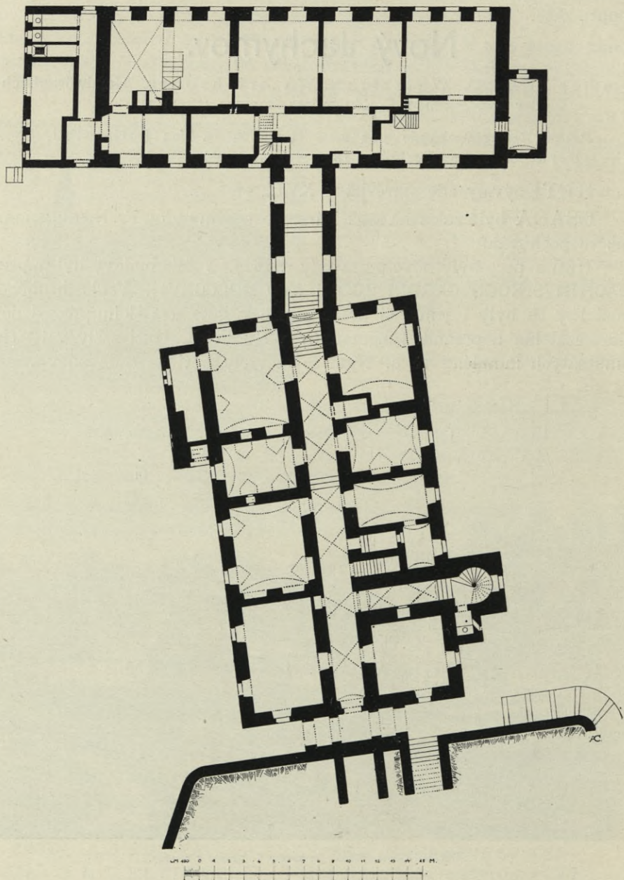
Obr. 83. Obora. (Leontinský zámek.) Půdorys přízemí.
