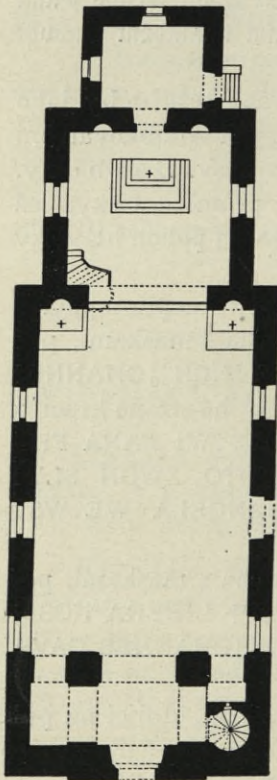
Obr. 63. Mutějovice. Půdorys farního kostela sv. Václava.
