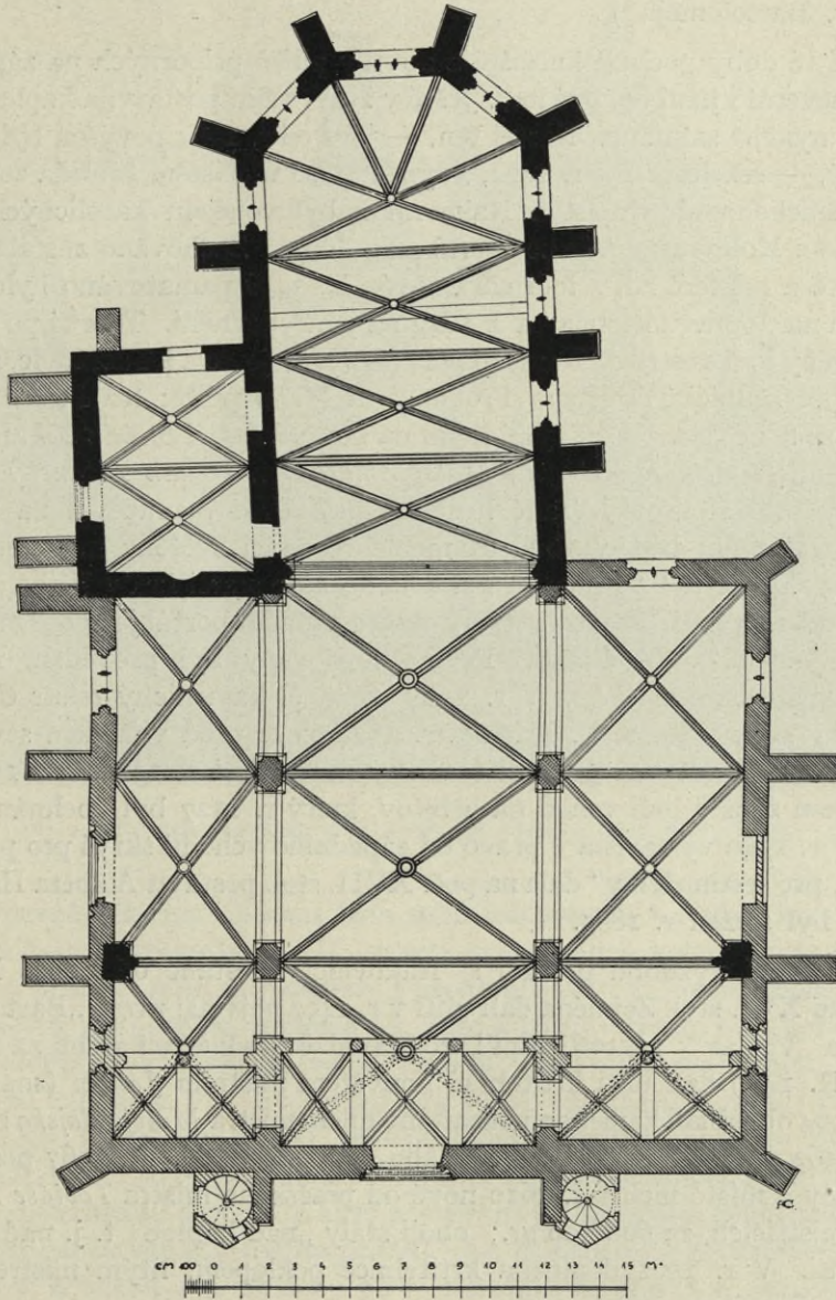
Obr. 134. Rakovník. Děkanský chrám sv. Bartoloměje. Půdorys: (černé zdivo starší než z konce XV. století, hustě čárkované zdivo z meze XV. a XVI. století, řídko čárkované zdivo z konce XIX. století).
