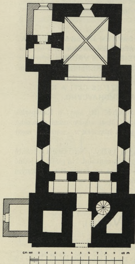
Obr. 284. Veliz. Půdorys far. kostela sv. Jana Křt.
