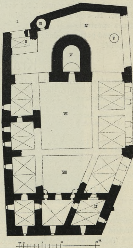
Obr. 28. Krakovec, Hrad. Půdorys.
