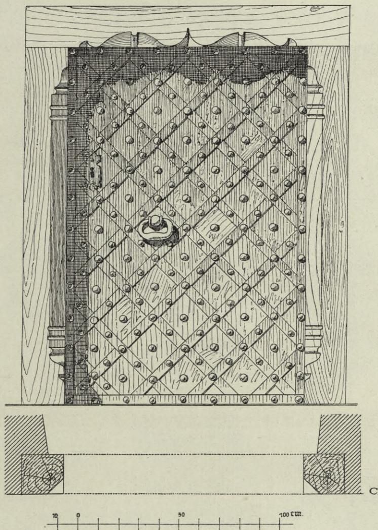
Obr. 259. Skřívaň. Fil. kostel sv. Štěpána. Dveře z kněžiště do sakristie.
