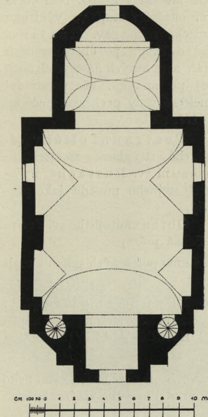
Obr. 80. Nový dům. Půdorys. fil. kostela sv. Maří Magdaleny.
