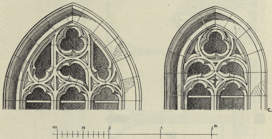
Obr. 140. Rakovník. Chrám sv. Bartoloměje. Dvě kružby oken bokových lodí.
