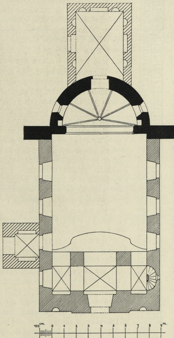
Obr. 280. Újezd Velký. Půdorys far. kostela Nanebevzetí P. Marie.
