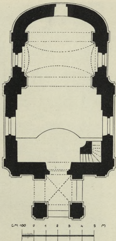
Obr. 250. Senomaty: Půdorys hřbitovního kostela sv. Štěpána.
