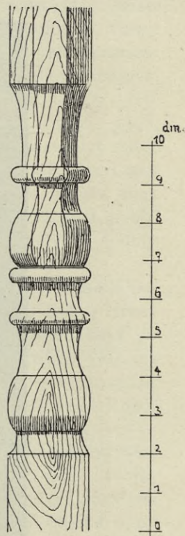
Obr. 191. Rakovník. Zvonice u kostela Nejsv. Trojice. Jeden ze šesti sloupků lucerny.
