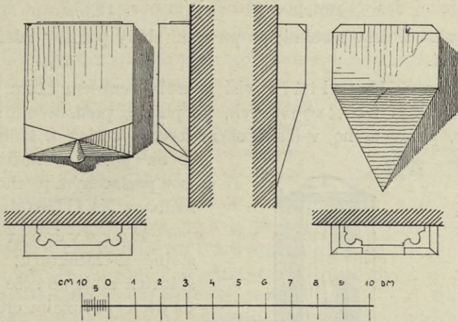
Obr. 182. Rakovník. Kostel sv. Jiljí. Konsoly pod klenbami v lodi.
