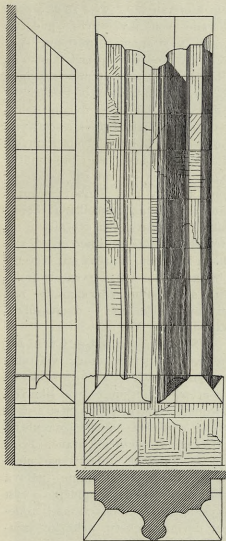
Obr. 145. Rakovník. Chrám sv. Bartoloměje. Zbytek patkový v jižní boční lodi.
