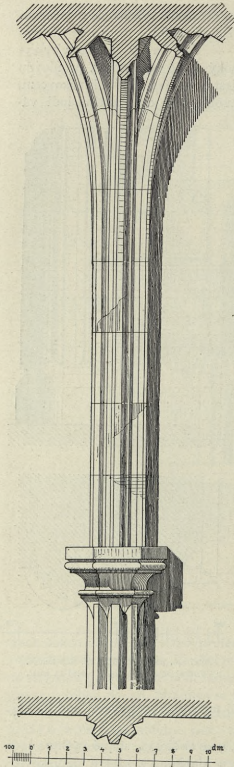
Obr. 147. Rakovník. Chrám sv. Bartoloměje. Přípora a patka klenby v kněžišti.
