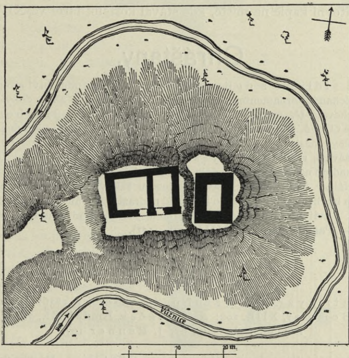
Obr. 14. Jenčov. Hrad. Situace a průřez.
