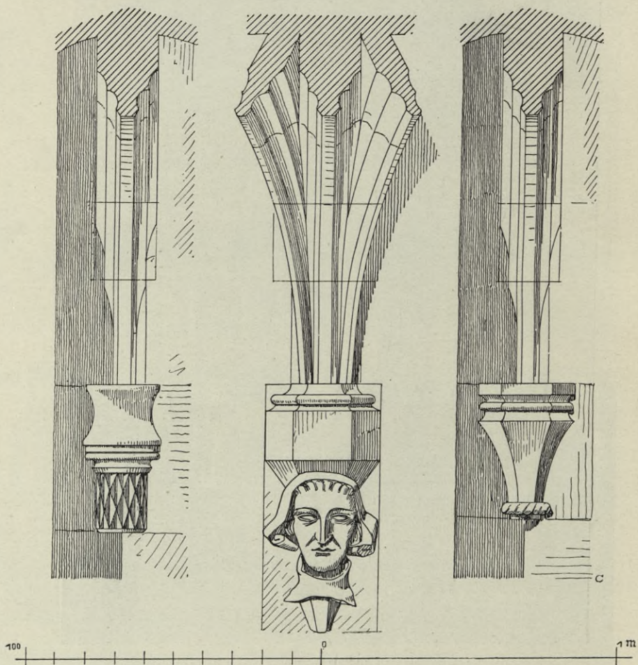
Obr. 47. Křivoklát. Farní kostel sv. Petra, Patky kleneb v presbytáři s konsolkami.
