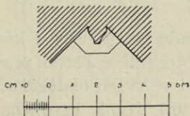
Obr. 32. Krakovec. Hrad. Patka klenby a konsolka v jihovýchodním křídle (ze XIV. st.)
