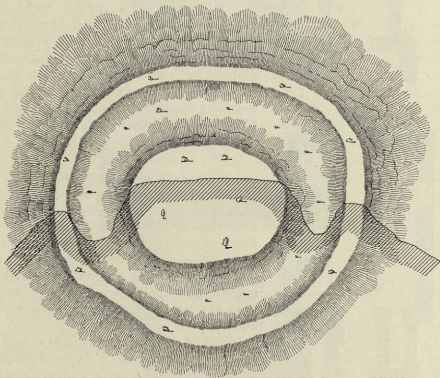
Obr. 272. Šanov. Situace a řez tvrziště.
