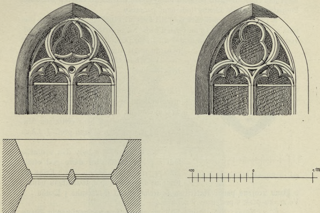
Obr. 187. Rakovník, Hřbitovní kostel Nejsv. Trojice. Půdorys oken a kružby.
