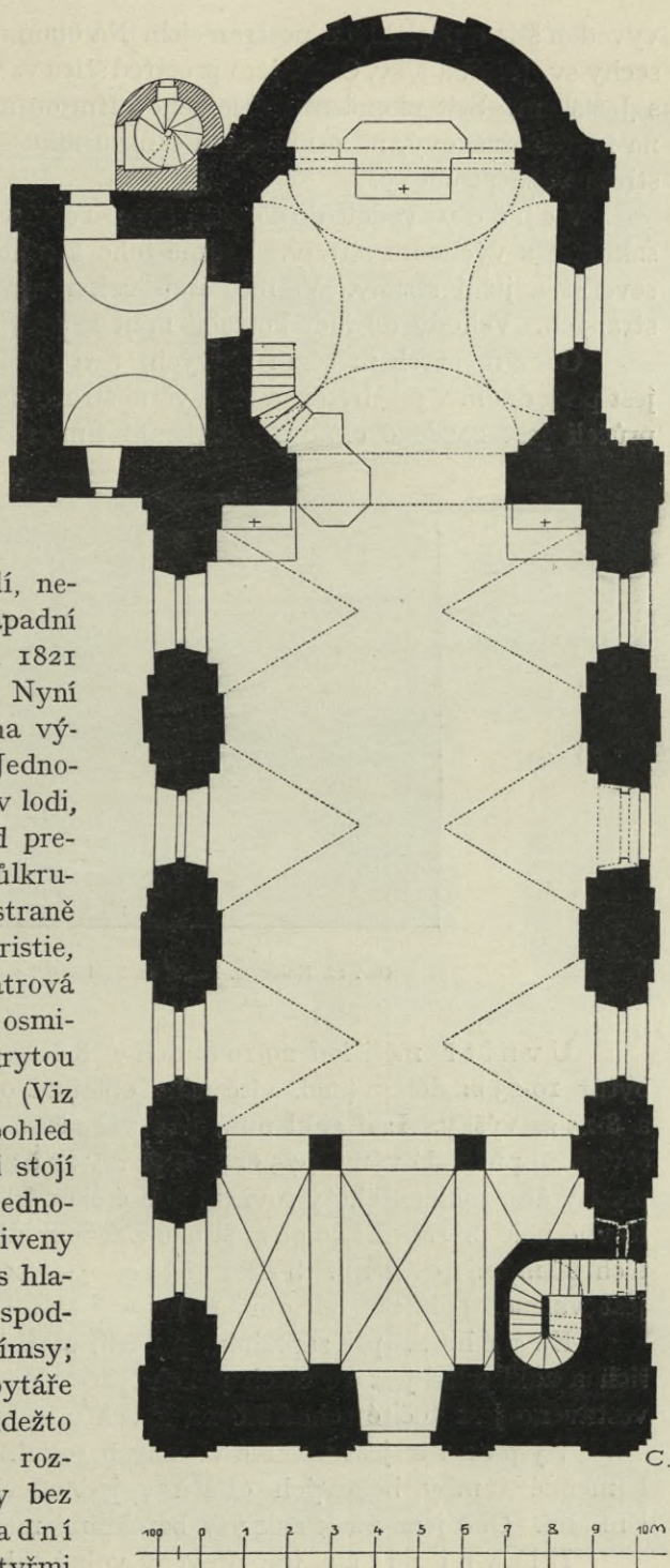
Obr. 15. Kněžves. Půdorys farního kostela sv. Jakuba.
