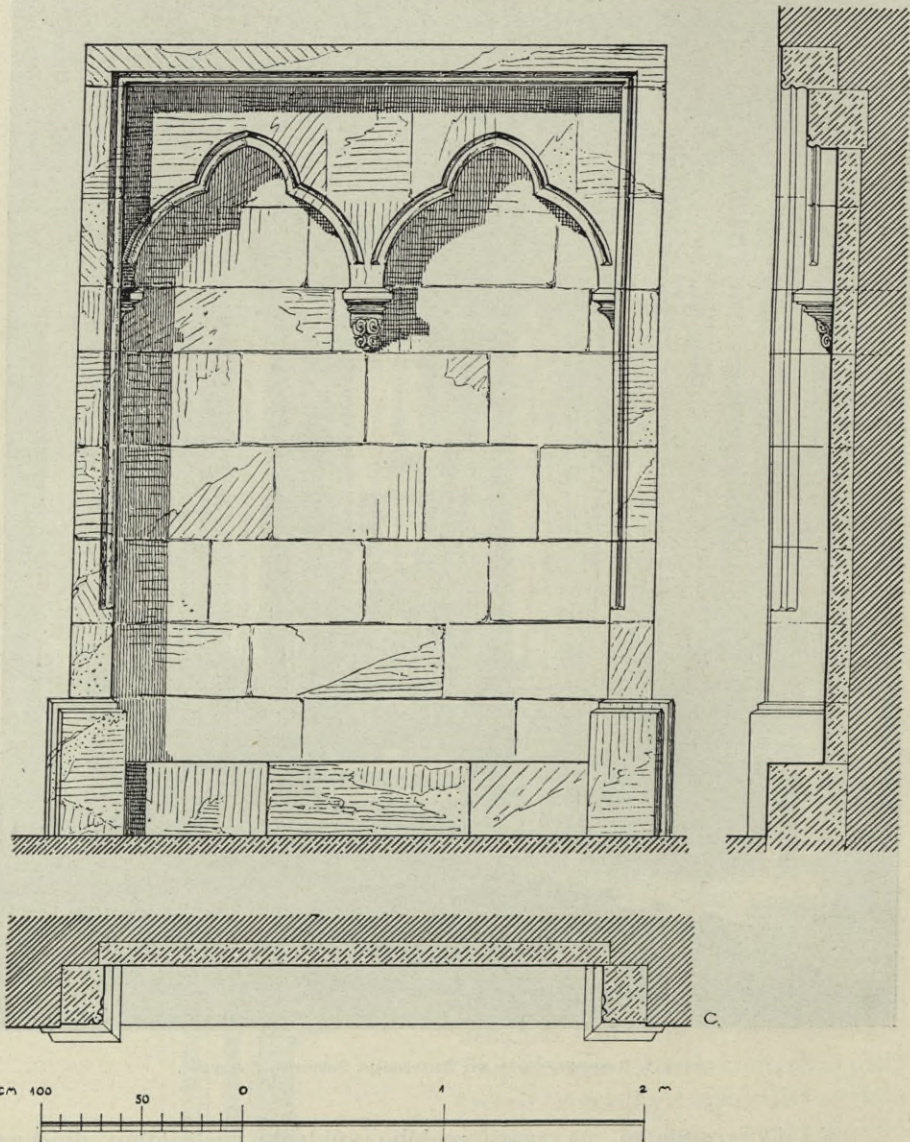
Obr. 149. Rakovnik. Chrám sv. Bartoloměje. Sedille v kněžišti. Pádorys, řez a pohled.
