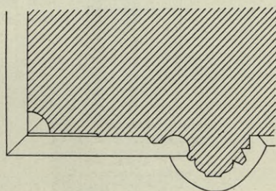
Obr. 146. Rakovník. Chrám sv. Bartoloměje. Vítězný oblouk; půdorys a pohled na trnož.
