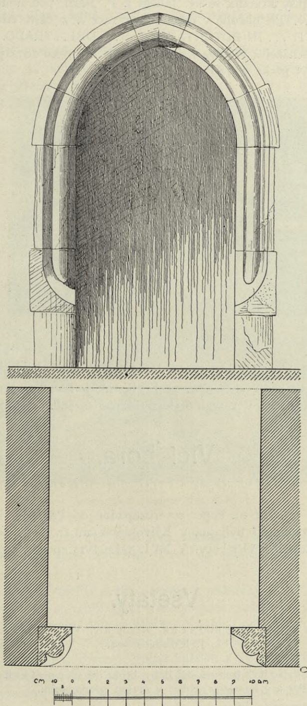
Obr. 289. Velíz. Far. kostel sv. Jana Křt. Ostění vchodu z kruchty do věže.
