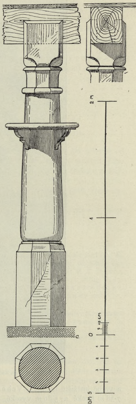
Obr. 25. Kněževse. Kamenný sloup v staré hospodě č. 102.
