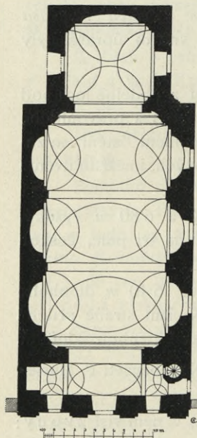
Obr. 126. Kukleny. Půdorys kostela sv. Anny.
