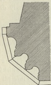
Obr. 23. Hradec Králové. Chrám sv. Ducha: Průsek ostění vchodu jihozápadního.
