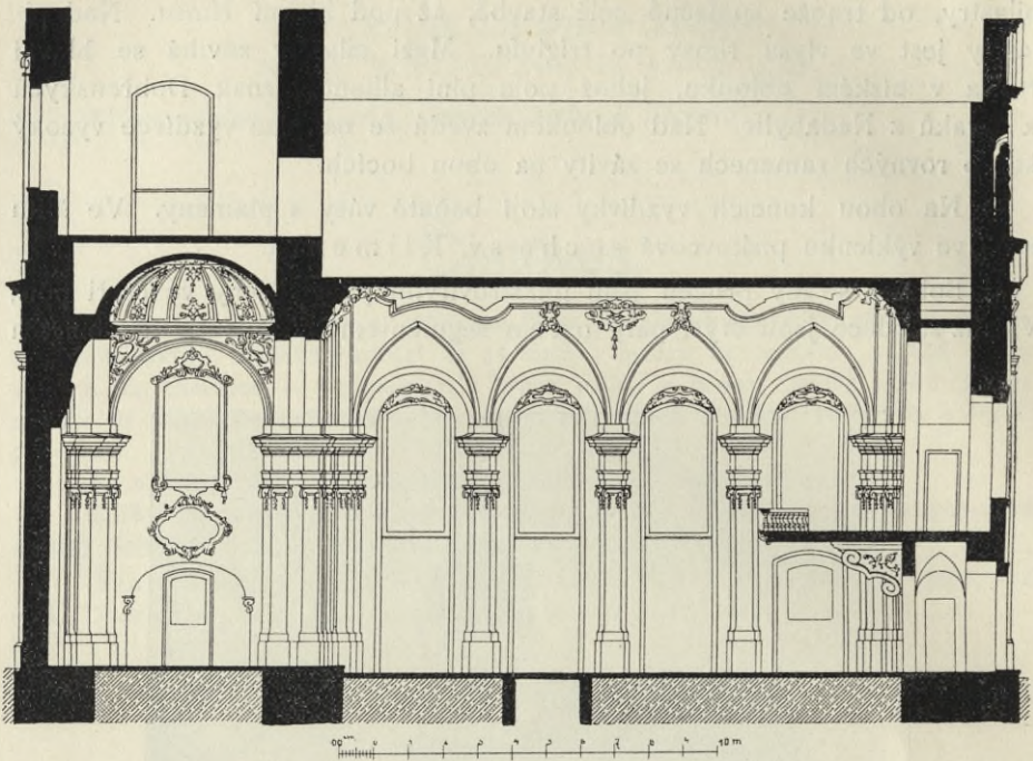
Obr. 8. Dobřenice. Podélný řez kostela sv. Klimenta.
