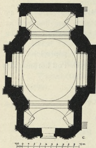
Obr. 63. Hradec Králové. Půdorys kostela sv. Jana Nep.
