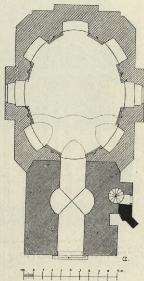
Obr. 52. Hradec Králové. Púdorys Bílé věže s kaplí sv. Klimenta.
