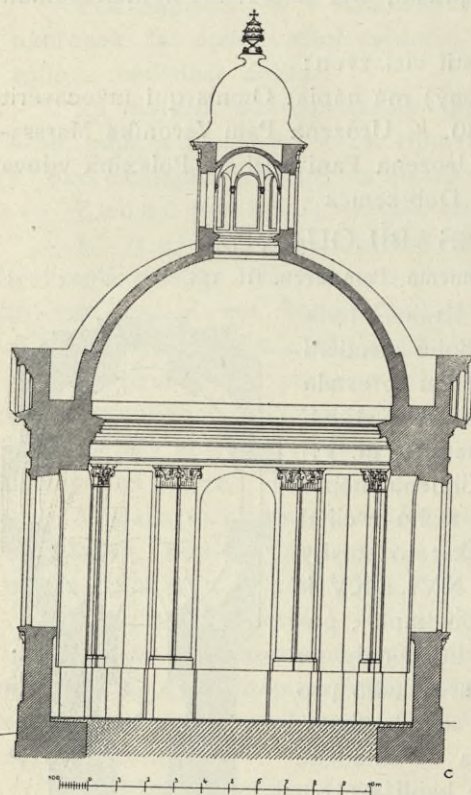
Obr. 53. Hradec Králové. Příčný řez kapli sv. Klimenta.
