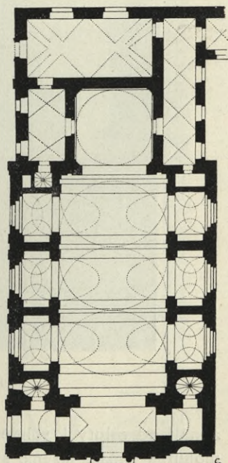
Obr. 56. Hradec Králové. Půdorys kostela P. Marie.
