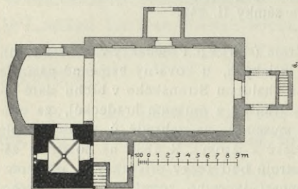
Obr. 138. Lochenice. Půdorys kostela.
