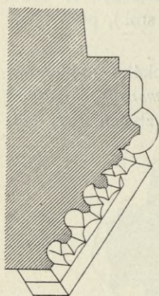
Obr. 25. Hradec Králové. Chrám sv. Ducha: Průsek ostění vchodu v král. předsíně do presbytáře.
