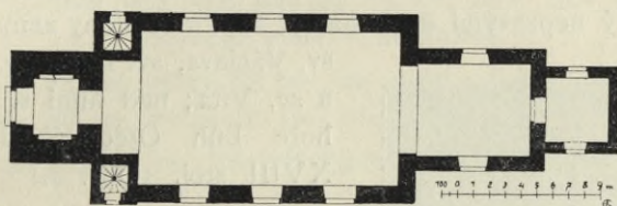
Obr. 1. Černilov. Půdorys kostela sv. Štěpána.
