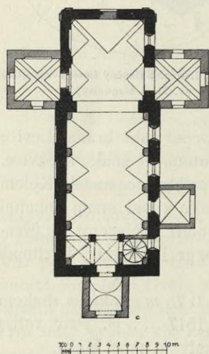
Obr. 132. Libčany. Půdorys kostela.
