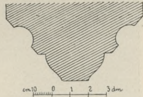
Obr. 157. Milevsko. Chrám sv. Jiljí. Profil vítězného oblouku.
