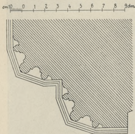
Obr. 92. Hodušín. Profil západního vchodu.
