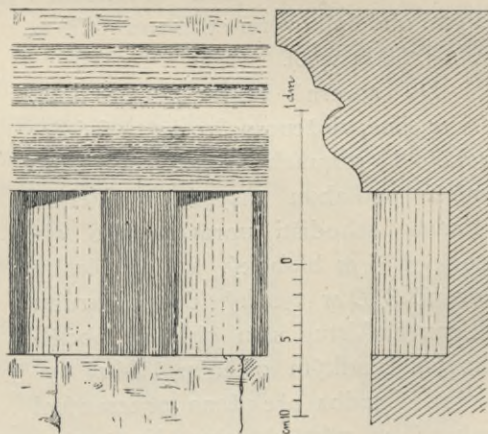
Obr. 154. Milevsko. Kostel sv. Jiljí. Zubořez s řimsou podstřešní.
