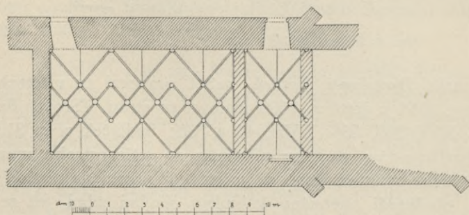
Obr. 43. Bechyně. Půdorys bývalého kostela v zámku.
