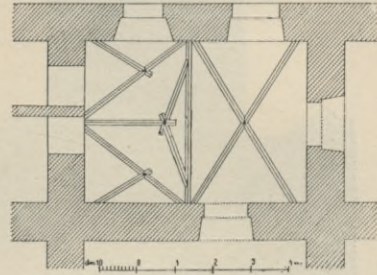
Obr. 186. Vlksice. Půdorys klenuté síně ve tvrzi.
