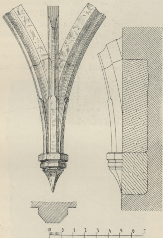
Obr. 45. Bechyně. Žebra v bývalém kostele zámeckém.
