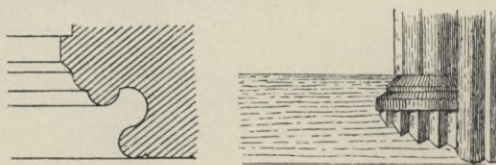
Obr. 143. a 144. Milevsko. Kaple opatská. Profil pažení okna a dolejší část orámování okna.
