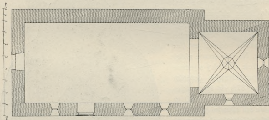
Obr. 86. Dobronice. Půdorys kostela.
