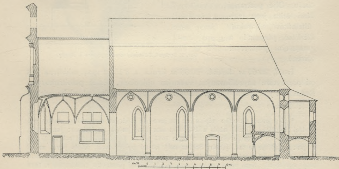
Obr. 7. Bechyně. Děkanský kostel: řez podélný.
