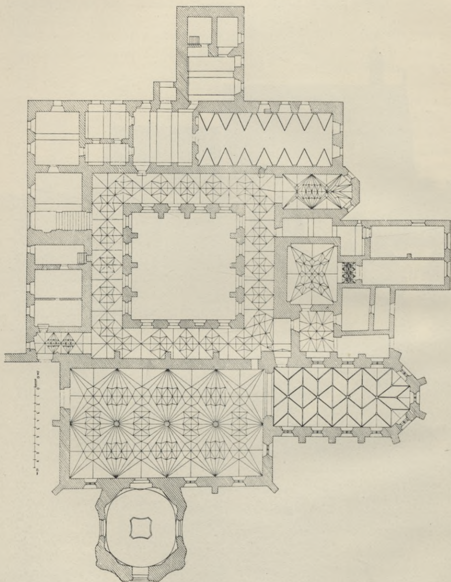
Obr. 18. Bechyň. Půdorys kláštera.
