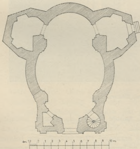
Obr. 73. Bechyň. Půdorys hřbitovního kostela.
