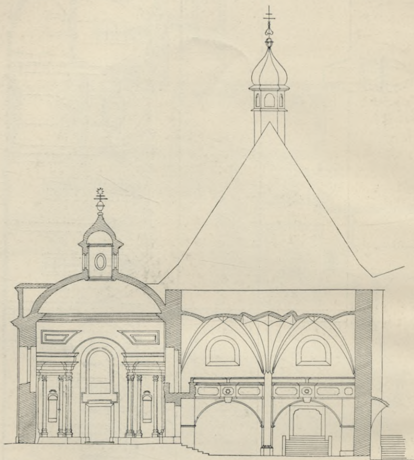
Obr. 20. Bechyně. Klášterní kostel: řez příčný.
