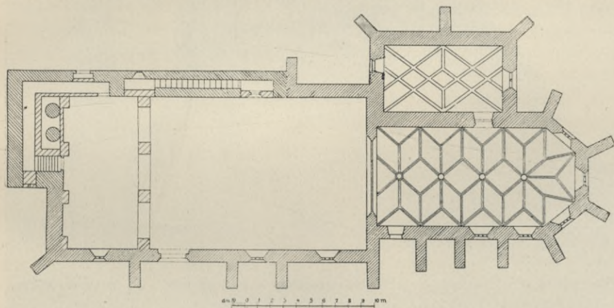
Obr. 146. Milevsko. Chrám sv. Jiljí. Půdorys.
