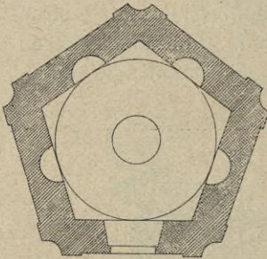
Kouřim: Půdorys kaple P. Marie.
