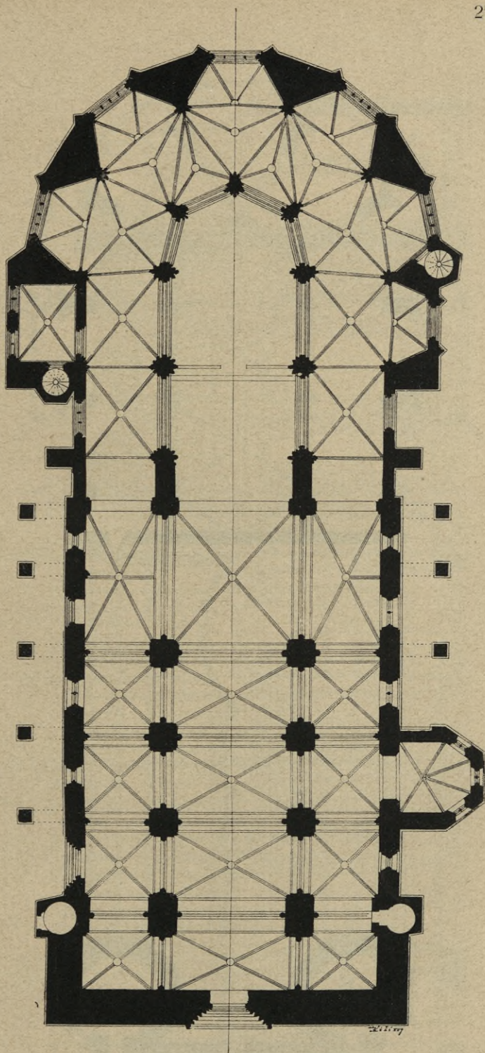
Kolín: Půdorys kostela sv. Bartoloměje.
