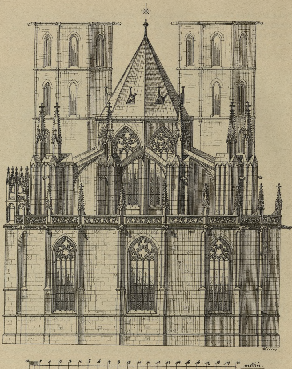
Kolín: Chor kostela sv. Bartoloměje (Rest. J. Mockera).
