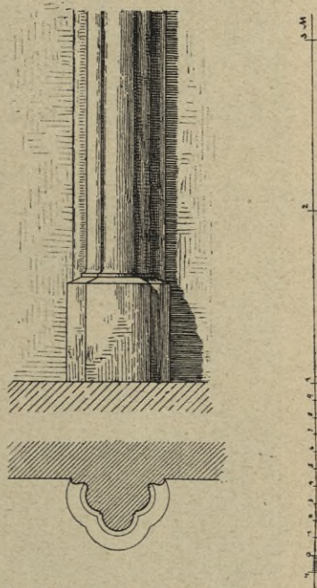
Kolín: Přípora kostela sv. Bartoloměje, stará část.
