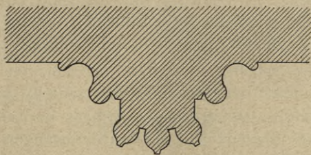
Skalice: Profil přípony.
