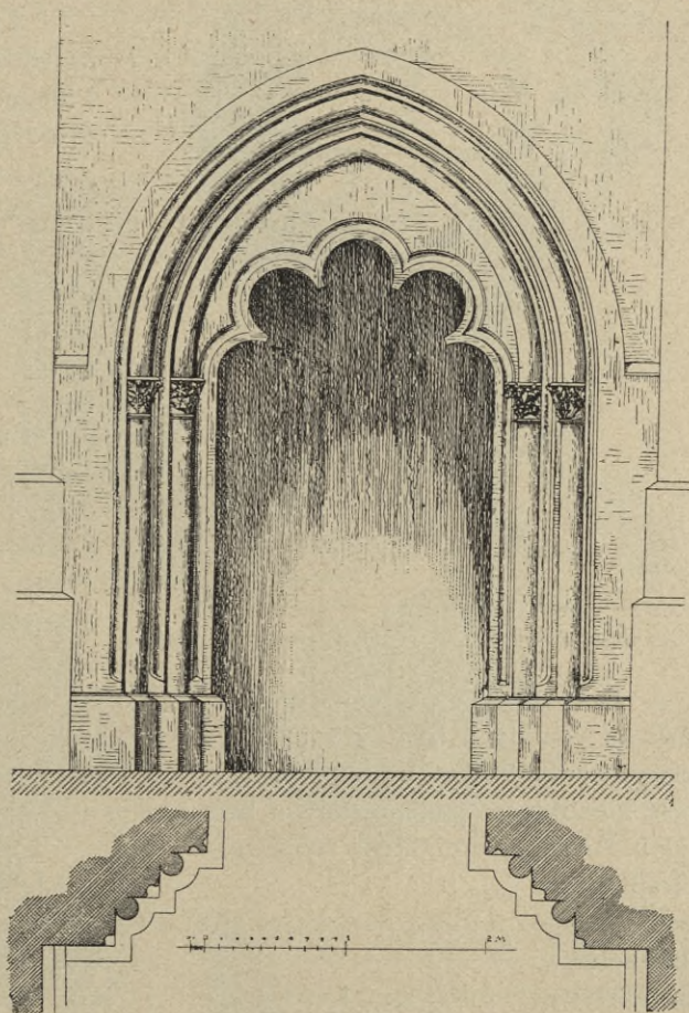
Kouřim: Severní portal kostela sv. Štěpána.
