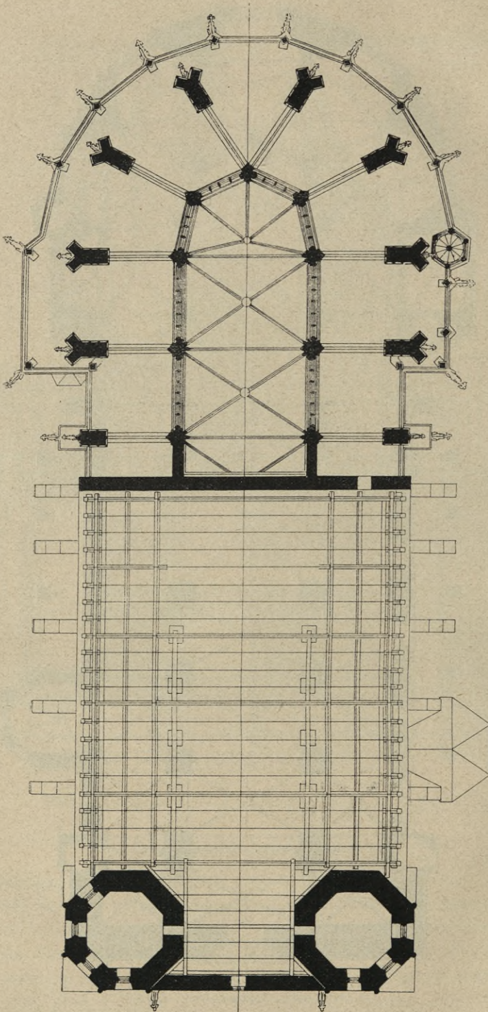
Kolín: Půdorys chrámu sv. Bartoloměje. — První patro.
