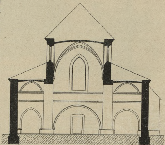
Kouřim: Příčný řez kostela sv. Štěpána.
