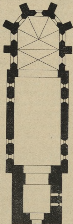
Plaňany: Púdorys kostela.
