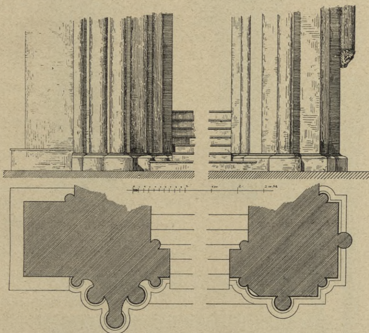
Kouřim: Nárožní pilíře triumfálního oblouku kostela sv. Štěpána.
