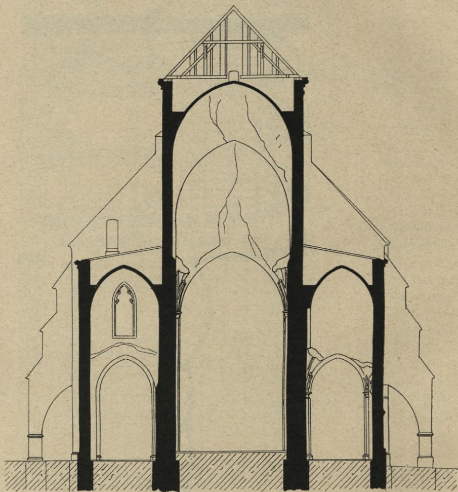
Kolín: Kostel sv. Bartoloměje. — Příčný řez nové části proti staré.
