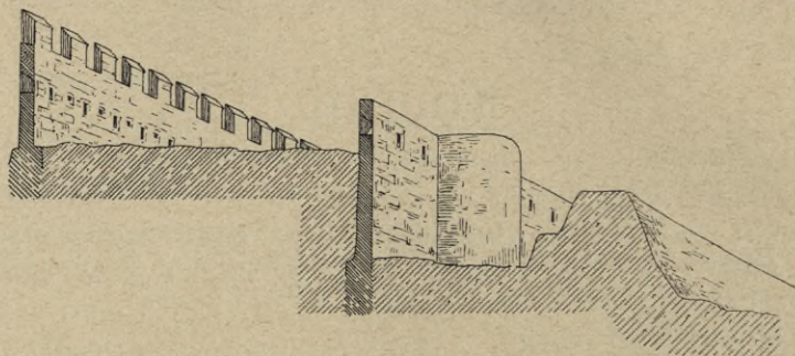
Kouřim: System městských hradeb.
