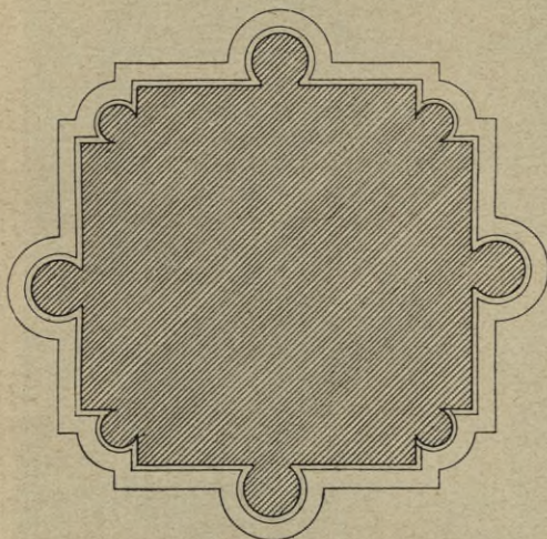
Kolín: Pilíř lodní kostela sv. Bartoloměje, stará část.
