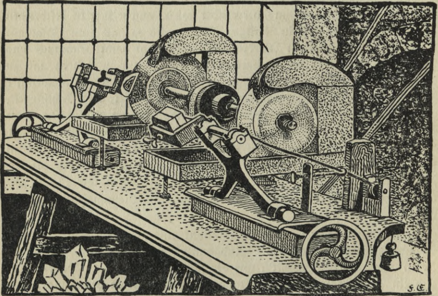
Abb. 60 Steinsäge.
