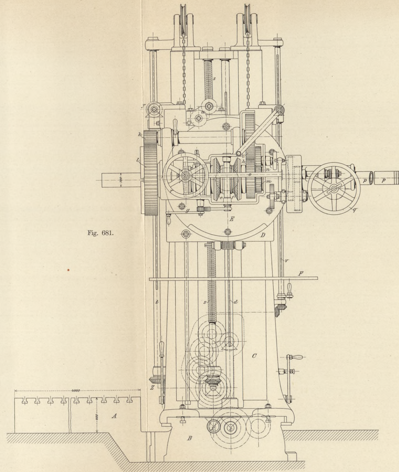
Liegende Bohrmaschine von Ernst Schiess in Düsseldorf. 1/25 wahrer Grösse.
