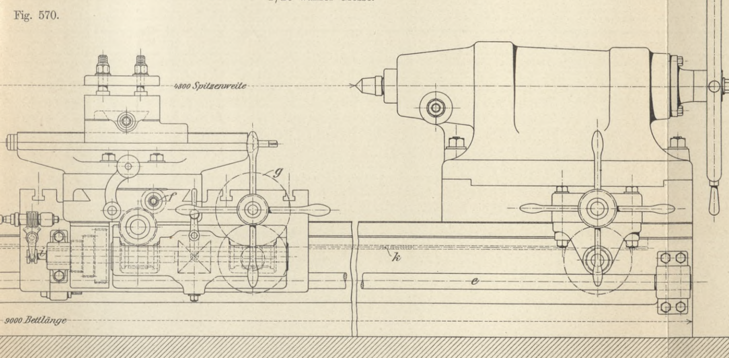
Fig. 570 u. 571: Plan- und Spitzendrehbank von Ernst Schiess in Düsseldorf. 1/20 wahrer Grösse.
