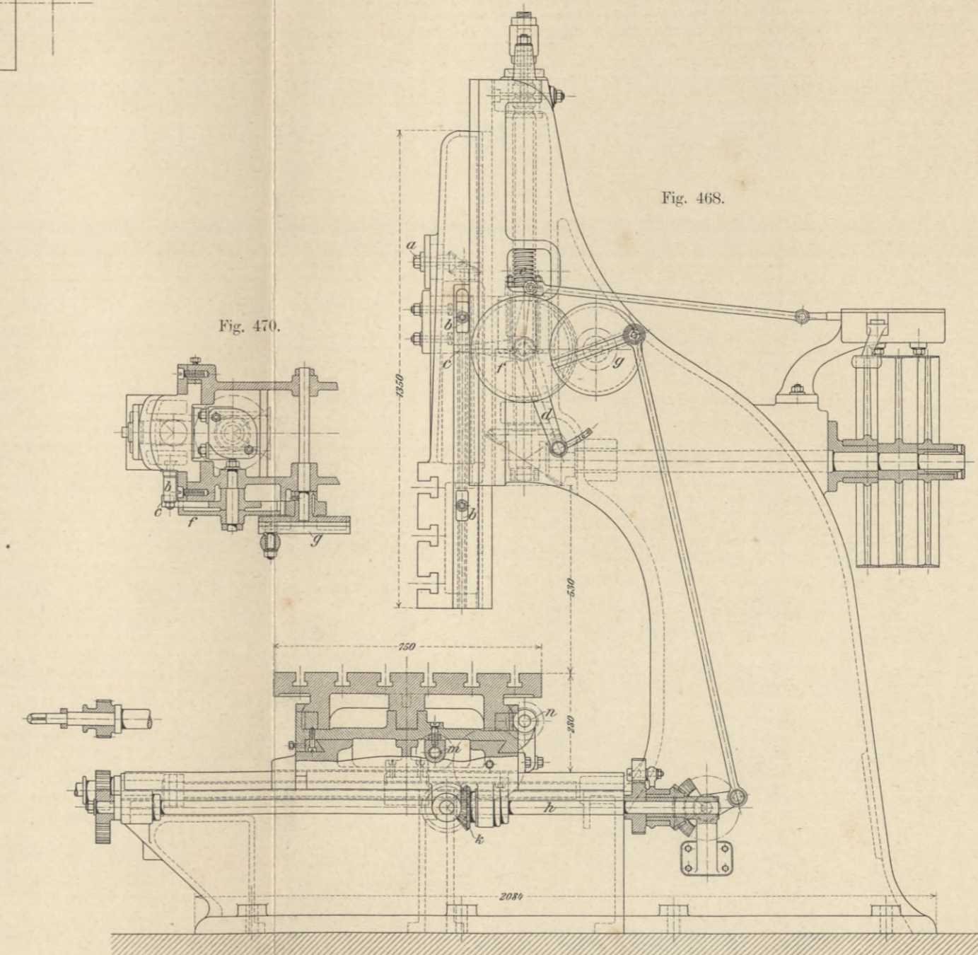
Fig. 468 bis 470. Stossmaschine von Droop & Rein in Bielefeld. 1/15 wahrer Grösse.
