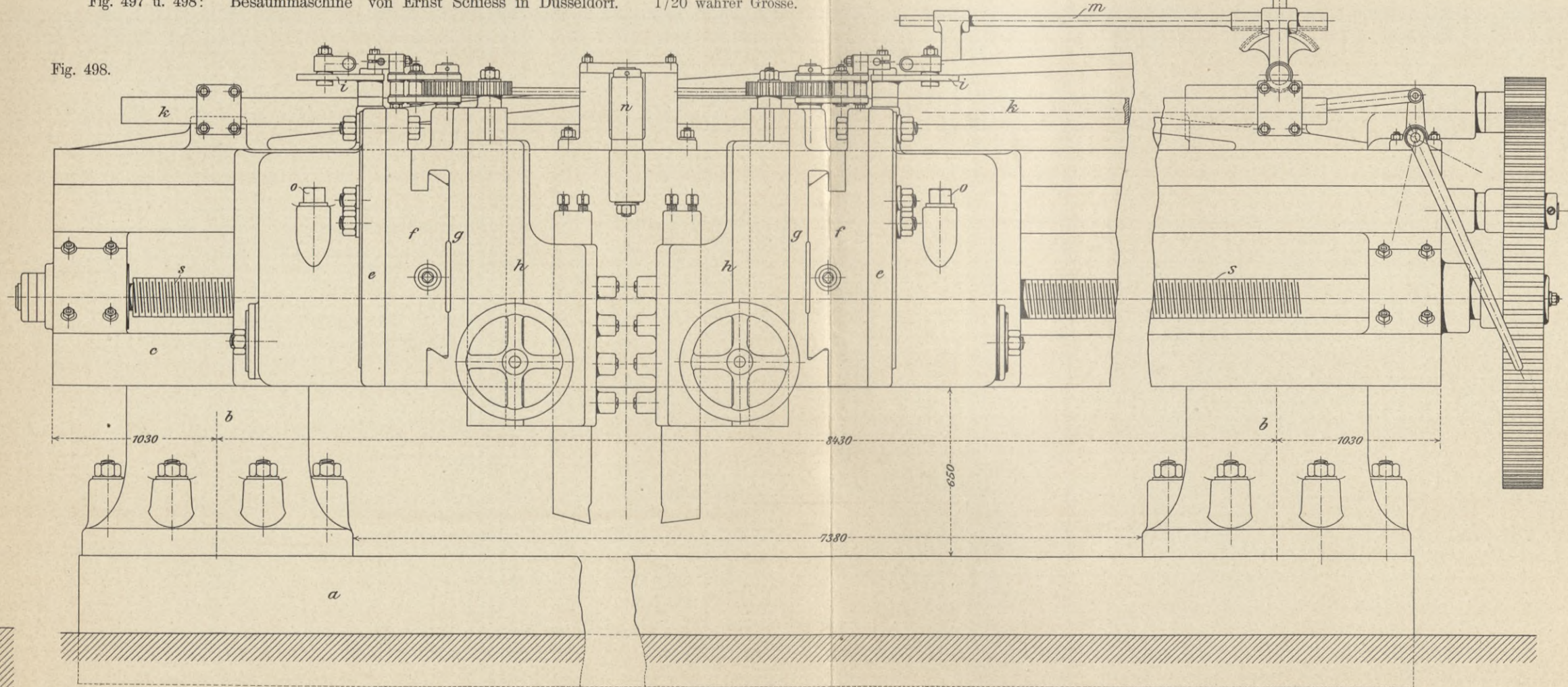
Fig. 497 u. 498: Besäummaschine von Ernst Schiess in Düsseldorf. 1/20 wahrer Grösse.
