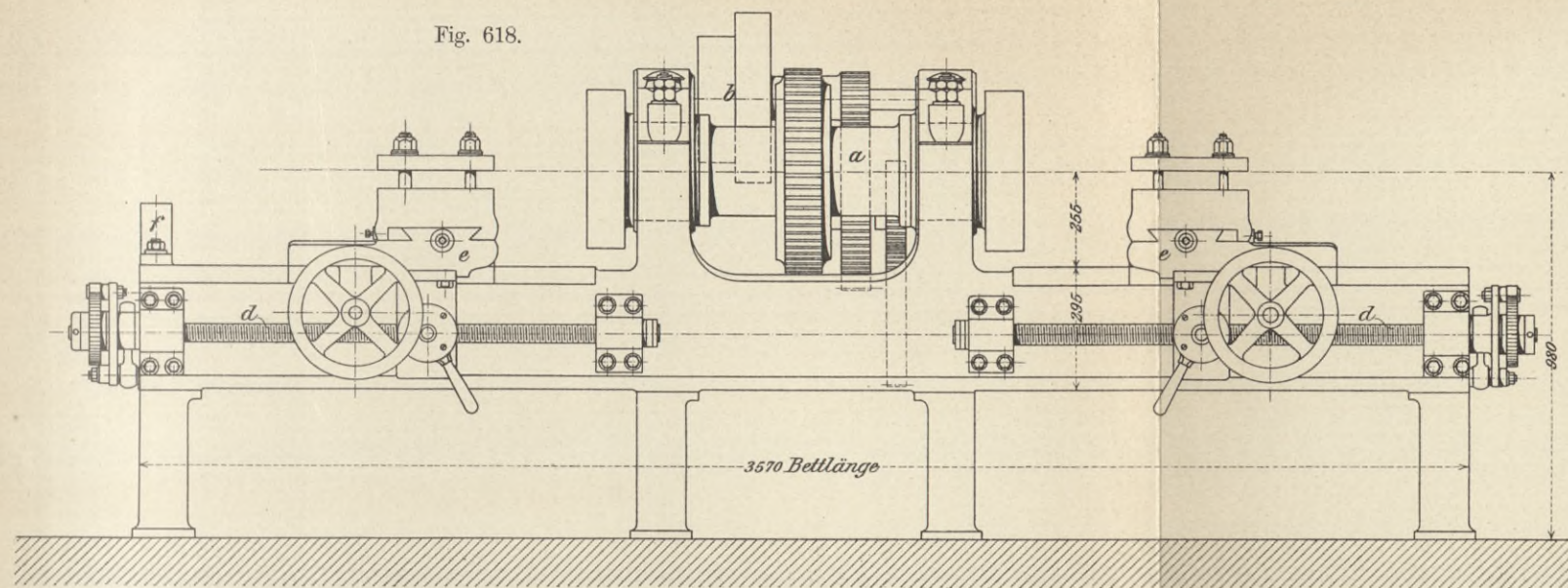
Fig. 618 u. 619: Achshalsdrehbank von Ernst Schiess in Düsseldorf. 1/20 wahrer Grösse.
