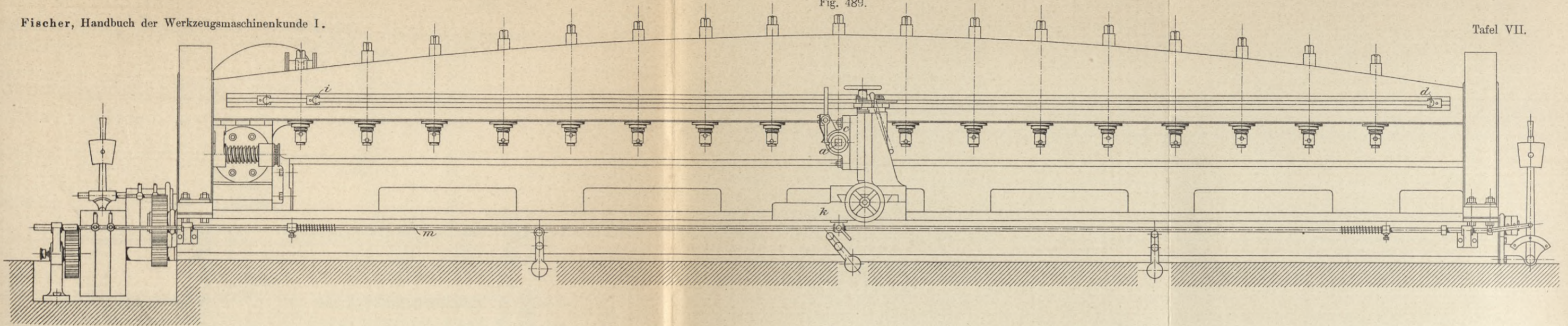
Blechkantenhobelmaschine von L. W. Breuer, Schumacher & Co. in Kalk bei Köln.
