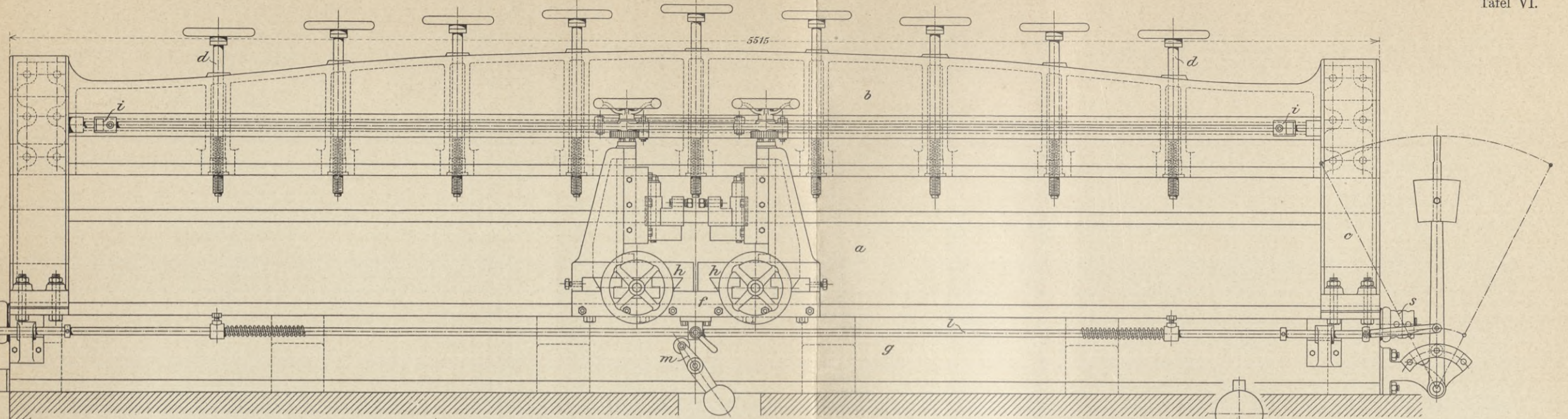
Fig. 497 u. 498: Besäummaschine von Ernst Schiess in Düsseldorf. 1/20 wahrer Grösse.
