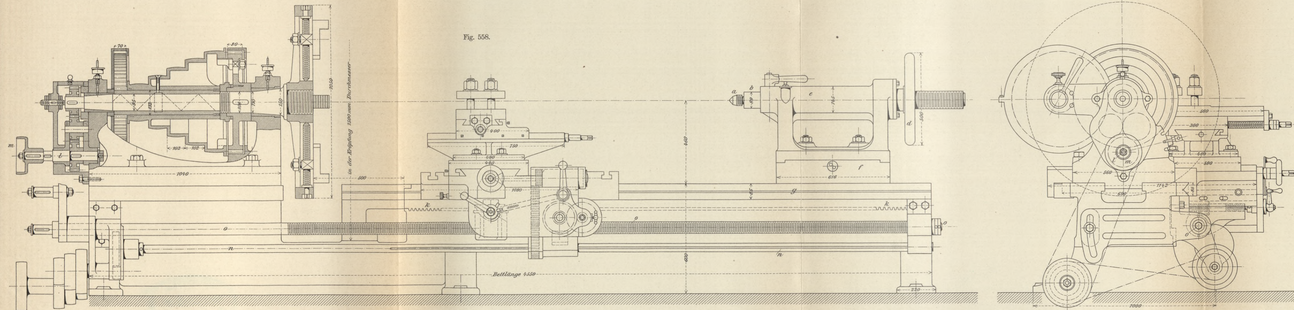
Spitzendrehbank von H. Wohlenberg in Hannover. 2/25 wahrer Grösse.
