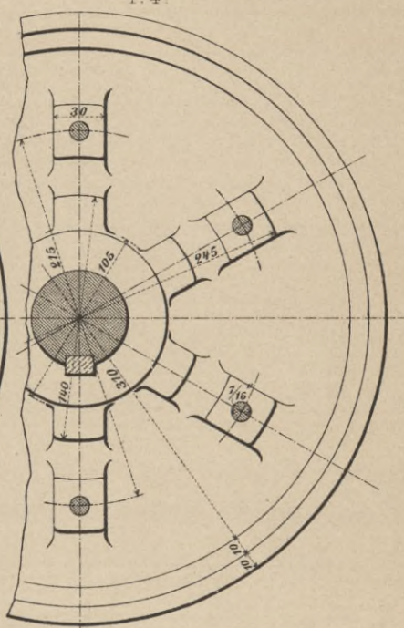
Kupplungshälfte für die Zahnscheibe.
