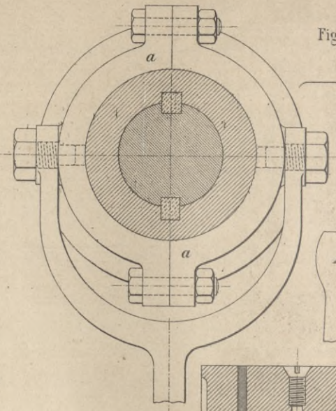
Schnitt: a b.
