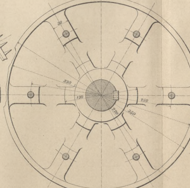
Kupplungshälfte für die Bürstenscheibe.
