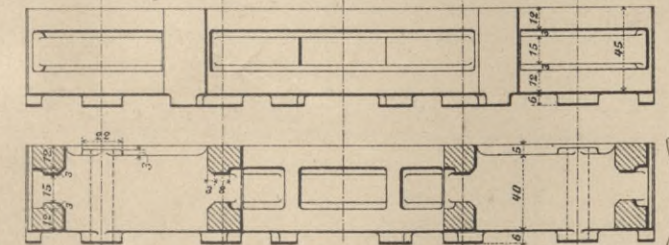
Rückansicht der Bürstenscheibe.
