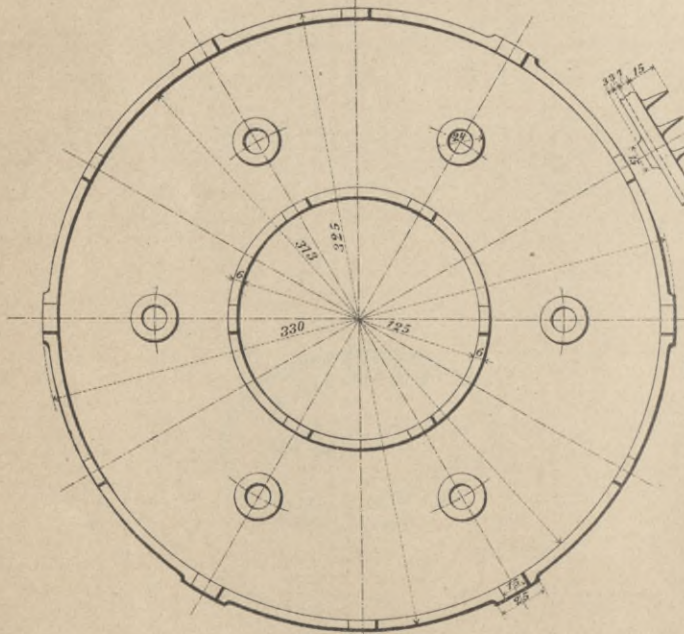
Rückansicht der Zahnscheibe.
