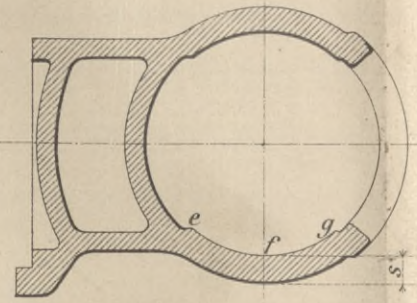
Schnitt: c d (Fig. 309, 311).
