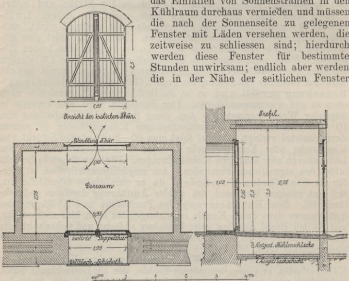
Fig. 119—121. Eingang zu einer Fleischkühlhalle.
