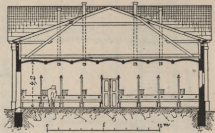
Fig. 196 u. 197. Musterplan für landw. Bauten in Niederösterreich. Bl. X.
