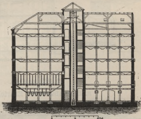
Fig. 47. Körner-Magazin System Opitz.
