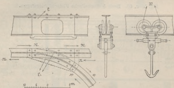
Fig. 61. Verbesserte Beck & Henkel'sche Fördervorrichtung.
