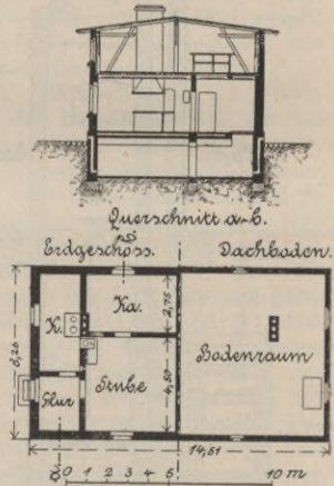
Fig. 5—8. Zweifamilienhaus der Regierung zu Stralsund.
