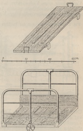
Fig. 4 u. 5. Entladebrücken.
