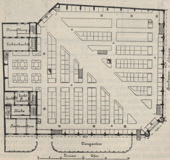
Fig. 32. Markthalle VII. zu Berlin (Dresdenerstrasse).
