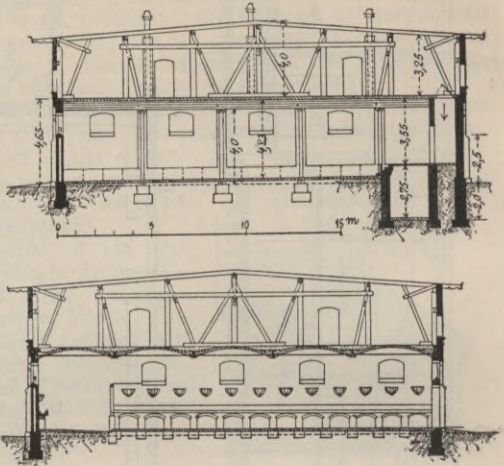
Stallgebäude zu Murkwitz, Prov. Posen. Arch. A. Schubert.
