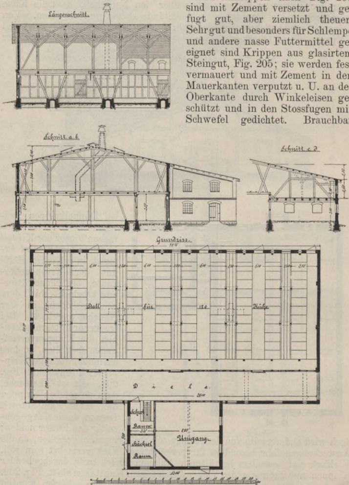
Fig. 223—226. Viehhaus zu Suckwitz. Arch. Wagner.
