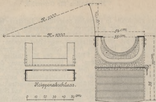
Fig. 20. Grossvieh- krippen.
