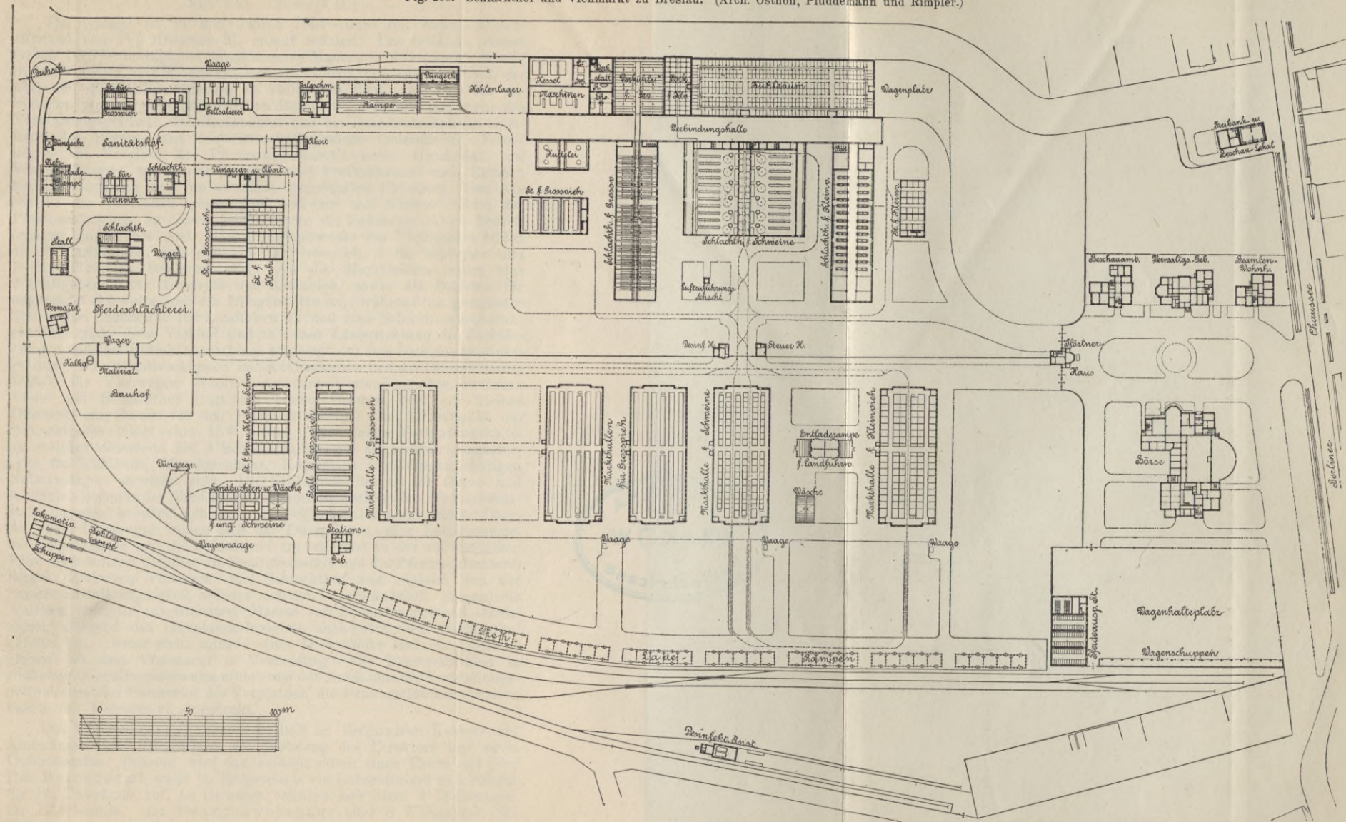
Fig. 200. Schlachthof und Viehmarkt zu Breslau. (Arch. Osthoff, Plüddemann und Rimpler.)
