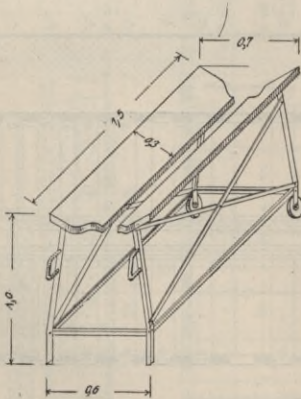
Fig. 74. Schlachtschragen für Kleinvieh.
