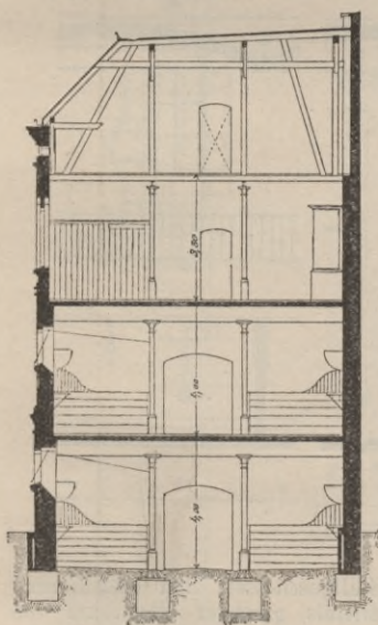
Fig. 55. Schnitt durch Stall VII.
