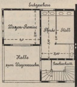
Fig. 21 u. 22. Stall für ein Landhaus. (Arch. B. Ebhardt.)
