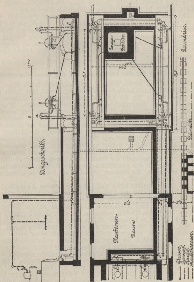
Fig. 36. Maschinelle Einrichtung einer Desinfektionsanstalt für Viehmarktsgeisse.
