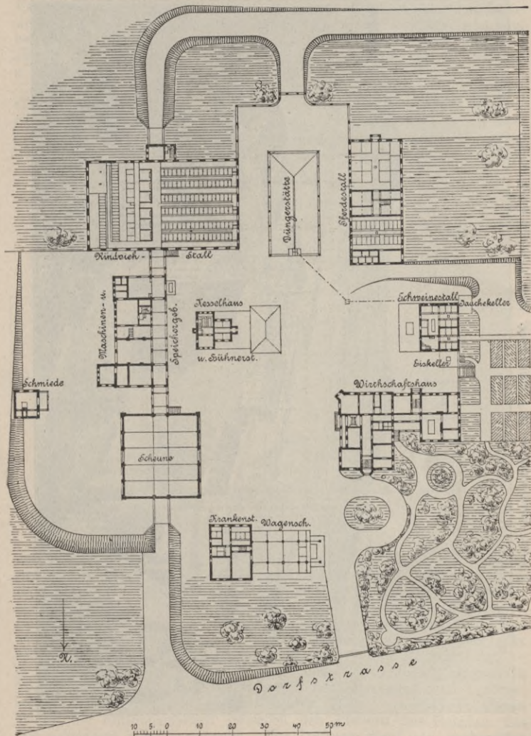
Fig. 42. Wirtschaftshof zu Landonvillers. Deutsche Bauzeitung 1892, No. 47. Arch. Reimer & Körte, Berlin.
