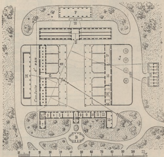
Fig. 37. Ferme nationale de Vincennes bei Paris.
