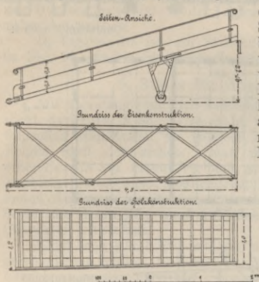
Fig. 6. Fahrbare Entladerampe.
