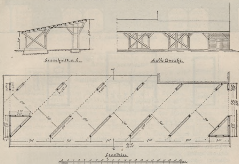
Fig. 338—340. Wagenschauer für Haegerfelde. Arch. Wagner.
