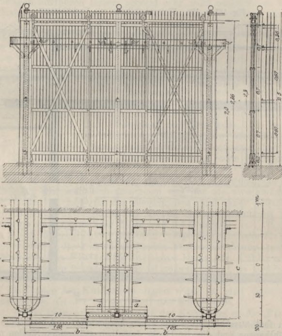
Fig. 127 u. 128. Zellenkonstruktion einer Fleischkühlhalle.
