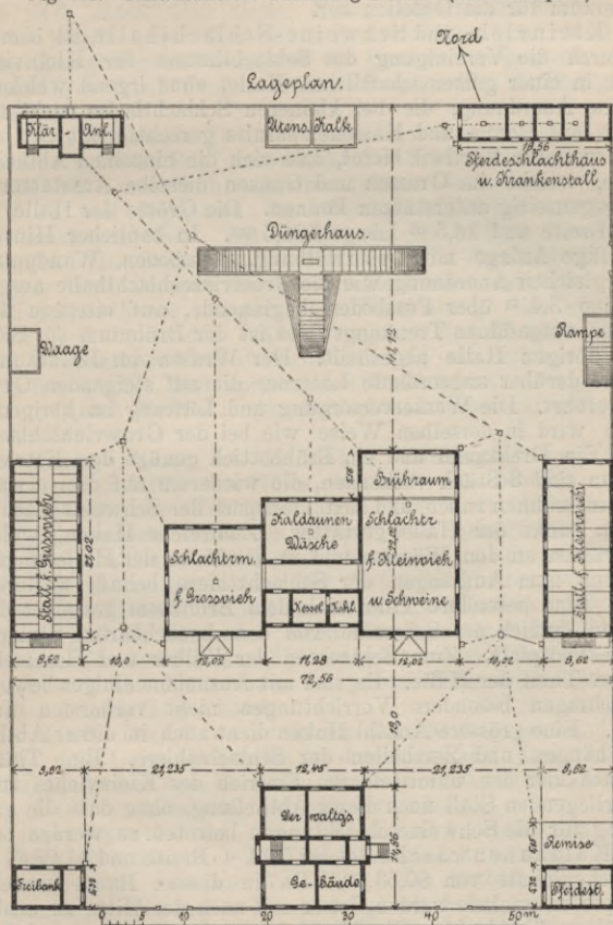
Fig. 188. Schlachthof zu Hirschberg i. Schl. (Arch. Rimpler.)
