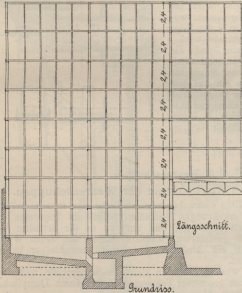
Fig. 72 u. 73. Possehl's Kohlenhof in Hamburg-Altona.
