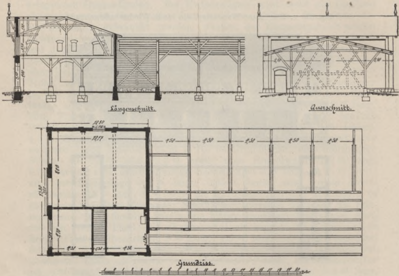
Fig. 335—337. Wagenschauer zu Penzin. Arch. Wagner.
