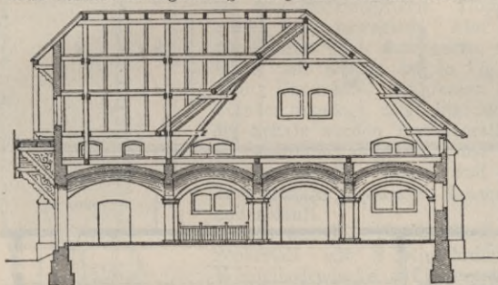
Fig. 243 u. 244. Schafstall zu Neudeck, Gräfl. Henkel'sche Begüterung. Länge des Gebäudes etwa 50 m.
