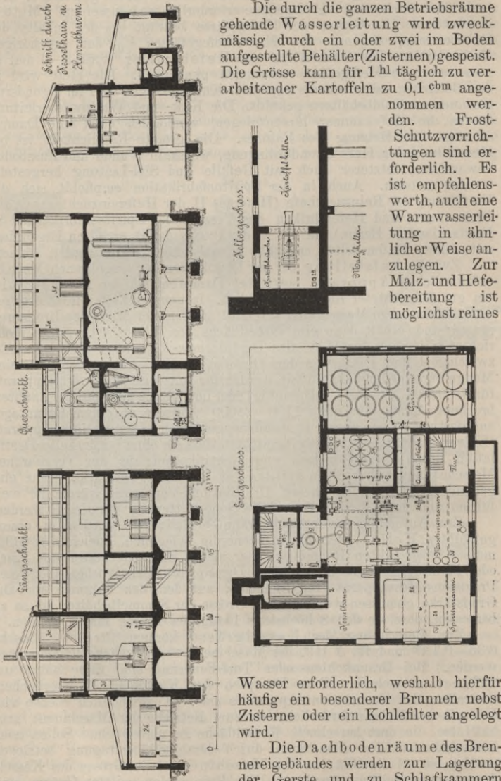
Fig. 405—409. Brennerei von H. F. Eckert Aktiengesellschaft, Berlin-Friedrichsberg.
