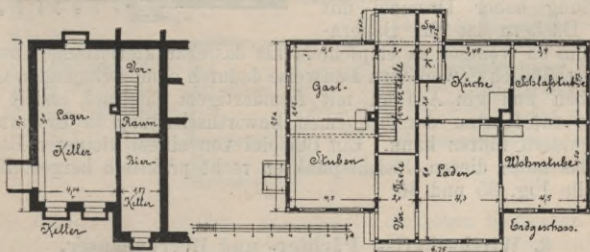
Fig. 33 u. 34. Kaufläden und Krughaus zu Borkow. (Arch. Wagner.)
