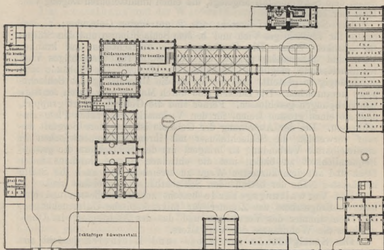
Fig. 189. Schlachthof zu Schwerin. (Arch. Osthoff.)
