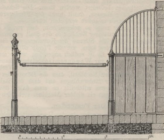
Fig. 11. Pferdestand-Abscheidung mit Lattirbaum. (Pflasterboden.)
