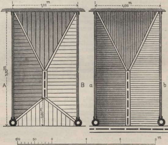
Fig. 12 u. 13. Fussboden in Pferdeständen.
