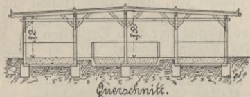
Fig. 17—19. Buchten für ungarische Schweine. (Viehmarkt Breslau).
