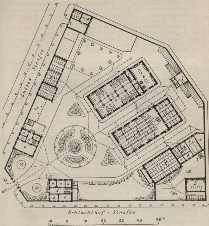
Fig. 191. Schlachthof zu Osnabrück. (Arch. Hackländer.)
