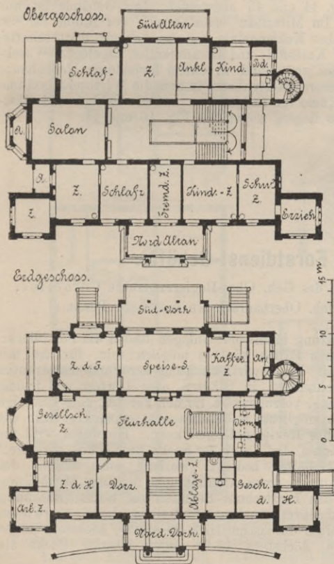
Fig. 46 u. 47. Herrenhaus zu Jessenitz. (Arch. Lange.)
