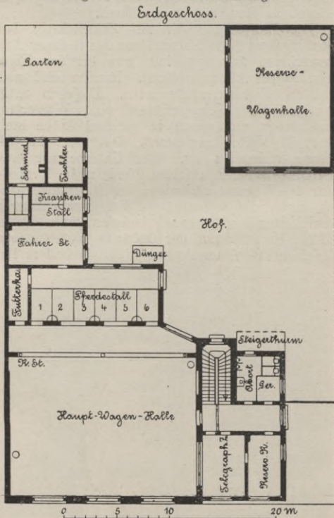
Fig. 61. Feuerwache in Hamburg.
