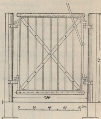
Fig. 28. Buchtenthür mit einseitigem Verschluss.
