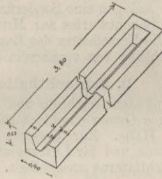
Fig. 42. Schlachtschragen aus Holz.
