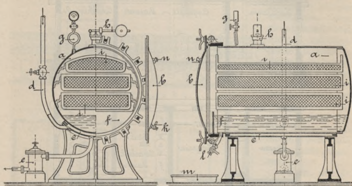
Fig. 137 u. 138. Rud. A. Hartmann'scher Fleisch-Sterilisator.
