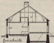
Fig. 24 u. 25. Kathen in Gustaveel. (Arch. Wagner.)
