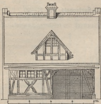
Fig. 21 u. 22. Stall für ein Landhaus. (Arch. B. Ebhardt.)
