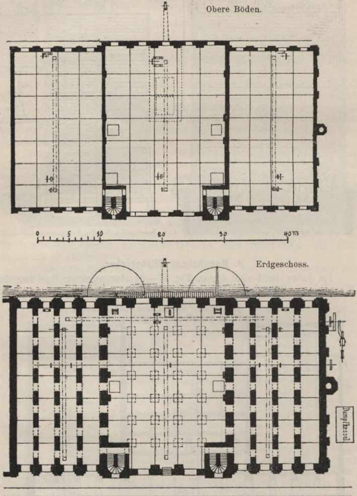
Fig. 58 u. 59. Mannheimer Silospeicher.
