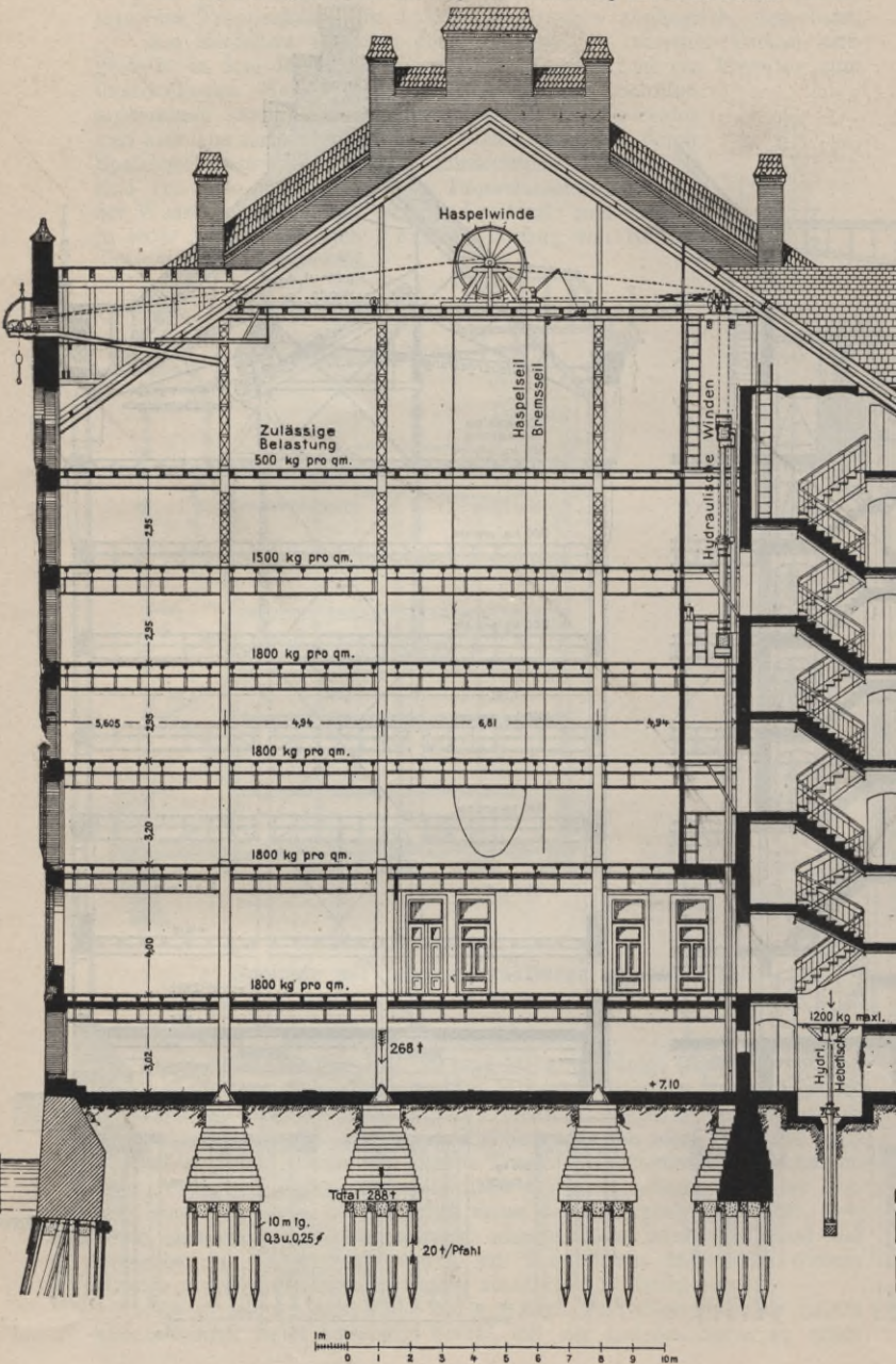
Fig. 30. Speicher in Hamburg. Aus: Hamburg und seine Bauten
