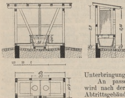
Fig. 60—62. Abtrittgebäude.
