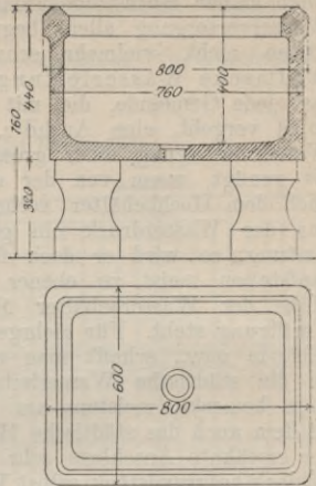
Fig. 158. Spültrog aus gebranntem Thon.
