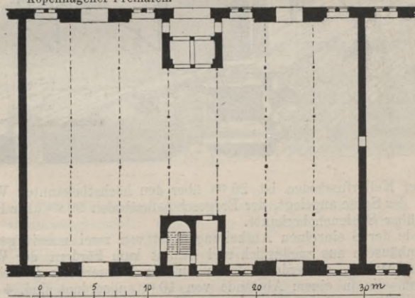
Fig. 45. Packhaus in dem Kopenhagener Freihafen.
