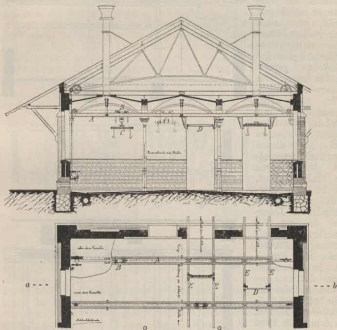
Fig. 53 u. 54. Unruh & Liebig'sche Fördervorrichtung für Grossviehschlachthallen.
