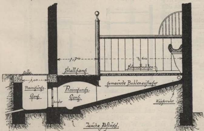
Fig. 16. Pferdestand-Abscheidung mit fester Standwand. Längsschnitt. (Im Stand Dielenboden; in der Stallgasse Klinkerpfaster.)
