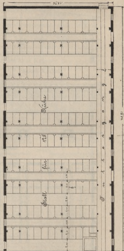
Fig. 231—233. Viehhaus zu Thurow i. M. Arch. Wagner.
