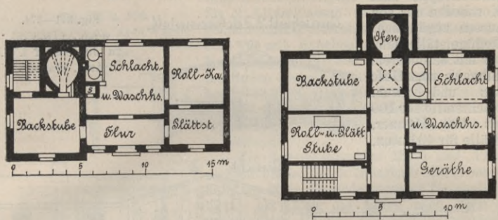
Fig. 369 u. 370. Wirtschaftshaus zu Dobbin i. M. Arch. Wagner.
