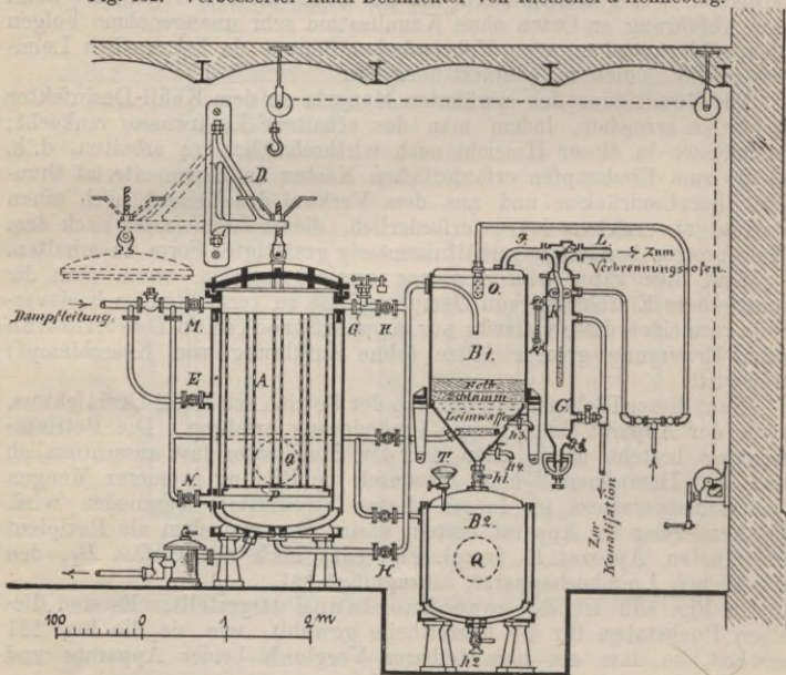
Fig. 132. Verbesserter Kaffil-Desinfektor von Rietschel & Henneberg.
