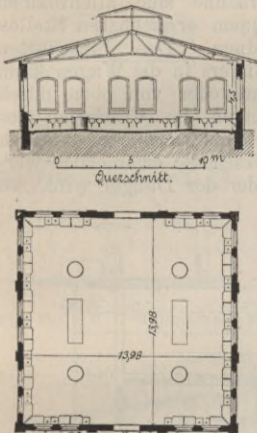
Fig. 103 u. 104. Kuttelei für Grossvieh. (Arch. Osthoff.)
