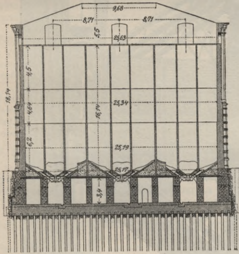
Fig. 64. Silospeicher in Galatz (Querschnitt).
