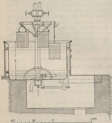
Fig. 100 u. 101. Brühbottich für Kutteleien.
