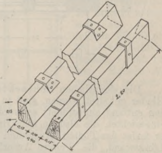
Fig. 42. Schlachtschragen aus Holz.
