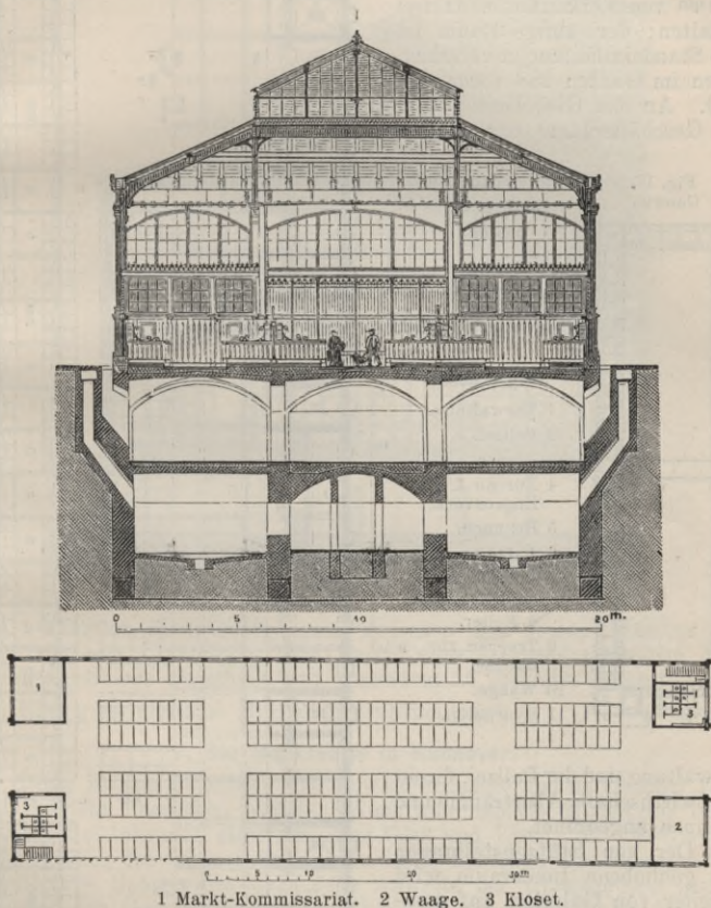
Fig. 16 u. 17. Detail-Markthalle an der Stubenbastei zu Wien. (Arch. Ob.-Ing. Haussmann)
