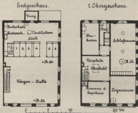
Fig. 61. Feuerwache in Hamburg.
