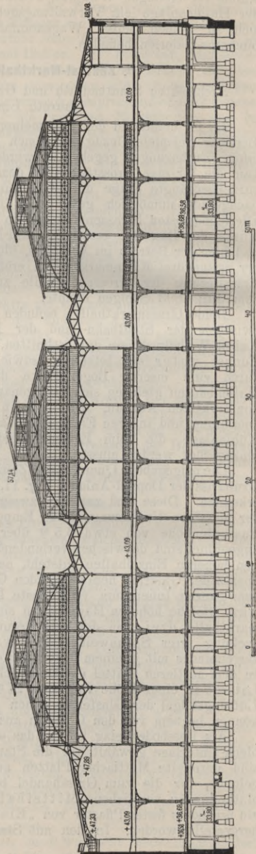
Fig. 10. Querschnitt durch die Zentral-Markthalle in Berlin.
