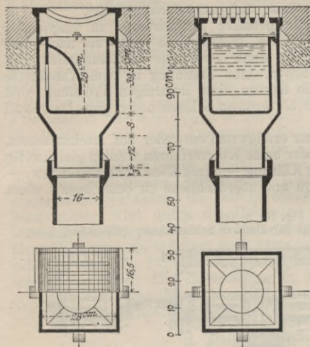
Fig. 159 u. 160. Sinkkasten mit Wasserverschluss.
