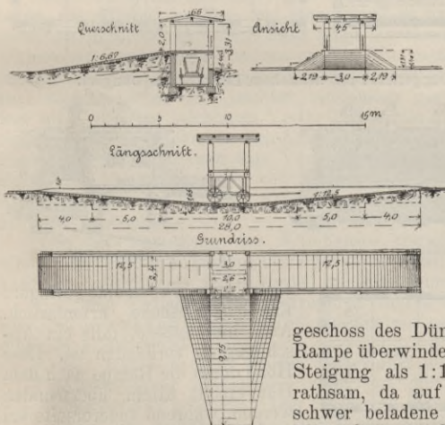
Fig. 110 u. 111. Düngerhaus für einen kleinen Schlachthof.
