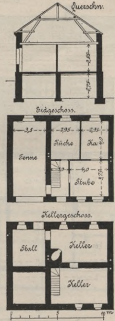
Fig. 19 u. 20. Wohnhaus f. ländl. Arb. in Waterneverstorff.
