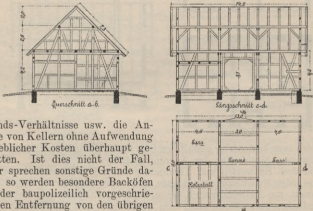
Fig. 57—59. Scheune.
