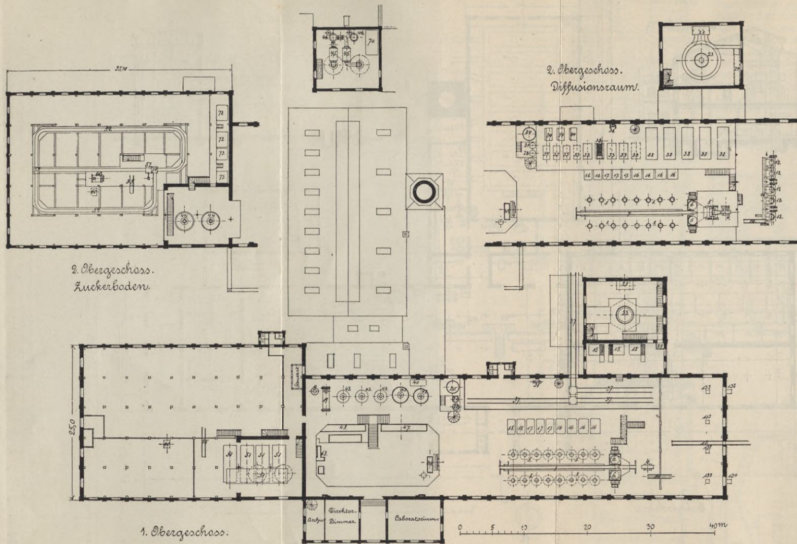
Fig. 419—422. Zuckerfabrik Friedrichsthal. Halle'sche Maschinenfabrik und Eisengiesserei.
