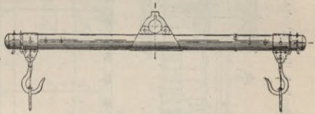
Fig. 64. Spreize mit Gelenkhaken.
