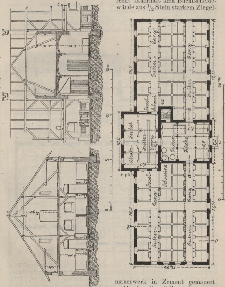
Fig. 262-264. Schweinstall auf der Domaine Kinderhof (Ostpreussen).
