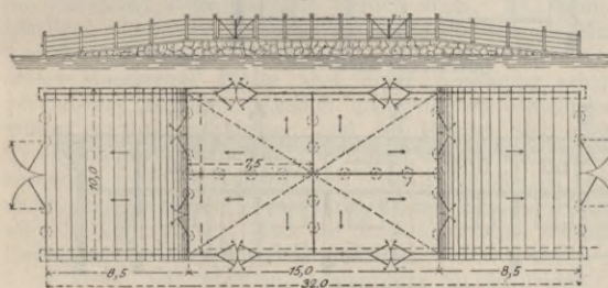
Fig. 7. Laderampe für Landfuhrwerk.
