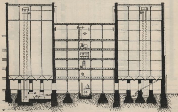
Fig. 57. Mannheimer Silospeicher (Längsschnitt).
