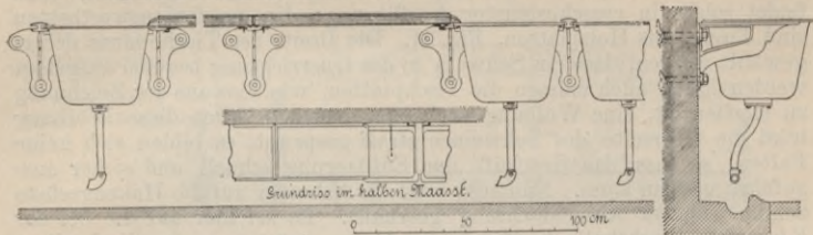
Fig. 98 u. 99. Kaldaunenwaschgefäße und Entfettungstischplatten.
