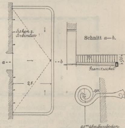
Fig. 81—83. Tödtbuchten mit Anbindehaken für Schweineschlachthallen.
