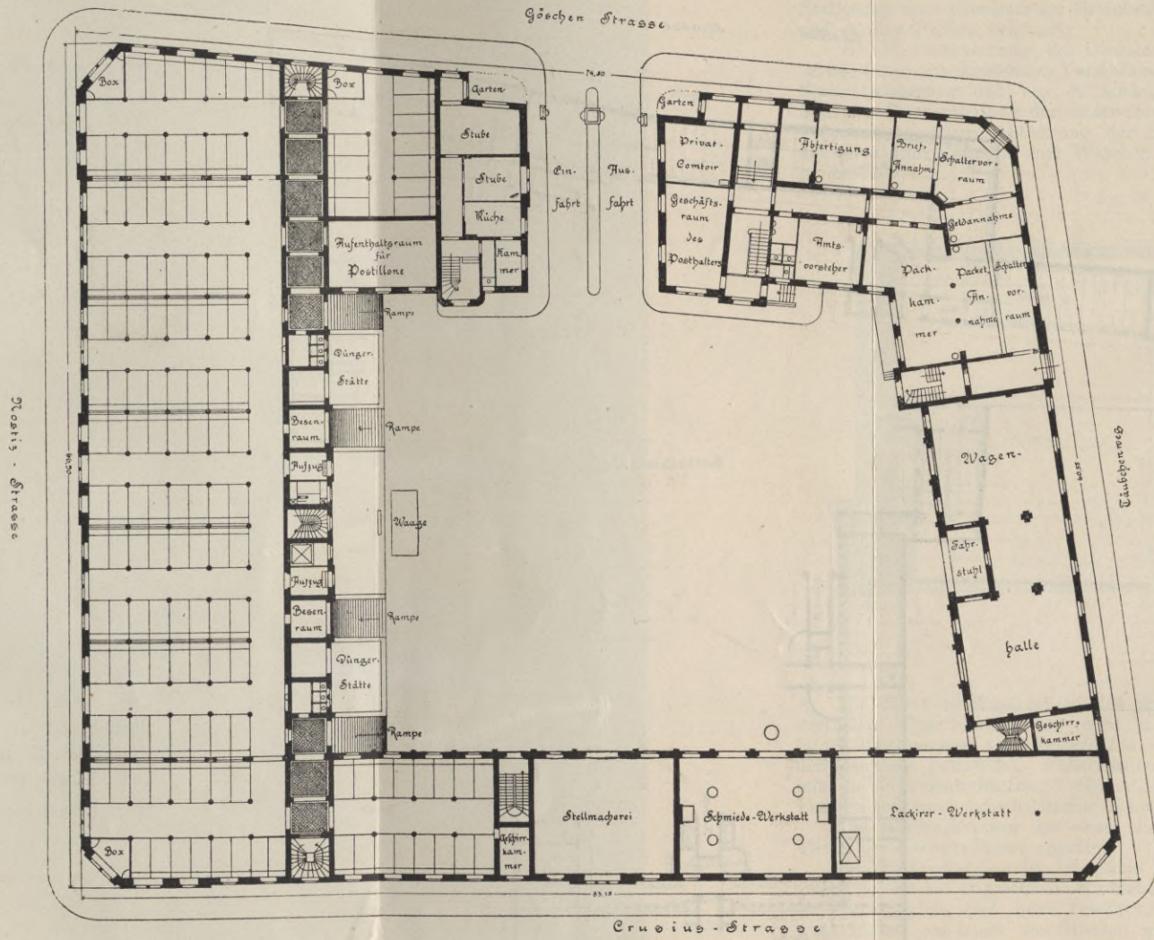
Fig. 57. Neues Posthalterei-Gebäude in Leipzig. Erdgeschoss. (Arch. Paul Jäger in Berlin.)
