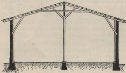
Binder im Bansen.
