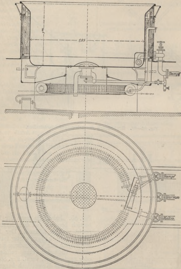
Fig. 89 u. 90. Brühbottich mit Alex. Huber'scher Lüftungsvorrichtung.
