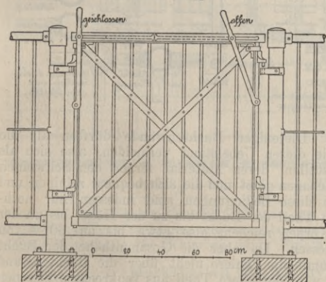
Fig. 24. Buchtenthür mit doppeltem Verschluss.
