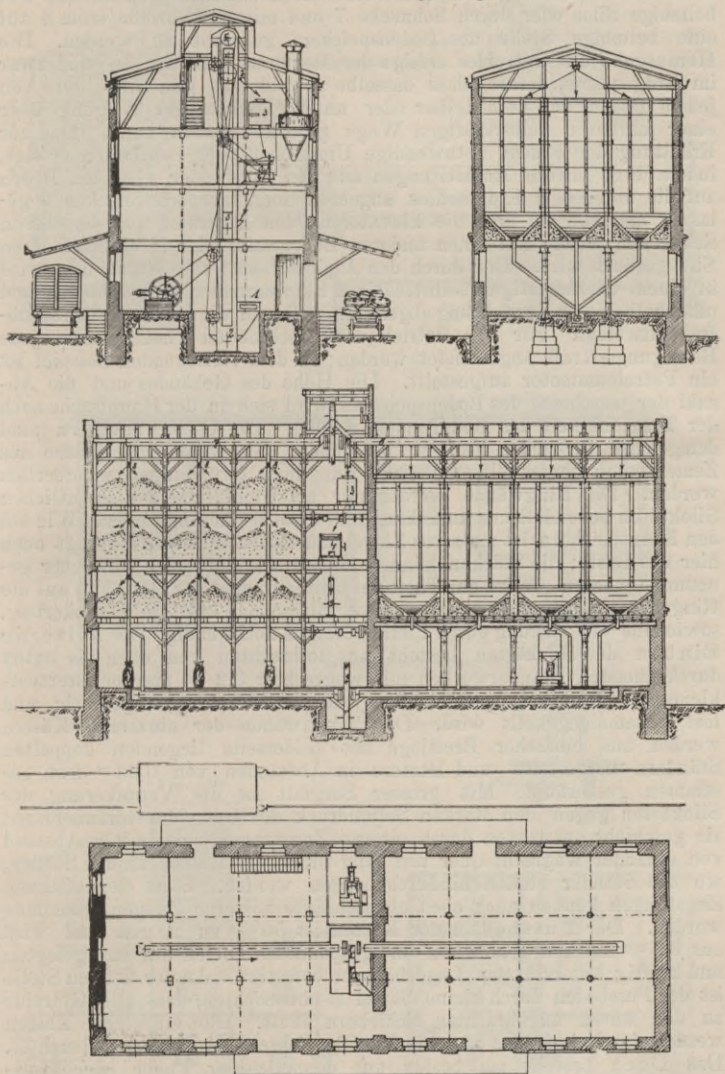
Fig. 124—127. Maschinenfabrik für Mühlenbau vorm. C. G. W. Kappler, Berlin. Aus „Illustr. Landw. Zeitung, Jahrg. 1896.“
