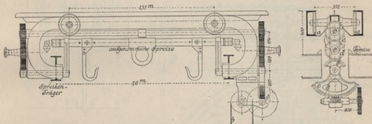
Fig. 59 u. 60. Beck & Henkel'sche Fleischförderwagen.
