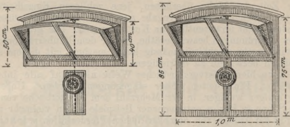
Fig. 2 u. 3. Lüftungs-Stallfenster besonders stark konstruiert, mit Rahmen und Stein- schrauben zum Einmauern. Mittels des Gegengewichtes lässt sich der obere Flügel, der den Zutritt der Luft von Aussen gestattet, beliebig offen halten.
