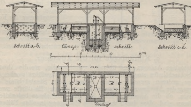
Fig. 161 u. 162. Beispiel einer Abwässer-Kläranlage für kleinere Schlachthöfe. (Hirschberg i. Schl.)
