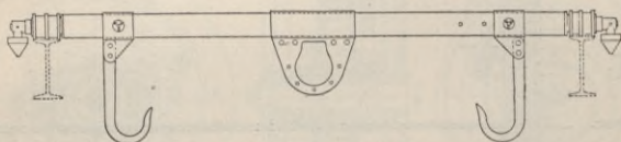
Fig. 52. Spreize für bewegliche Winden.
