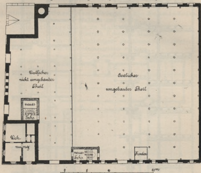
Fig. 19. Ehemaliger Silospeicher in Hamburg.
