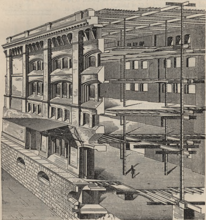
Fig. 43. Niederlagsgebäude der neuen Packhofsanlage in Berlin.
