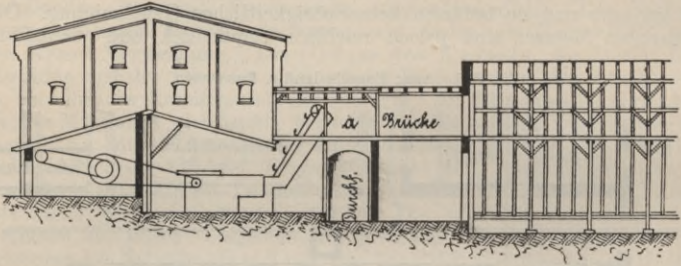
Fig. 347 u. 348. Maschinenhaus zu Wahrstorf i. M. Aus: Engel's landw. Bauten.
