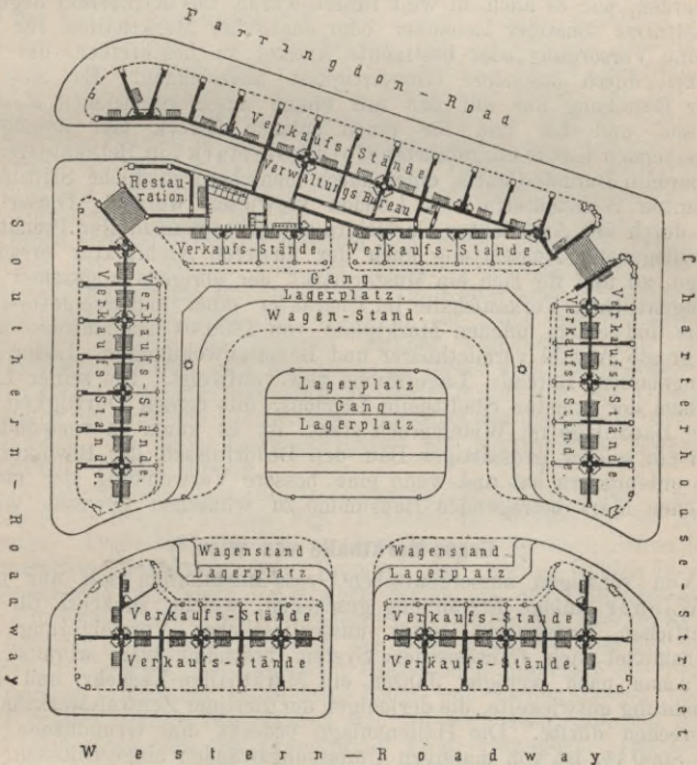
Fig. 9. Früchte- und Gemüse-Markthalle in London, Smithfield.
