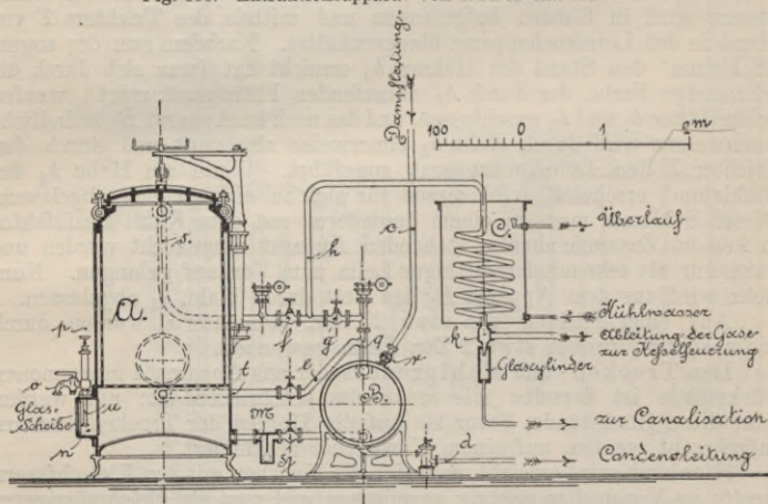
Fig. 133. Extraktionsapparat von Rud. A. Hartmann.
