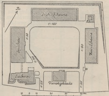
Fig. 92. Proviantamt zu Gleiwitz. (Vorentwurf.)
