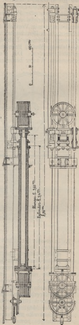
Fig. 3. Presswasserwinde.
