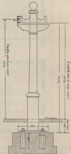
Fig. 75 u. 76. Gerüstsäulen mit Hakenrahmen für Kleinviehslachthallen.
