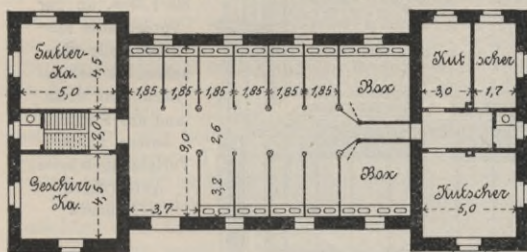
Fig. 1. Schema zu einem Stall für 12 Pferde.
