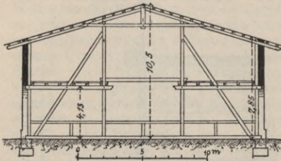
Binder an der Tenne.
