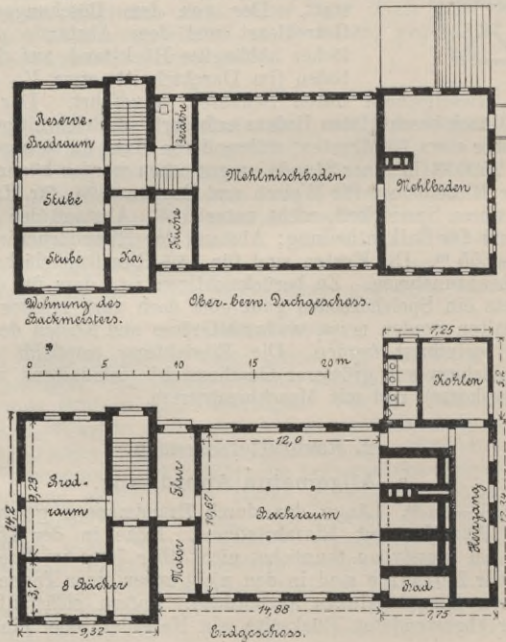
Fig. 96 u. 97. Garnison-Bäckerei zu Saarbrücken.
