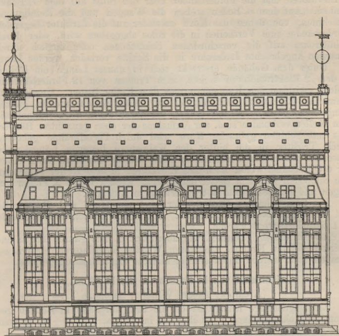
Fig. 68 u. 69. Silospeicher in dem Freihafengebiet zu Kopenhagen.
