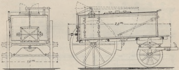
Fig. 110 u. 111. Düngerhaus für einen kleinen Schlachthof.
