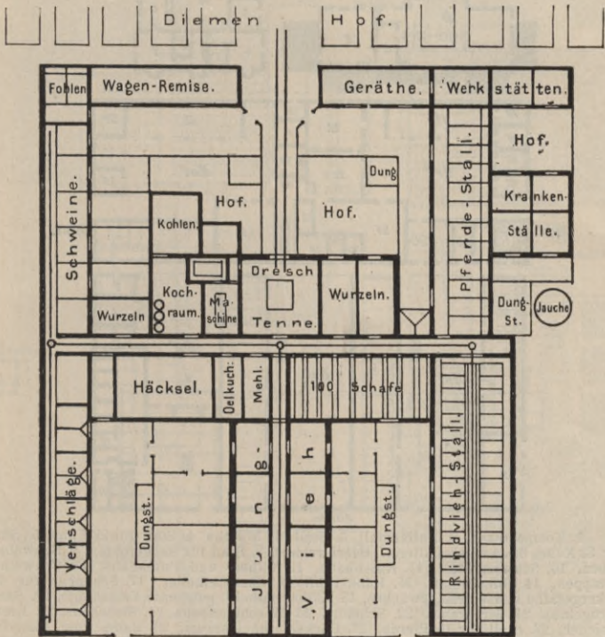
Fig. 40. Schottische Farm.
