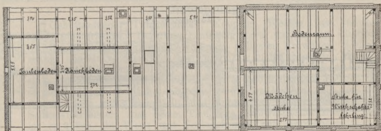
Fig. 369 u. 370. Wirtschaftshaus zu Dobbin i. M. Arch. Wagner.
