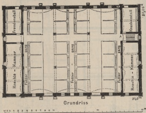
Fig. 189. Arch. Thormann-Wismar.
