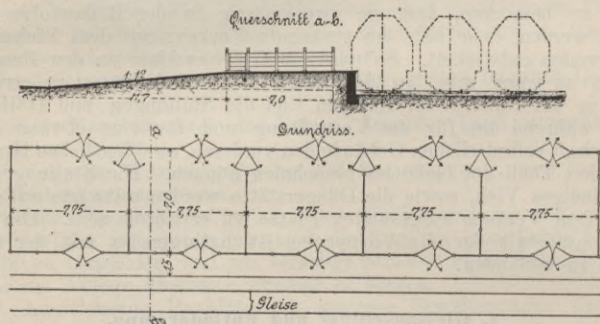
Fig. 1. Entladerampe für Eisenbahnbetrieb.
