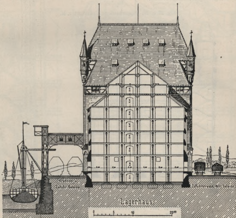
Fig. 26. Lagerhaus zu Worms.
