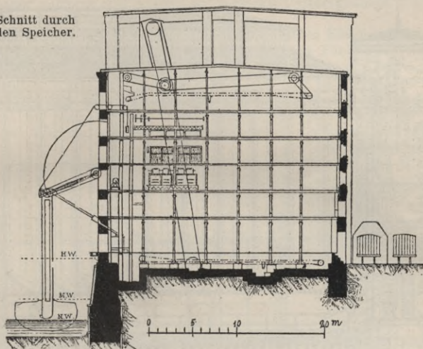
Fig. 60 u. 61. Mannheimer Silospeicher.
