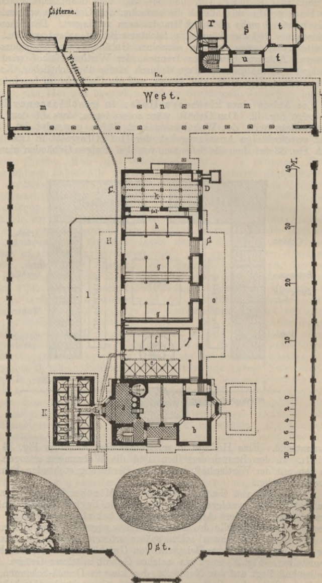
Fig. 33. Hof „Obergott“ in Oberösterreich. (Arch. Achill Wolf.)
