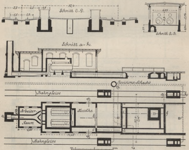
Fig. 32—35. Desinfektionsanstalt für Viehmarktgleise.
