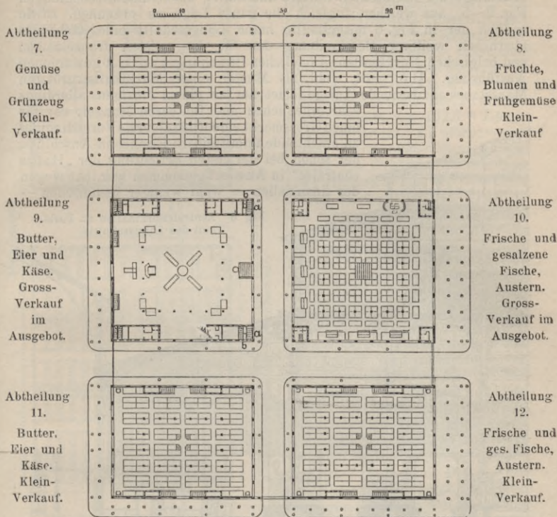
Fig. 5. Untergeschoss unter den Abteilungen 9-12.
