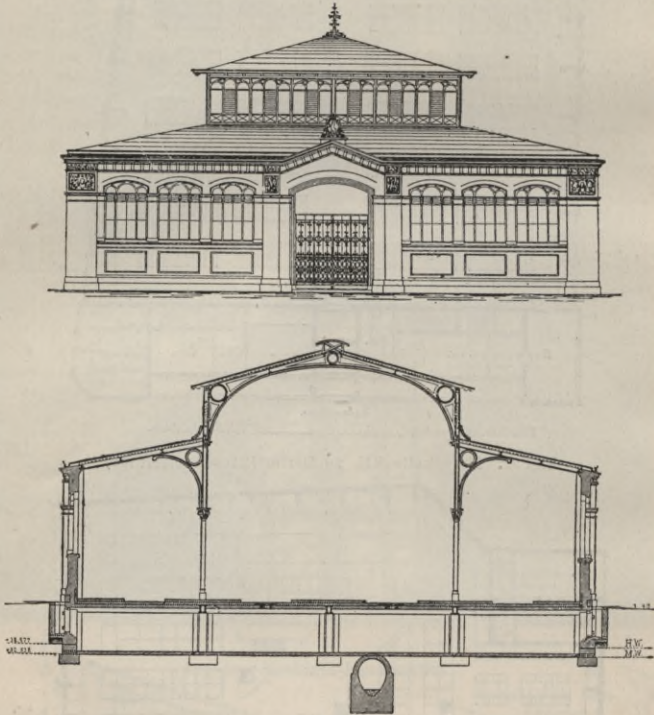
Fig. 33 u. 34. Markthalle V. zu Berlin (Magdeburger Platz).
