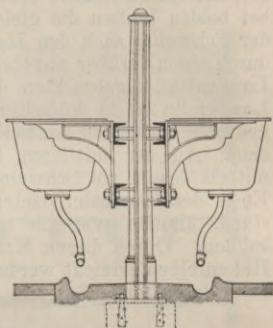
Fig. 102. Waschtisch für Kutteleien.
