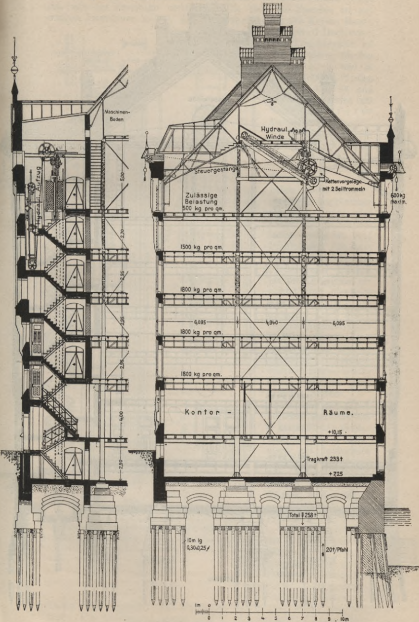
Fig. 29. Speicher in Hamburg. Aus: Hamburg und seine Bauten
