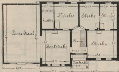
Fig. 33 u. 34. Kaufläden und Krughaus zu Borkow. (Arch. Wagner.)
