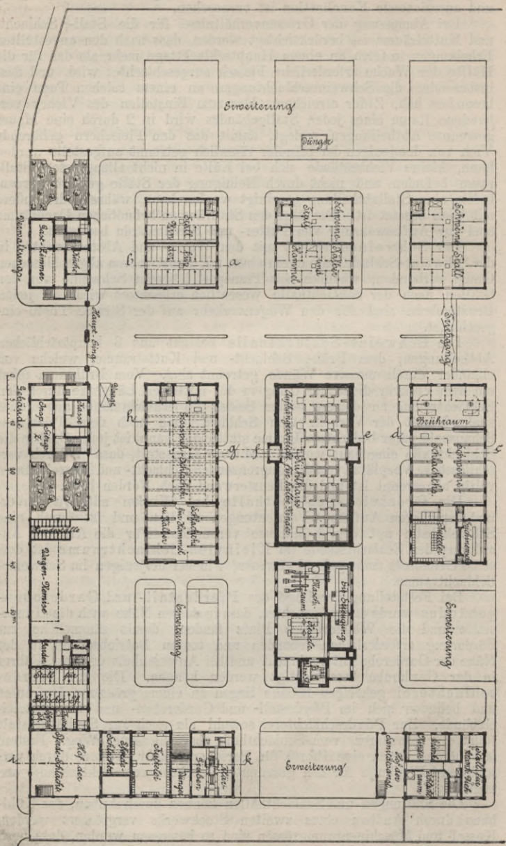
Fig. 190. Schlachthof zu Gera. (Arch. Kögler.)
