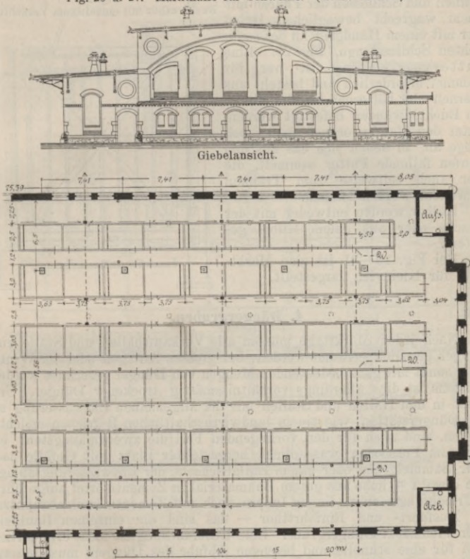
Fig. 26 u. 27. Markthalle für Schweine. (Arch. Osthoff.)
