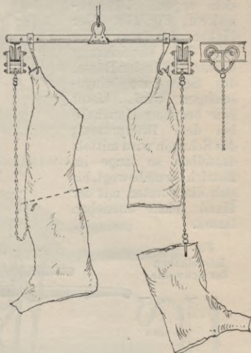
Fig. 175. Vorrichtung zum Vierteln der Rinder bei beweglichen Winden.
