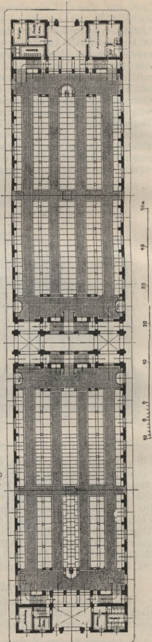
Fig. 23. Markthalle zu Dresden (auf dem Antonplatz). Unterer Grundriss.
