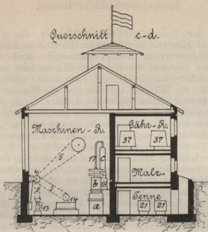
Fig. 410—412. Brennerei nach System Hampel in Dresden.
