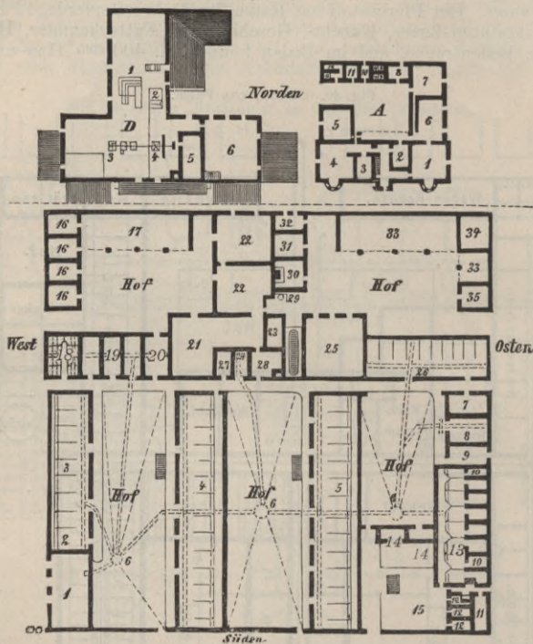
Fig. 41. Englischcs Mustergehöft Farm Liscard in Cheshire.
