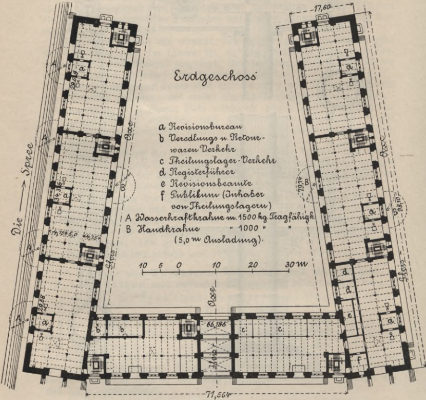
Fig. 42. Niederlagsgebäude der neuen Packhofsanlage in Berlin.
