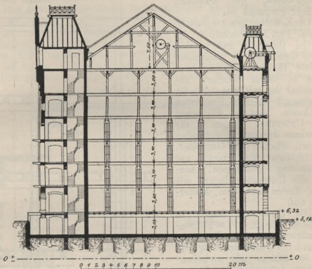
Fig. 16 u. 17. Bremer Freihafenspeicher
