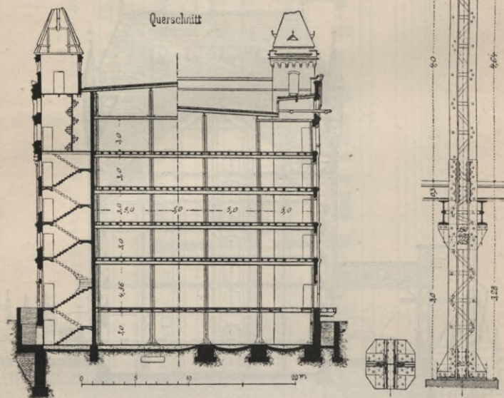
Fig. 27 u. 28. Lagerhaus zu Frankfurt a. M.
