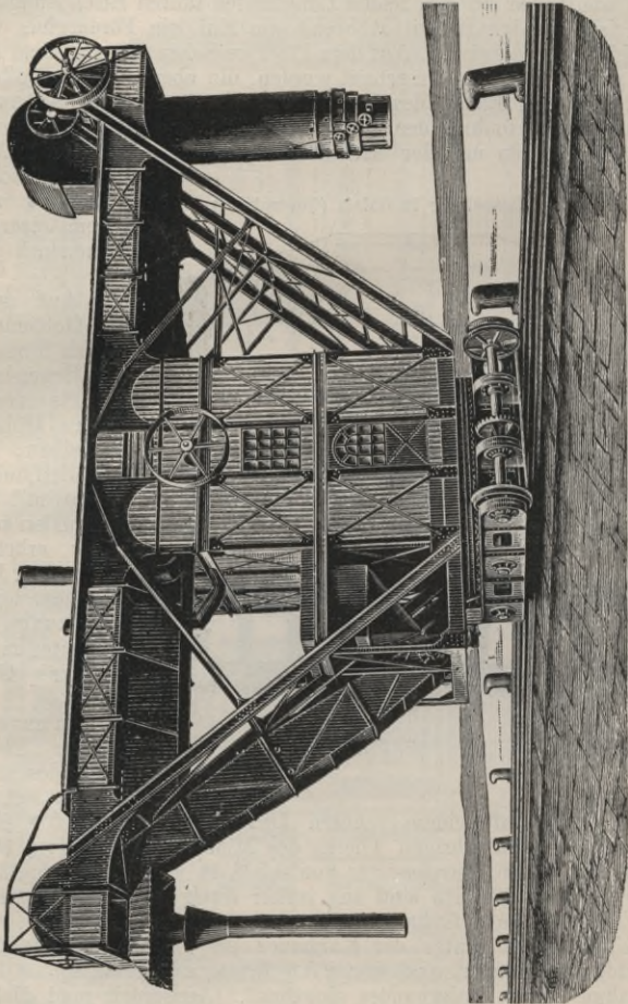
Fig. 65. Fahrbarer Teleskop-Elevator am Kai der Dockanlagen zu Galatz und Braila.
