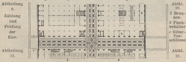
Fig. 2-5. Zentral-Markthallen zu Paris. Grundrisse. (Arch. V. Baltard.)
