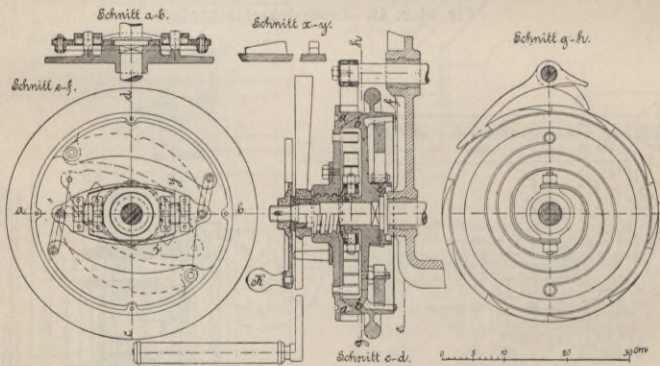
Fig. 46—48. Sicherheitsantrieb mit Geschwindigkeitsbremse für Grossviehschlachtwinden.
