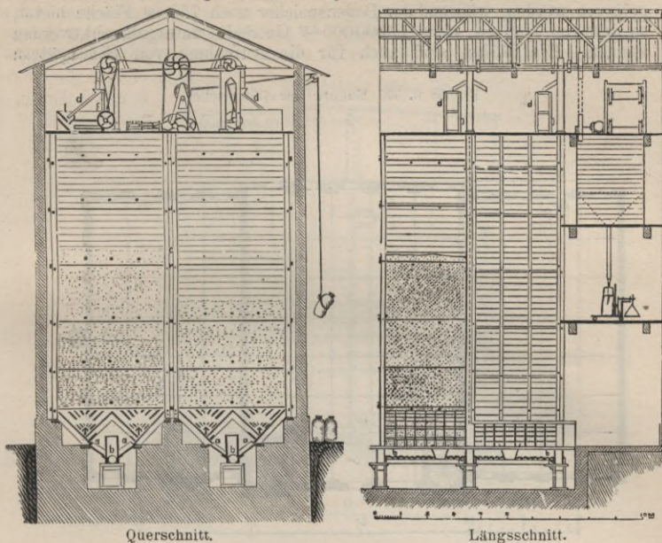
Fig. 55 u. 56. Silospeicher in Cambray.
