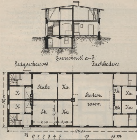
Fig. 14 u. 15. Vierfamilienhaus der Regierung zu Stettin.
