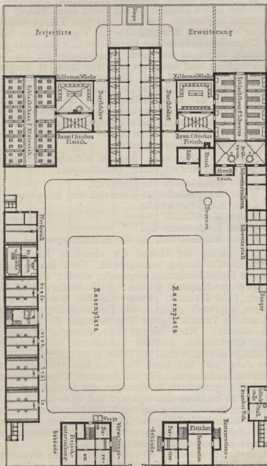
Fig. 187. Schlachthof zu Erfurt. (Arch. Spielhagen.)
