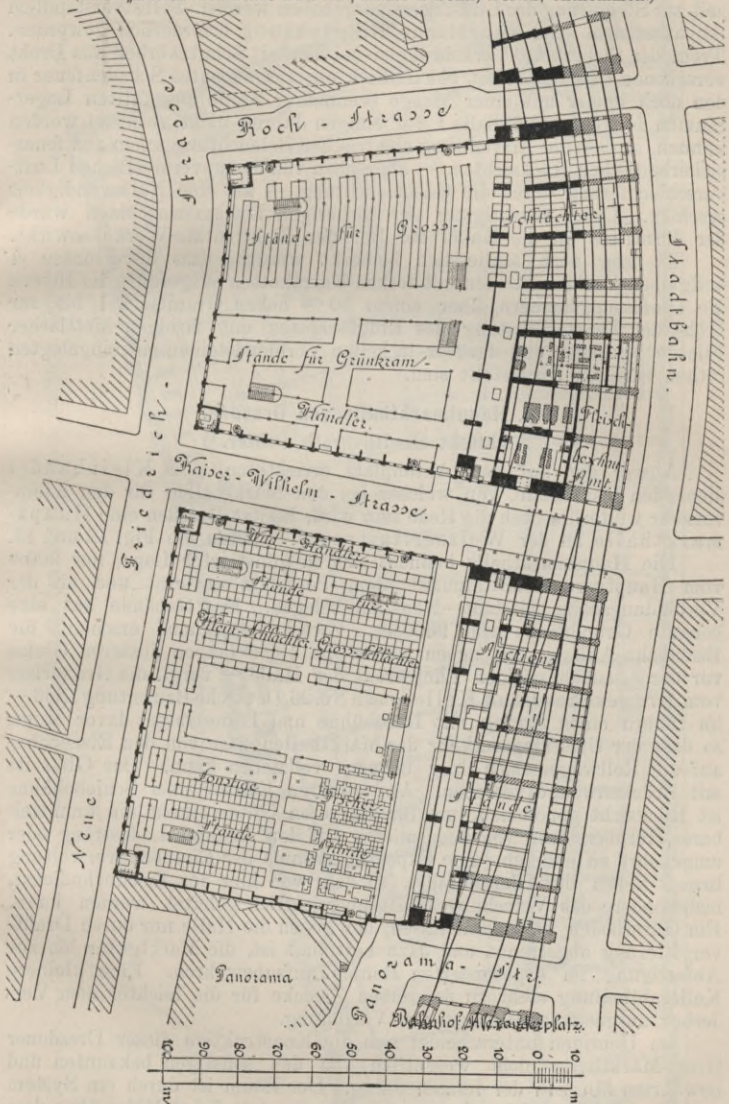
Fig. 11. Zentral-Markthalle in Berlin. (Aus „Berlin und seine Bauten“, Ernst & Sohn, Berlin, entnommen.)
