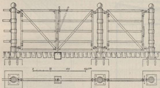
Fig. 2. Einzelkonstruktion der Buchten für feste Entladerampen.
