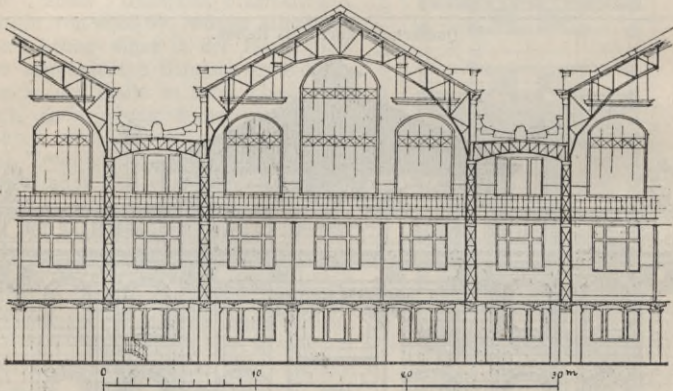
Fig. 26. Markthalle zu Leipzig. (Arch.: Stadtbrth. Licht.)
