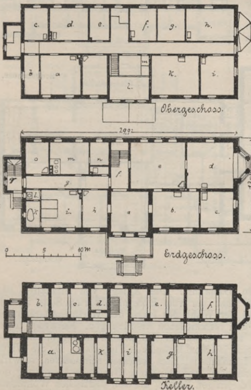
Fig. 41—43. Herrenhaus in Ostpreussen. (Arch. Engel.)
