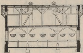
Längenschnitt durch den Hutschstall.
