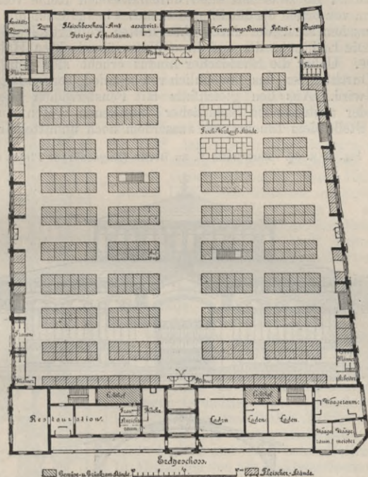
Fig. 32. Markthalle VII. zu Berlin (Dresdenerstrasse).
