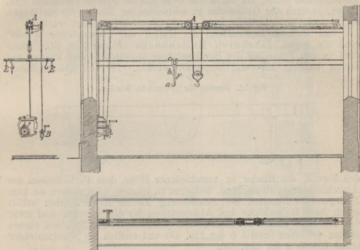
Fig. 49—51. Bewegliche Winde für Grossviehschlachthallen.
