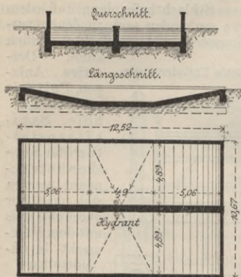
Fig. 3. Wäsche für Schweine.
