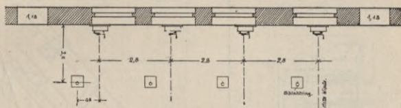
Fig. 39. Anordnung von Winden und Einriebthüren.
