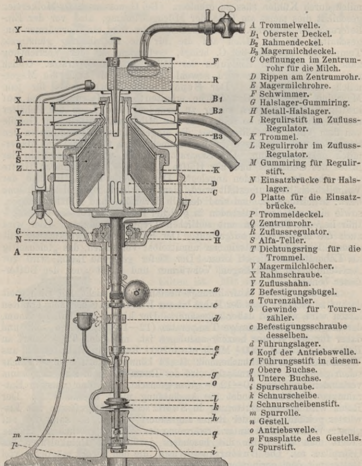
Fig. 390. Alfa-Separator. Bergedorfer Eisenwerke.
