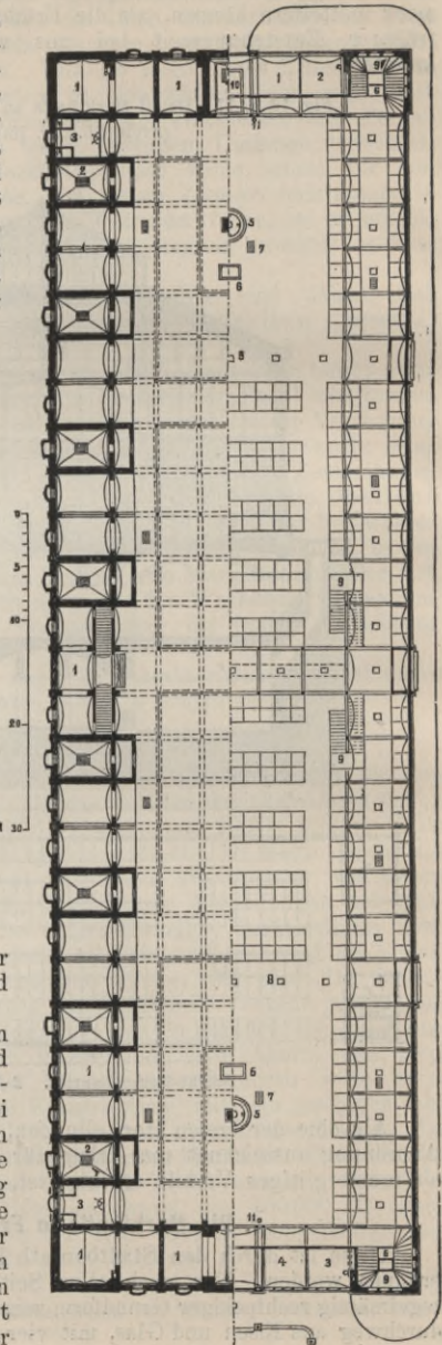
Fig. 19. Markthalle zu Frankfurt a. M. (Arch. Behnke.) Keller. Erdgeschoss.
