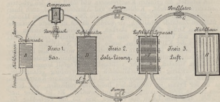
Fig. 129. Schematische Darstellung einer Schlachthof-Kühlanlage.
