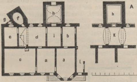
Fig. 38 u. 39. Wirtschaftshaus für ein grösseres Gut. (Arch. Wagner.)
