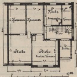
Fig. 29. Wohnhaus für Gutsunterbeamte. (Arch. Wagner.)
