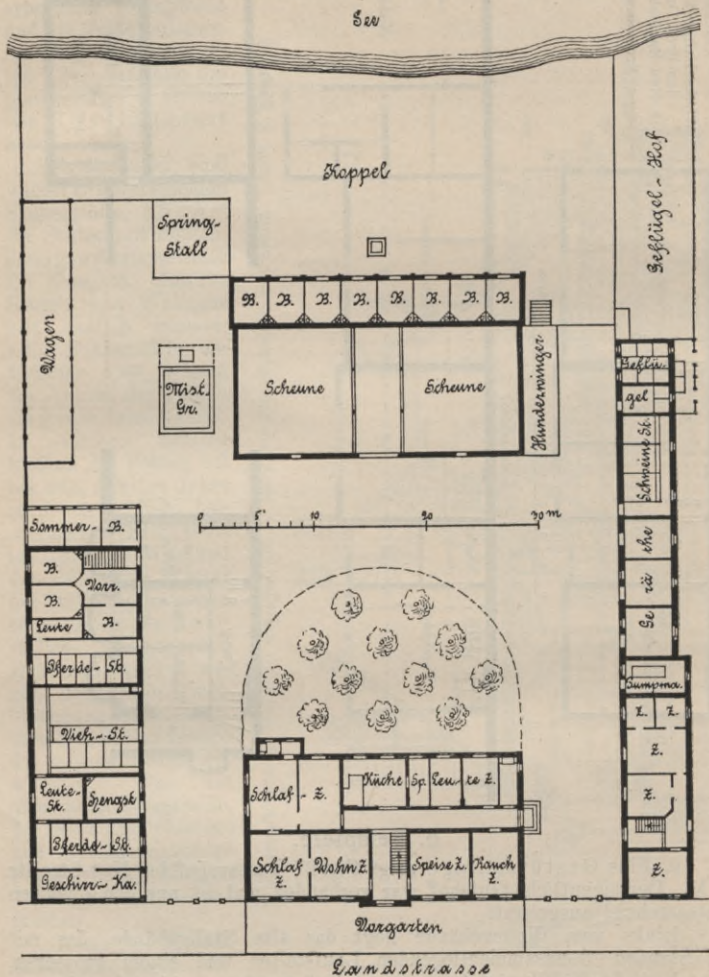
Fig. 27. Gestüt Gustavshof bei Neu-Strelitz i. M. (Arch. B. Ebhardt)
