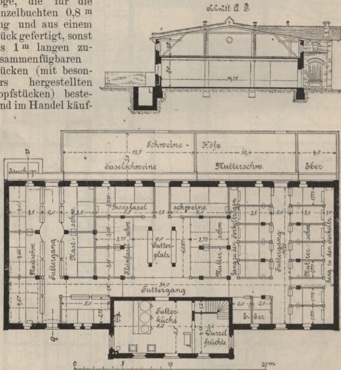
Fig. 265 u. 266. Deutsche Landw. Gesellschaft. Entw. vom Eisenhütten- und Emailirwerk Neusalz a. O.]
