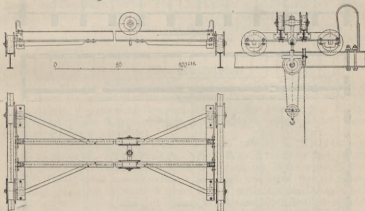
Fig. 92—94. Fahrbarer Krahn mit Laufkatze.
