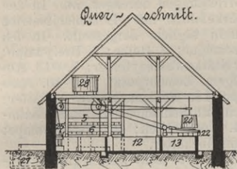
Fig. 413—415. Fabrikanlage von W. Schneider & Co. in Frankfurt a. O. Aus: „Engel's landw. Bauwesen.“
