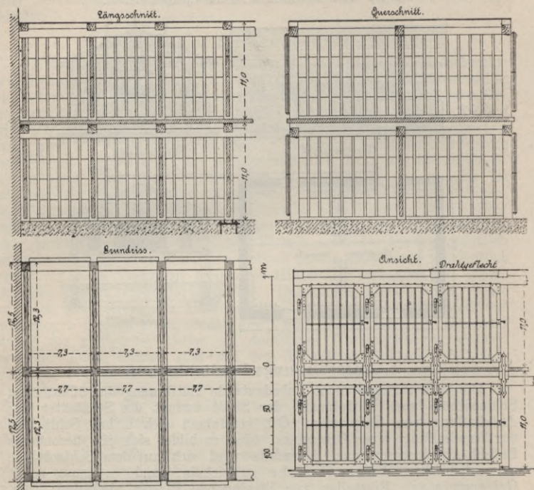
Fig. 154—157. Konstruktion der Hundekäfige.
