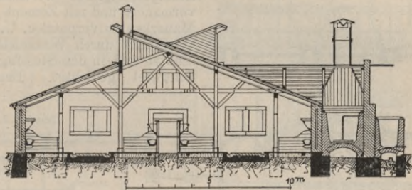
Fig. 221 u. 222. Kuhstall einer Meierei bei St. Petersburg.
