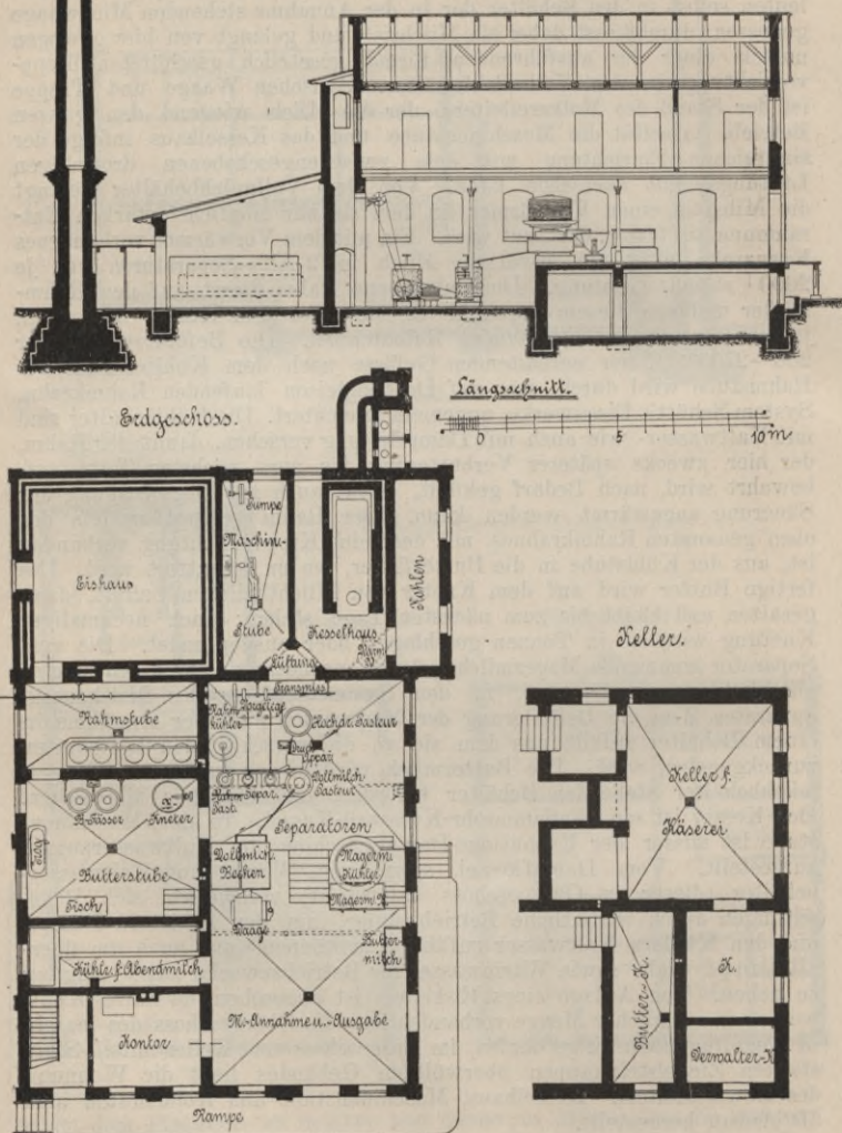
Fig. 399—401. Genossenschafts-Molkerei Triebsees i. Pom. Schütt's Eisenwerke in Gnoiën.
