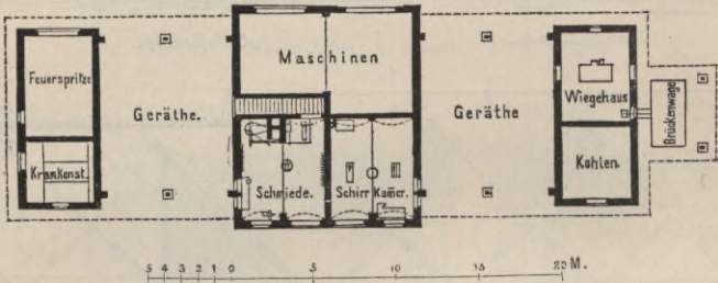
Fig. 344 u. 345. Schmiede zu Melkof i. M. Hofzimmerstr. Heins.
