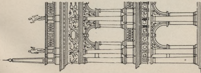
A. Bibliothek S. Marco Venedig
