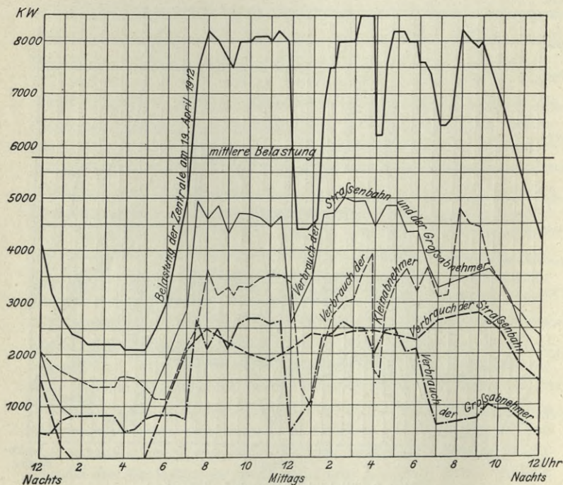
Fig. 3. Elektrizitätswerk I. (Sommer.)
