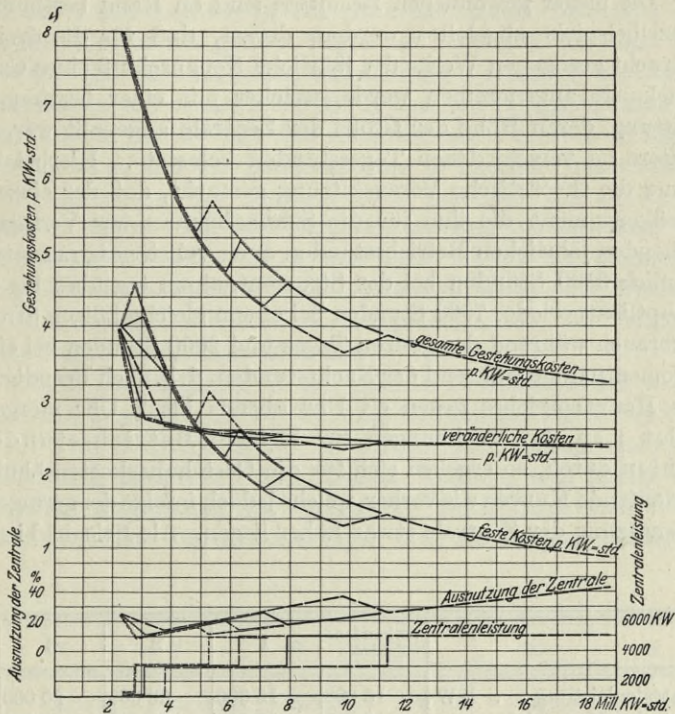
Fig. 11. Elektrizitätswerk III. Stromerzeugungskosten.
