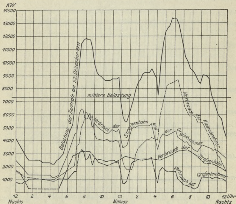
Fig. 2. Elektrizitätswerk I. (Winter.)
