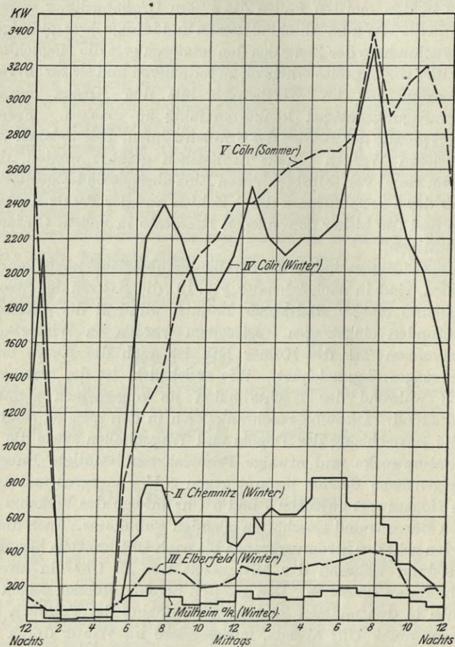
Fig. 13. Stromverbrauch städtischer Straßenbahnen.
