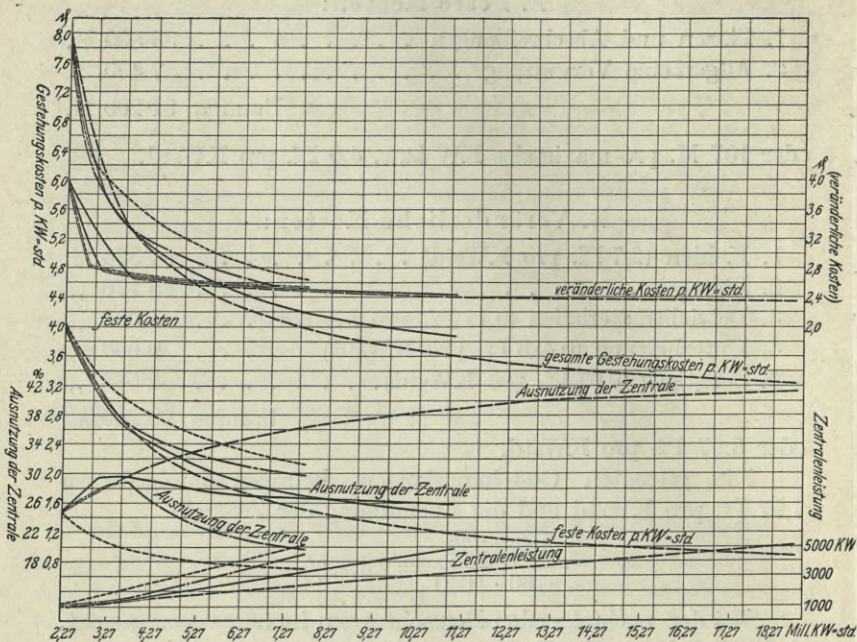
Fig. 10. Elektrizitätswerk III. Stromerzeugungskosten.
