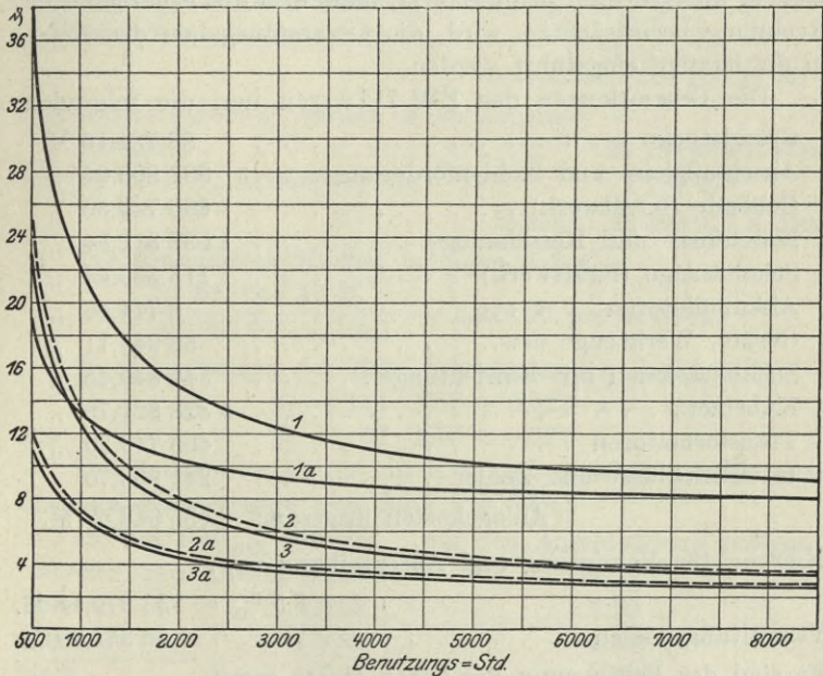
Fig. 16. Gestehungskosten pro nutzbare KWstd.
