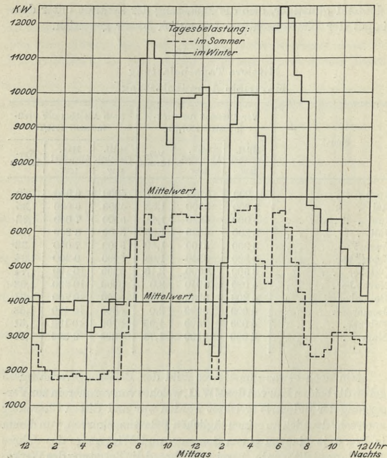
Fig. 4. Elektrizitätswerk II.
