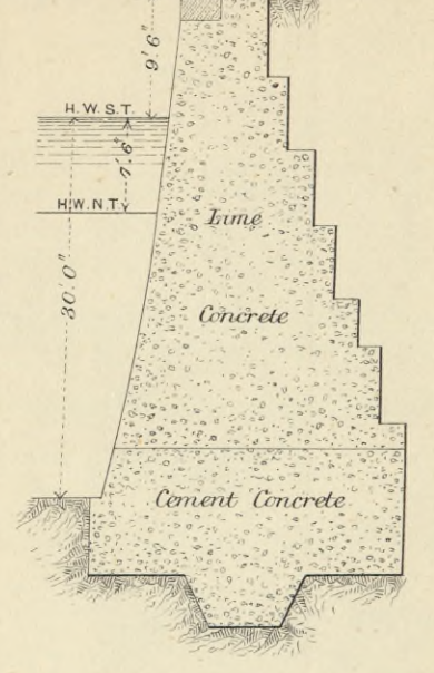
Fig. 13. BARROW TIDAL BASIN.
