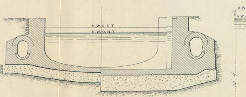
Fig. 10. SECTION ON D.D.
