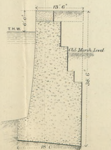
Fig. 7. LONDON. ALBERT DOCK
