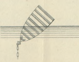
Fig. 20. CAN BUOY.
