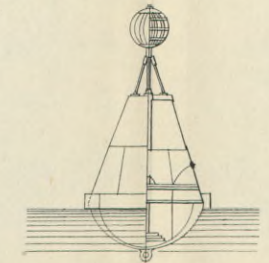
Fig. 14. BEACON BUOY.
