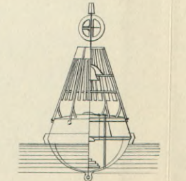
Fig. 16. BELL BUOY.
