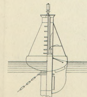
Fig. 17. WHISTLING BUOY.
