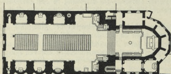
Abb. 43. St. Michael. Grundriß. Nach den Kunſtdenkmälern des Königreichs Bayern.
