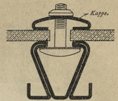
Sprosse von Rendle . (System Invincible 153).
