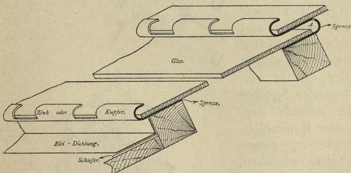
Deckung von Rendle (System Simple 153).
