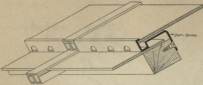
Deckung von Rendle. (System Acme 1858). 1/4 n. Gr.
