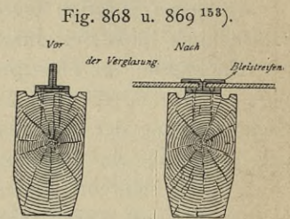
Sprosse von Drummond 153). 1/2 n. Gr.
