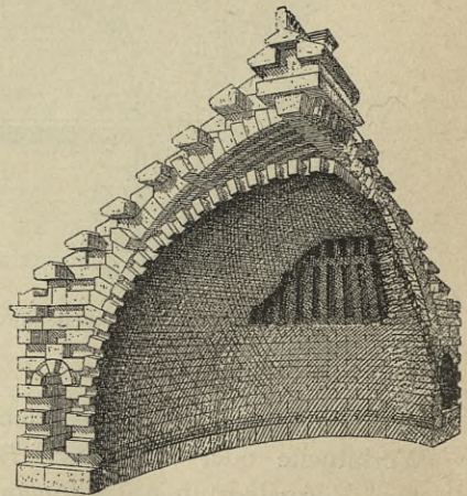
Vom Chordach der Kirche Sacré-Coeur de Montmartre zu Paris 203) .
