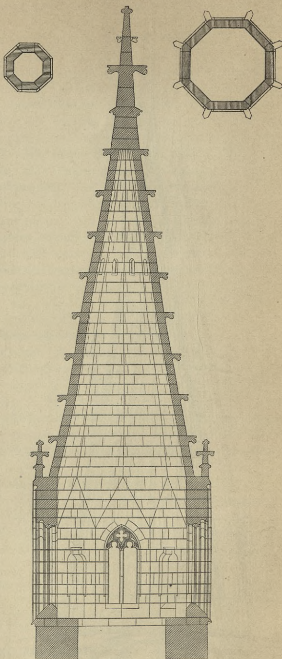
Thurmhelm der Oberhohen-Kirche zu Göppingen.
