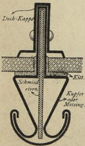
Sproffe System Hayes 153) .
