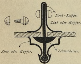
Sproffe von Shelley.
