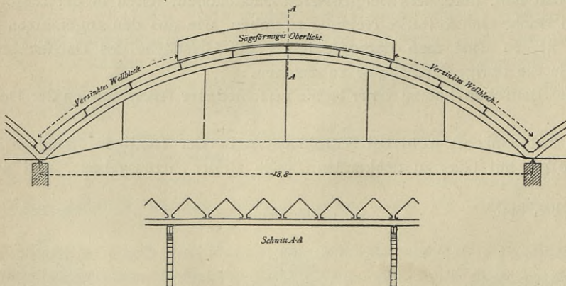
Von der Bahnhofshalle zu Oberhausen 153 . 1/200 n. Gr.
