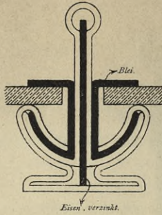
Sproffen von Pennycook 153) .
