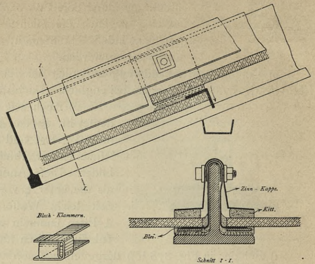
Glasdeckung von Göller 153 , 1/2 n. Gr.
