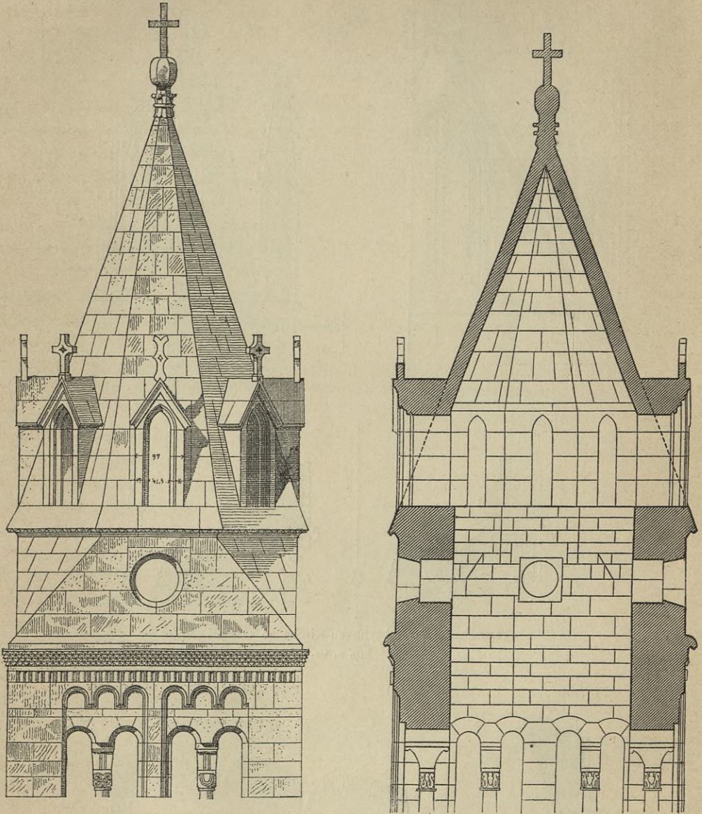
Helm des nördlichen Chorthurmes der Abtei-Kirche zu Groß-Comburg 197 .
