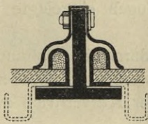
Sproffen von Drummond 153) . 1/2 n. Gr.
