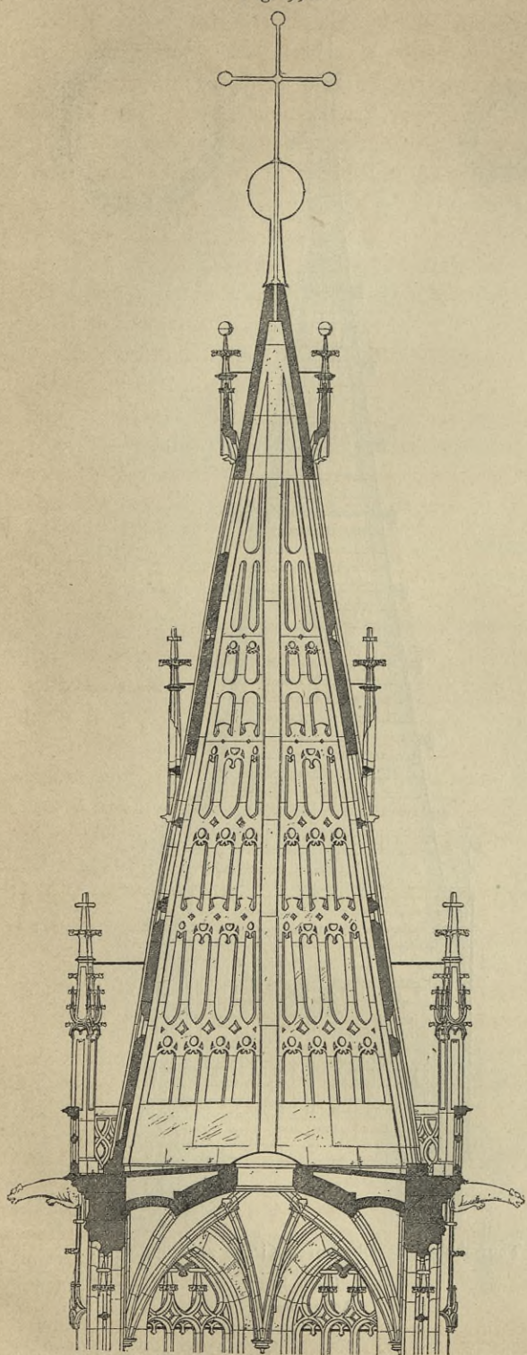
Thurmhelm der Pfarrkirche zu Bozen 195) .
