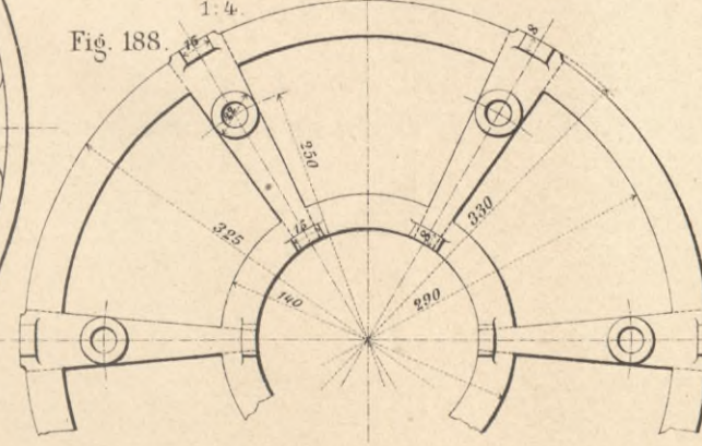
Rückansicht der Bürstenscheibe.
