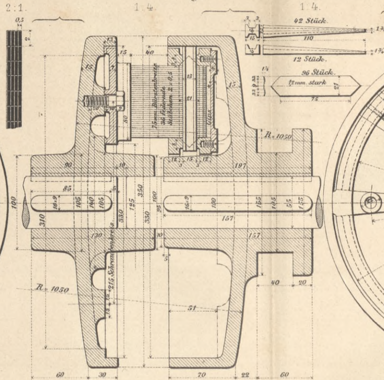
Fig. 186. Kupplungshälfte für die Bürstenscheibe. 1:4.
