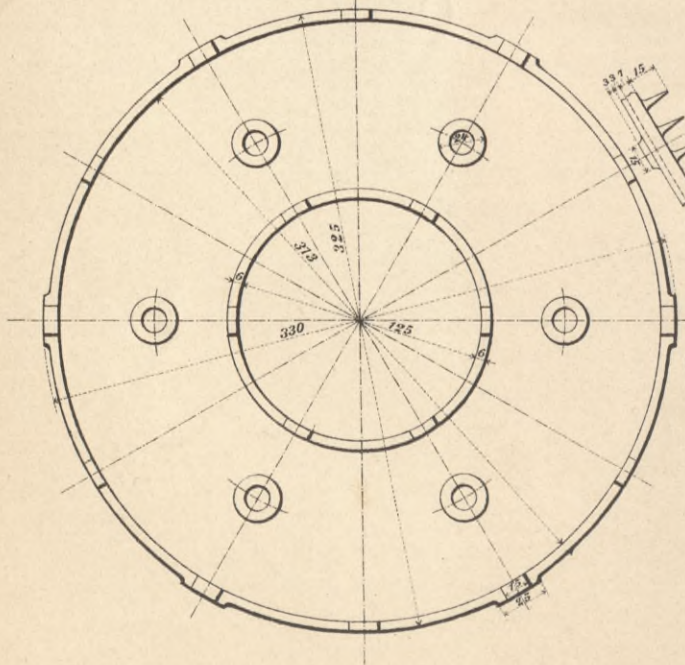
Fig. 185. Rückansicht der Zahnscheibe. 1:4.
