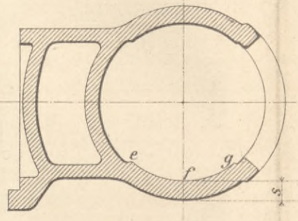
Schnitt: c d (Fig. 309, 311).
