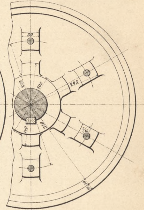
Kupplungshälfte für die Zahnscheibe. 1:4.
