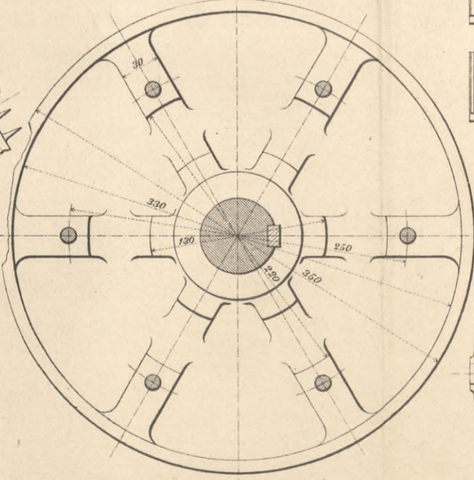
Fig. 186. Kupplungshälfte für die Bürstenscheibe. 1:4.
