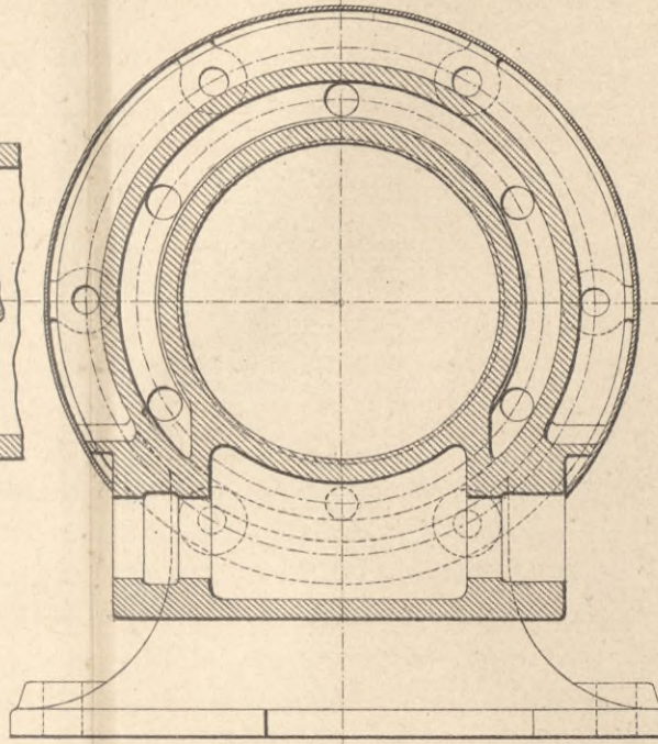
Fig. 380. Schnitt A B, in Richtung des Pfeiles gesehen. 1:10
