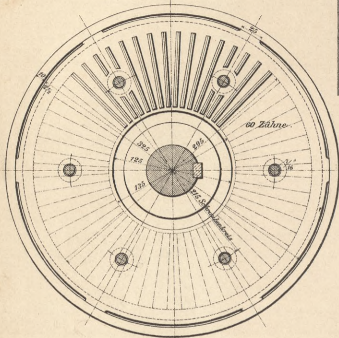
Fig. 185. Rückansicht der Zahnscheibe. 1:4.
