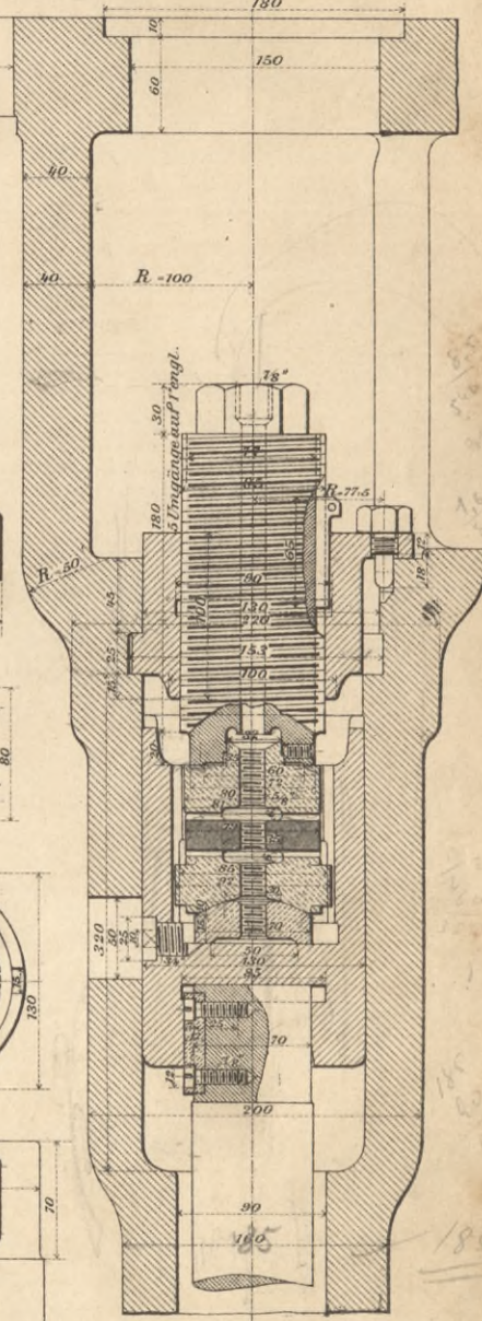
Fig. 217. Schnitt: a b c. 1:5.
