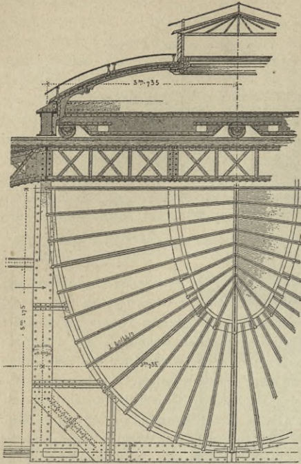
Vom Eden-Theater in Paris 121) , \frac{1}{100} n. Gr.
