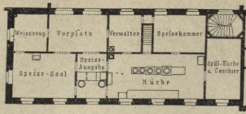
Speisehaus im Arbeiterdörfchen bei Stuttgart 91) .
