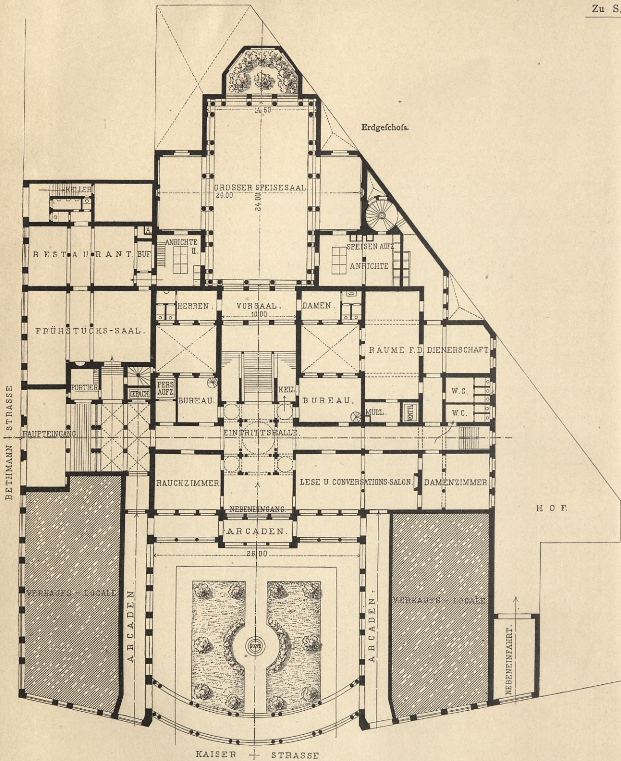
Hotel „Frankfurter Hof“ in Frankfurt a. M.
