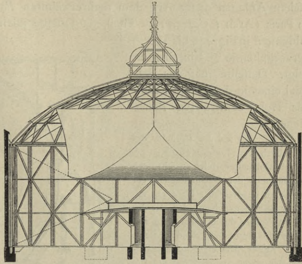
Fig. 446. Durchschnitt.
