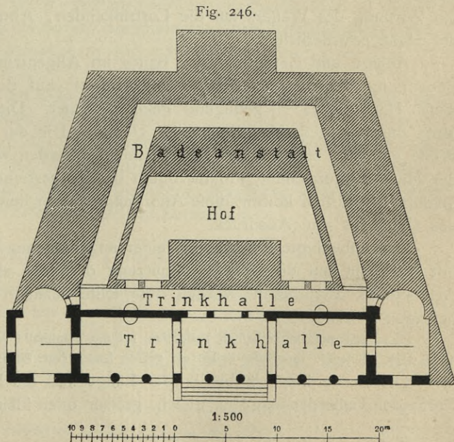
Trinkhalle der Cur- und Bade-Anstalt zu Ragatz 217) .
