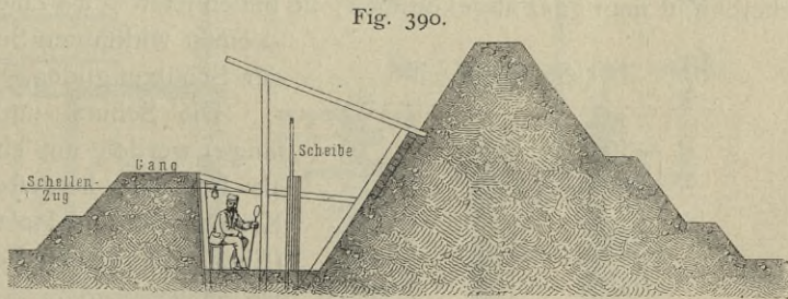
Scheibenstand vom Schützenfest in Frankfurt a. M. 1862 362) .
