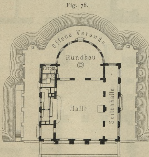
Alter-Pavillon zu Hamburg 61) .
