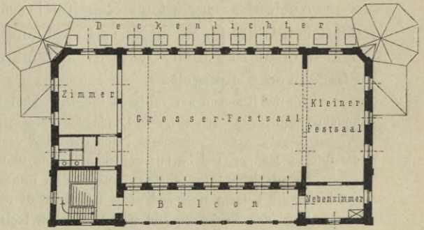
Fig. 408. Obergefchofs.
