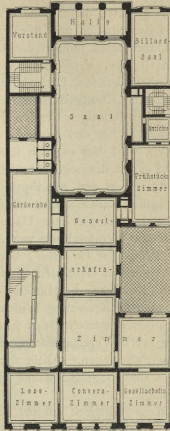
Haus der Kaufmännischen Ressource in Berlin 314 ).
