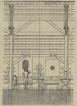
Fig. 372. Längenschnitt.
