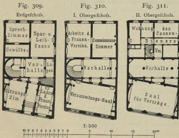
Haus der Gesellschaft freiwilliger Armenfreunde in Kiel 324 ).
