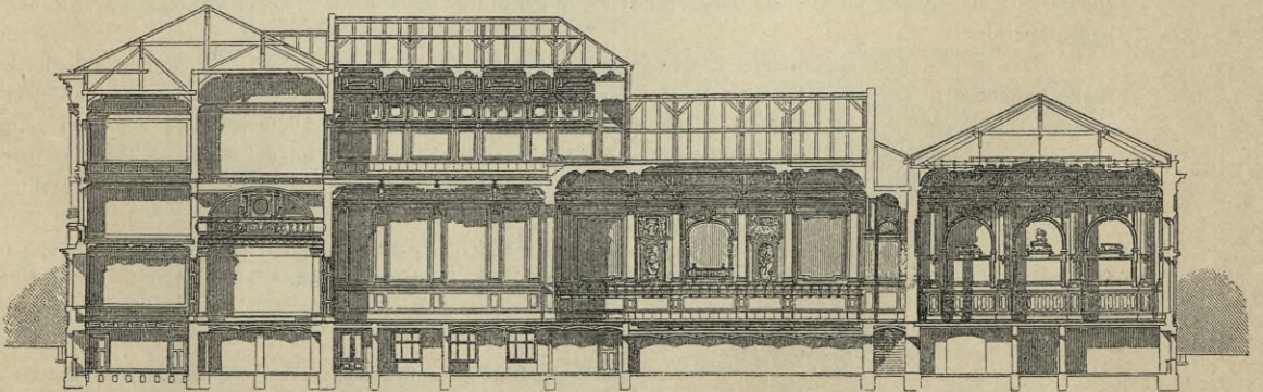
Haus der Loge Royal York in Berlin 286)
