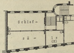
Fig. 230. IV. Obergefchofs.
