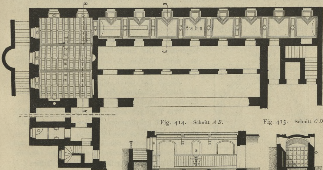
Fig. 413. Grundriss.
