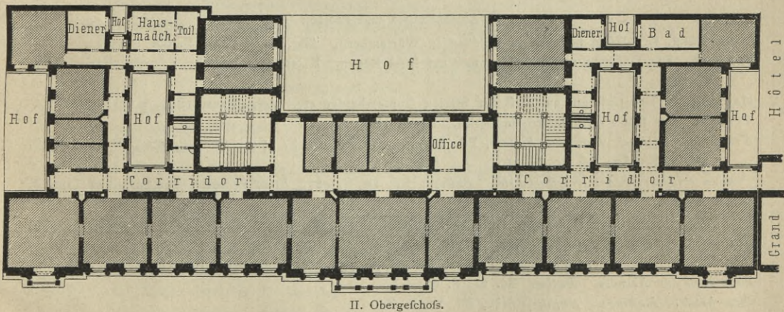
II. Obergechoß. Hôtel garni in Wien 177) . Arch.: C. Tiets .
