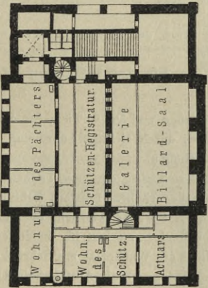
Fig. 395. Zwischengeschoss.
