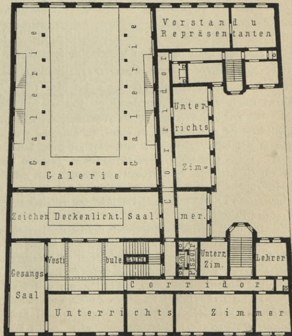
Haus des Berliner Handwerker-Vereines 319) .
