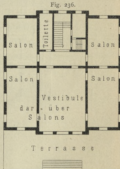
Casino-Gebäude der Actien-Bade-Anstalt zu Kiffingen 207 ). — 1/500 n. Gr.
