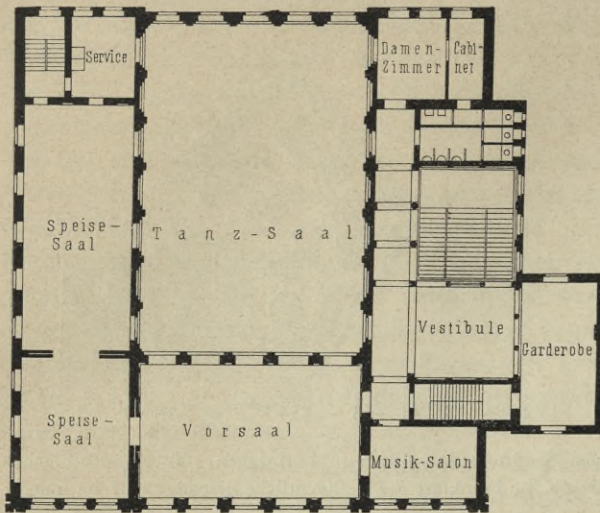
Hauptgefchofs zu Fig. 256 239 ). — 1/500 n. Gr.
