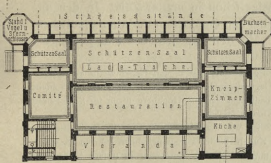
Fig. 407. Erdgefchofs.
