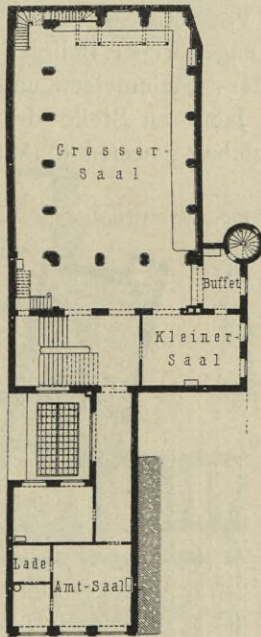
Fig. 285. I. Obergeschoss.
