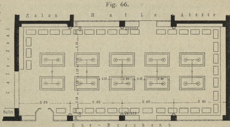
Vom Café du libre échange in Paris 45) . — \frac{1}{250} n. Gr.
