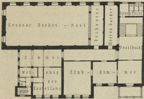
Fig. 278. Zwischengeschofs.
