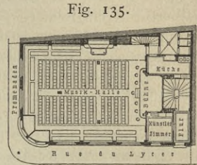
Cafino zu Troyes 115) . 1/500 n. Gr. Arch.: Fontaine.
