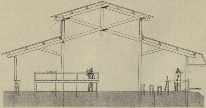
Fig. 371. Querschnitt.
