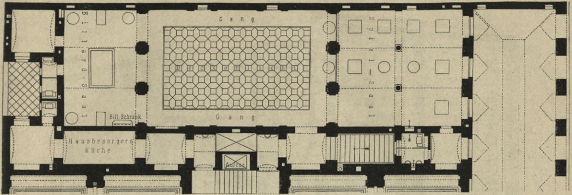
Zwischengechofs.
