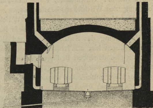
Weinkeller 22) . — 1/125 n. Gr.
