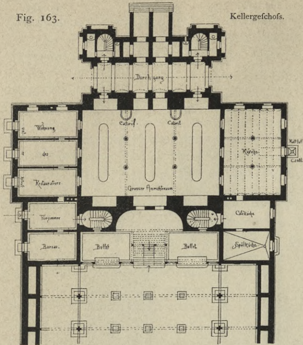
Festhalle in Karlsruhe. — \frac{1}{500} n. Gr.
