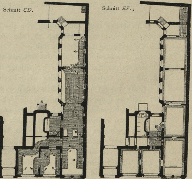
Lüftungs-Anlage im Siechen'schen Restaurant zu Berlin 12) .
