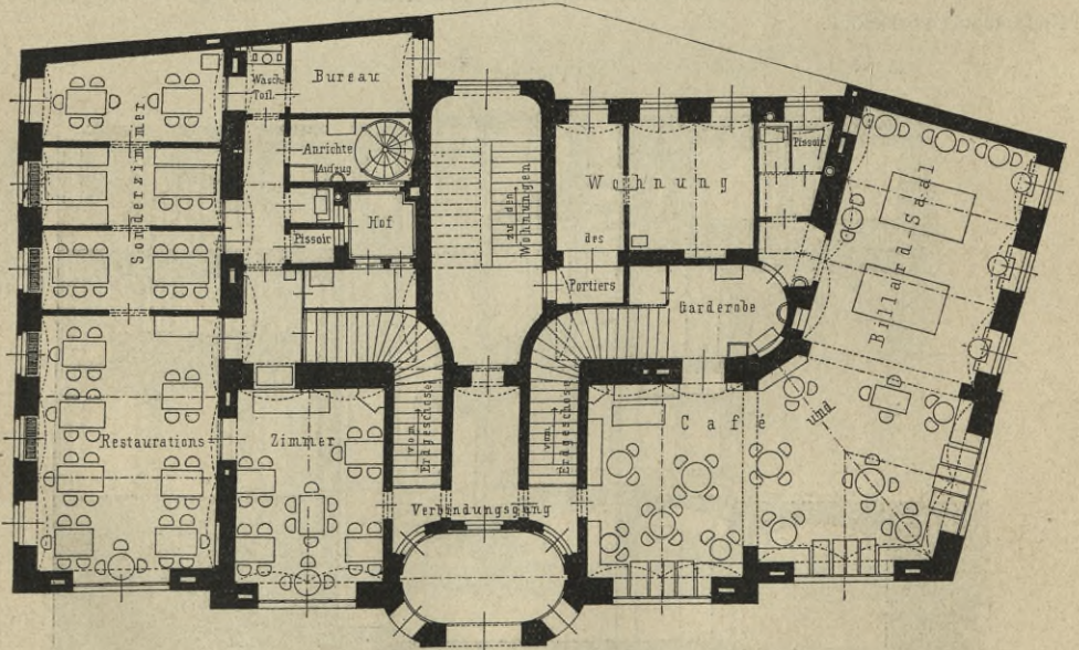
Obere Abteilung des Erdgeschosses.
