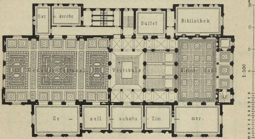
Fig. 259. Obergeschoss.
