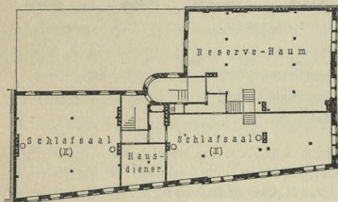
Fig. 231. Dachgefchofs.
