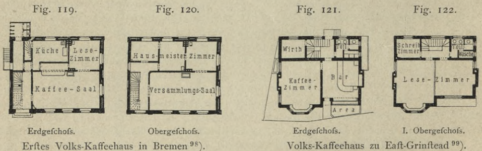
Erstes Volks-Kaffeehaus in Bremen 98) .
