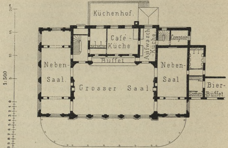
Restaurations-Gebäude im zoologischen Garten zu Hamburg 65 .
