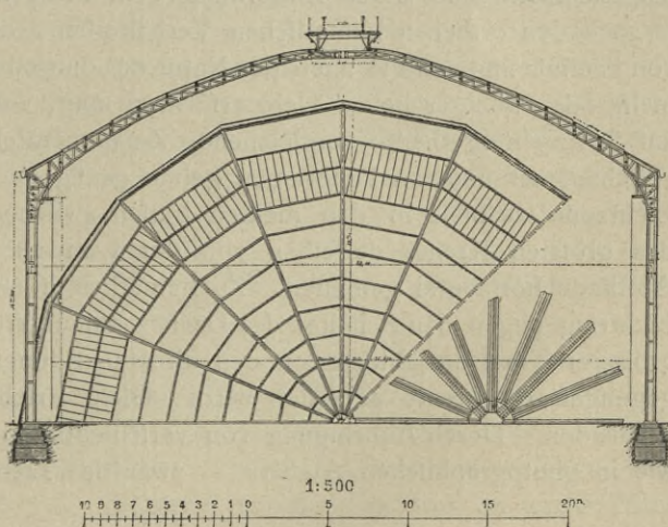
Panorama zu Genf 402) .
