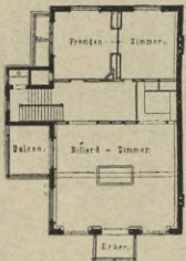
Fig. 83. Obergeschoss.
