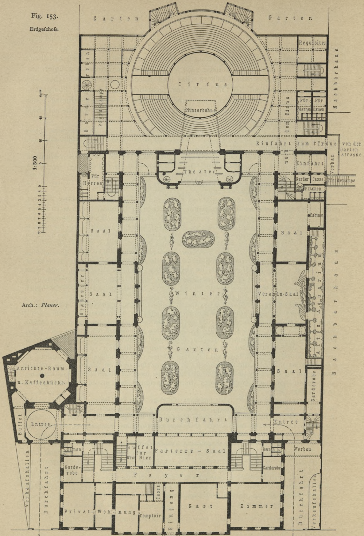
Kry stall-Palast in Leipzig 136).
