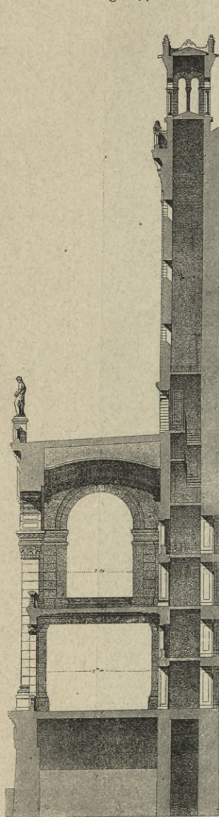
Trocadéro-Palast in Paris 150) .
