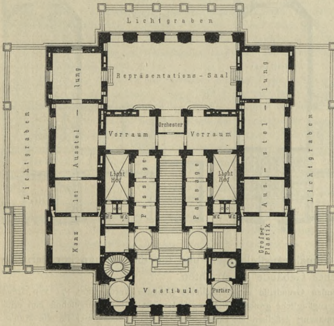
Fig. 348. Erdgeschoss.
