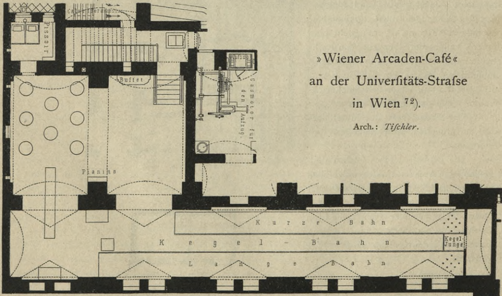
Theil des Kellergeschoßes.
