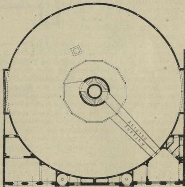
Fig. 447. Grundriss.
