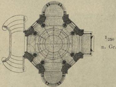
Schnitt und Grundriss zu Fig. 476 439) .
