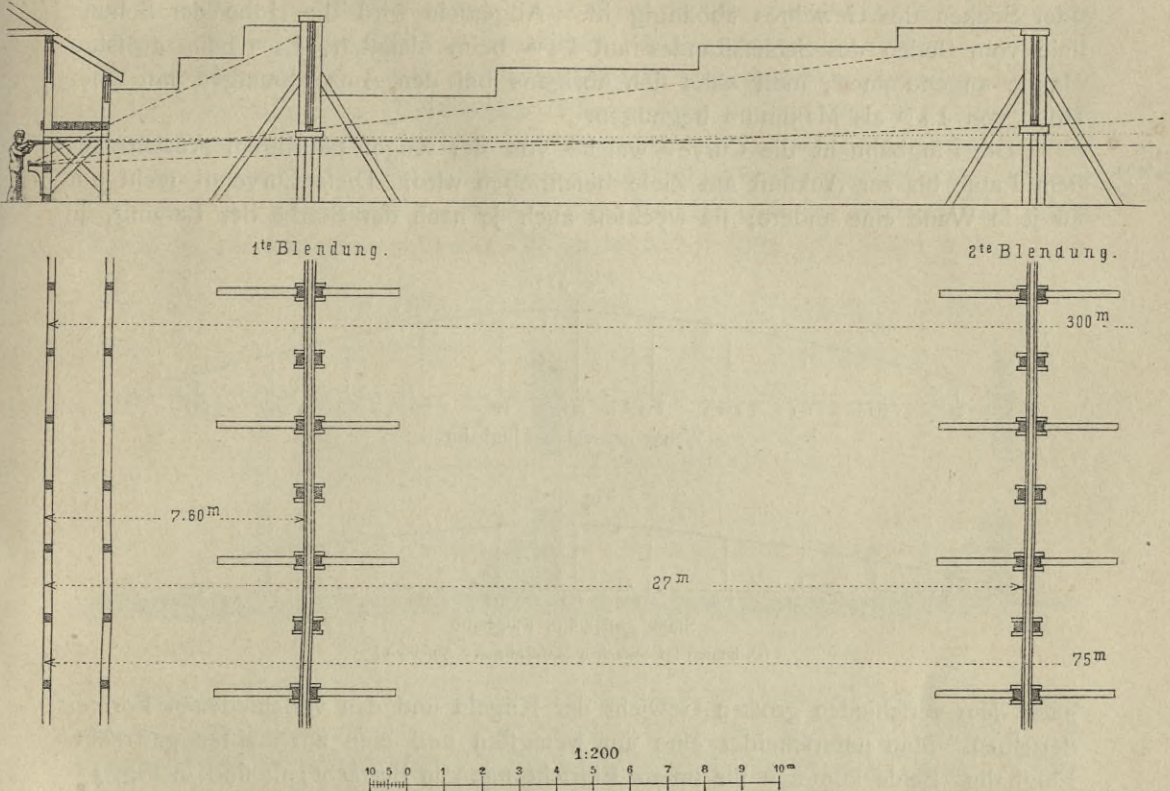
Theil des Schiefsfeldes und Schiefsstand vom eidgenössischen Schützenfest zu Zürich 1872 361) .
