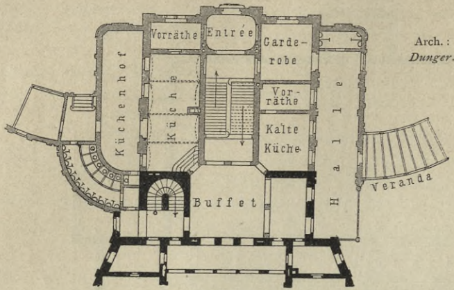
Erdgeschoss — Anbau.
