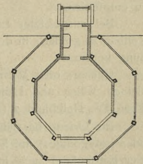
Grundriß zu Fig. 471 437 ).
