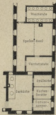
Speisehaus der Zeche Hamburg bei St. Annen 87) .
