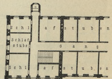
Obergeschoss.
