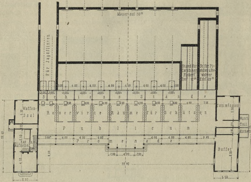
Fig. 404. Erdgeschoss des Schießhauses.
