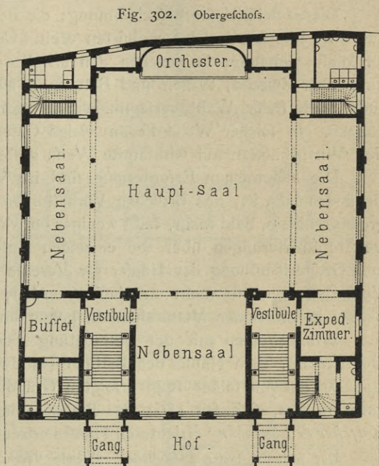
Gewerbehaus in Dresden 318 ). — 1/500 n. Gr.
