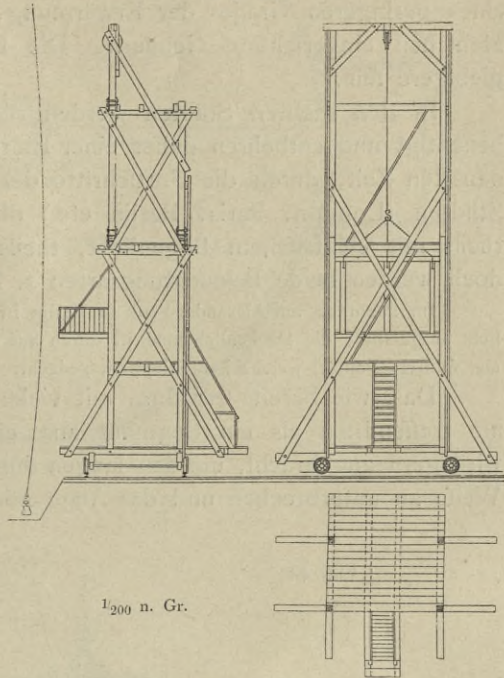
Malergeriüst (verwendet im Panorama zu München).
