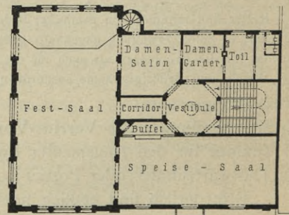
Fig. 254. Hauptgeschofs.
