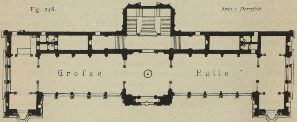
Grosse Halle des Friedrichsbades zu Baden-Baden 225) .
