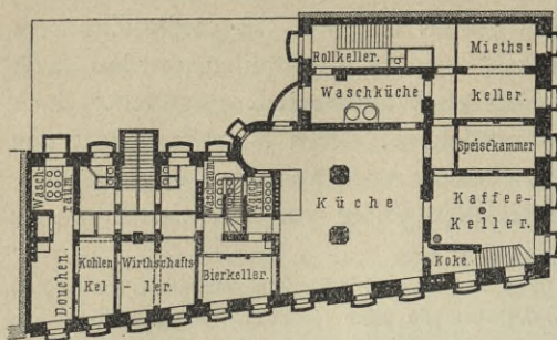
Fig. 228. Erdgefchofs.
