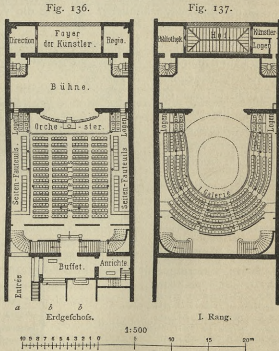
Concert de la Scala in Paris 116) . Arch.: Delarue.
