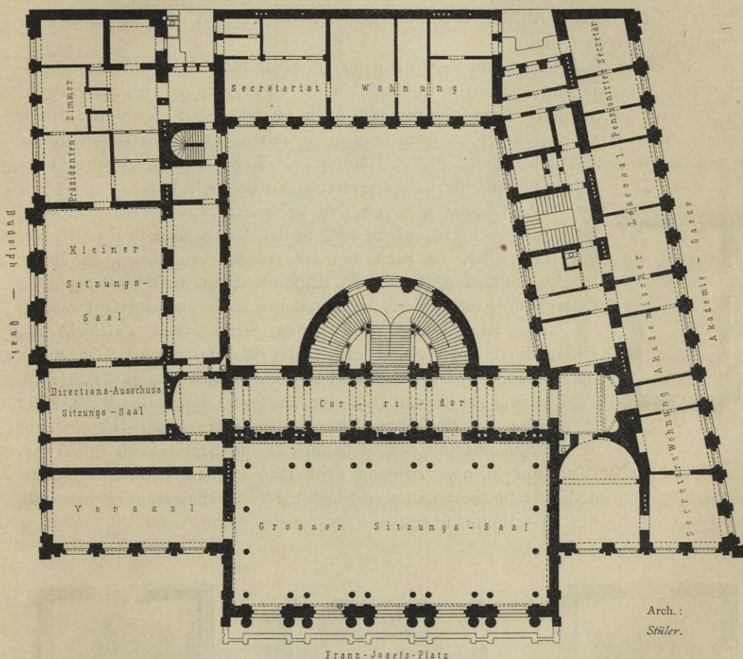
Fig. 315. Hauptgeschoß.
