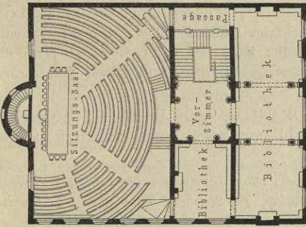
Fig. 339. Obergeschoss.
