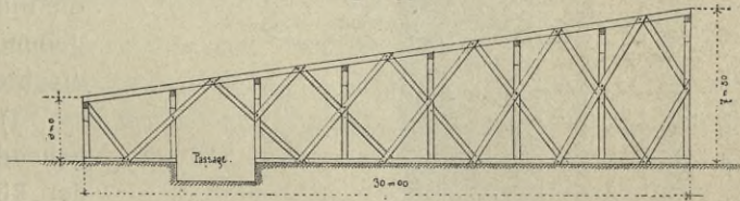
Schnitt durch das Podium. — 1/500 n. Gr.
