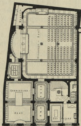
Fig. 334. Erdgeschoss.
