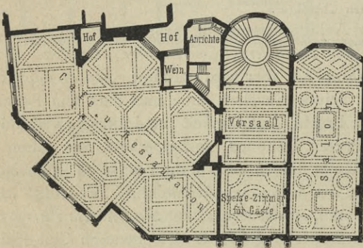
Fig. 270. II. Obergeschoss.
