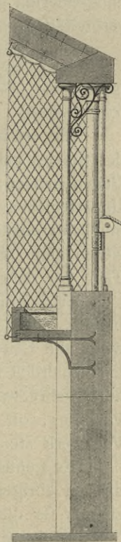
Schnitt durch die Galerie-Wand 392) . 1/25 n. Gr.
