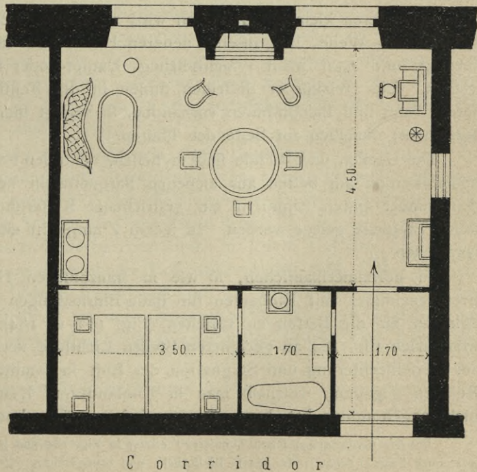
Fremdenzimmer in französischen Hotels.
