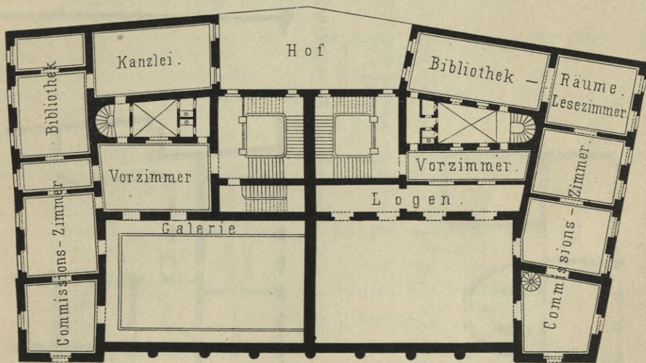
Fig. 297. II. Obergefchofs.
