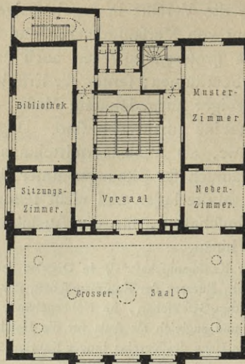
Fig. 292. Hauptgeschoss.
