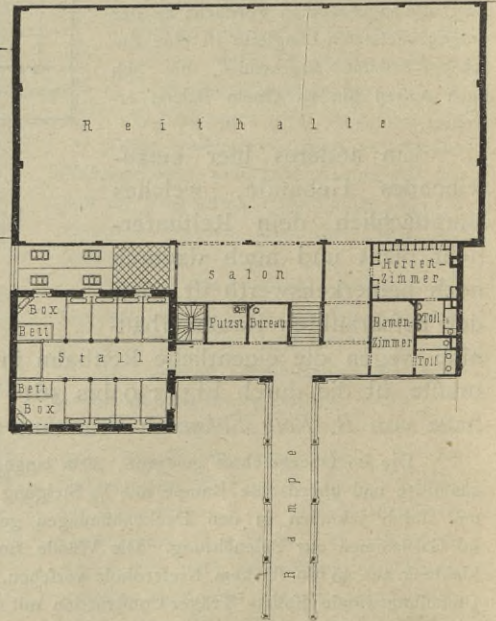
Fig. 361. Obergeschoß.
