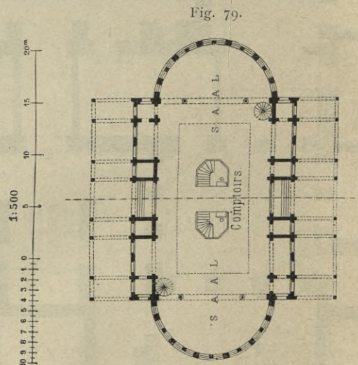
Restaurant Belge auf der Weltausstellung zu Paris 1878 62) .
