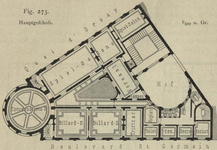
Haus des landwirthschaftlichen Vereins ( Cercle agricole ) zu Paris 263 ).
