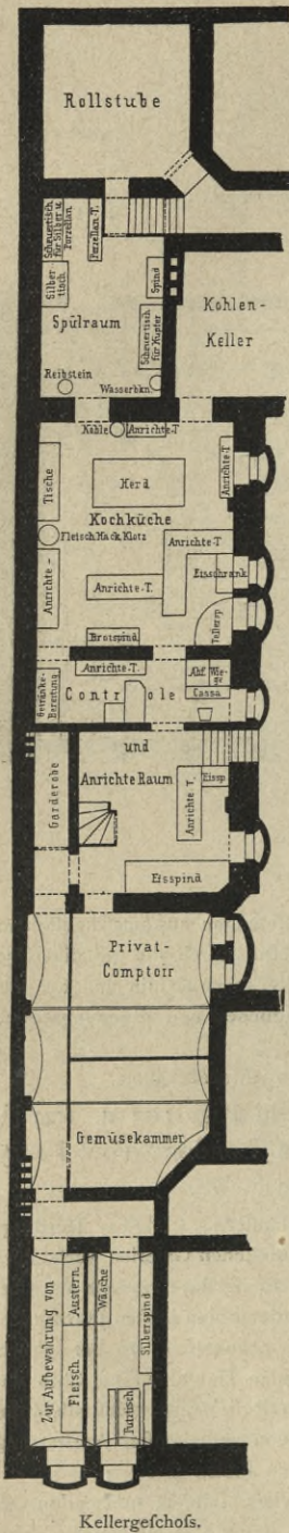
Kellergeschoß.
