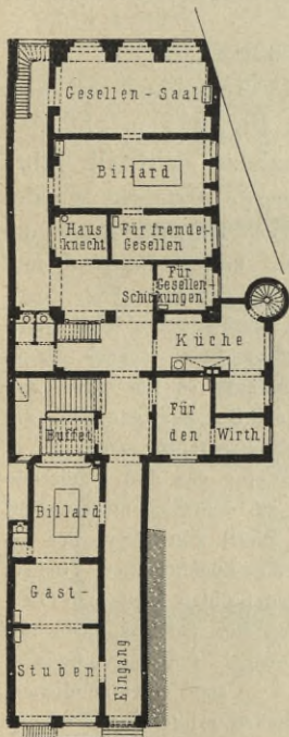
Fig. 284. Erdgeschoss.
