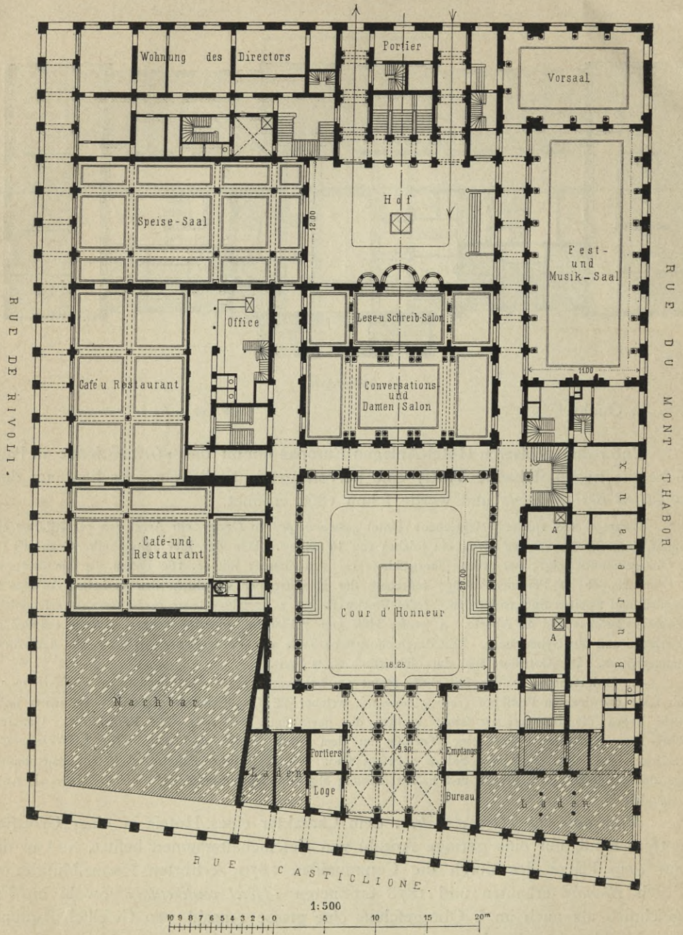
»Hôtel continental« in Paris. — Grundrifs des Erdgeschosses 176 .
