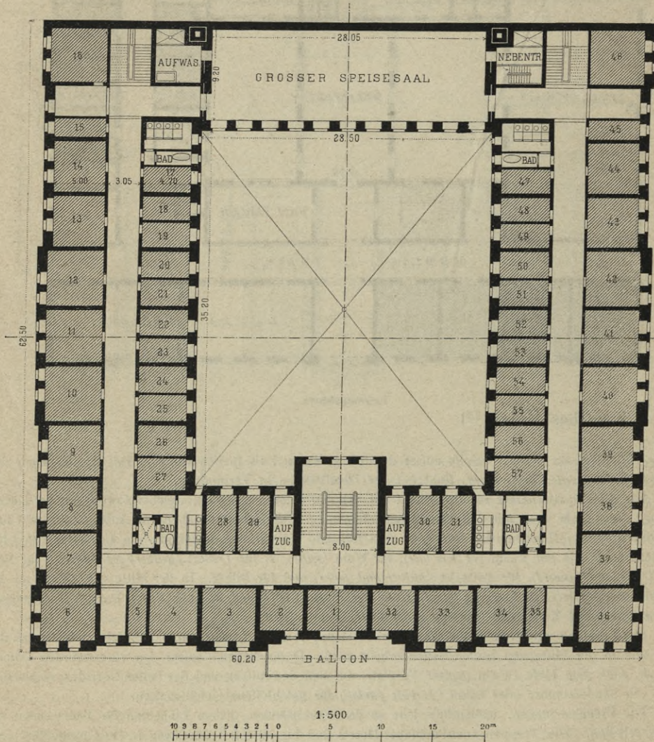
Stewart's Hotel für Arbeiterinnen in New-York. — I. Obergeschoss 169 ).
