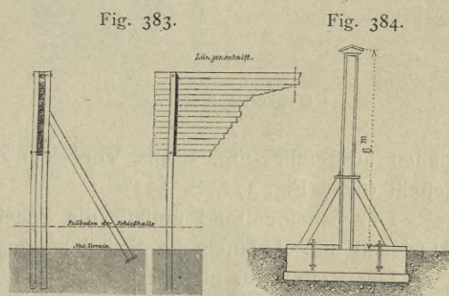
Holzblenden vom Schützenfest in Wien 1868 360 ).
