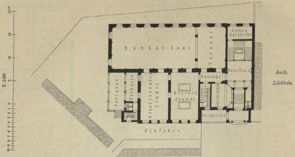
Fig. 277. Erdgeschoss.
