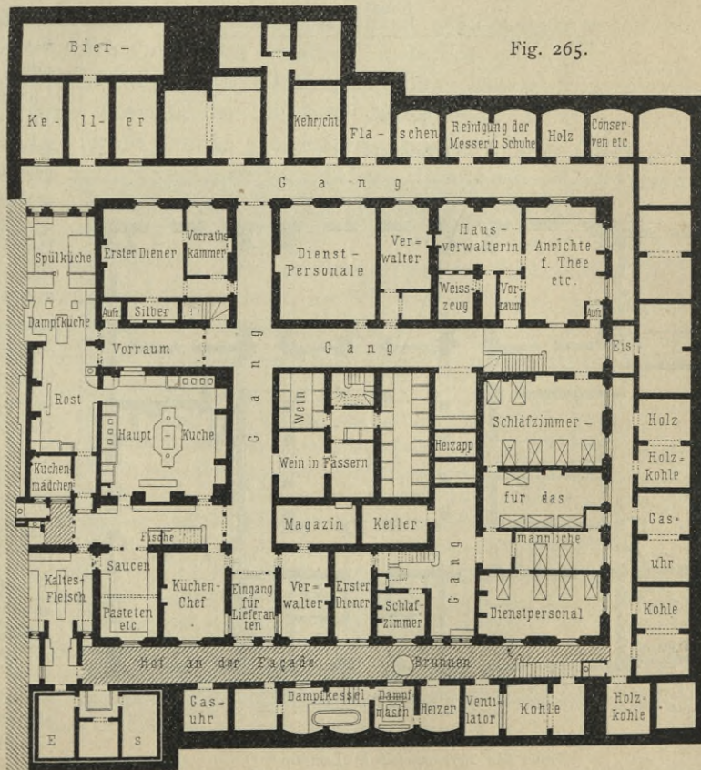
Kellergeschoß zu Fig. 266 u. 267 257 ). — 1/500 n. Gr.
