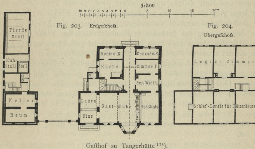
Gasthof zu Tangerhütte 178) .
