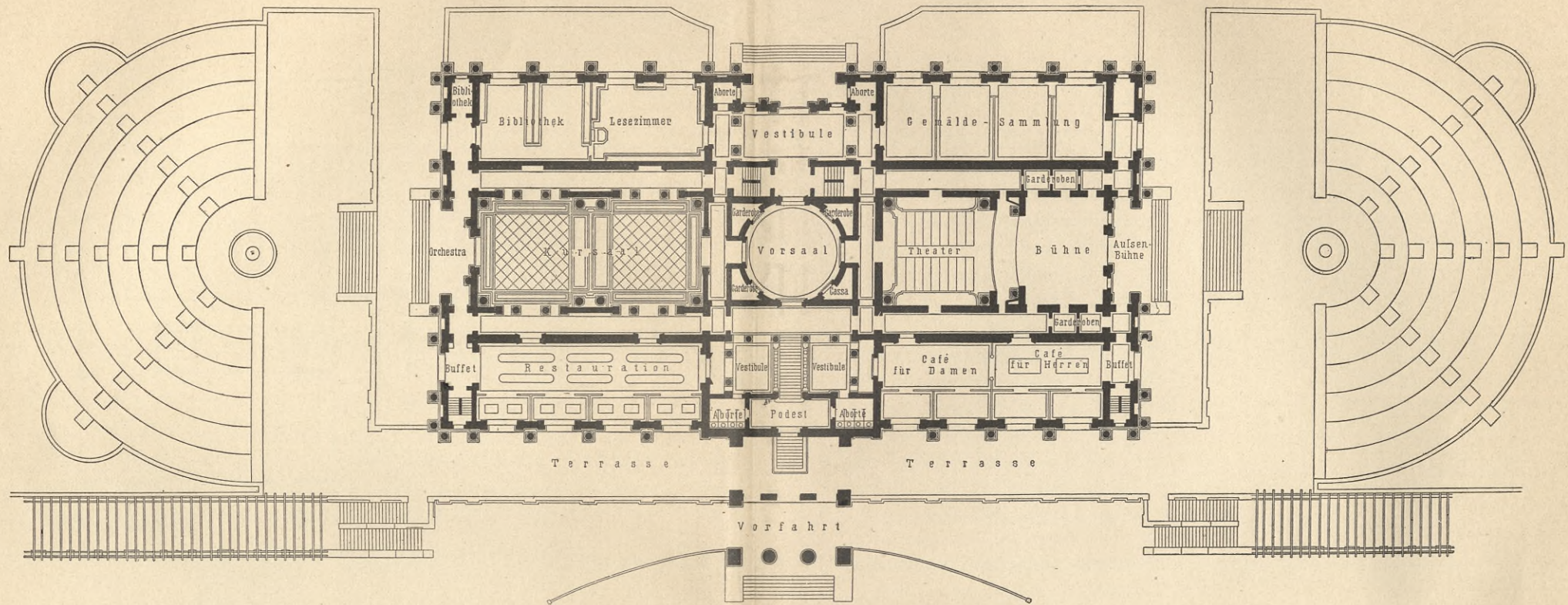
Semper's Entwurf zu einem Conversations-Haus zu Baden (Schweiz).
