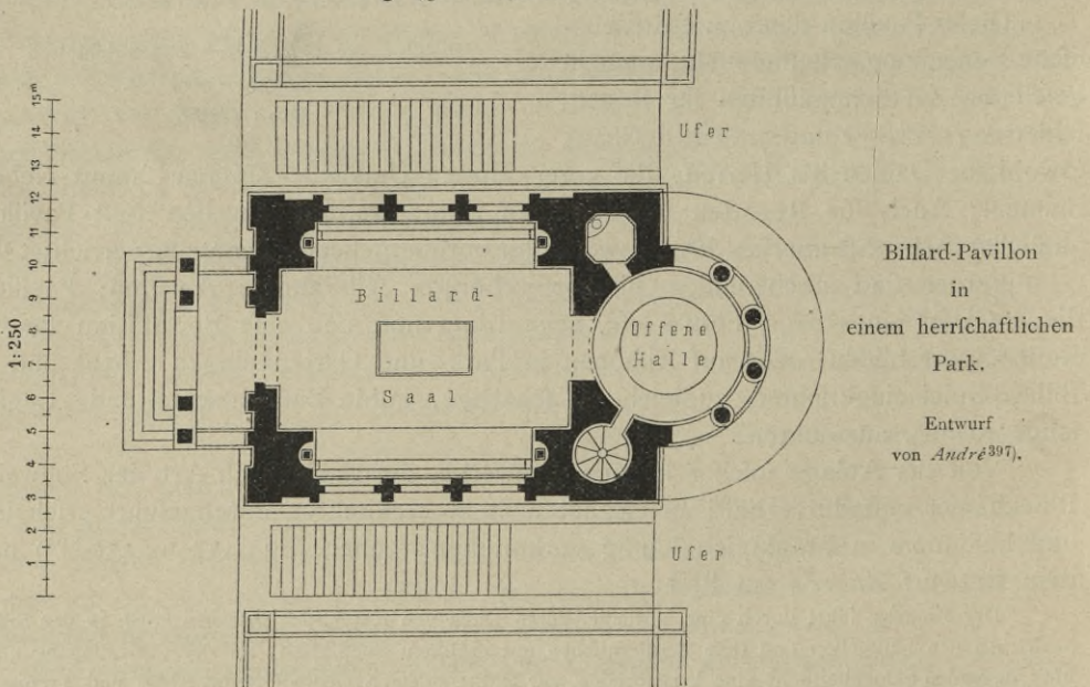
Fig. 436. Grundriss.
