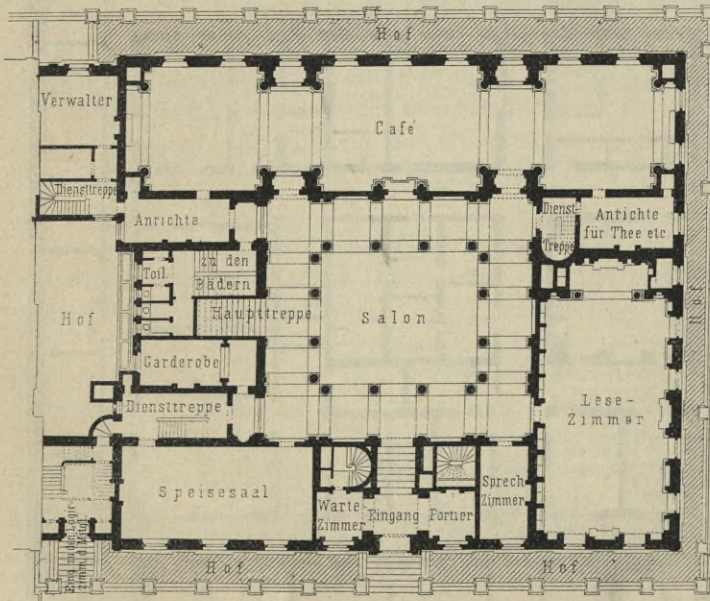
Haus des Reform-club in London 257 ).
