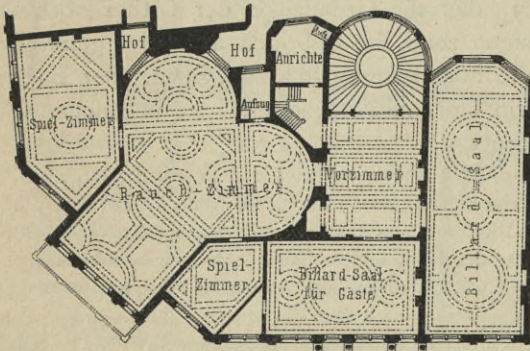
Fig. 270. II. Obergeschoss.
