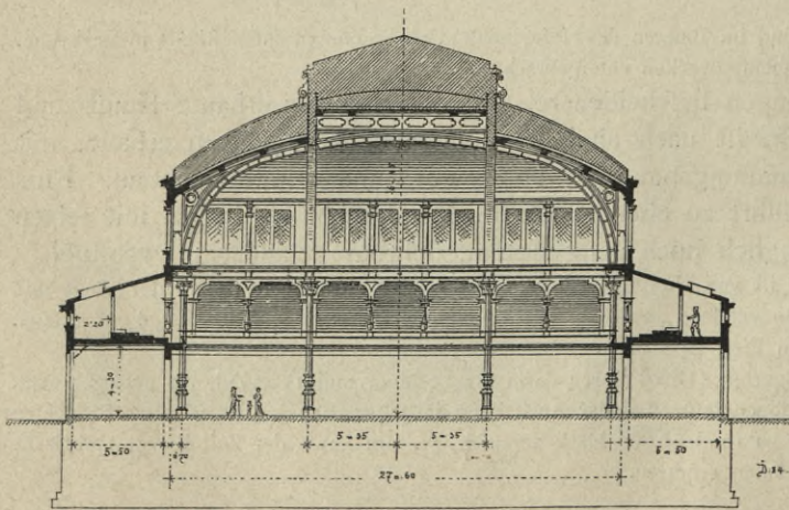
Querchnitt der Stadhalle in Mainz 145 ). — 1/500 n. Gr.
