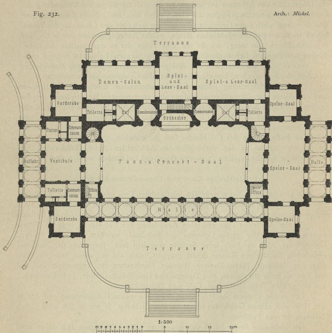
Cur-Saal in Ischl 202 ).
