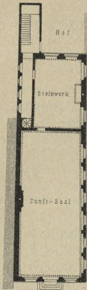
Kramer-Amtshaus zu Münster i. W. 301) 1500 n. Gr.
