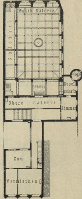
Fig. 286. II. Obergeschoss.
