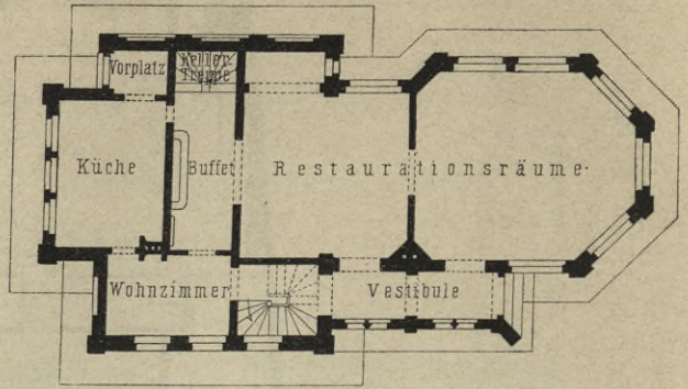
Restaurations-Gebäude des Bahnhofes Almelo 67) .
