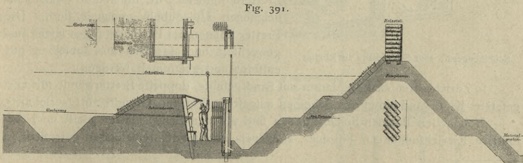
Scheibenstand vom Schützenfest in Wien 1868 359) .
