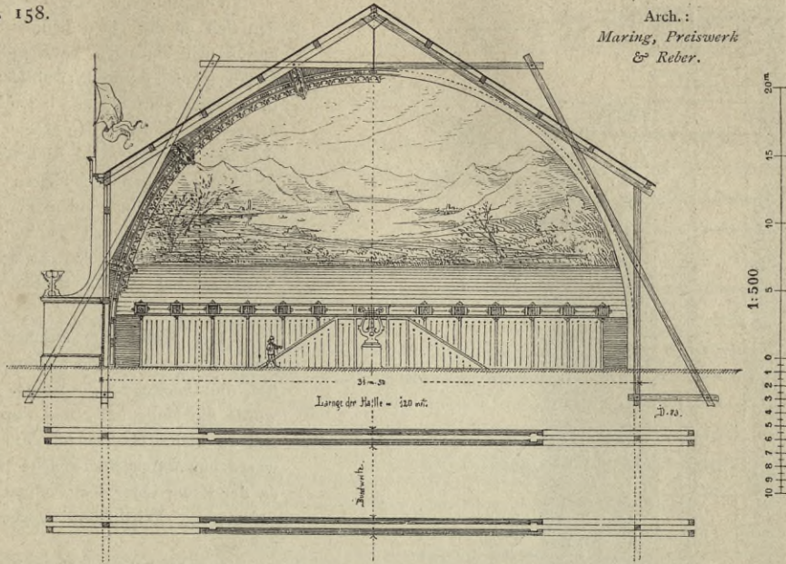
Querchnitt durch die Halle für das Sängertfest in Basel 1875.
