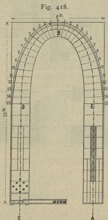
Kiebits's Rundkegelbahn 375) . 150 n. Gr.
