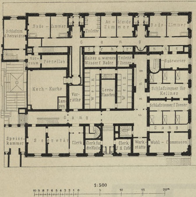
Fig. 266. Sockelgefchofs.
