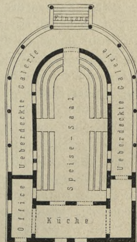
Arbeiter-Speisehaus zu Petersburg 95) .
