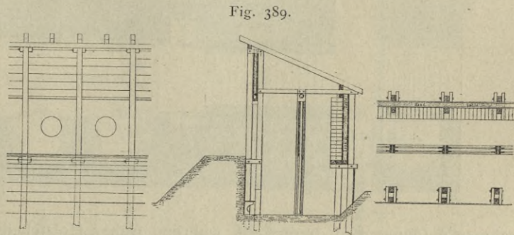
Scheibenstand vom eidgen. Schützenfest in Zürich 1872 361) .
