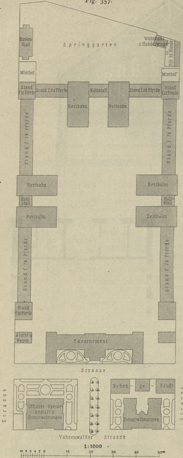
Militär-Reit-Institut zu Hannover 348 ).
