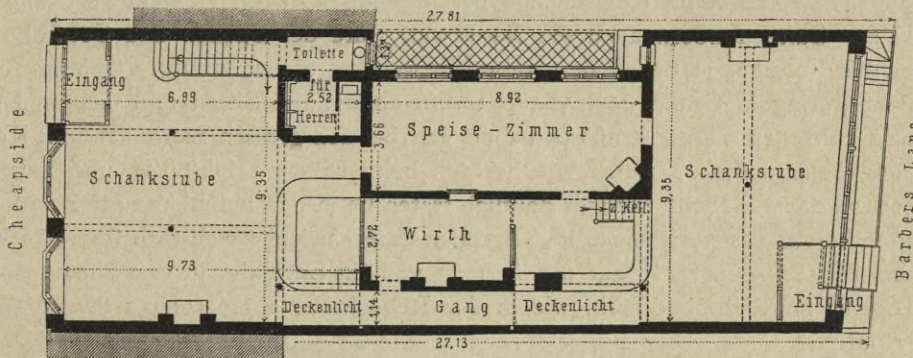
Fig. 47. Obergeschloß.
