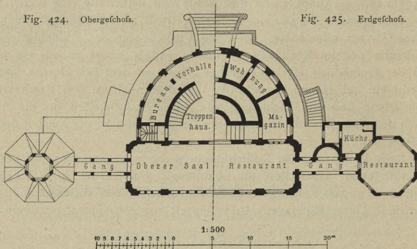
Pavillon des Budapester Eislauf-Vereins 378) .
