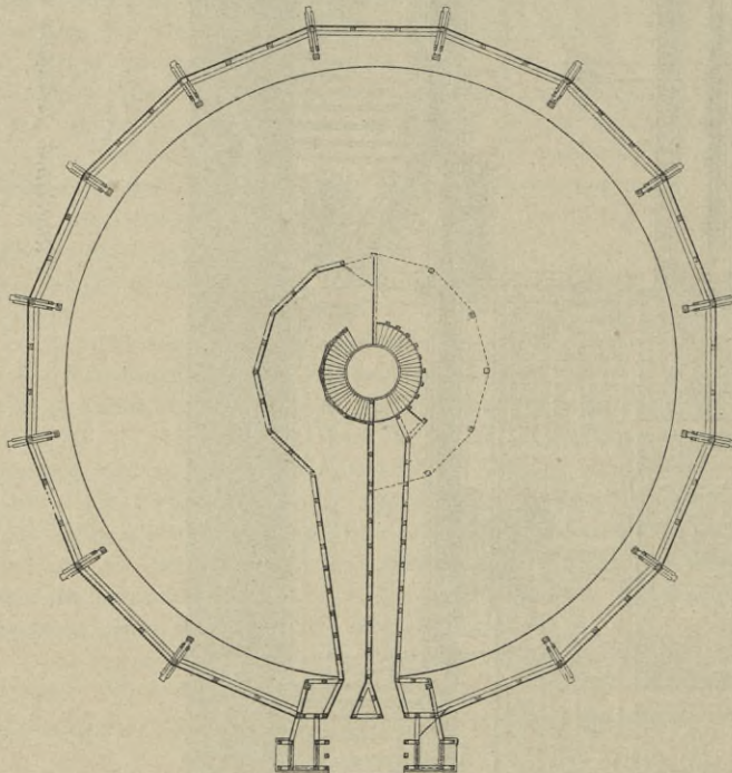
Fig. 453. Grundriss.
