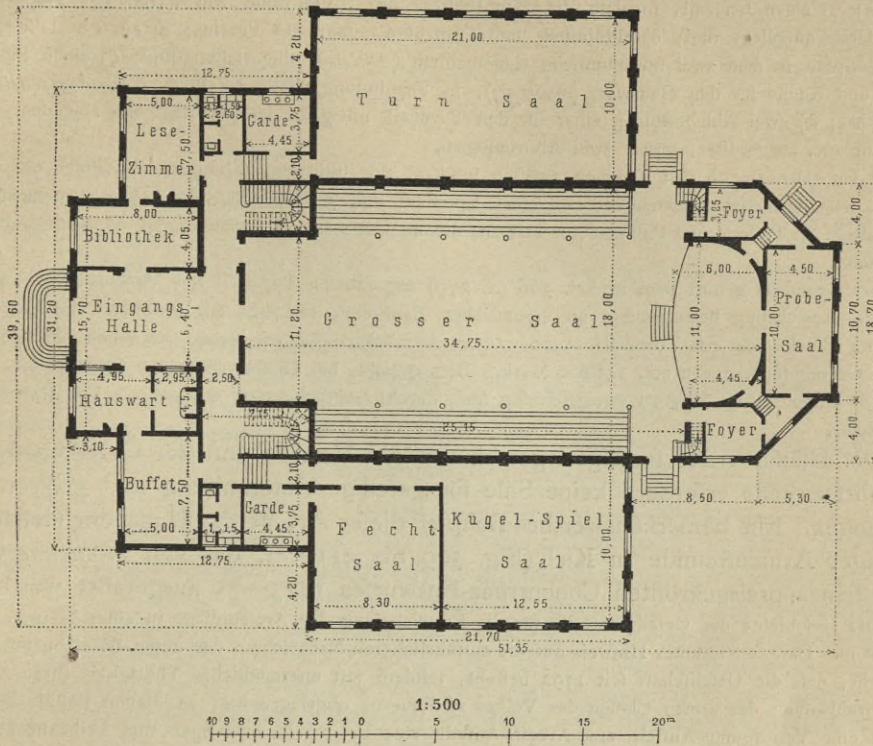
Fig. 307. Erdgeschoss.
