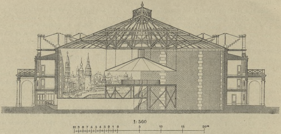
Querschnitt zu Fig. 437: Hittorf's Panorama in Paris 400) .
