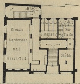
Fig. 293. Zwischengeschofs.
