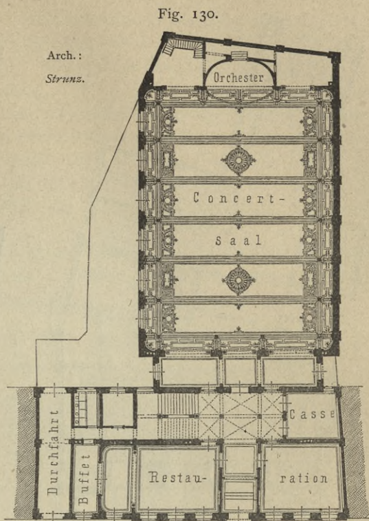
Victoria-Salon in Dresden 107) . — 1/500 n. Gr.
