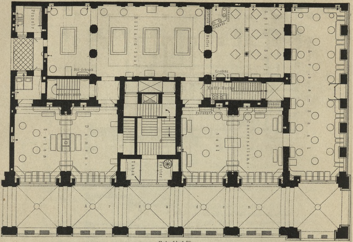
Erdgeschoss 71).
