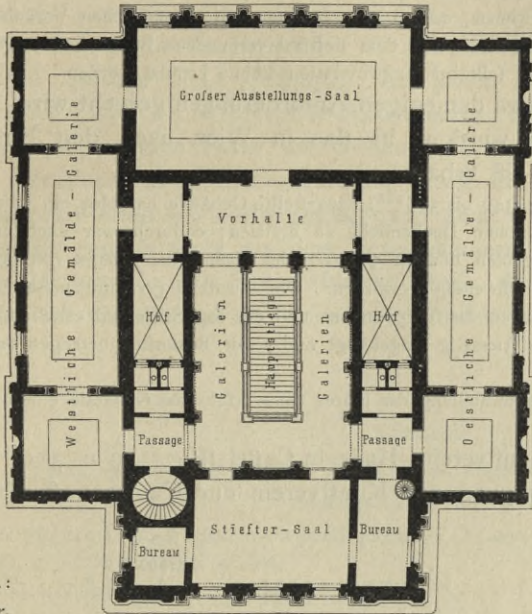
Fig. 348. Erdgeschoss.
