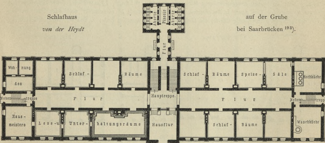
Erdgeschoß.
