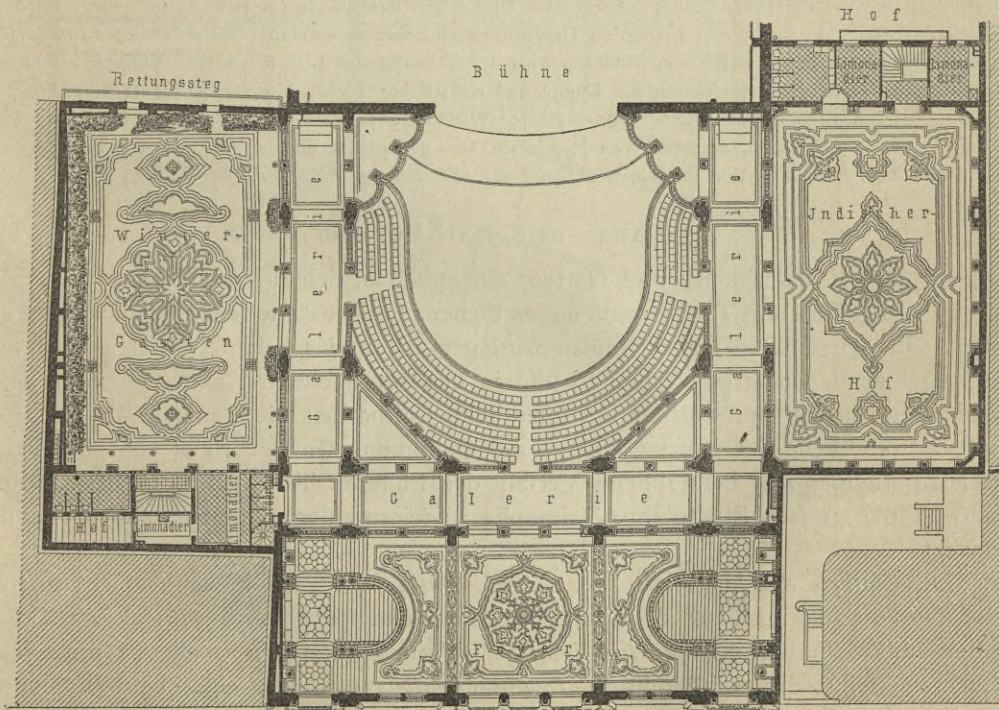
Fig. 143. Hauptgeschofs.
