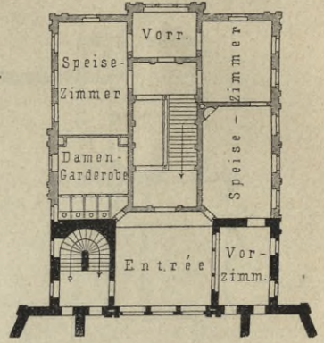
Obergeschoss — Anbau.
