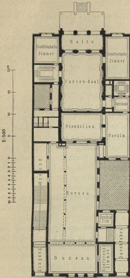
Haus der Kaufmännischen Ressource in Berlin 314 ).
