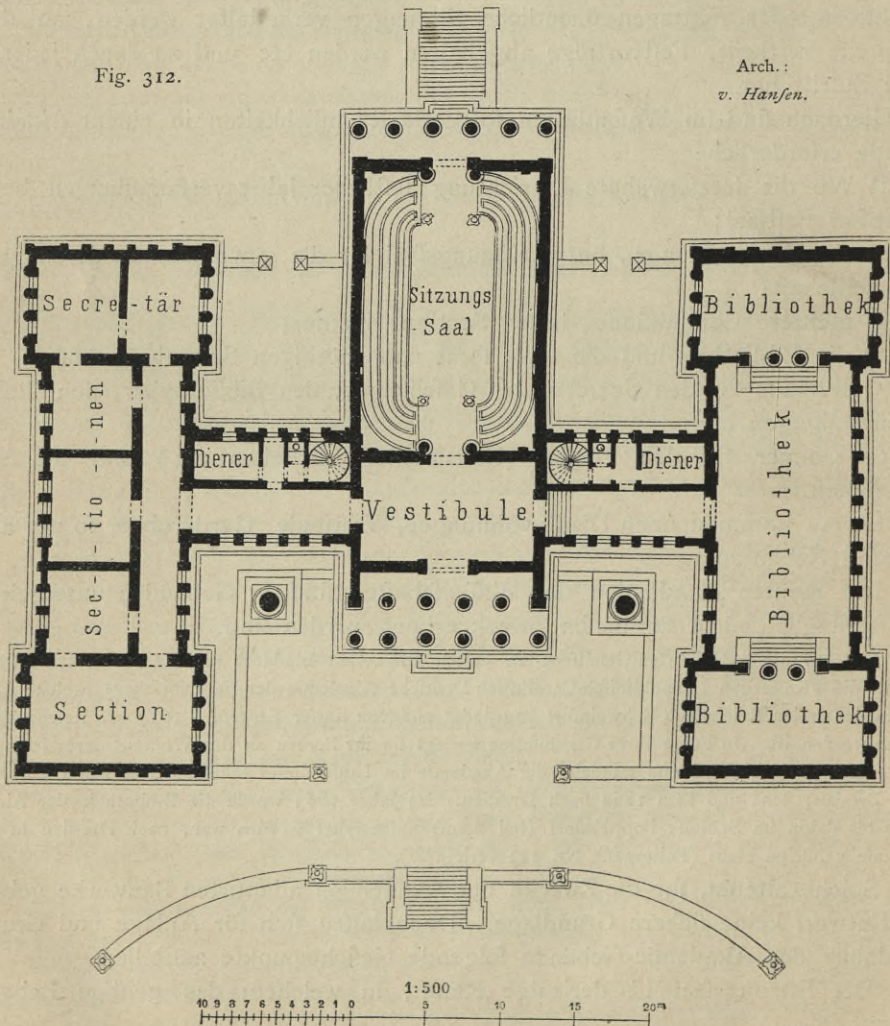
Akademie der Wissenschaften zu Athen 327 ).
