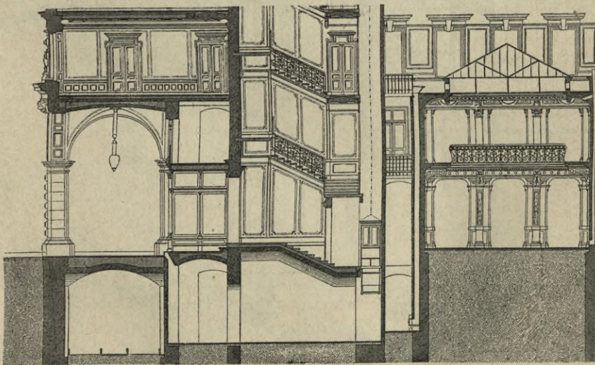
Querchnitt 73) .
