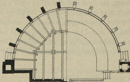
Fig. 456. Grundriß 423) .
