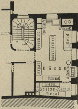
Küche der Bierstube »Zur Stadt Ulm« in Frankfurt a. M. — 1/250 n. Gr.
