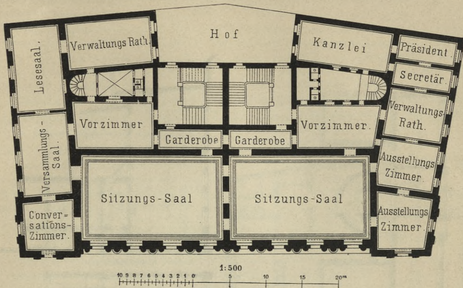
Fig. 297. II. Obergefchofs.
