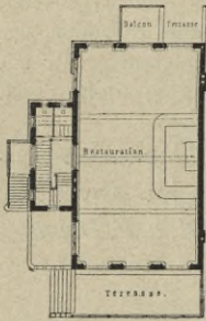
Fig. 83. Obergeschoss.
