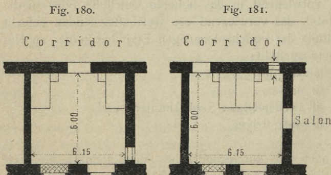
Fremdenzimmer in deutschen Hotels. — \frac{1}{250} n. Gr.
