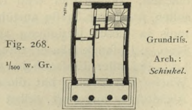
Ehemalige Wache am Potsdamer Thor zu Berlin 104 .
