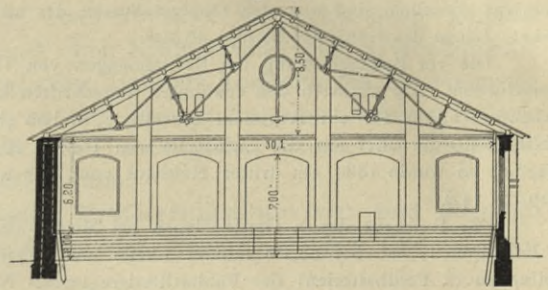
Querschnitt zu Fig. 258. — \frac{1}{500} w. Gr.
