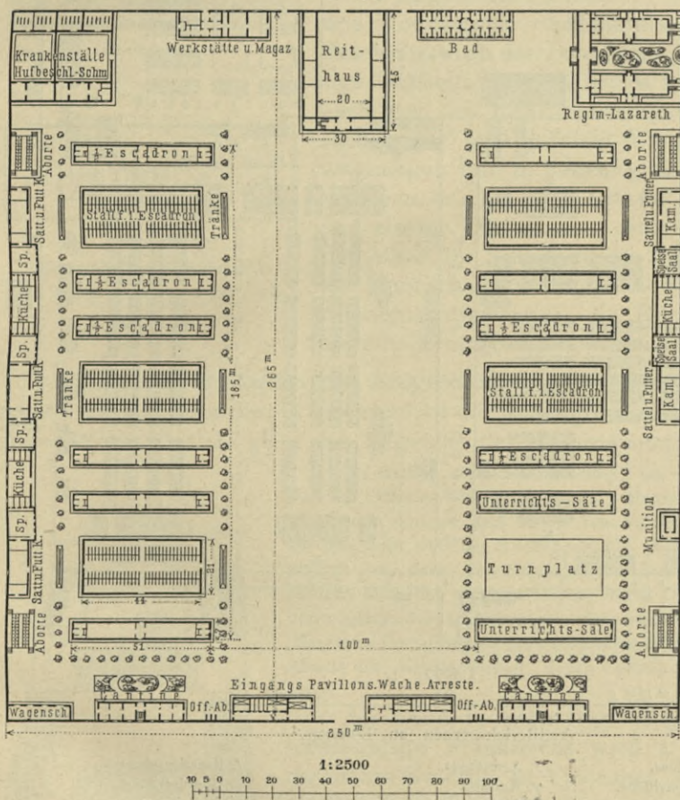
Tollet's Kaserne für ein Kavallerieregiment.
