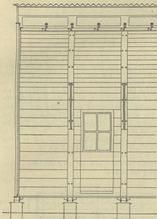
Längenschnitt. — \frac{1}{50} w. Gr.
