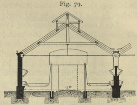
Stall für französische Kavalleriekasernen.
