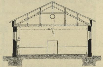
Querschnitt eines älteren Reithauses. 1/500 w. Gr.
