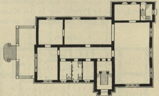
Offiziers-Speiseanstalt des 2. Eisenbahnregiments zu Berlin. 1/1000 w. Gr.
