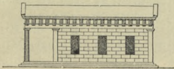
Ansicht. — 1/1000 w. Gr.
