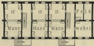
System der Militärquartierhäuser (Bataillonskasernen) zu Schwerin.
