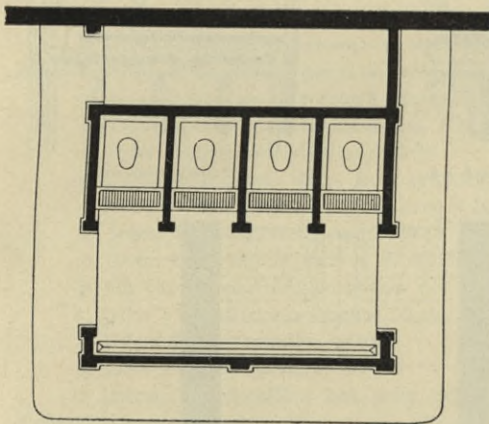
Tagesabort in französischen Kasernen.
