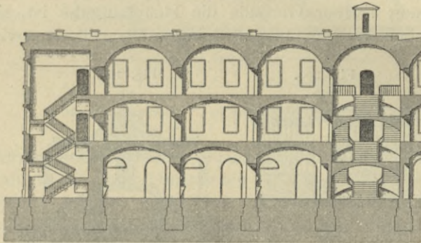
Schnitt GHH'.
