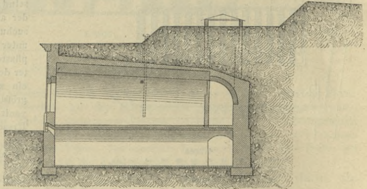
Querschnitt. — \frac{1}{350} w. Gr.
