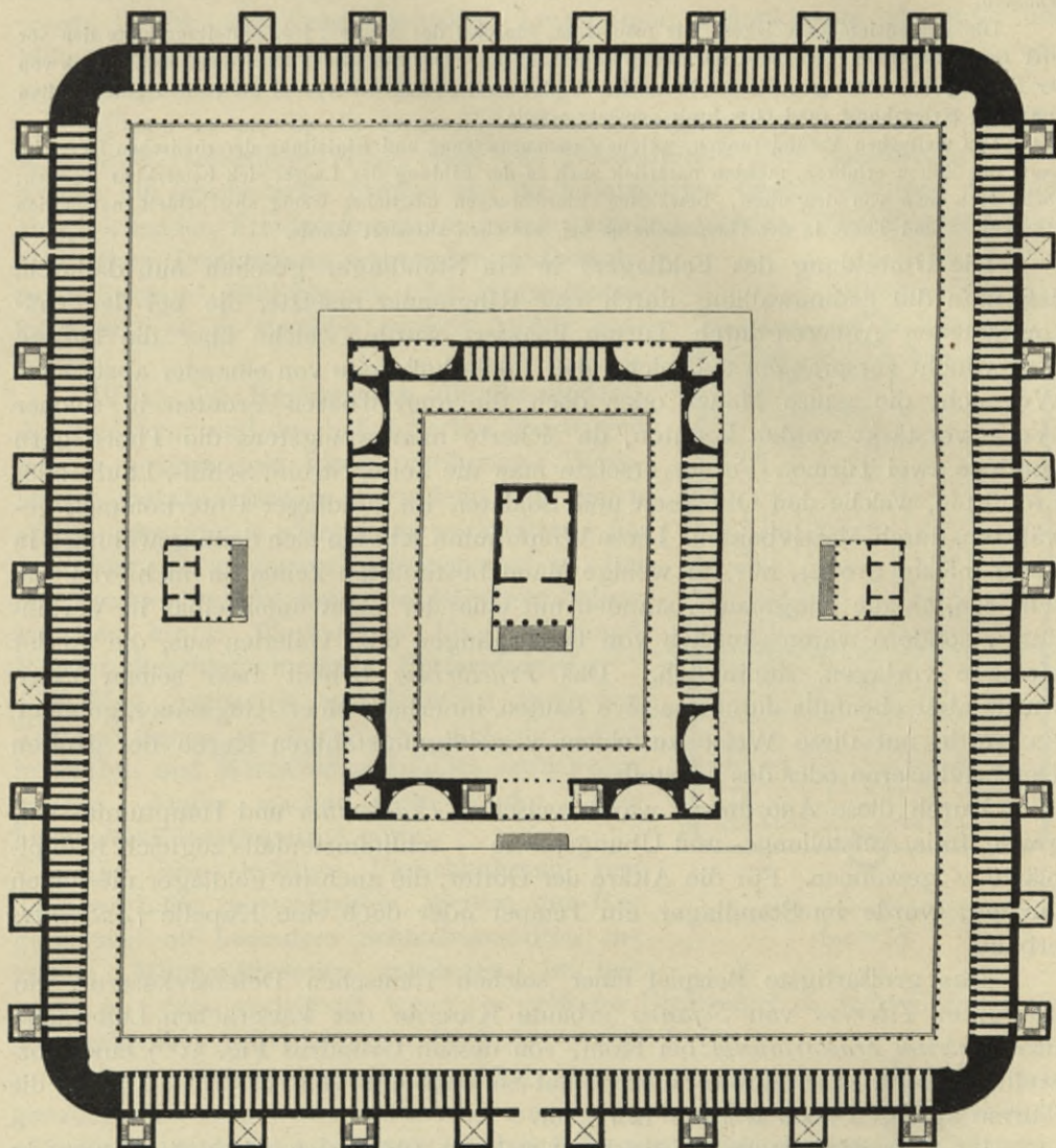
Castrum praetorianum bei Rom 01 ). — \frac{1}{3000} w. Gr.
