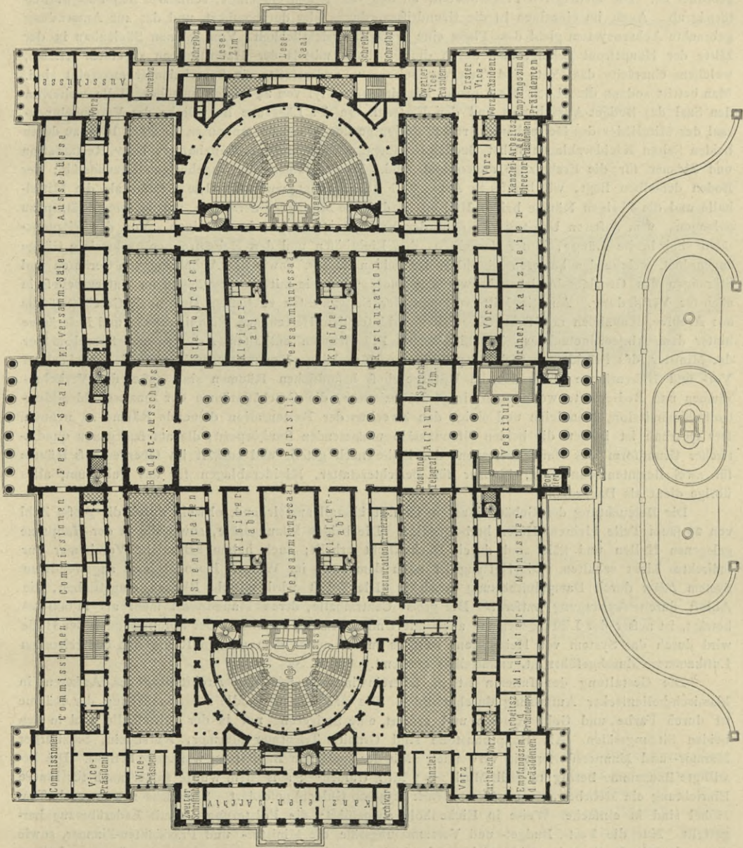
Reichsratshaus zu Wien (48).
