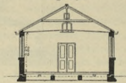
Querschnitt. — 1/250 w. Gr.
