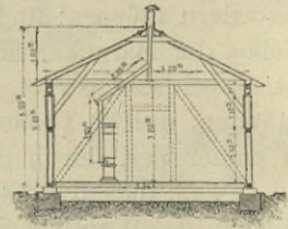
Hölzerne Mannschaftsbaracke.
