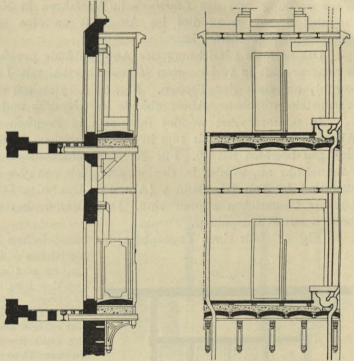
Schnitt nach c d.
