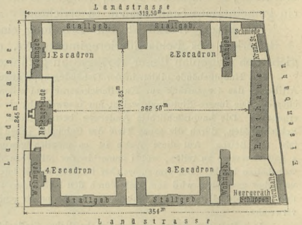
Kaserne für 4 Eskadronen Kavallerie zu Großenhain. 1/5000 w. Gr.
