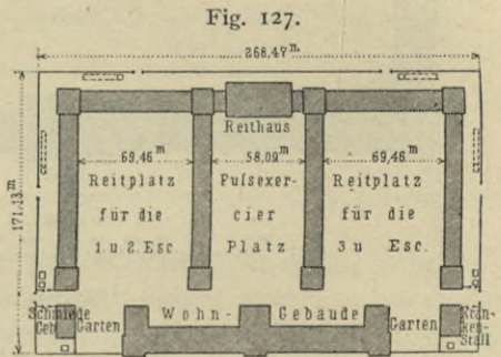
Kaserne für das 2. Garde-Ulanenregiment zu Moabit 138) . — \frac{1}{5000} w. Gr.
