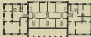
Hauptwache zu Dresden 103) .
