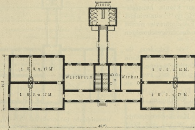
Mannschafts-Wohngebäude für 1 Eskadron. — Erdgeschoss 143) .
