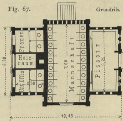
Fig. 67. Grundriss. Abortgebäude für ein Bataillon in preussischen Kasernen.
