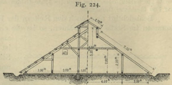
Hölzerne Stallbaracke. — \frac{1}{250} w. Gr.
