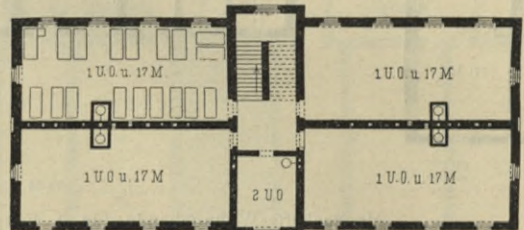
I. und II. Obergeschosß.
