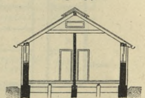
Querschnitt. — 1/250 w. Gr.
