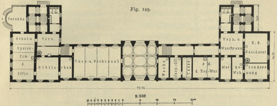
Stabsgebäude für eine österreichische Infanterieregiments-Kaserne 140) .
