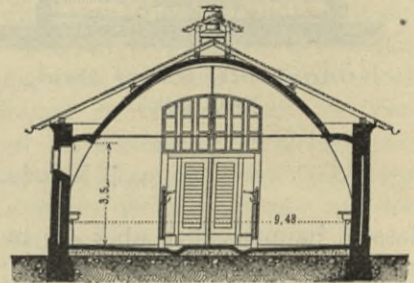
Stallsystem Gruber-Völckner .
