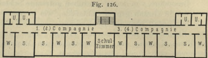
System der althannoverschen Kasernen (I. u. II. Obergeschofs).
