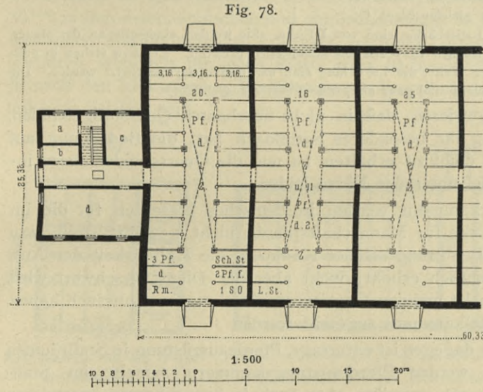
Österreichische Eskadronstallung 120) .
