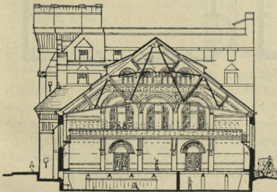
Querschnitt zu Fig. 251 u. 252.
