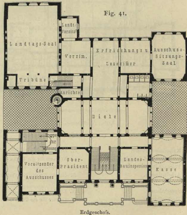
Landeshaus der Provinz Westpreußen zu Danzig 82) .
