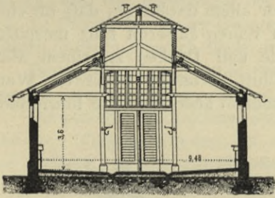
Österreichische Stallung älterer Konstruktion.
