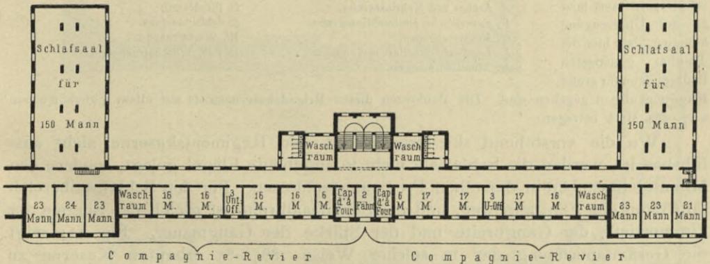
Linker Flügel (III. Obergeschoss). Infanterieregiments-Kaserne zu Dresden.
