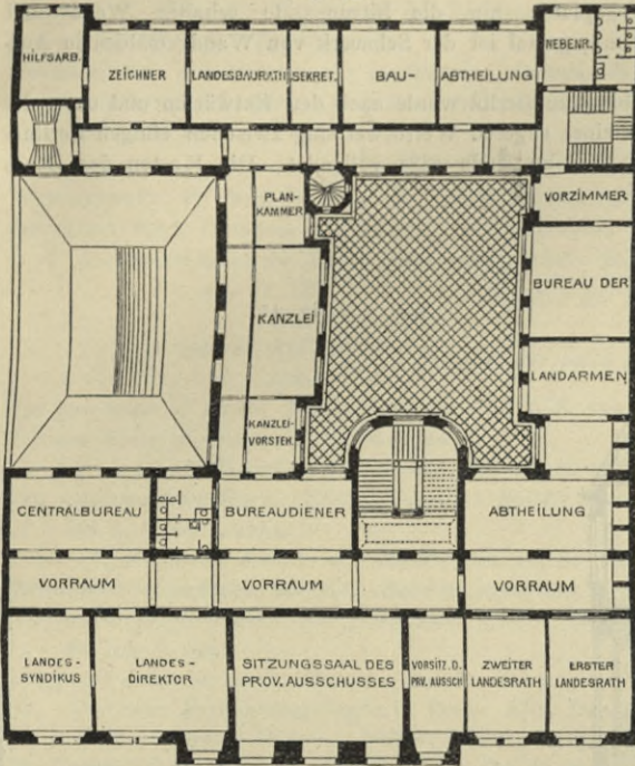
I. Obergeschoß.
