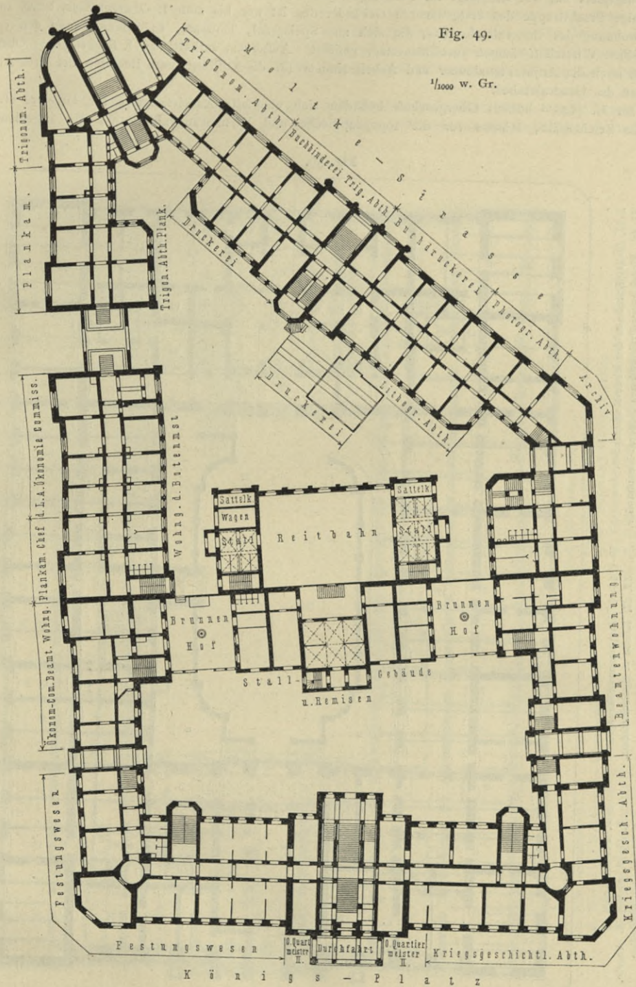
Generalstabs-Dienstgebäude zu Berlin.
