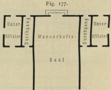
Tolle's Mannschaftspavillon mit Anbauten.
