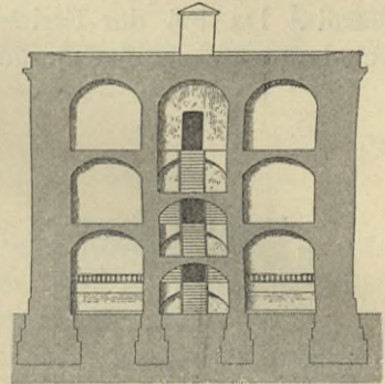
Schnitt I I'.
