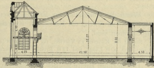
Querschnitt.
