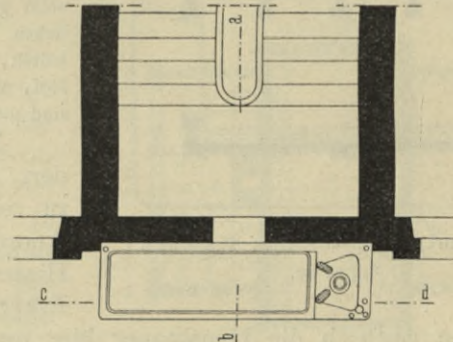
Grundriß.
