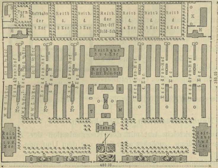
Österreichische Kavallerieregiments-Kaserne 113 ), — 1/5000 w. Gr. Pavillon-System Gruber-Völckner.
