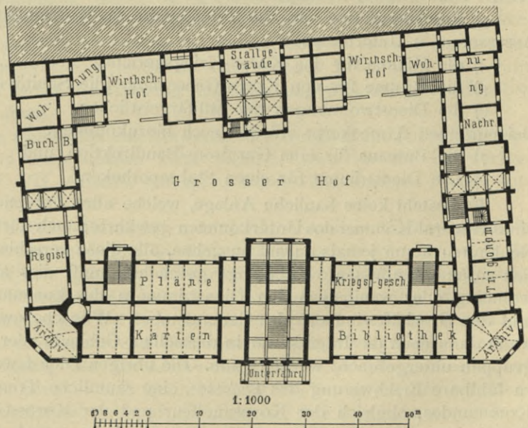
Generalstabs-Gebäude zu Berlin. — Ursprüngliche Anlage 87) . Arch.: Goedeke .
