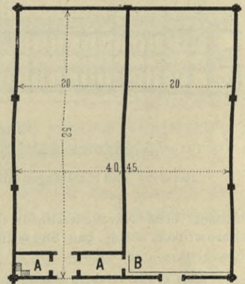
Französisches Reithaus.
