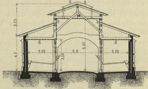
Neueres sächsisches Stallgebäude.
