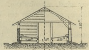
Blockwand- Flechtwerk- Baracke.
