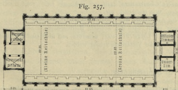
GroÙe gedeckte Reitschule in Österreich-Ungarn 161) .
