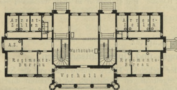
Grundriß.
