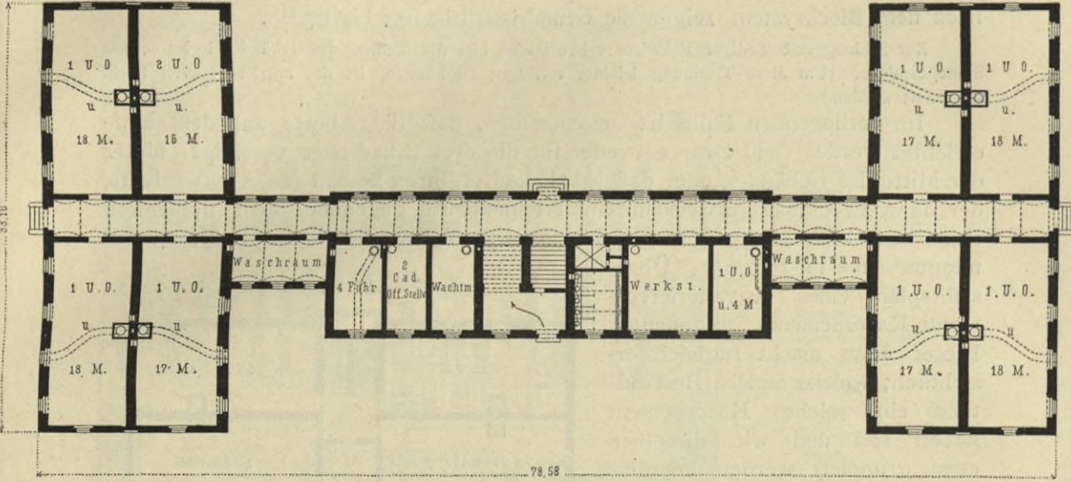
Mannschafts-Wohngebäude für 3 Eskadronen. — Erdgeschoss 142) .
