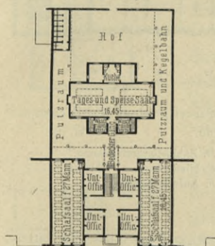
Guillaume's Entwurf für das Kompagniegebiet einer eng- lischen Infanteriekaserne.
