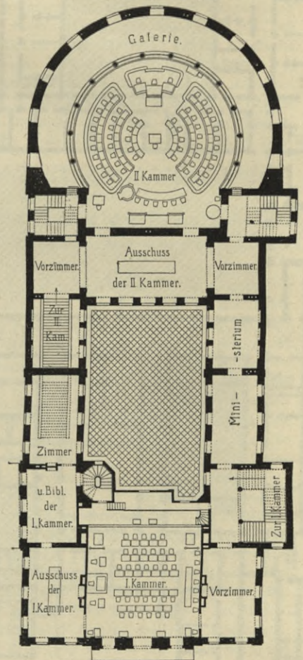
Ständehaus zu Darmstadt 57) . — 1/600 w. Gr. Arch.: Lerch.
