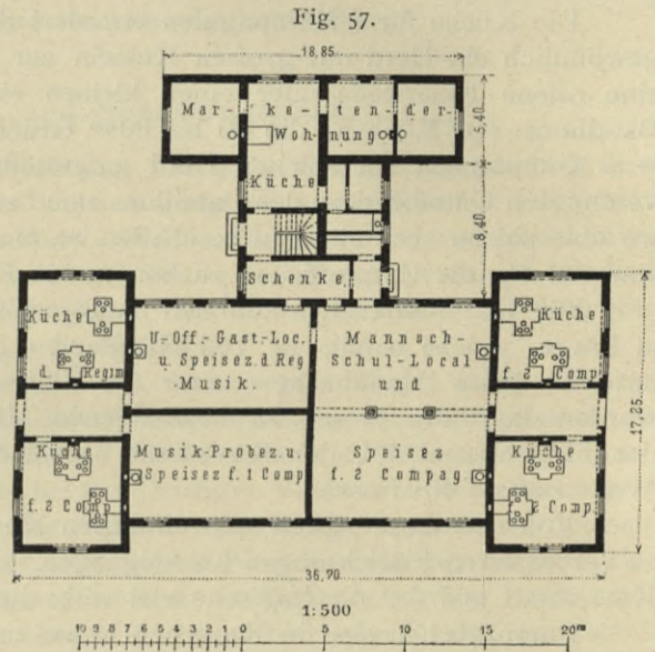
Marketenderei- und Küchengebäude einer österreichischen Regimentskaserne 101) .
