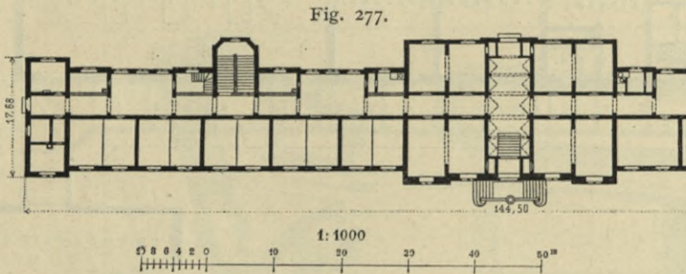
Kadettenhaus zu Dresden.
