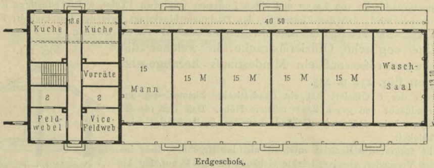
Lager bei Zeithain. Arch.: Portius.
