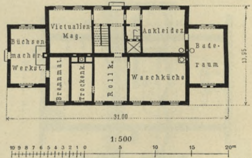
Bade- und Waschküchengebäude einer österreichischen Infanteriekaserne 107) .
