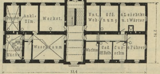
Osterreichische Eskadronkaserne 143) . — 1/600 w. Gr.
