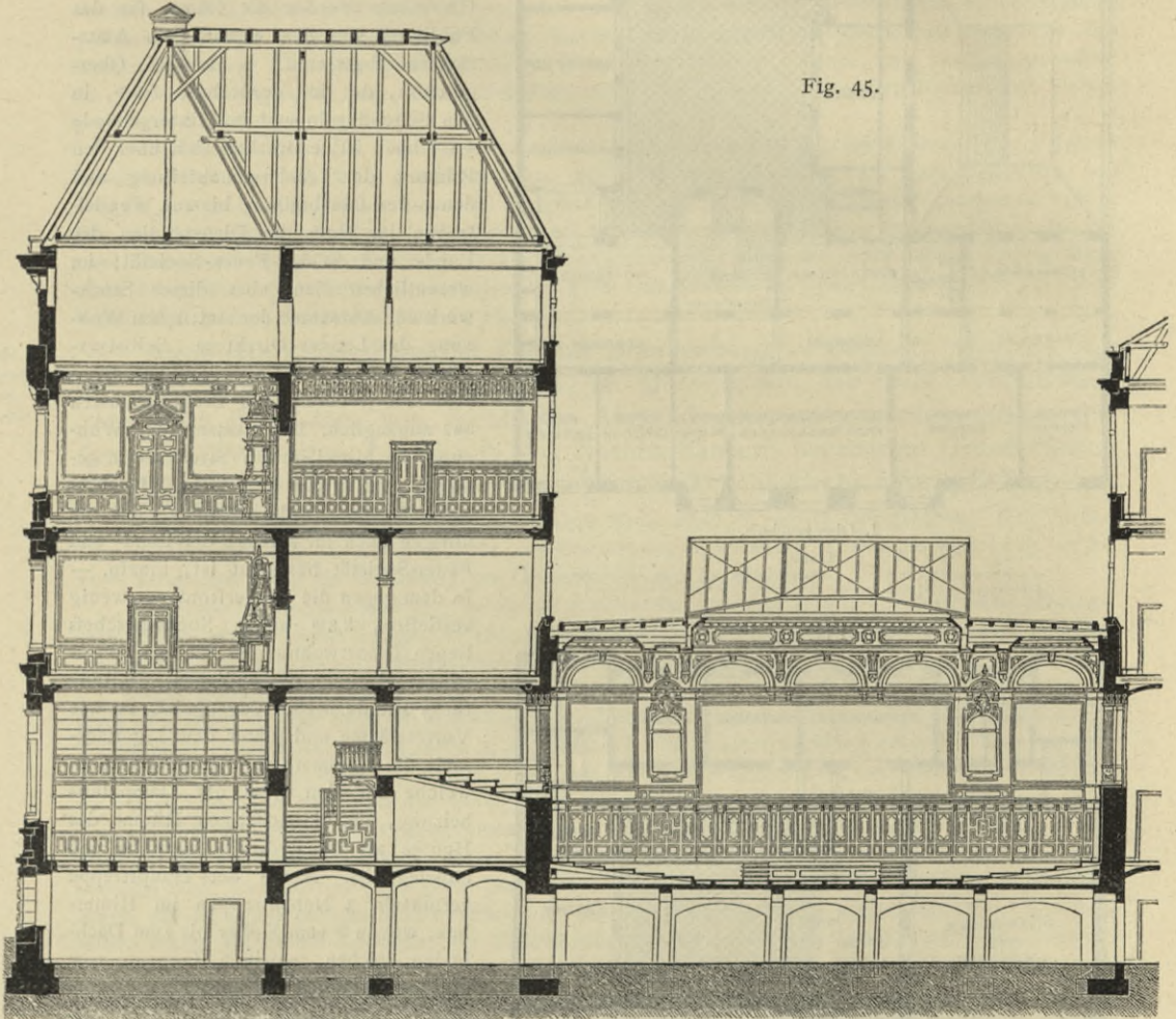
Landeshaus der Provinz Brandenburg zu Berlin. — Querschnitt 84) .
