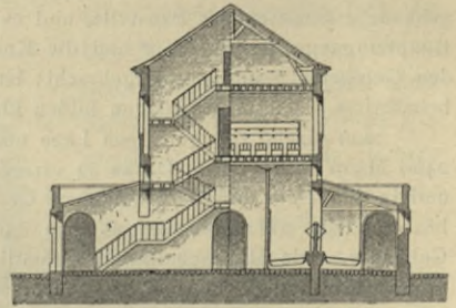
Querschnitt nach CD. — 1/1000 w. Gr.
