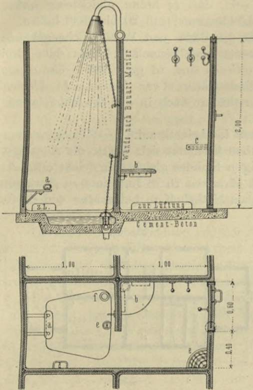
Brausebad von Knoblauch . \frac{1}{65} w. Gr.
