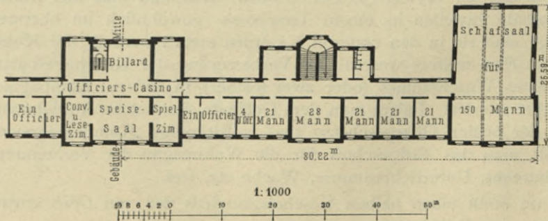
Pionierkaserne zu Dresden. — II. Obergeschoß.
