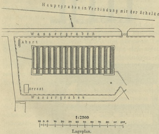
Kaserne der Festung Termonde 152) .
