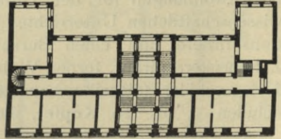
Alte Artillerie- und Ingenieurschule zu Berlin 169 ). — 1/1000 w. Gr.
