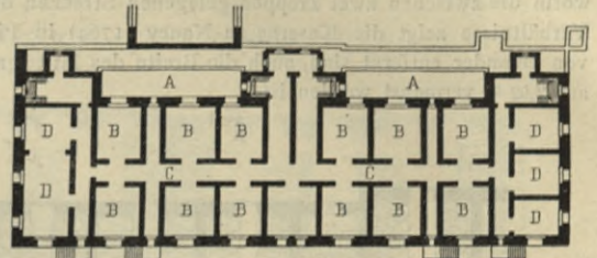
Kaserne im Schloß Edinburg 129) .
