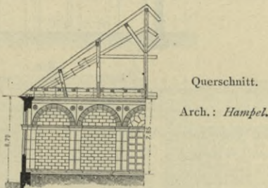
Exerzierhaus bei Berlin 157) .
