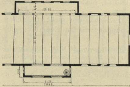
Grundriß.
