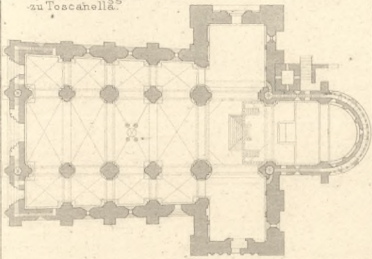
Grundriss zu Fig. 1. 3.
