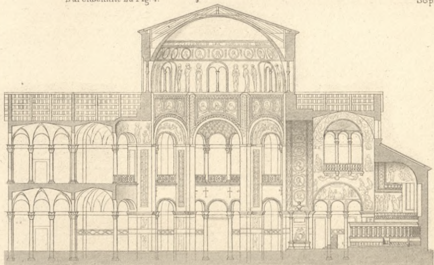
S. Vitale zu Ravenna. 8
