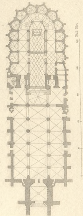
Münster zu Freiburg. Grundriss. 4.
