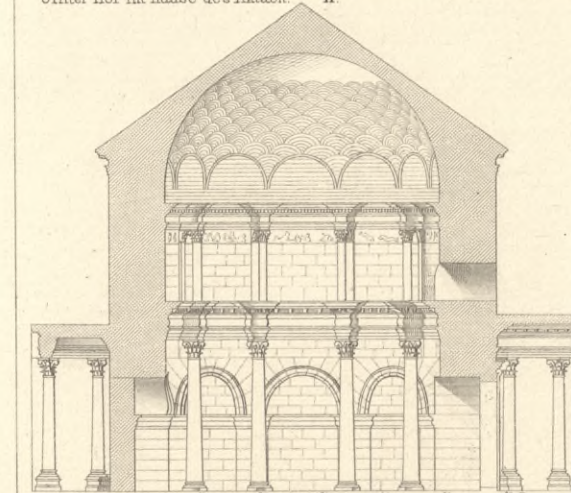
Kuppelsaal im Palast des Diocletian. (Spalatro.)
