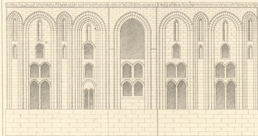
Palast der Kuba bei Palermo.
