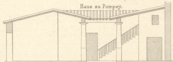
Haus zu Pompeji.
