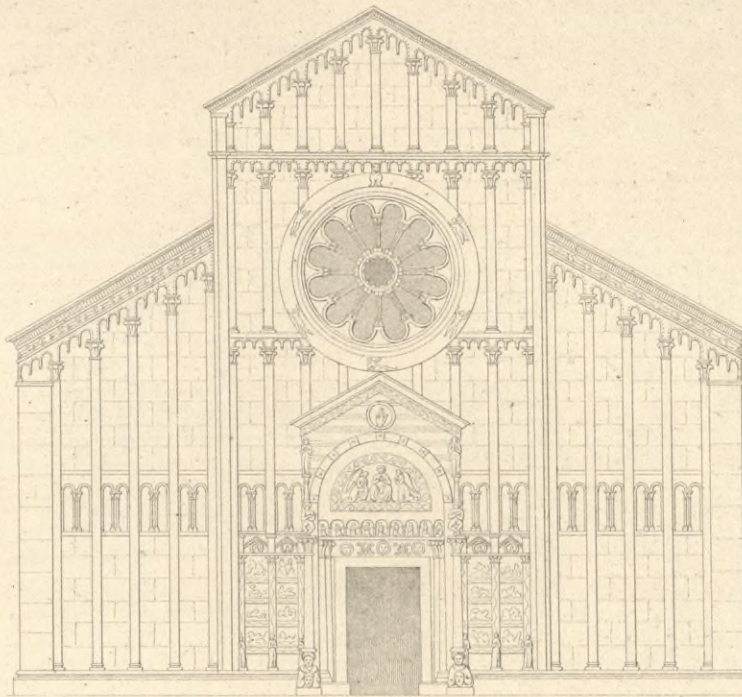
Façade von S. Zeno zu Verona. 3.
