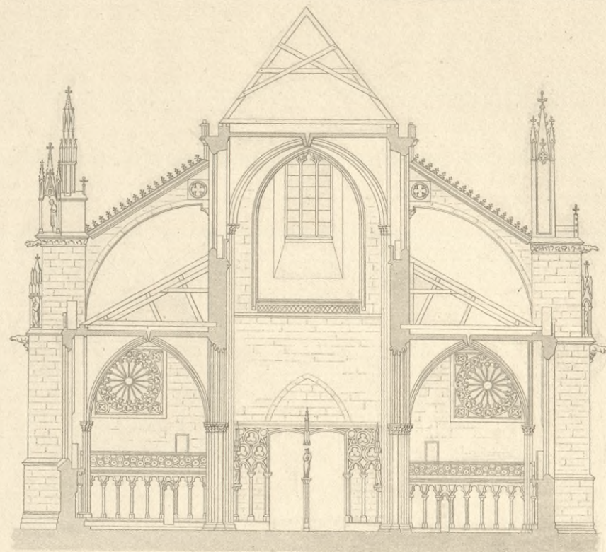
Querschnitt des Münsters zu Freiburg 3.
