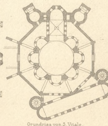
Grundriss von S. Vitale. 9
