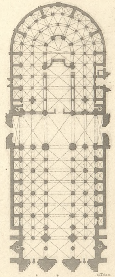
Grundr. zu Fig. 1. 2.
