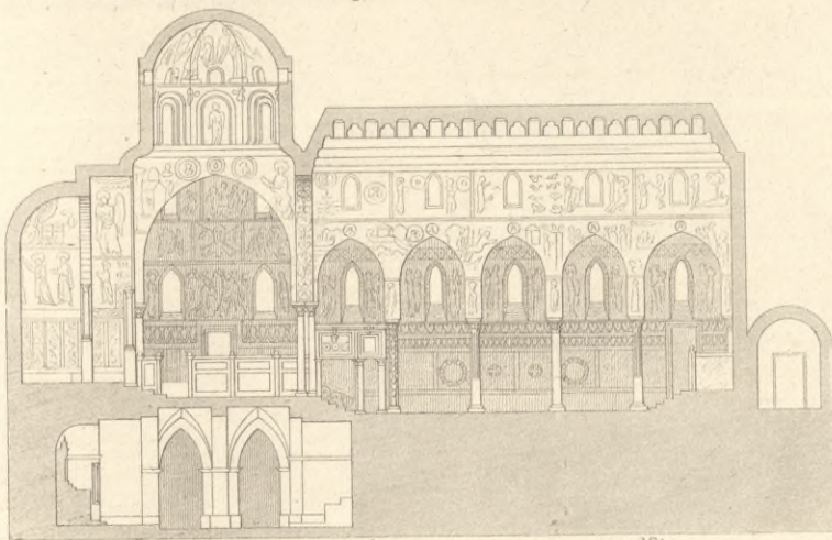
Capella Palatina zu Palermo. 5.
