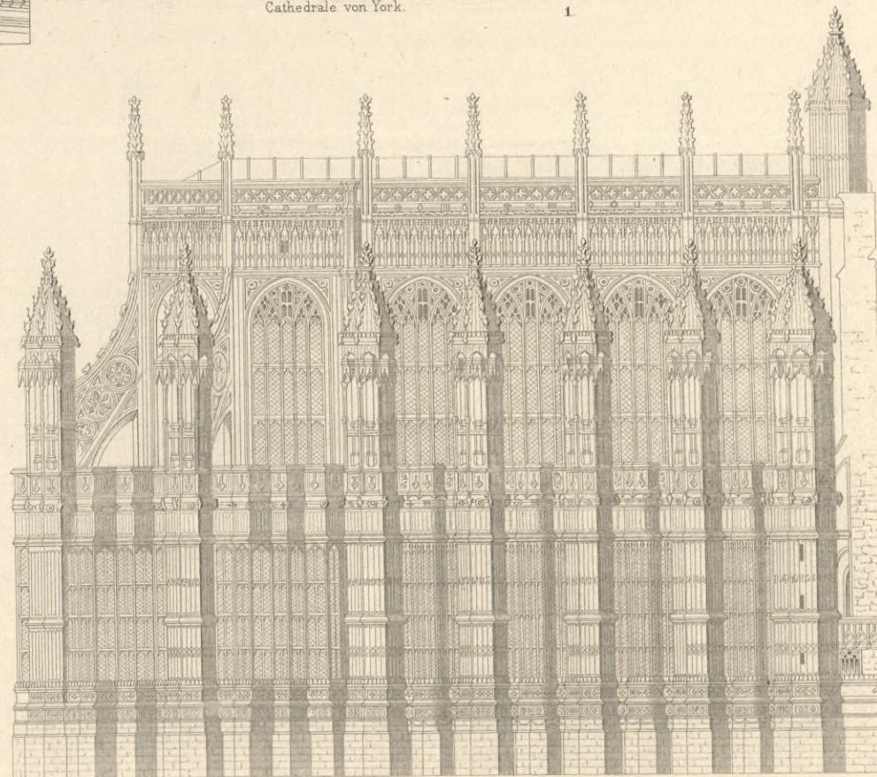
Aufriß der Capelle Heinrichs VII. Westminster.
