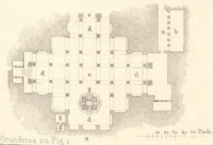
Grundriss zu Fig. 1
