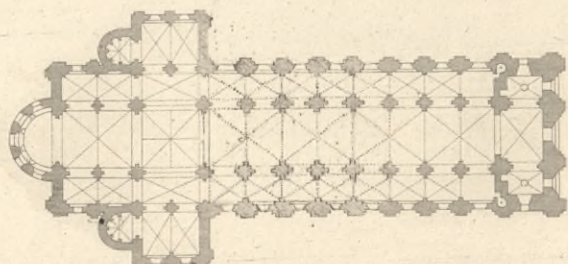
S. Etienne zu Caen. 10.
