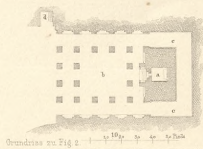
Grundriss zu Fig. 2
