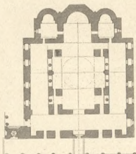
S. Sophia. Thessalonica.
