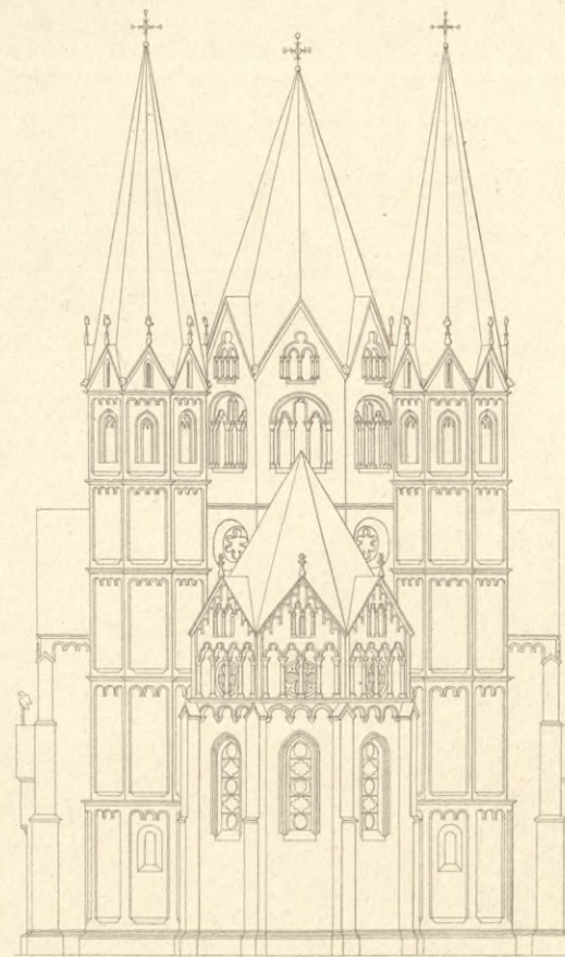
Kirche zu Gelnhausen. 7.
