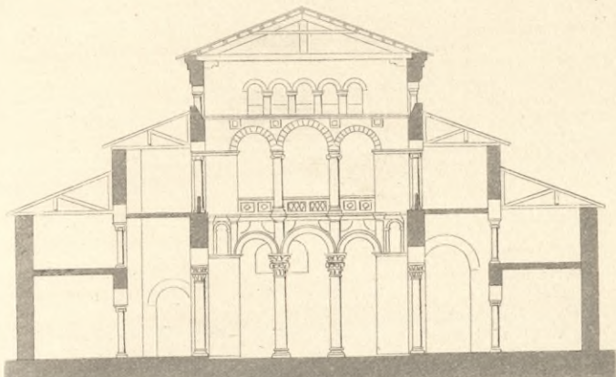
S. Demetrius. Thessalonica.
