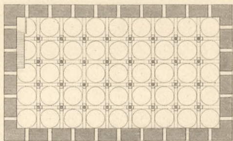
Cisterne bei Constantinopel. (Grundr.) 4
