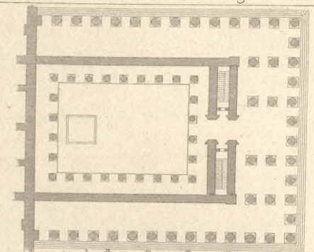
4. Grundr. Fig. 3.
