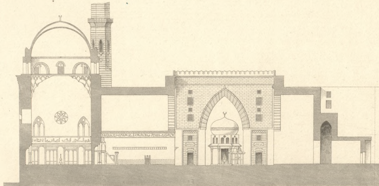
Moschee des Sultans Hassan zu Kairo.
