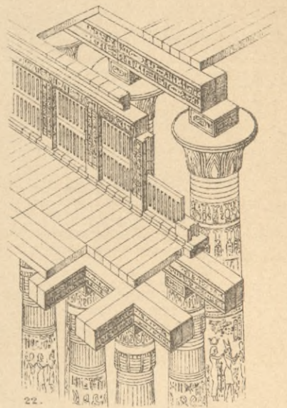
22. Attika des Tempels von Karnak.
