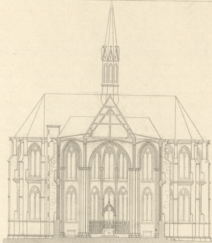
Querschnitt der Elisabethkirche zu Marburg 6.
