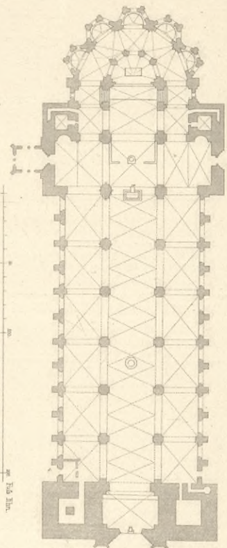
Dom zu Magdeburg. 5.
