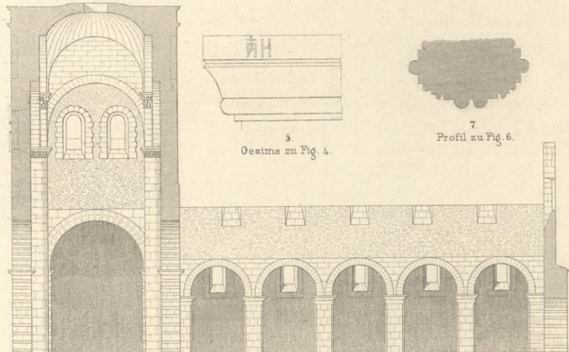
S. Martin zu Angers.
