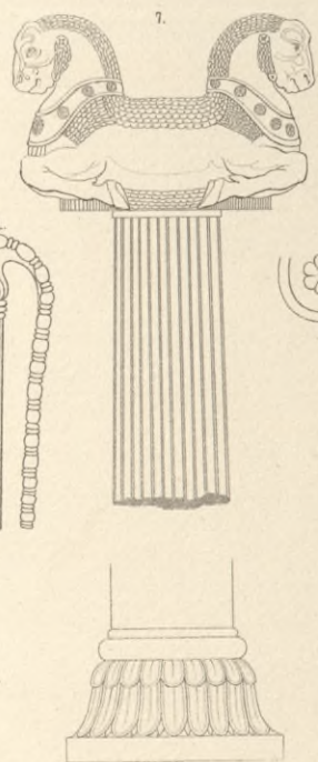
7. 13. 6-15. Details von den Säulen zu Persepolis
