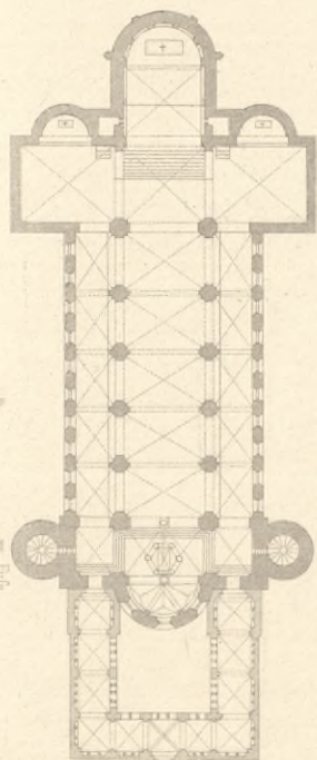
Grundr. der Kirche zu Laach. 2.
