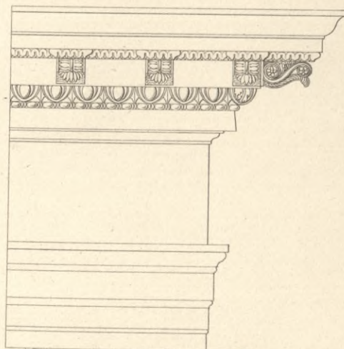
Pantheon. (Aufriss.) 5
