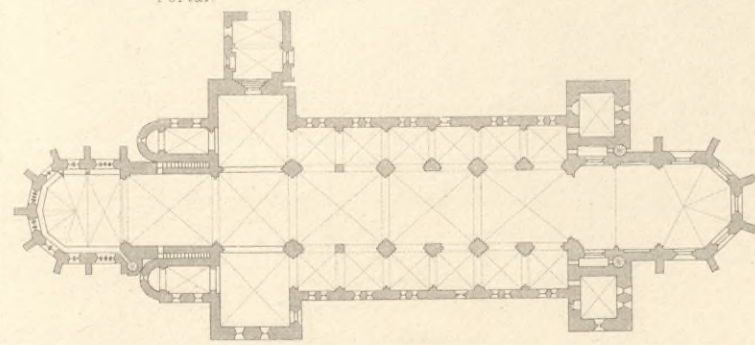
Grundr. des Doms zu Naumburg. 5
