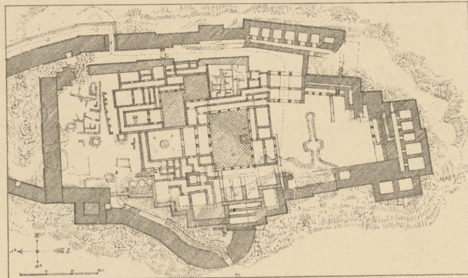
22. Plan der Burg von Tiryns.
