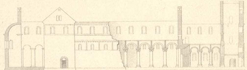
Kirche zu Paulinzelle. 2
