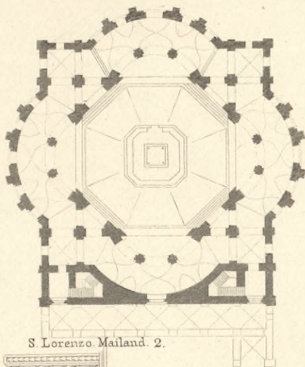
S. Lorenzo, Mailand.
