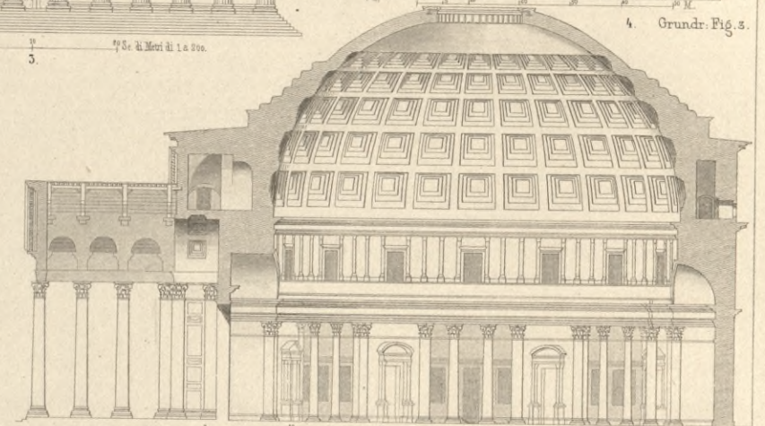
6. Pantheon. (Durchschnitt.)
