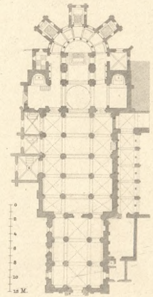
S. Philibert. Tournus. 6.
