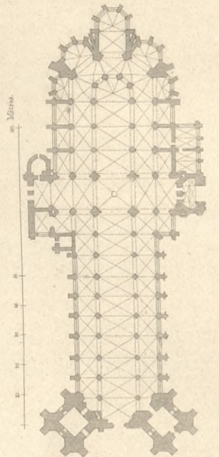
S. Ouen zu Rouen. Grundriss. 3
