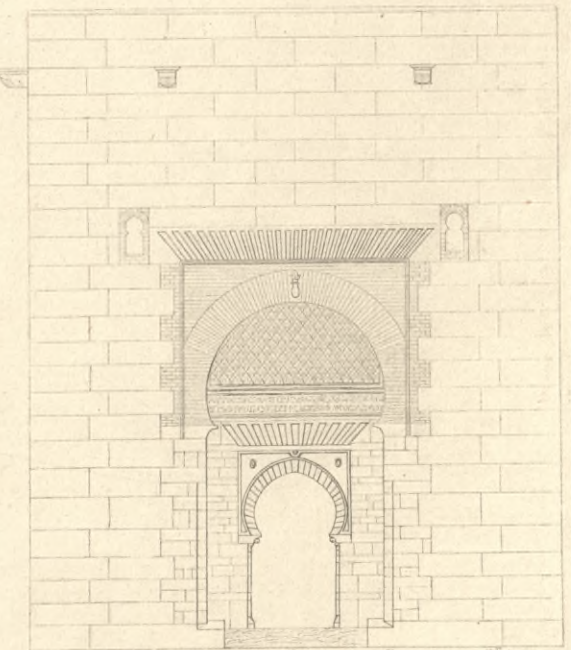
Thor der Alhambra. 12.
