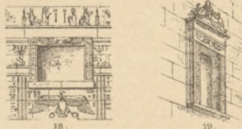
18-19. Fenster des Königspavillons von Medinet-Habu.
