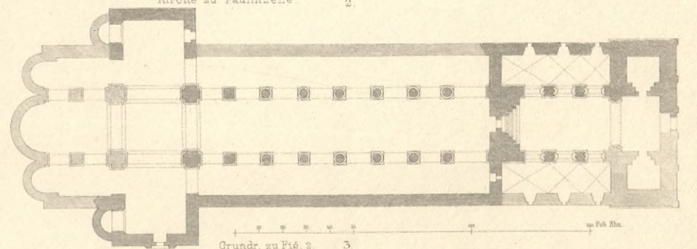
Grundr. zu Fig. 2. 3
