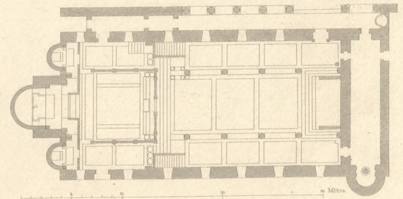
Grundriss zu Fig. 5.
