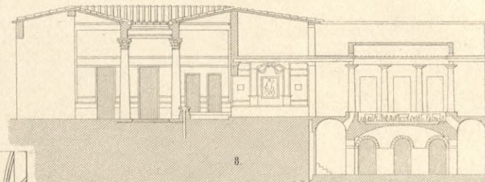
Haus zu Pompeji. 1 2 3 4 5 6 7 8 9 10 11 12 13 14 15 16 17 18 19 20 21 22 23 24 25 26 27 28 29 30 31 32 33 34 35 P.
