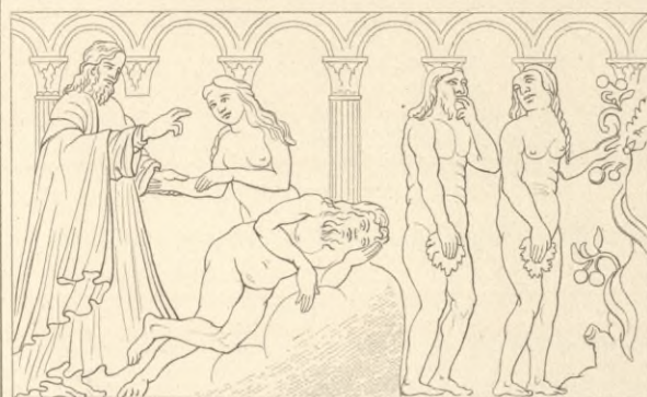
Rel. vom Dom zu Modena. 1.
