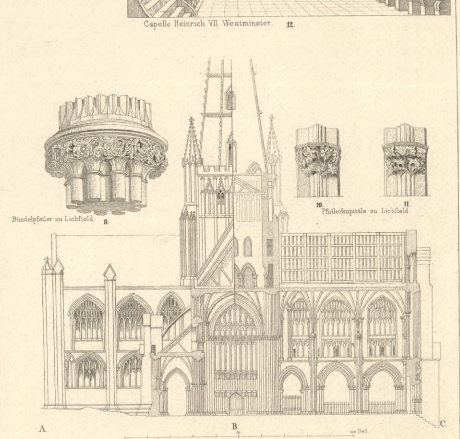
Querschnitt der Cathr. von Lichfield. 8
