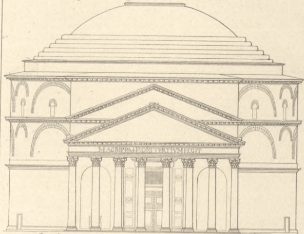
Pantheon. (Aufriss.) 5
