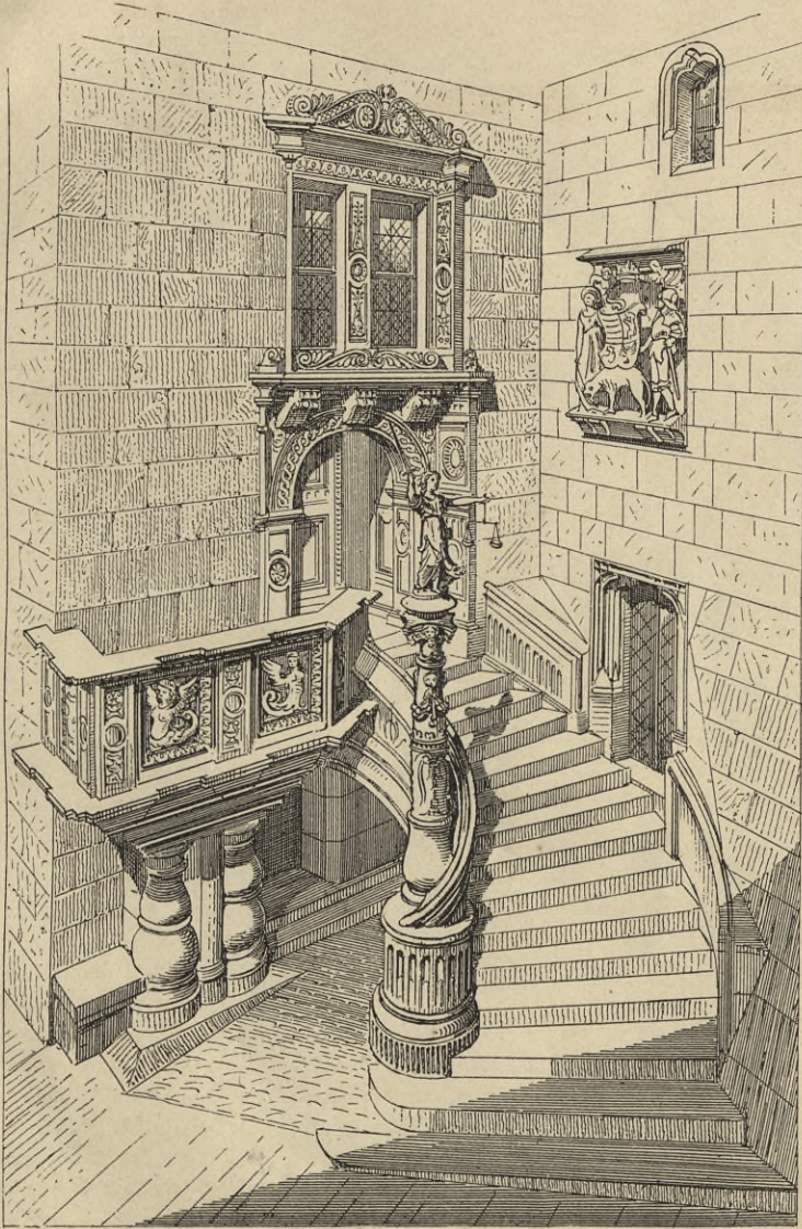
Vom Rathhaus zu Görlitz.
