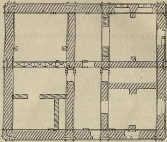
Fig. 104. Grundrifs.
