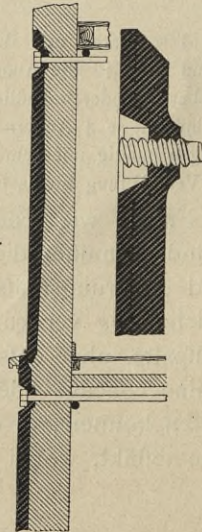
Fig. 115. Verankerungsplatten für die Zwischenmauern.
