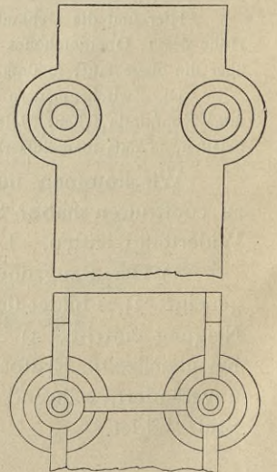
Fig. 115. Verankerungsplatten für die Zwischenmauern.
