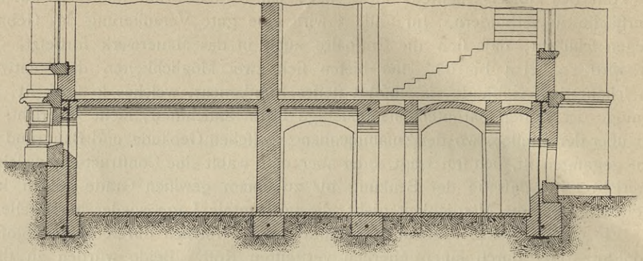
Vom Landgerichtsgebäude in Essen. — \frac{1}{250} n. Gr.
