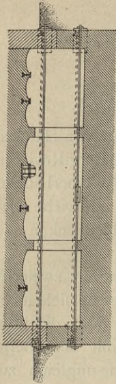
Fig. 103. Querschnitt.
