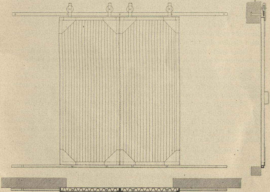
Eisernes Schiebethor von Hein, Lehmann & Co. in Berlin. 1/30 n. Gr.
