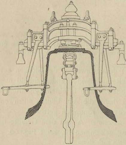
Pozdech'sche Glocken-Armierung.
