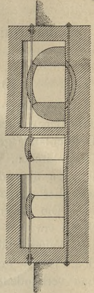
Fig. 105. Querschnitt.
