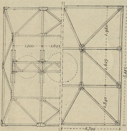
Glockenstuhl zu Neuenkirchen. 1/100 n. Gr.
