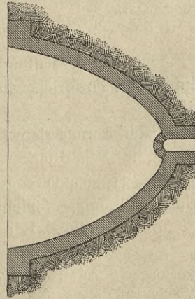
Gemauerte Eisgrube. — \frac{1}{400} n. Gr.
