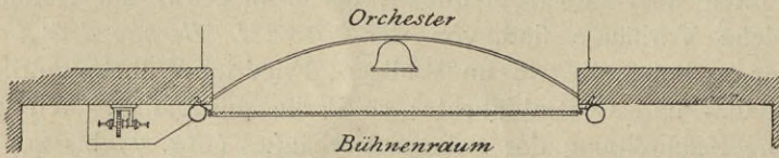
Eiferner Schutzvorhang im Stadttheater zu Pofen.
