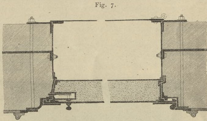
Trefor-Eingang mit Cassenschrank-Thür von Carl Ade in Stuttgart 9) .
