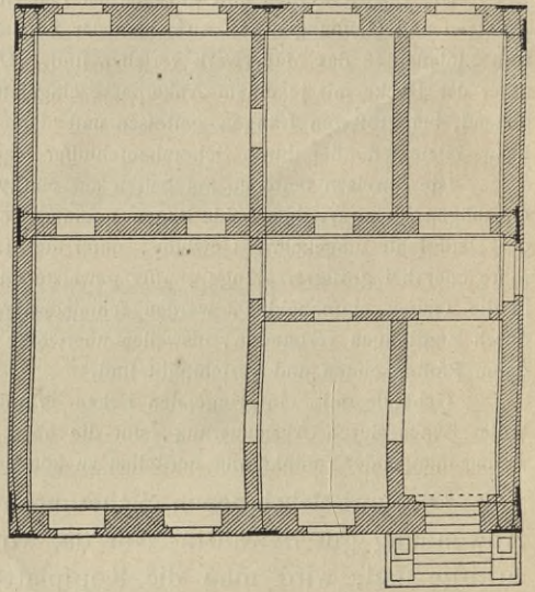
Fig. 114. Grundriss des Erdgefchoffes.
