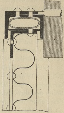
Hydraulische Dichtung am Schutzvorhang im Stadttheater zu Hamburg. — 1/8 n. Gr.
