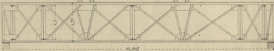
Glocken-Gebälk der Katharinen-Kirche zu Osnabrück.
