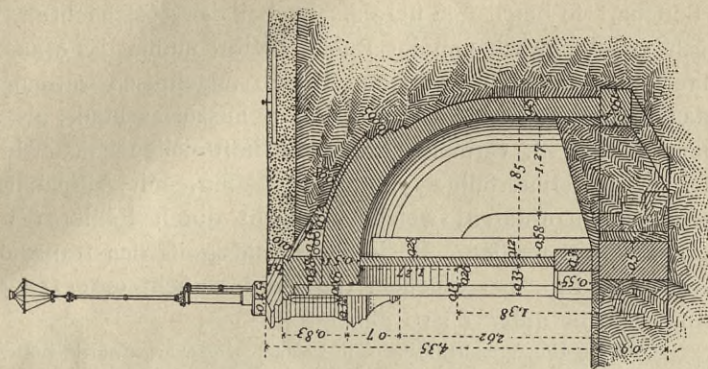
Fig. 147 Querschnitt.
