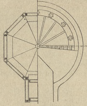
Hölzerne Eisgrube in Nachrodt 207). \frac{1}{1000} n. Gr.
