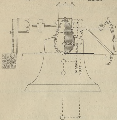
Ritter's Glocken-Aufhängung.
