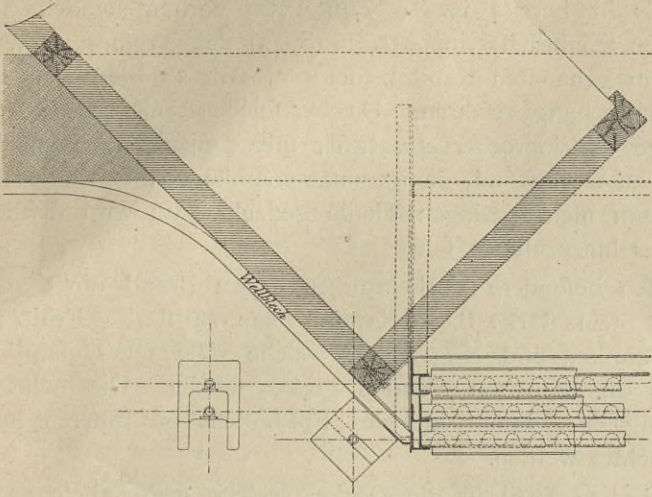
Grundriß-Detail vom Schutzvorhang des Walhalla-Theaters zu Berlin. 1/30 n. Gr.
