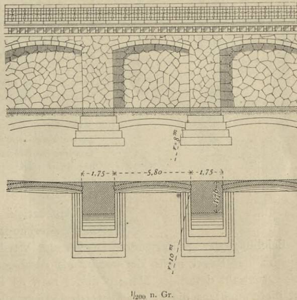
Stützmauer am Bahnhof Malsfeld 161) .
