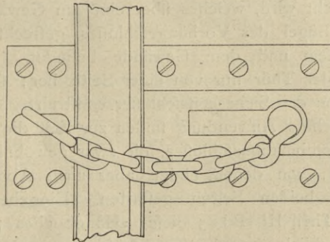
Sicherheitskette 10) . — ca. 1/5 n. Gr.
