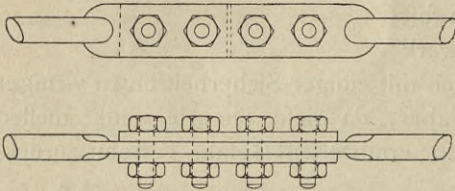
Fig. 107. Fester Zuganker.
