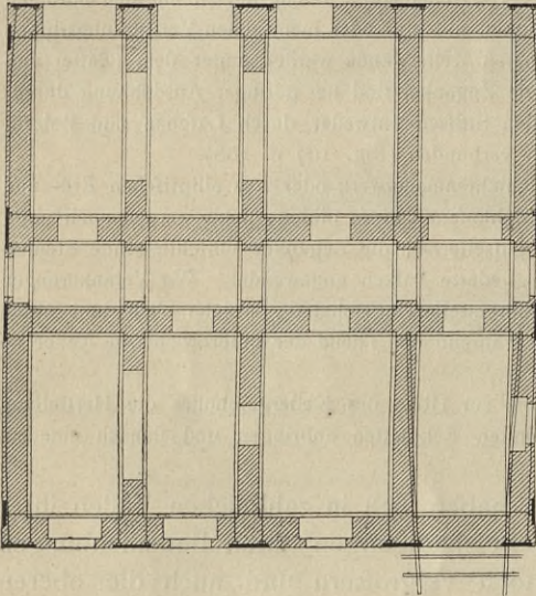
Fig. 113. Grundriss des Kellergefchoffes.
