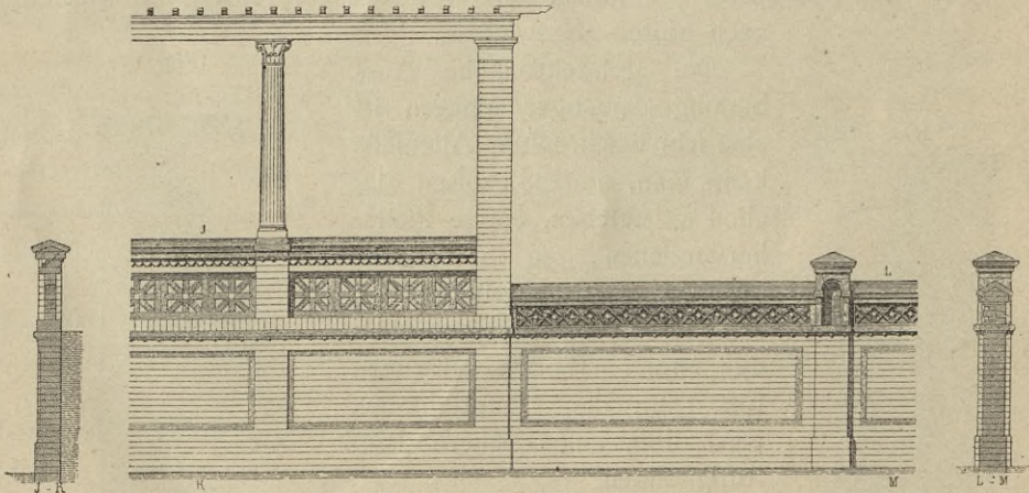
Von der Villa v. d. Heydt bei Berlin 159) , ca. \frac{1}{100} n. Gr.
