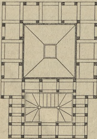
Eishaus auf dem Rittergut Lagowitz bei Schwiebus 215) . \frac{1}{4} 150 n. Gr.
