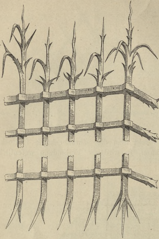
Ebenes Korbgiitter 28) .
