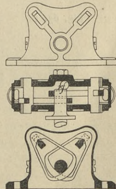
Bochumer Glockenlager 85) .
