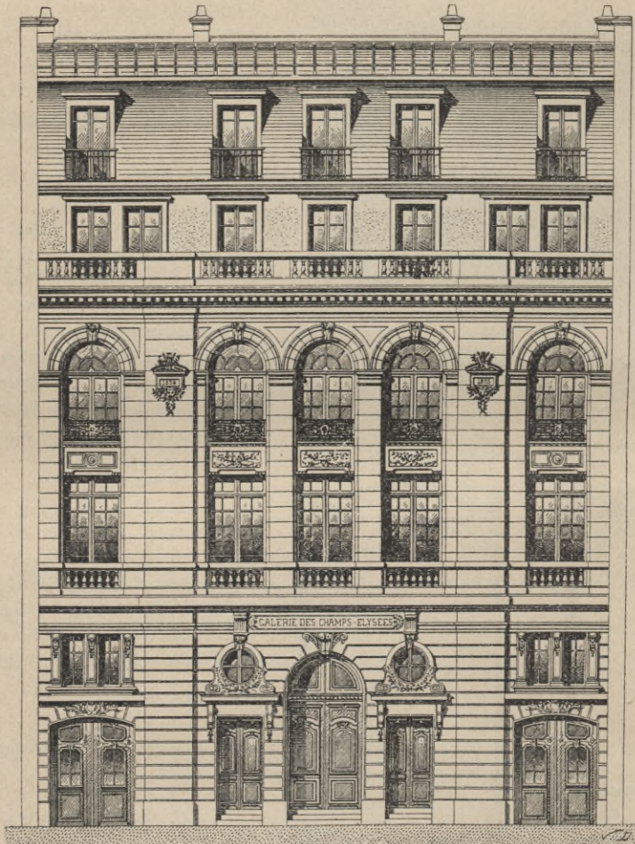
1:200 10 5 0 1 2 3 4 5 6 7 8 9 10 m Saalbau »Galerie des Champs-Elysées« zu Paris 198) . Arch.: Viennois.
