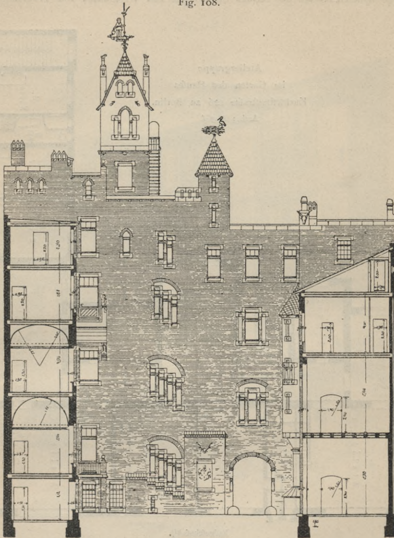
Querschnitt 61) .
