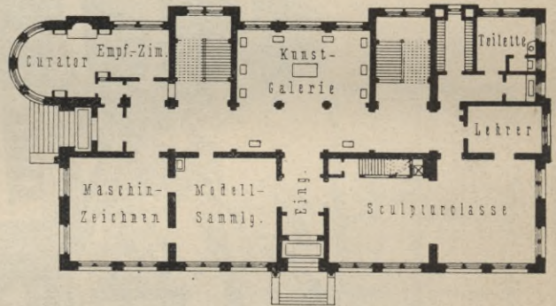
I. Obergeschoßes 98 ). Normal-Kunstschule zu Boston. Arch.: Hartwell & Richardson .
