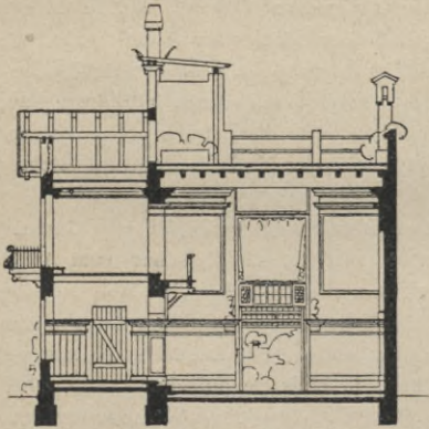
Schnitt durch das Atelier.
