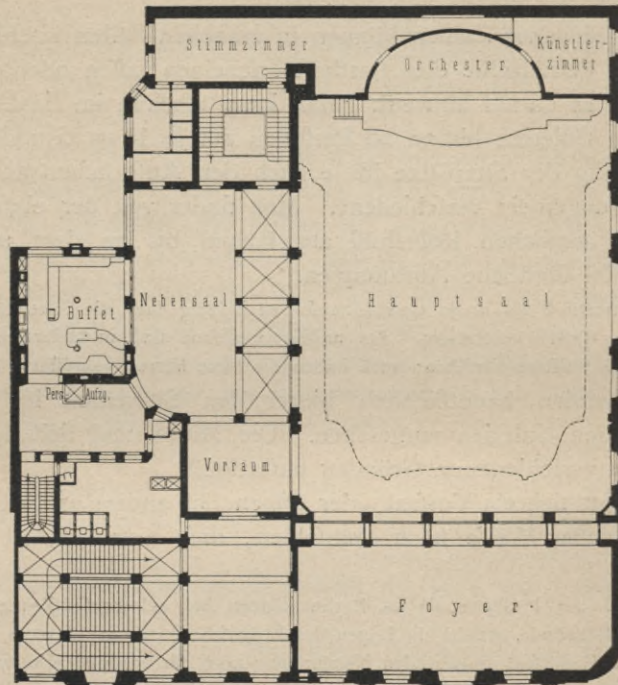
Saalgefchofs 180) .
