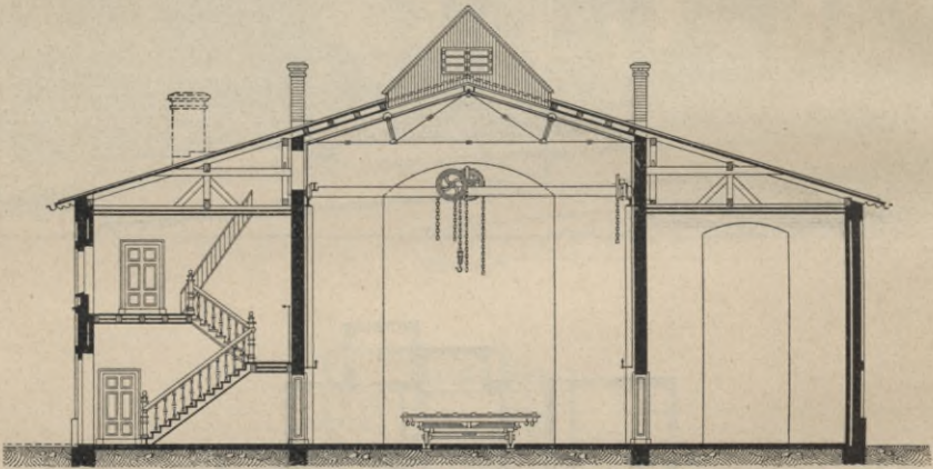
Längenschnitt.
