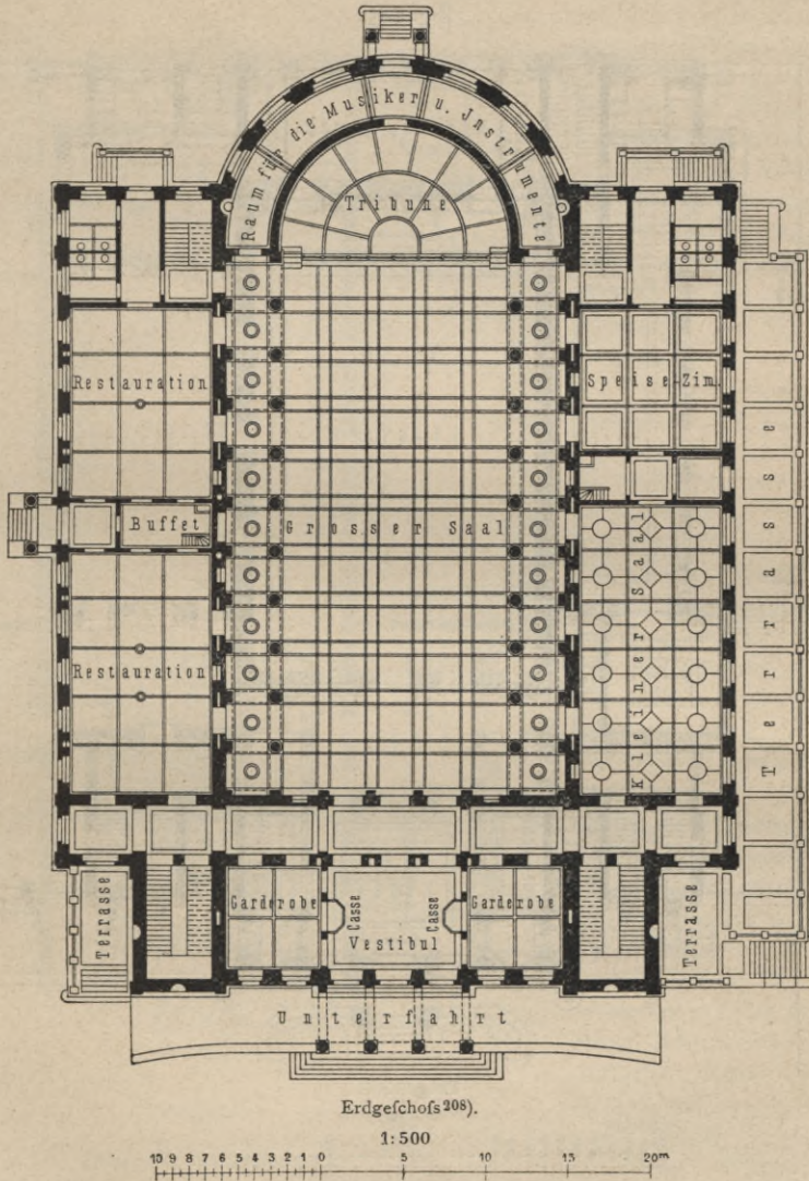
Saalbau zu Neustadt a. H.
