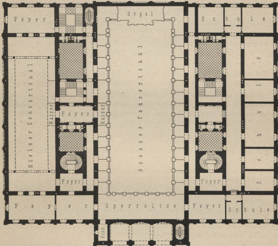
II. Obergeschoß 179) .
