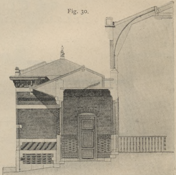
Querschnitt.
