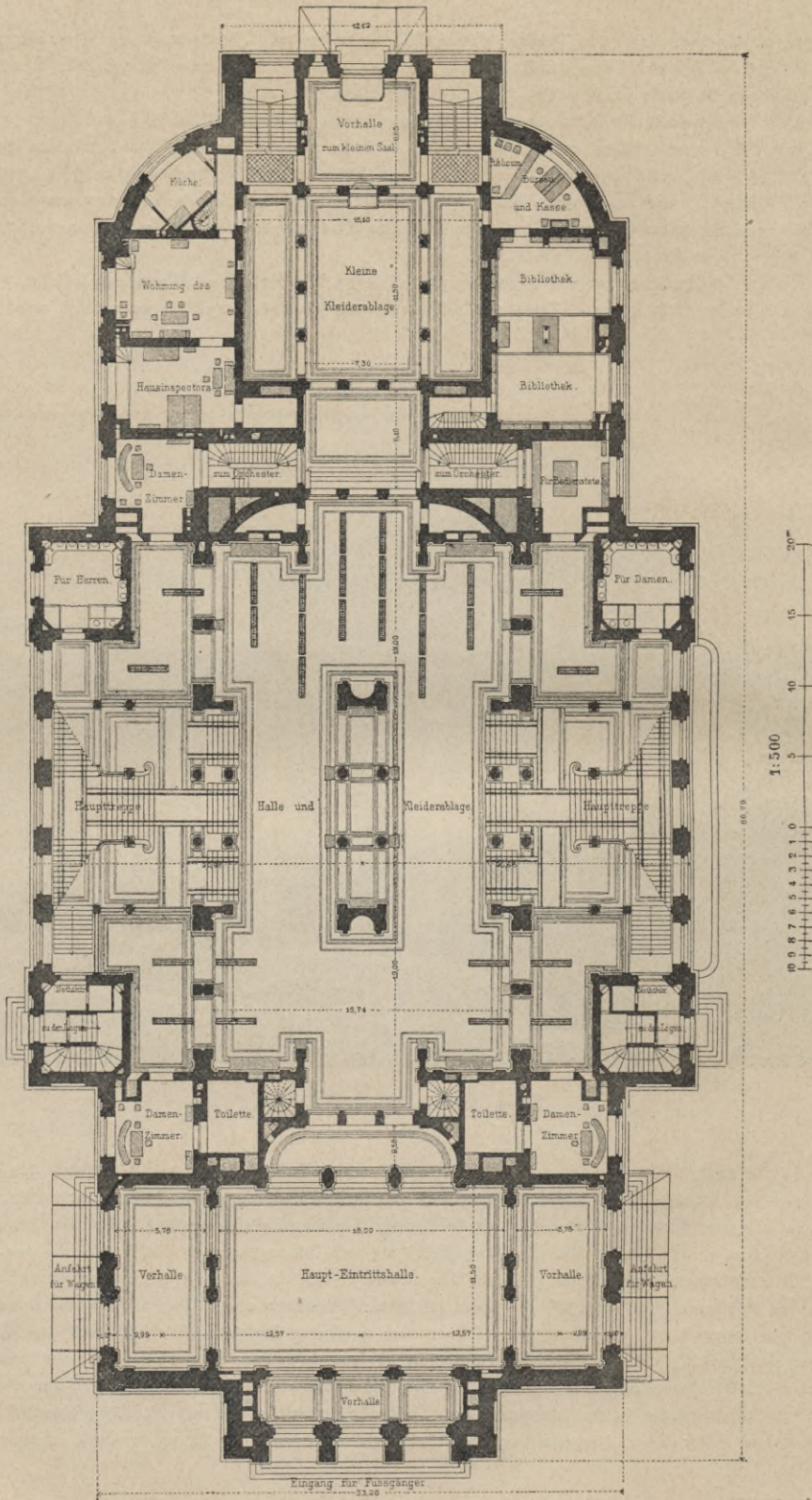
Fig. 276. Grundriß des Erdgeschosses.
