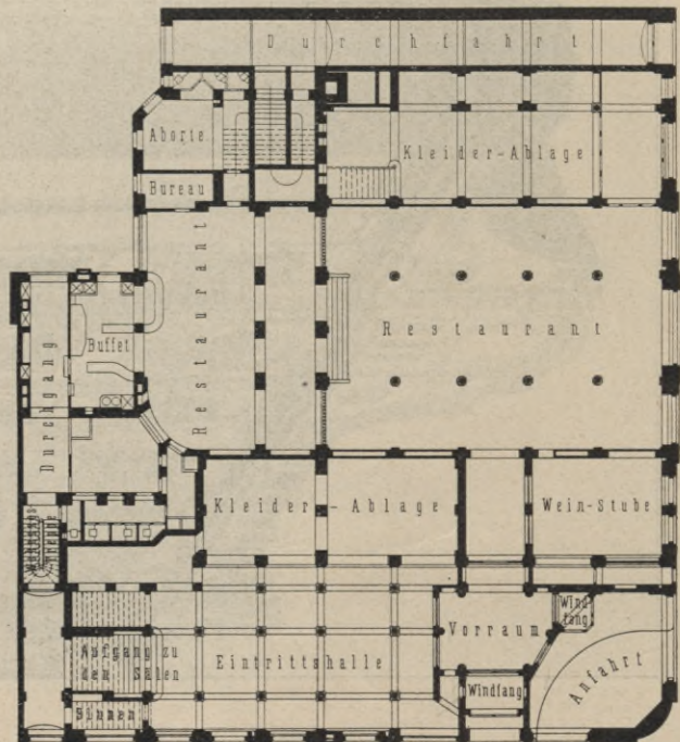
Erdgeschoß.
