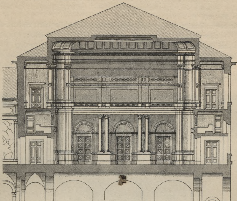
Querschnitt 159).
