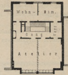
I. Obergeschoss, 1/500 w. Gr.
