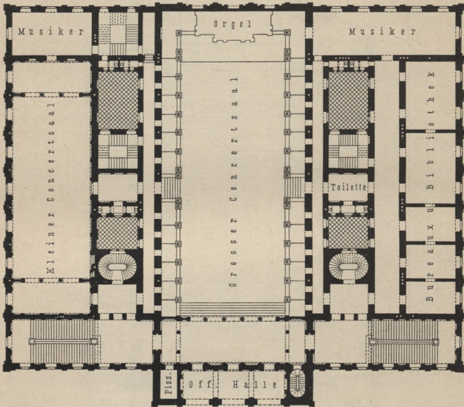
I. Obergeschoss 179).
