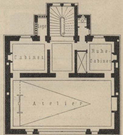
Grundriss des Obergeschosses zu Fig. 48 u. 49 23 ). \frac{1}{250} w. Gr.
