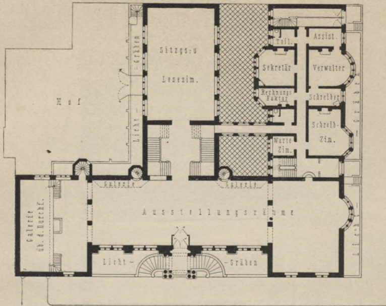
Erdgeschoss 128) .
