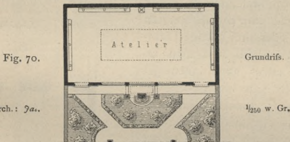
Atelier des Malers Jollivet in der Cité Malesherbes bei Paris 36) .
