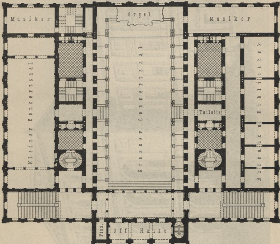
I. Obergefchofs.
