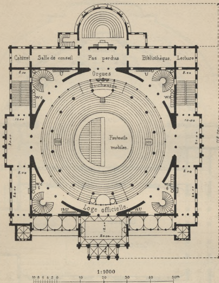
Oppermann's Entwurf für einen großen Versammlungsfaal 152 , (10000 Personen.)
