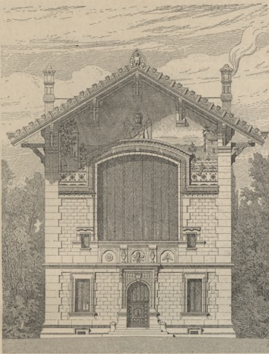
Anfsicht.
