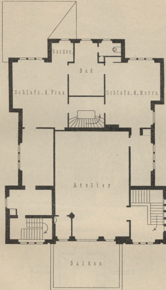
Obergeschoss zu Fig. 51.
