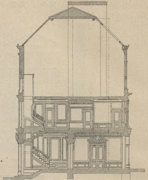
Querschnitt.
