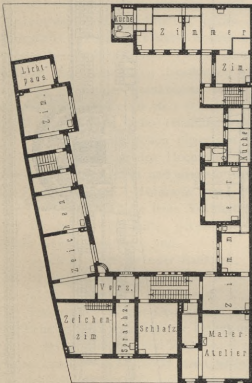
II. Obergeschoss 60 ).
