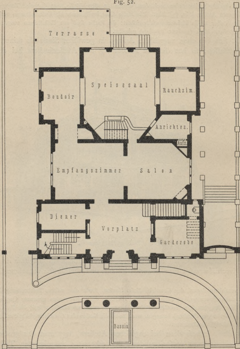
Erdgefchofs zu Fig. 51.
