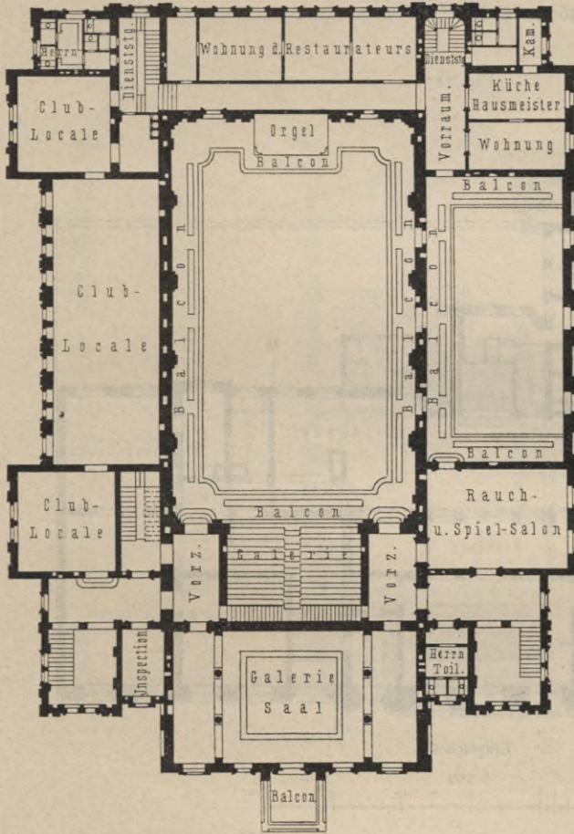
Obergeschoss.
