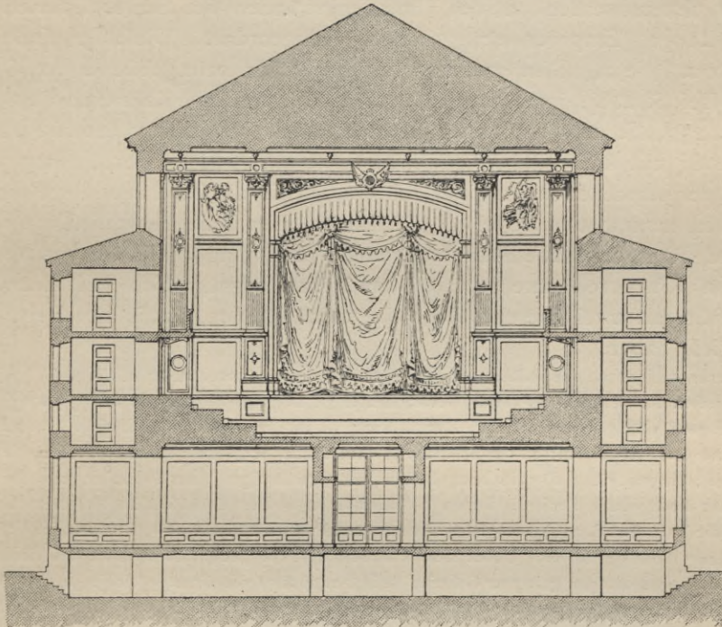
Querchnitt durch den Saal 164) .
