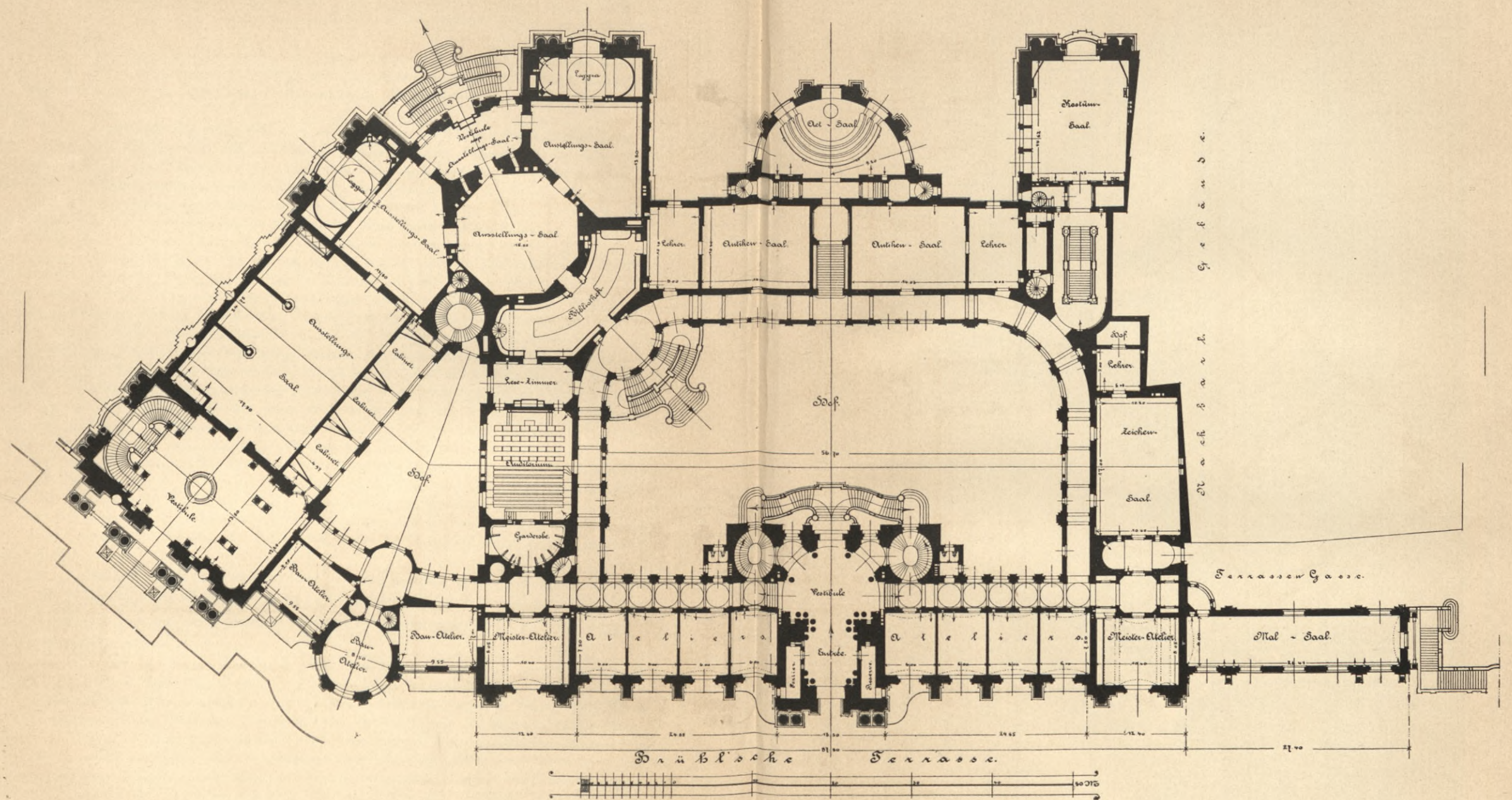
Kunstakademie- und Kunstausstellungsgebäude zu Dresden.
