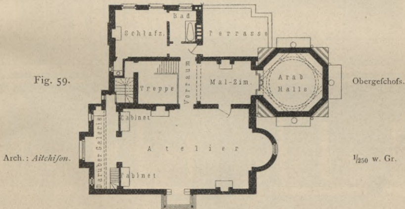
Atelier des Malers Leighton zu Kenfington 30) .
