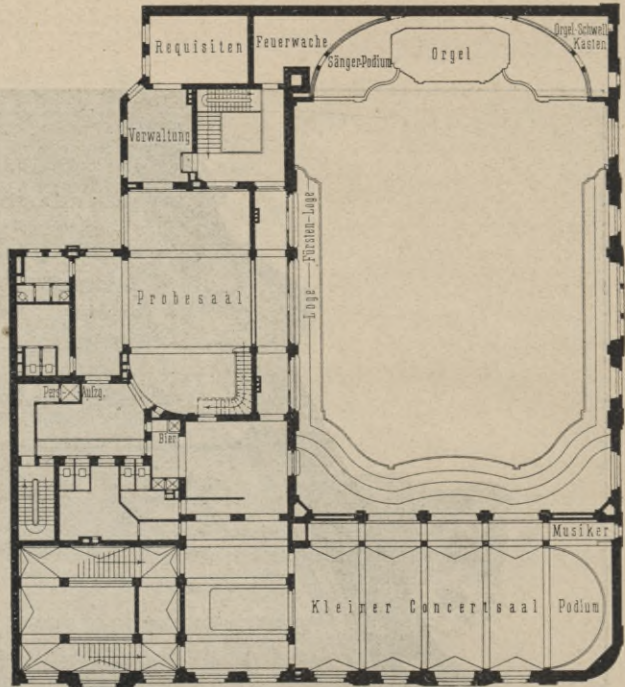
Galeriegeschoß.
