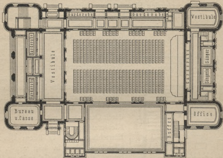
Erdgeschoss 187) .
