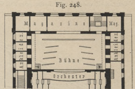
Bühne im Kassinogebäude zu Kopenhagen 176 ). 1/600 w. Gr.
