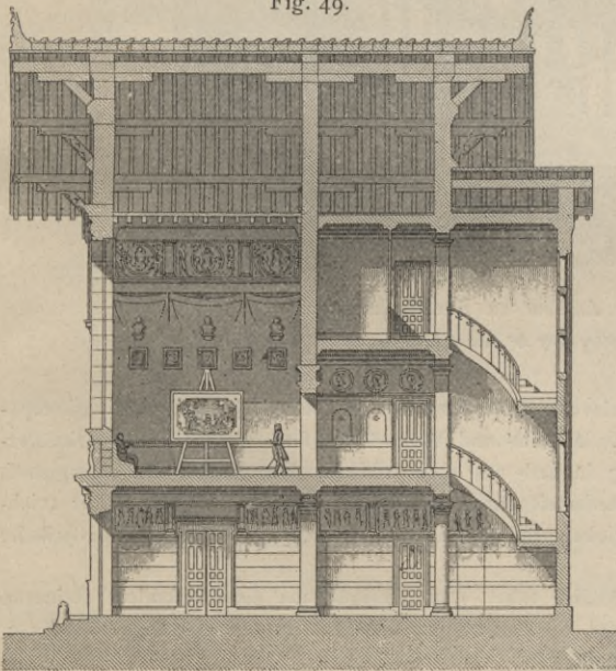
Querchnitt.
