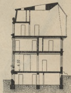
Querschnitt. — 1/500 w. Gr.
