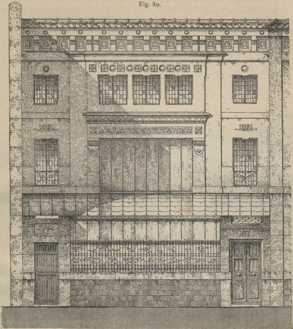
Ansicht. — \frac{1}{125} w. Gr.
