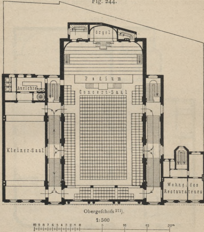
Konzerthaus des Vereins Liedertafel zu Mainz.
