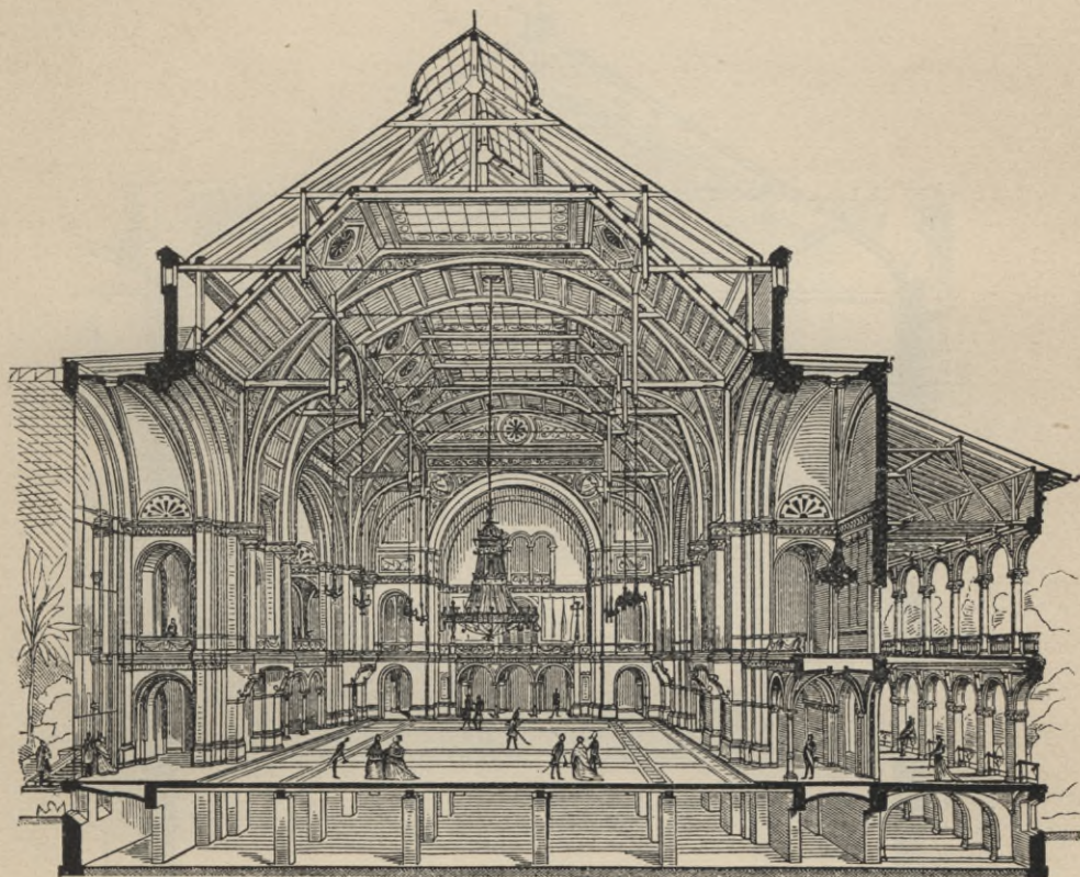
Querschnitt 162).
