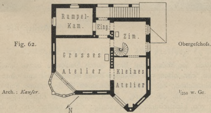
Malerheim des Fräulein Konck zu Budapest 32) .
