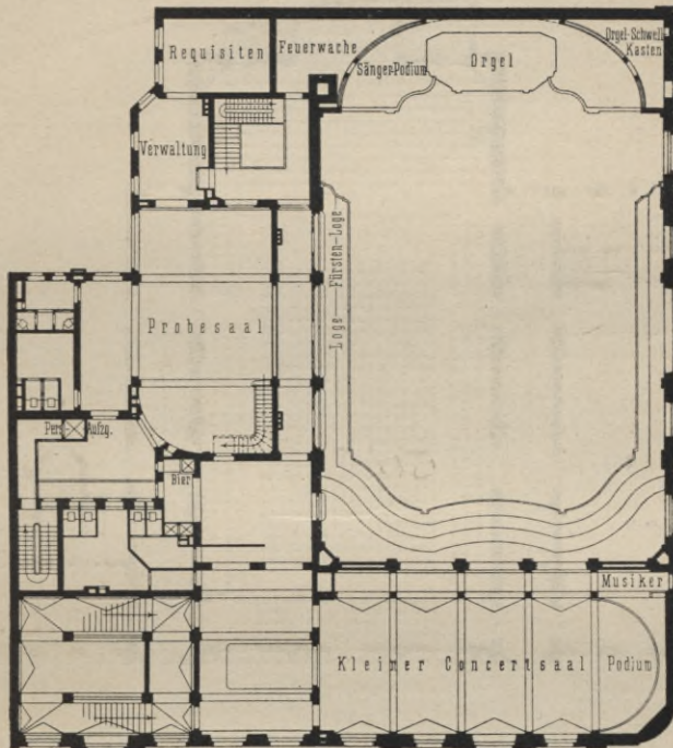
Galeriegeschoss 170) .
